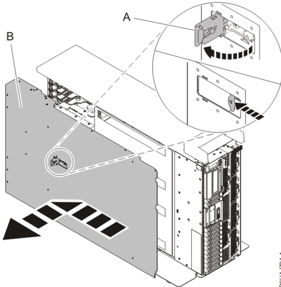
Abbildung 23. Serviceabdeckung ausbauen
