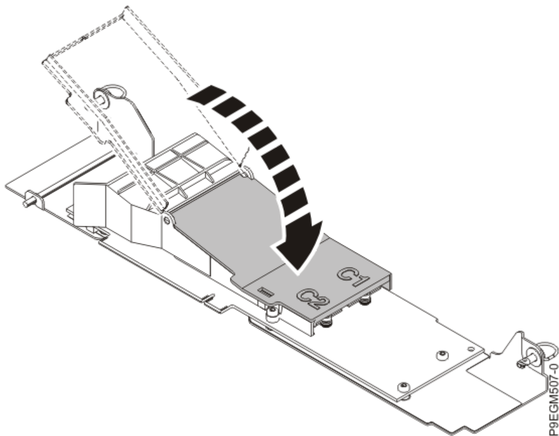
Abbildung 10. Schwarze Abdeckung der NVMe M.2-Trägerkarte schließen
