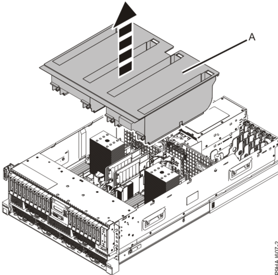
Abbildung 24. Luftführung aus einem Einschubsystem ausbauen
