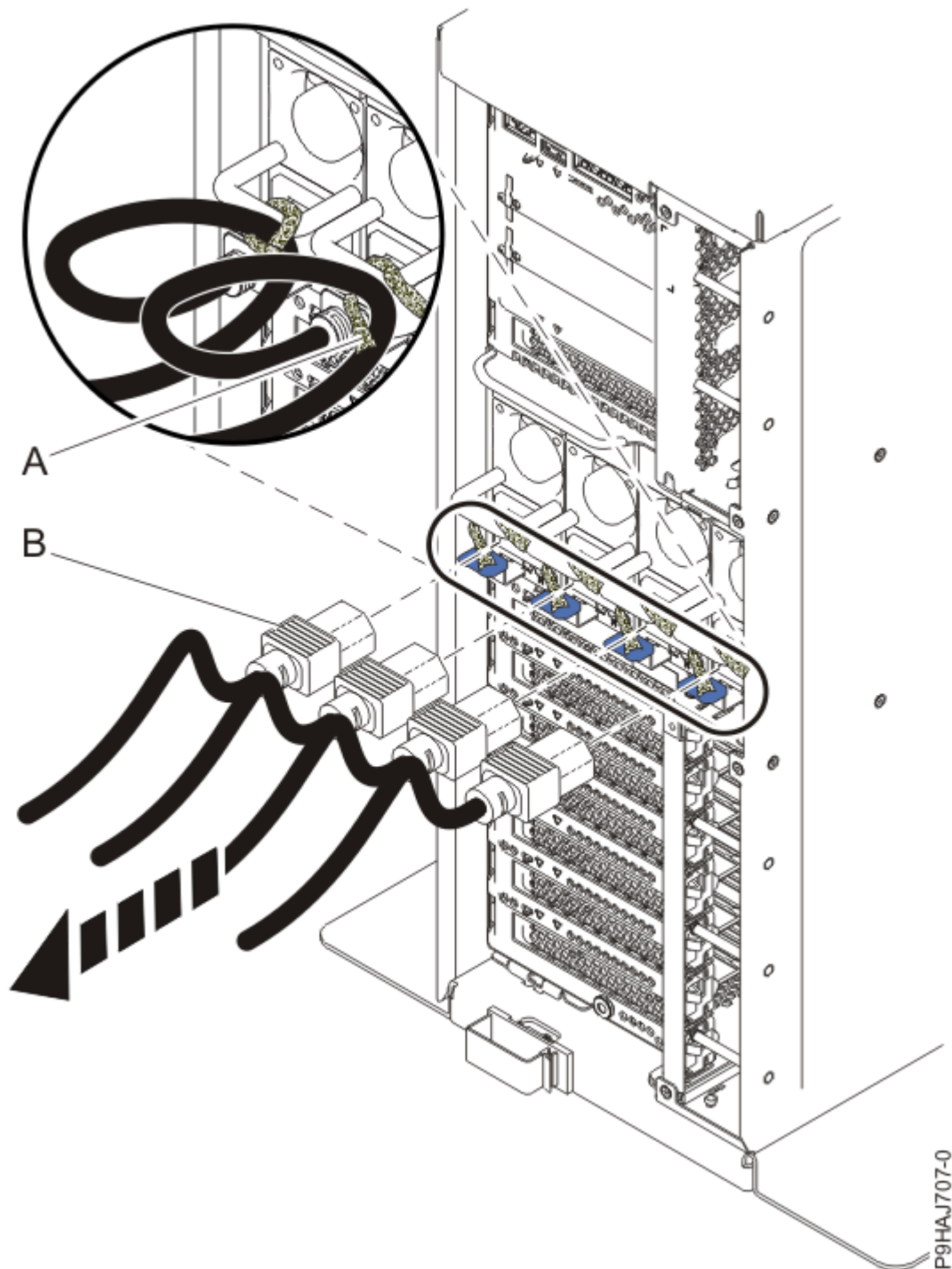
Abbildung 20. Netzkabel von einem Standalone-Server abziehen
