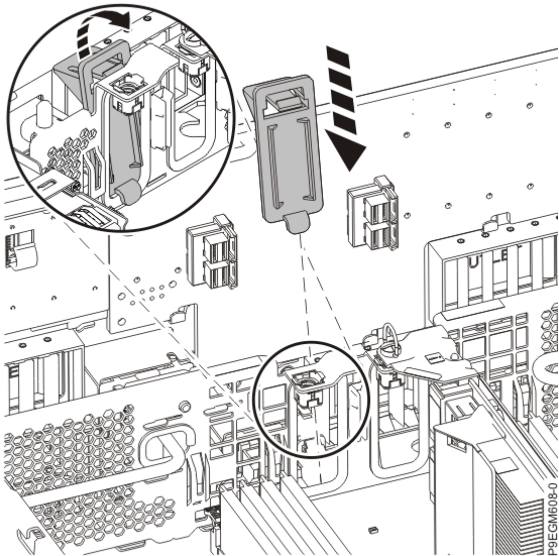
Abbildung 30. Einsteckbare Abdeckblende installieren
