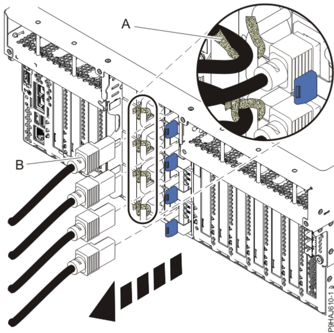
Abbildung 19. Netzkabel von einem Einschubserver abziehen
