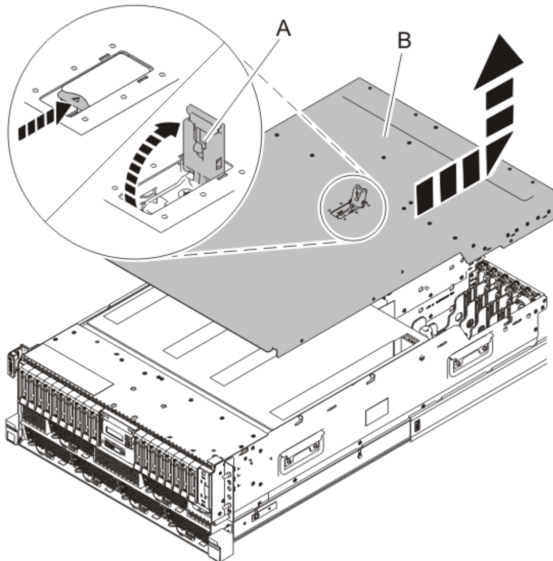
Abbildung 22. Serviceabdeckung eines Einschubsystems ausbauen
