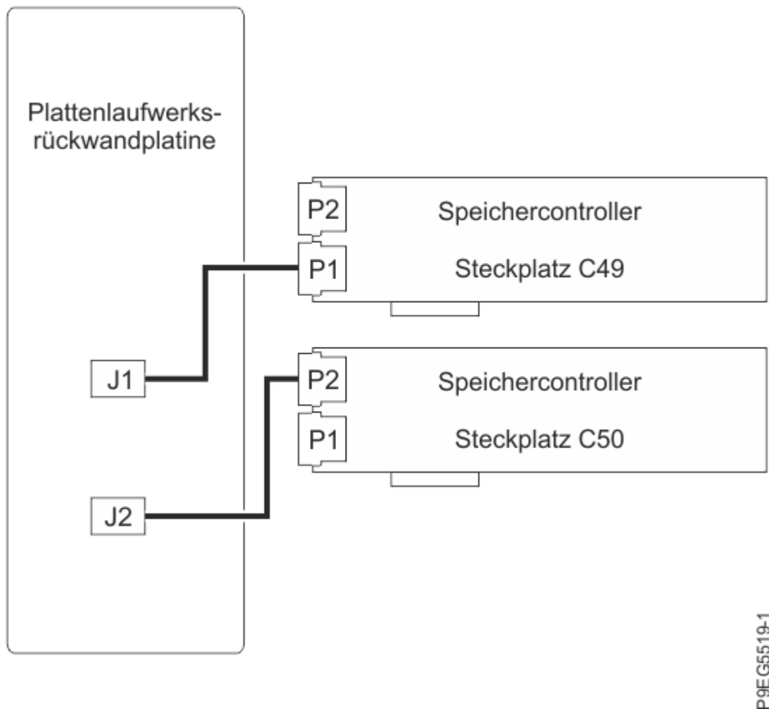
Abbildung 9. SAS-Kabel in einer Konfiguration mit unterteilter Festplatte wieder anschließen
