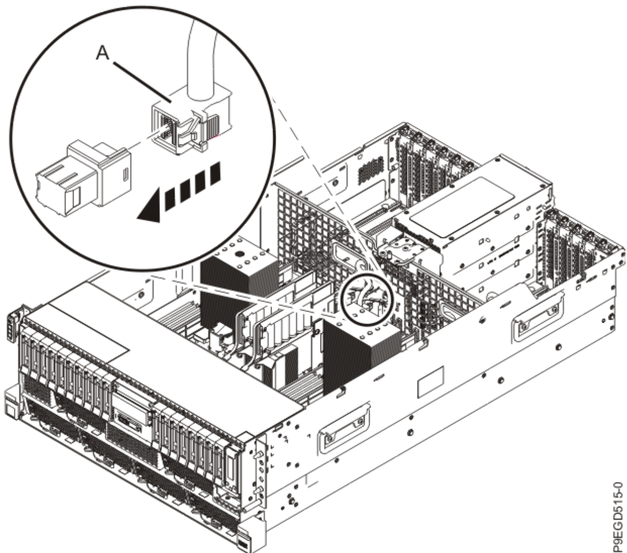
Abbildung 38. Hintere SAS-Kabel wieder anschließen
