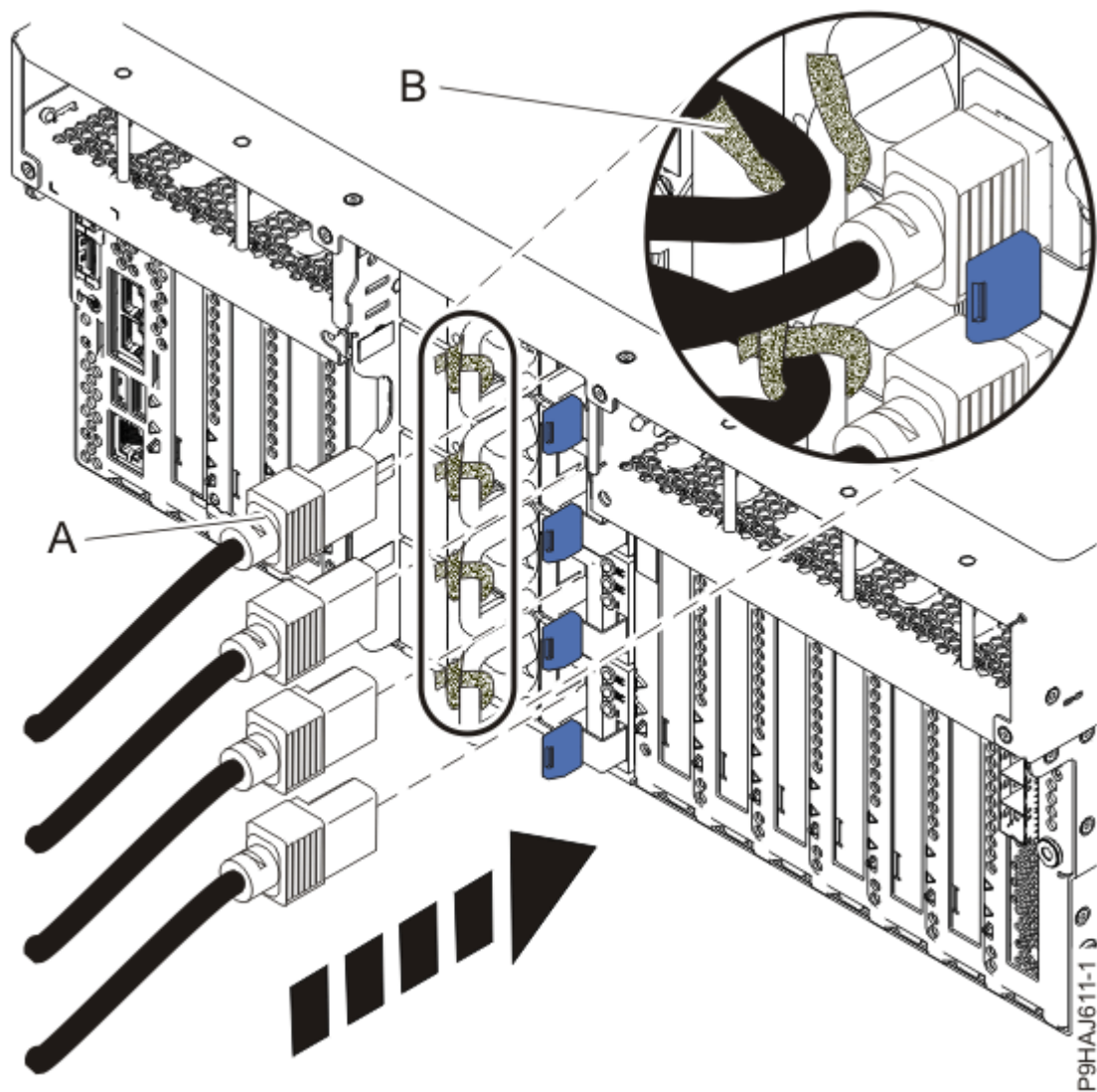
Abbildung 21. Netzkabel an ein Einschubsystem anschließen
