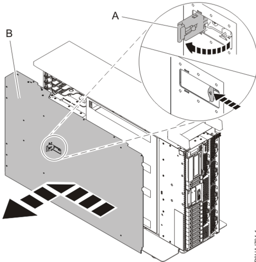
Abbildung 27. Serviceabdeckung ausbauen
