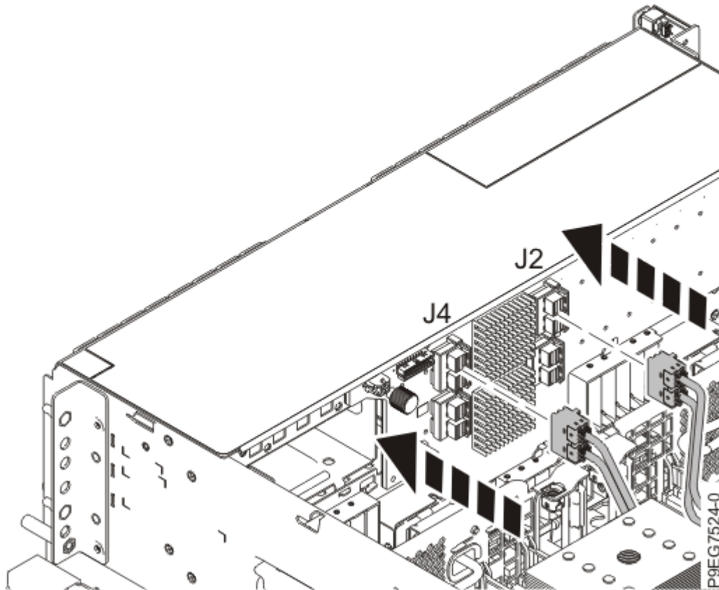
Abbildung 40. Vordere SAS-Kabel für die Plattenlaufwerk-Rückwandplatine der Ausführung "12-Laufwerk mit erweiterter Funktion" oder "18-Laufwerk mit erweiterter Funktion" wieder anschließen
