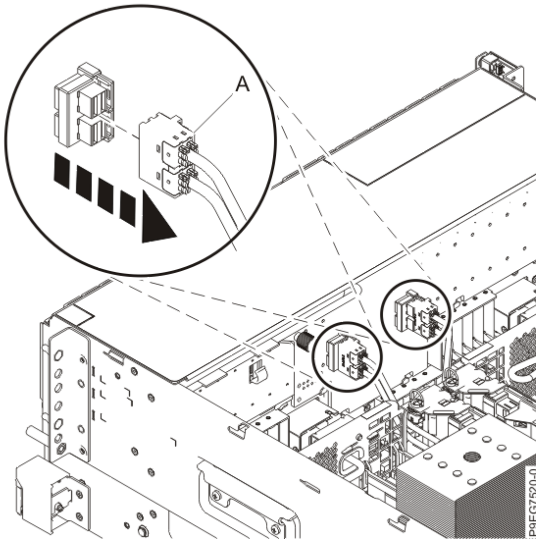
Abbildung 30. Vordere SAS-Kabel herausziehen
