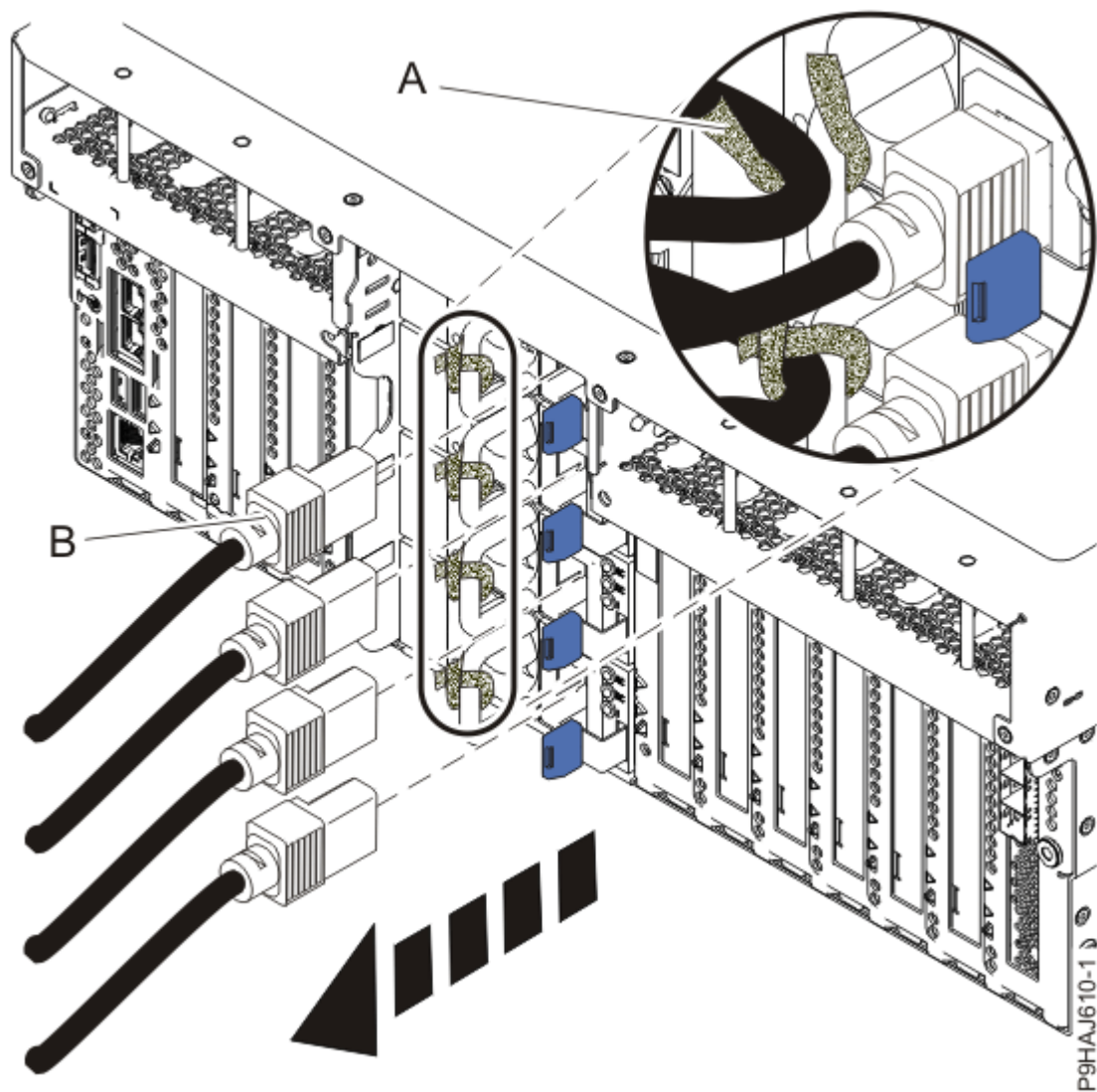
Abbildung 23. Netzkabel von einem Einschubserver abziehen
