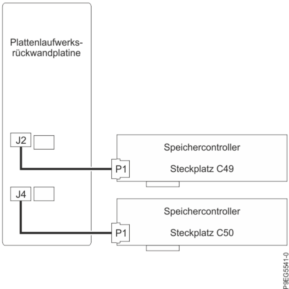
Abbildung 35. SAS-Kabel in einer Konfiguration vom Typ "12-Laufwerk mit erweiterter Funktion" wieder anschließen
