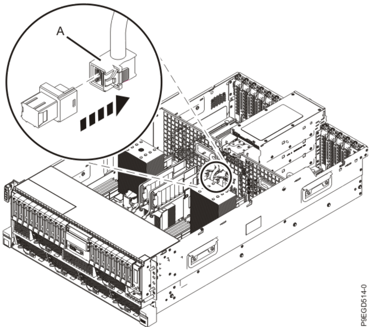
Abbildung 31. Hintere SAS-Kabel vom internen SAS-RAID-Adapter in den Steckplätzen P1-C49 und P-C50 abziehen
