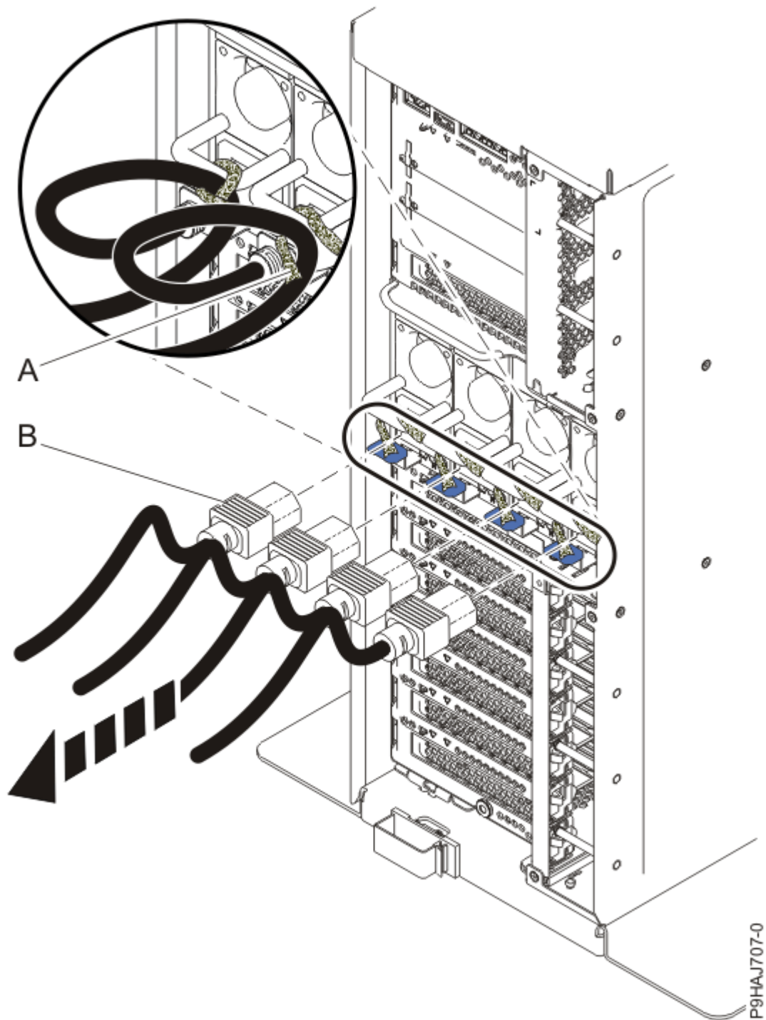
Abbildung 24. Netzkabel von einem Standalone-Server abziehen
