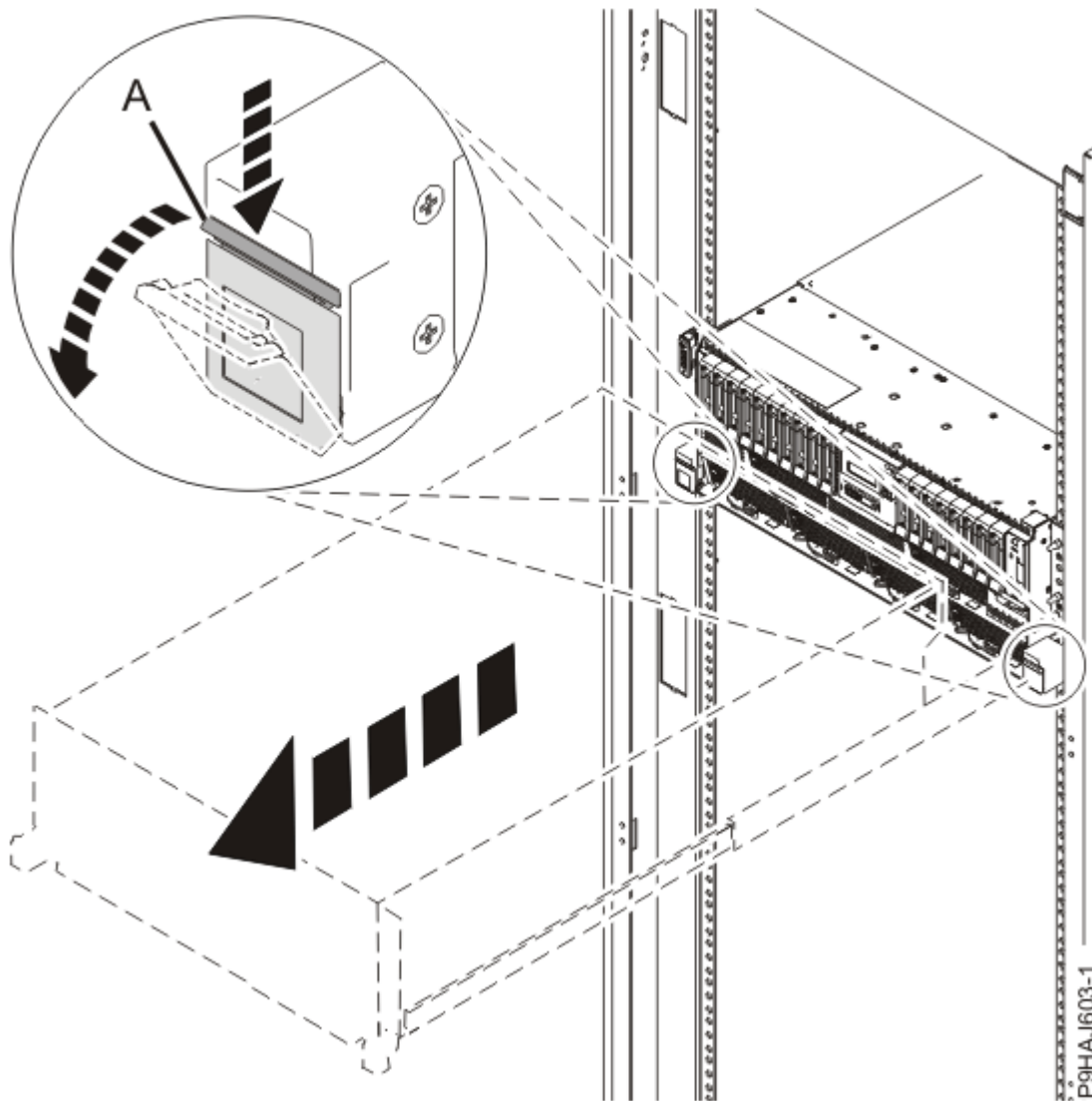
Abbildung 25. Seitliche Verriegelungen entriegeln
