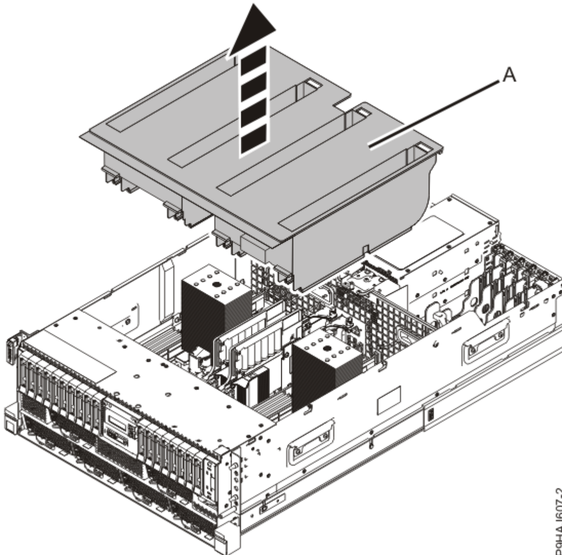
Abbildung 28. Luftführung aus einem Einschubsystem ausbauen
