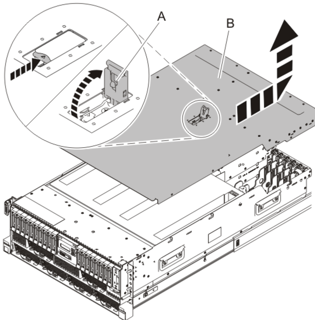
Abbildung 26. Serviceabdeckung eines Einschubsystems ausbauen
