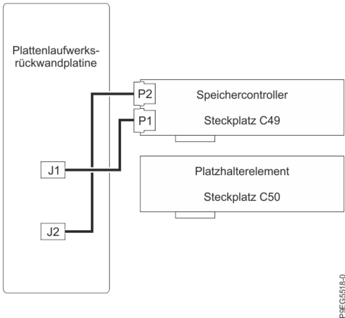
Abbildung 8. SAS-Kabel in einer Basisspeicherkonfiguration wieder anschließen
