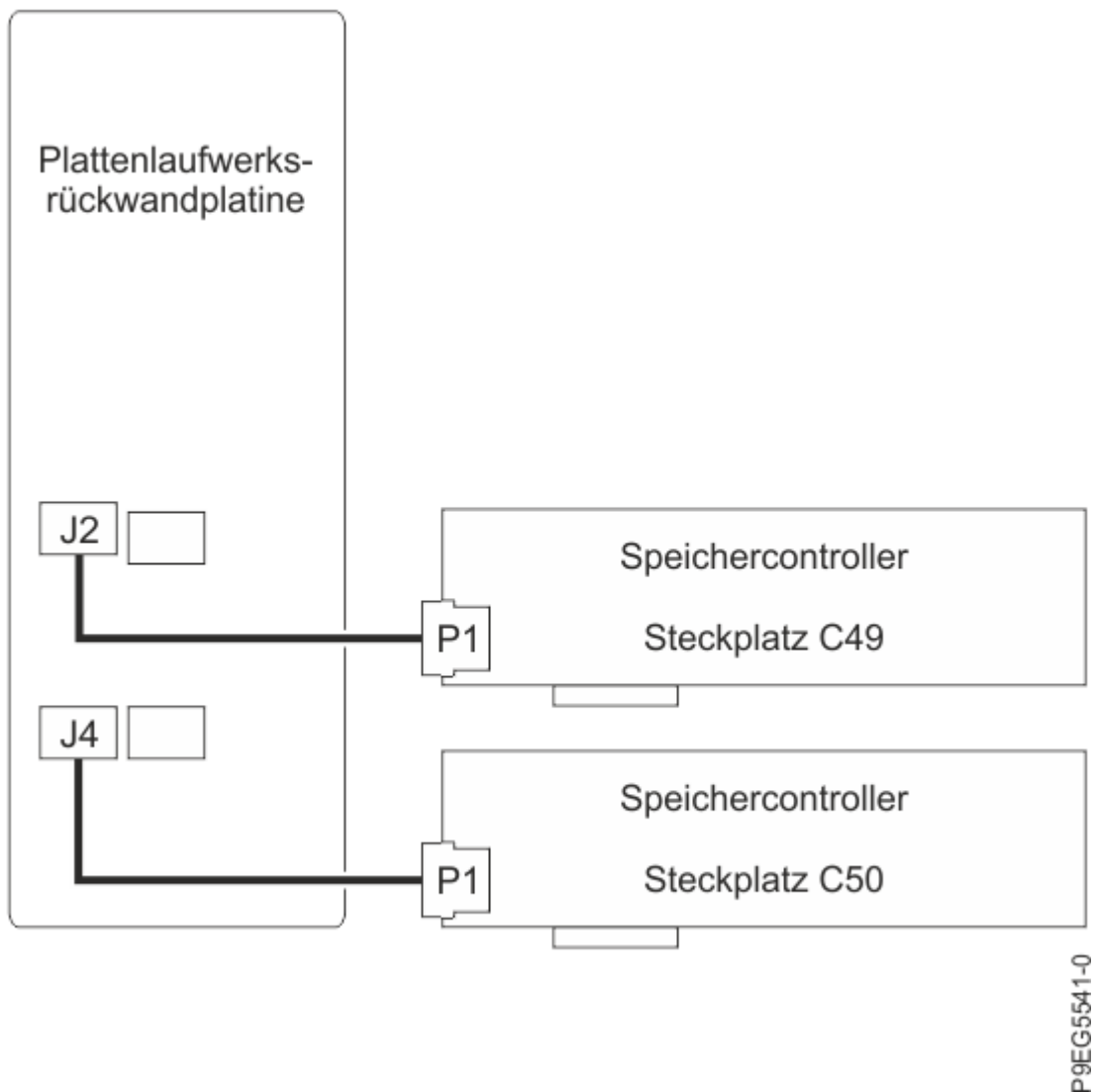
Abbildung 36. SAS-Kabel in einer Konfiguration vom Typ "18-Laufwerk mit erweiterter Funktion" wieder anschließen
