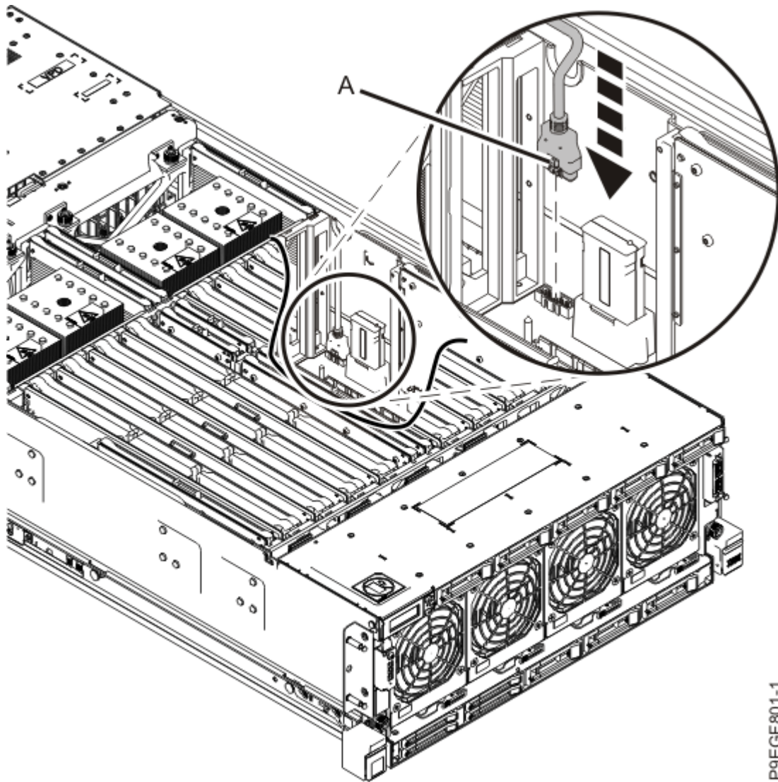
Abbildung 11. Hinteres USB-Kabel in der Systemrückwandplatine wiederanschließen
