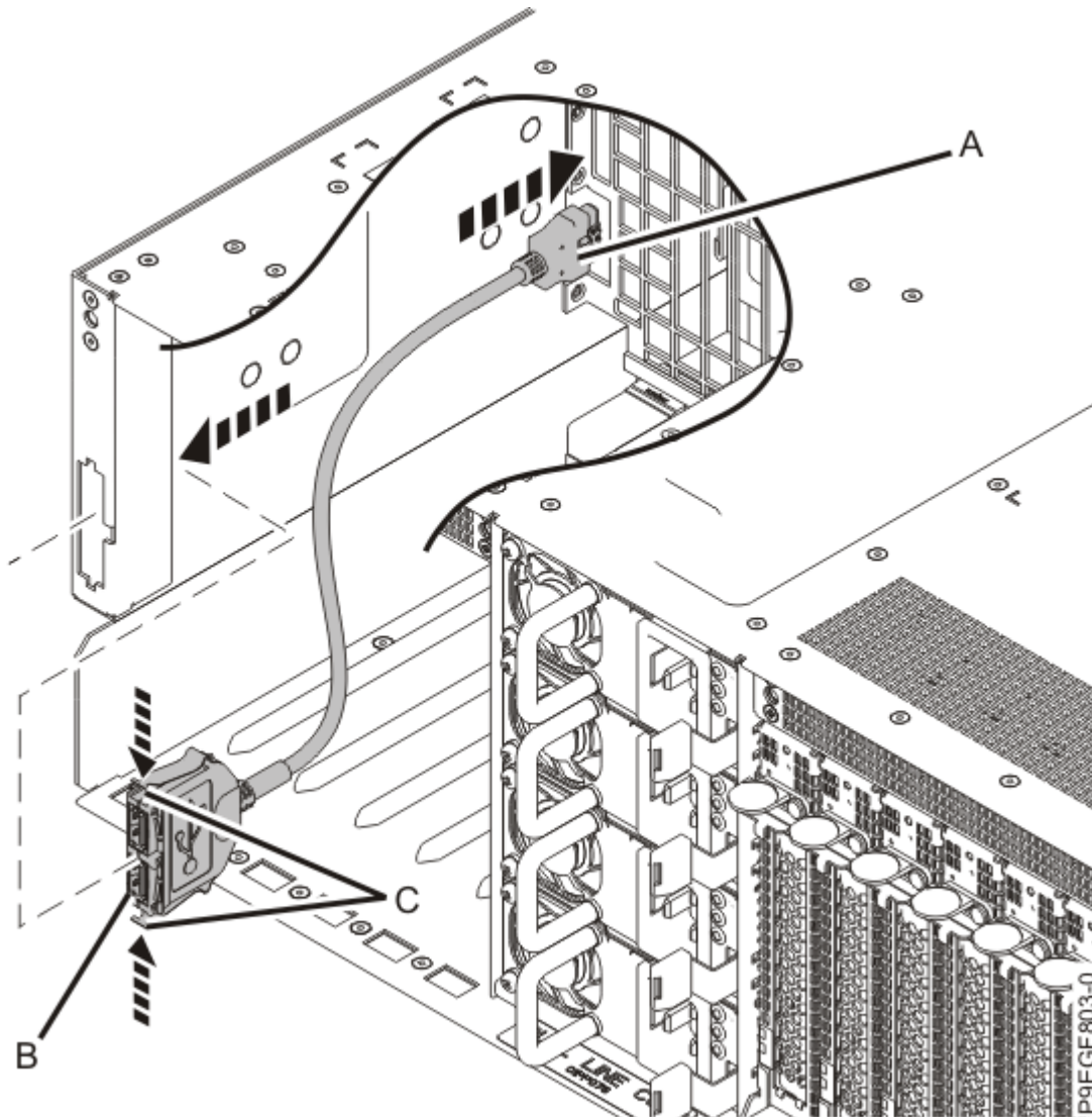
Abbildung 9. Hinteren USB-Anschlusstecker wiedereinbauen
