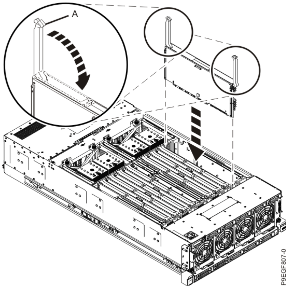
Abbildung 12. Speicherriserkarte installieren
