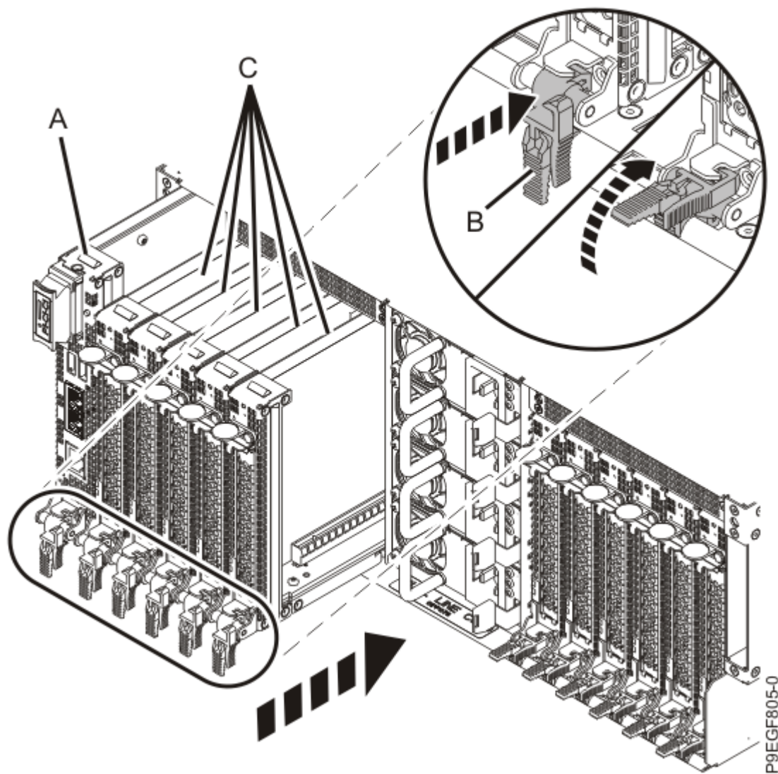
Abbildung 15. Serviceprozessorkarte und PCIe-Kassetten wieder einsetzen
