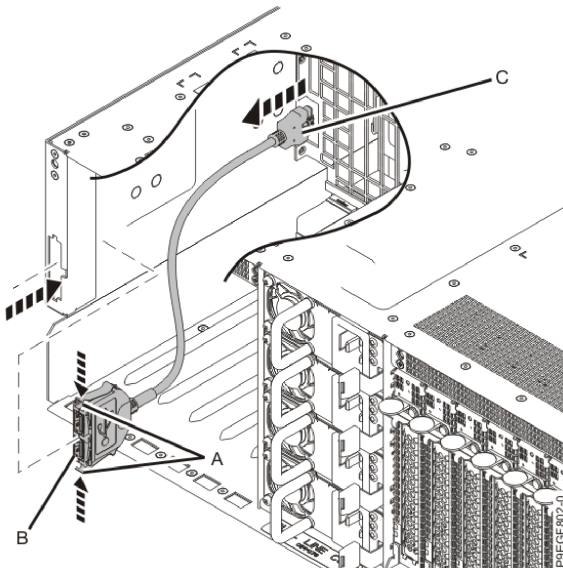
Abbildung 8. Hinteren USB-Anschlusstecker ausbauen
