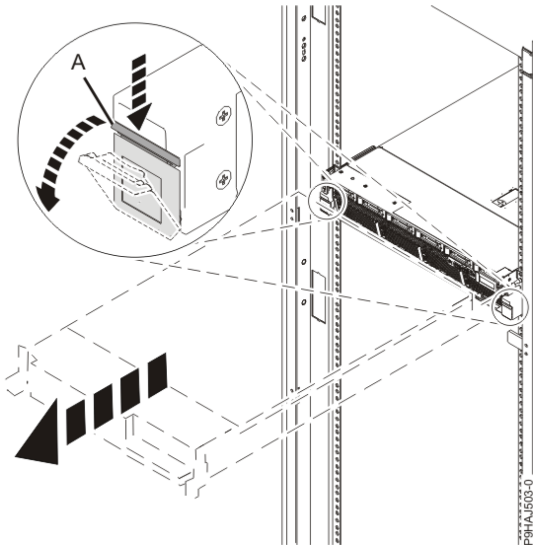
Abbildung 2. Seitliche Verriegelungen entriegeln
