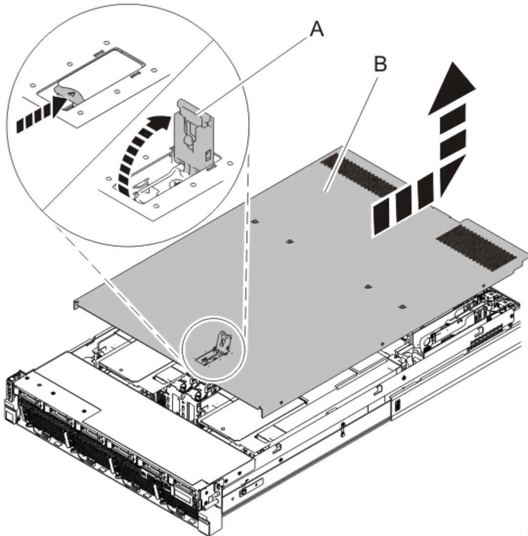
Abbildung 4. Serviceabdeckung ausbauen
