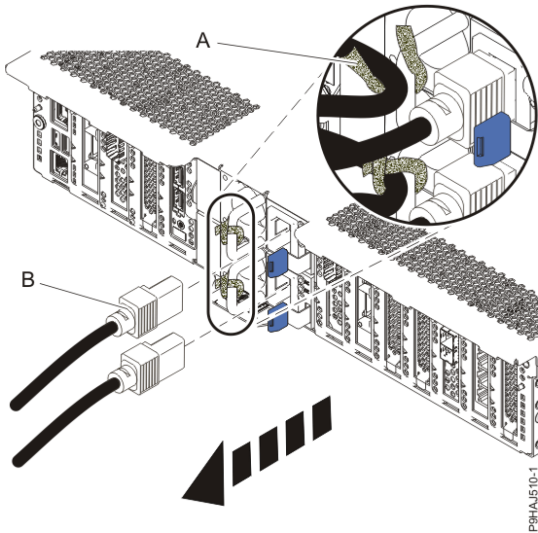
Abbildung 1. Netzkabel abziehen
