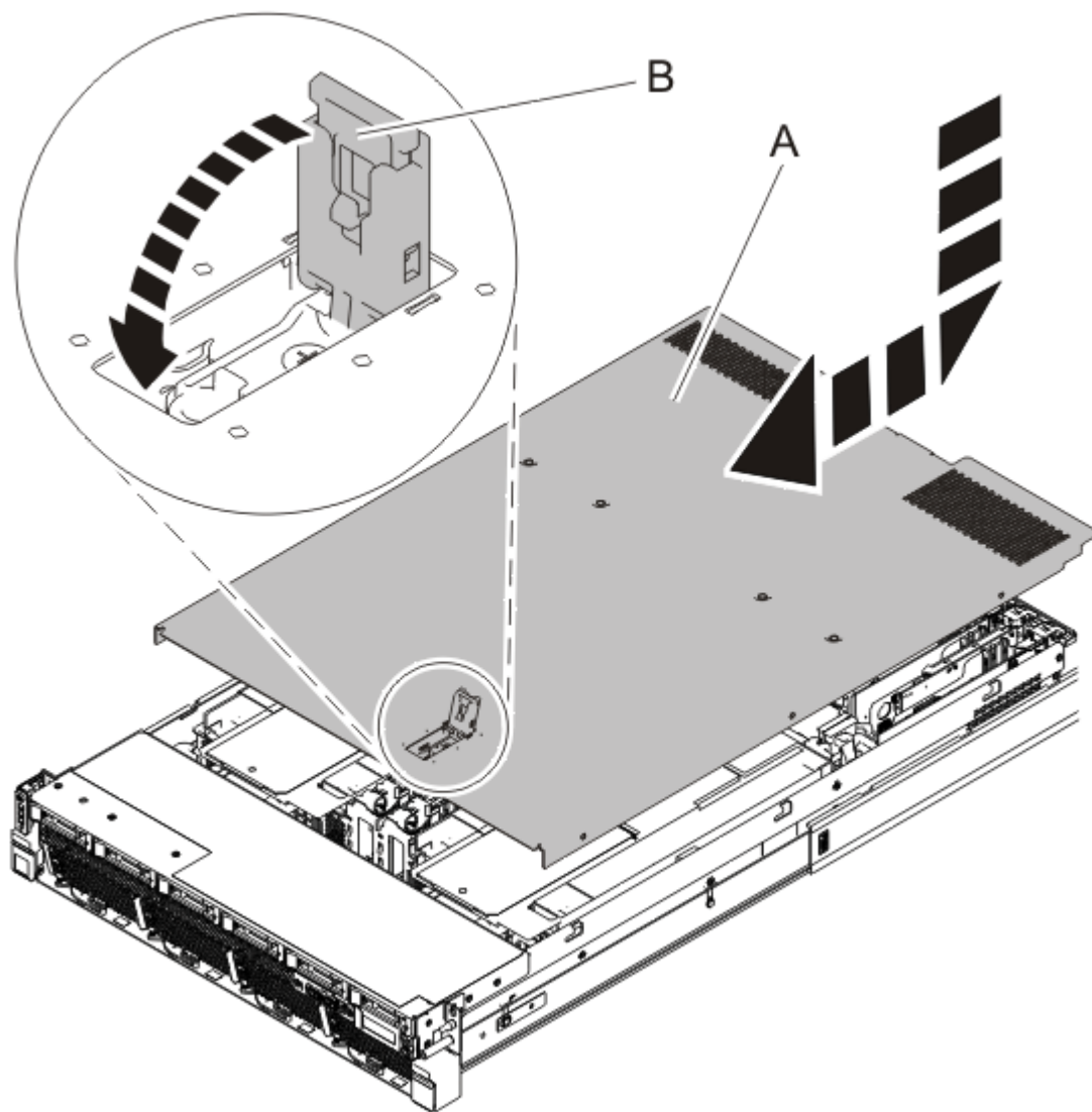
Abbildung 7. Serviceabdeckung installieren
