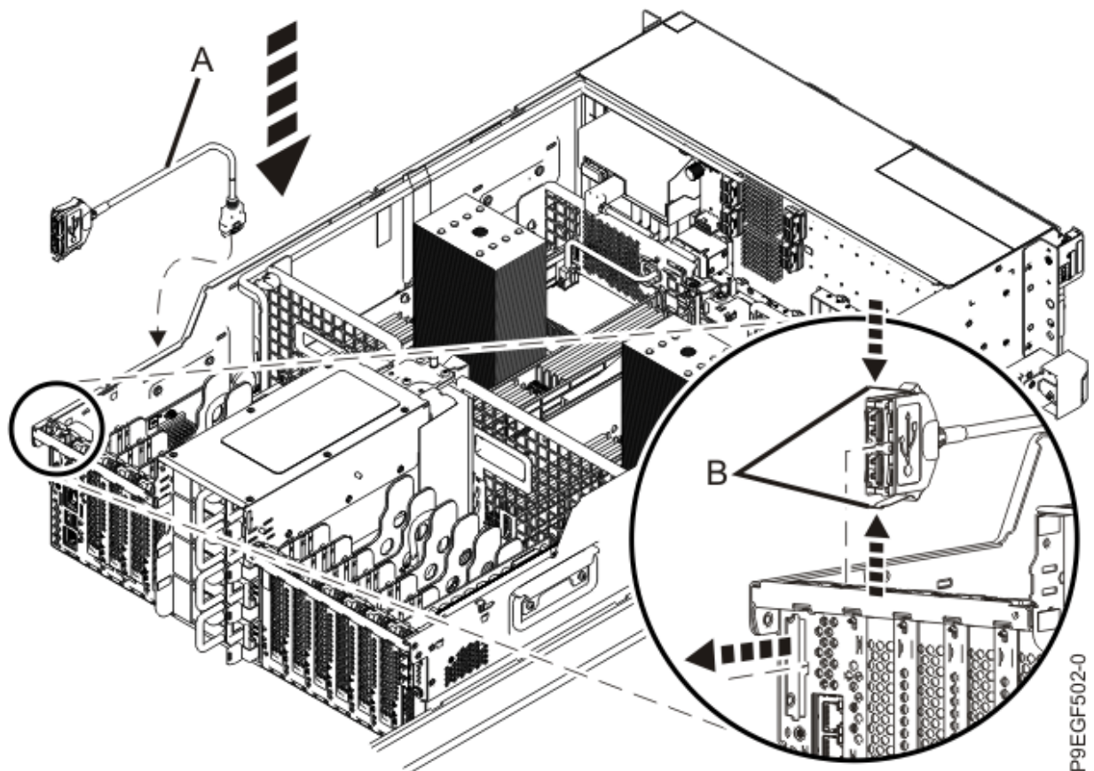
Abbildung 11. Hinteres USB-Kabel im System wiederanschießen
