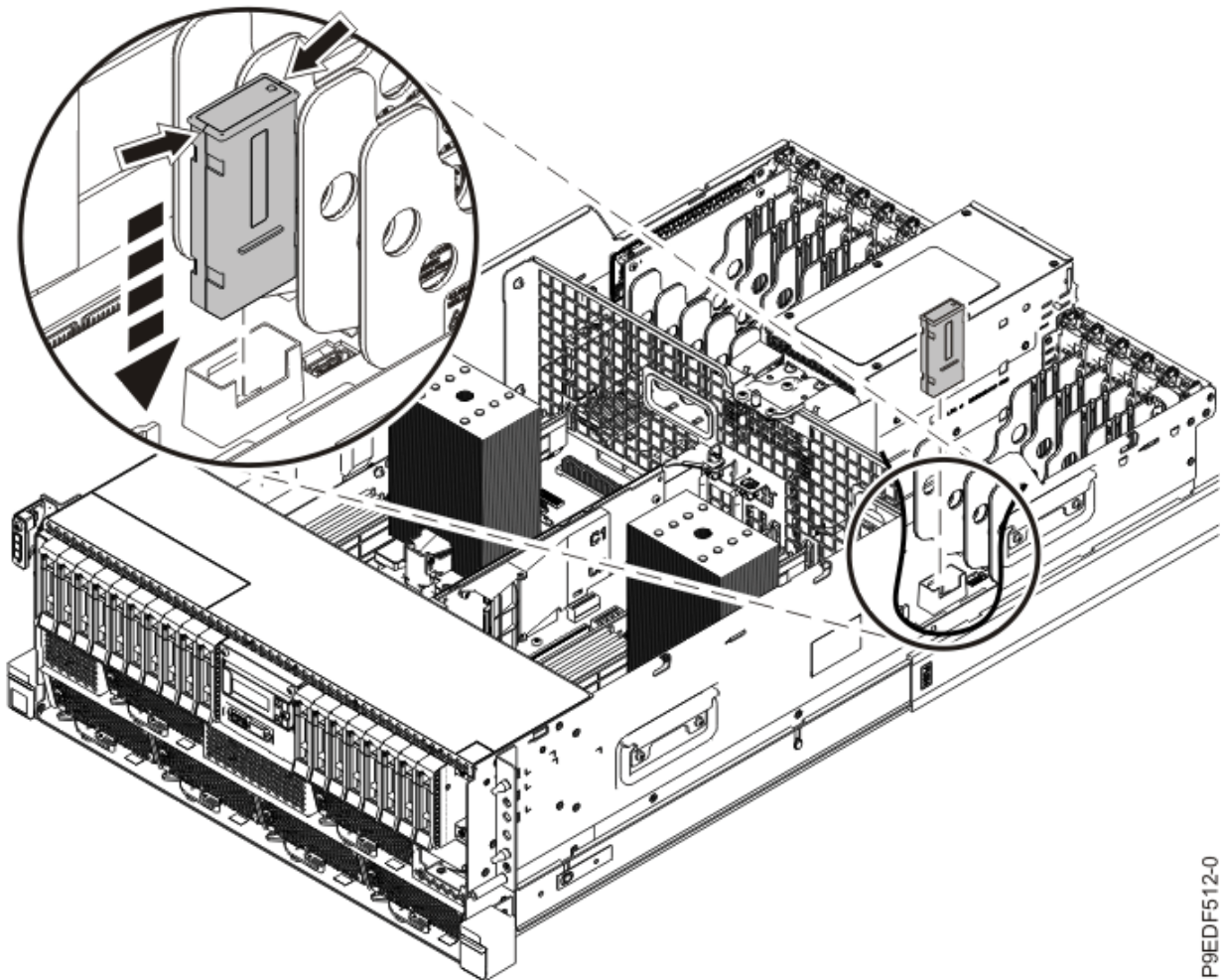
Abbildung 14. Karte mit den elementaren Produktdaten wieder einsetzen
