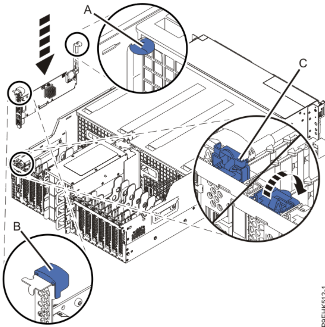
Abbildung 12. Serviceprozessorkarte in Steckplatz P1-C1 installieren
