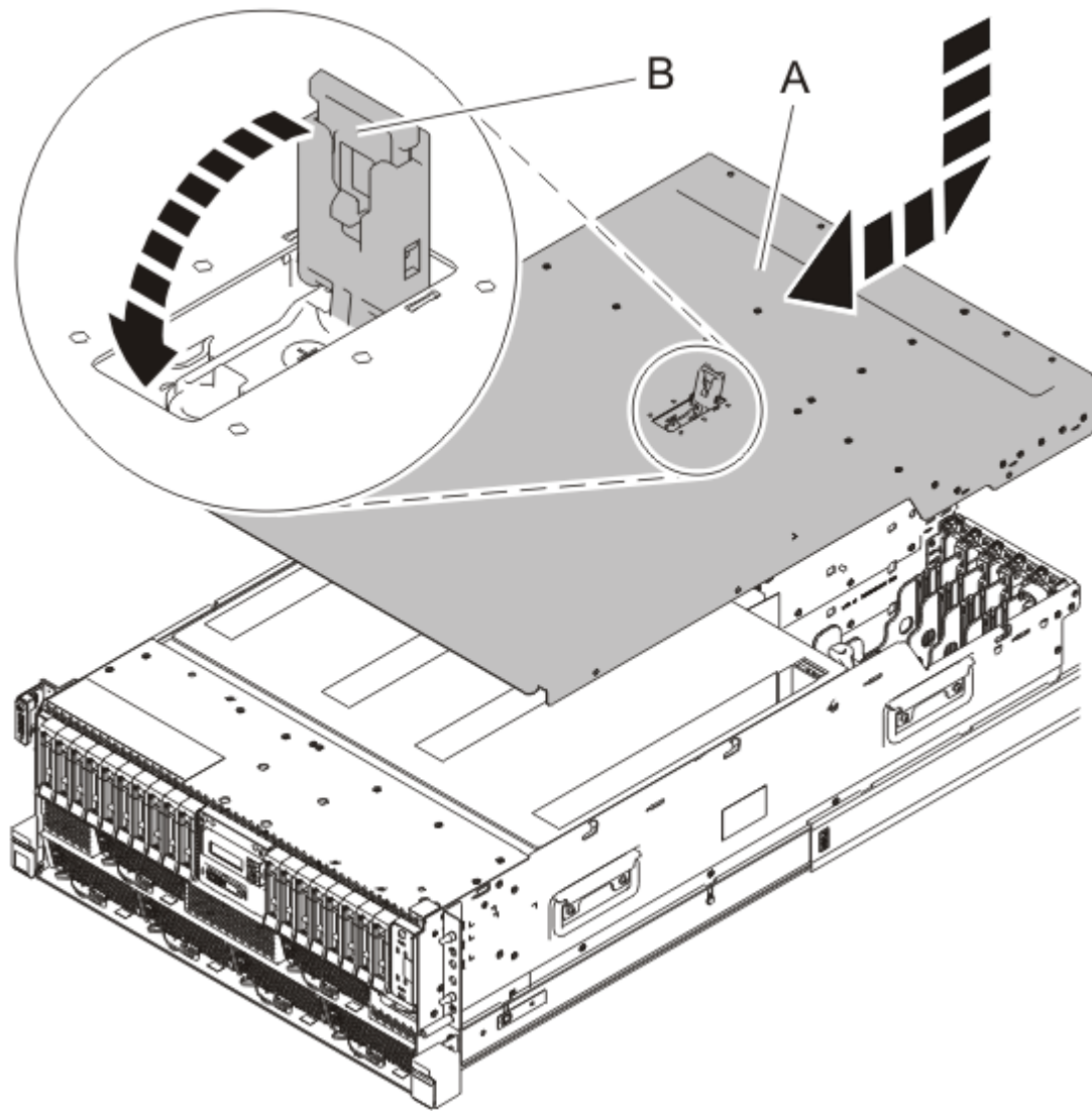
Abbildung 15. Serviceabdeckung installieren
