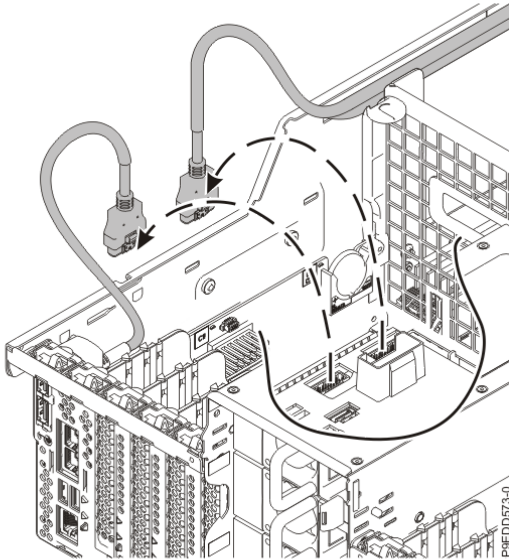
Abbildung 8. Vordere und hintere USB-Kabel entfernen
