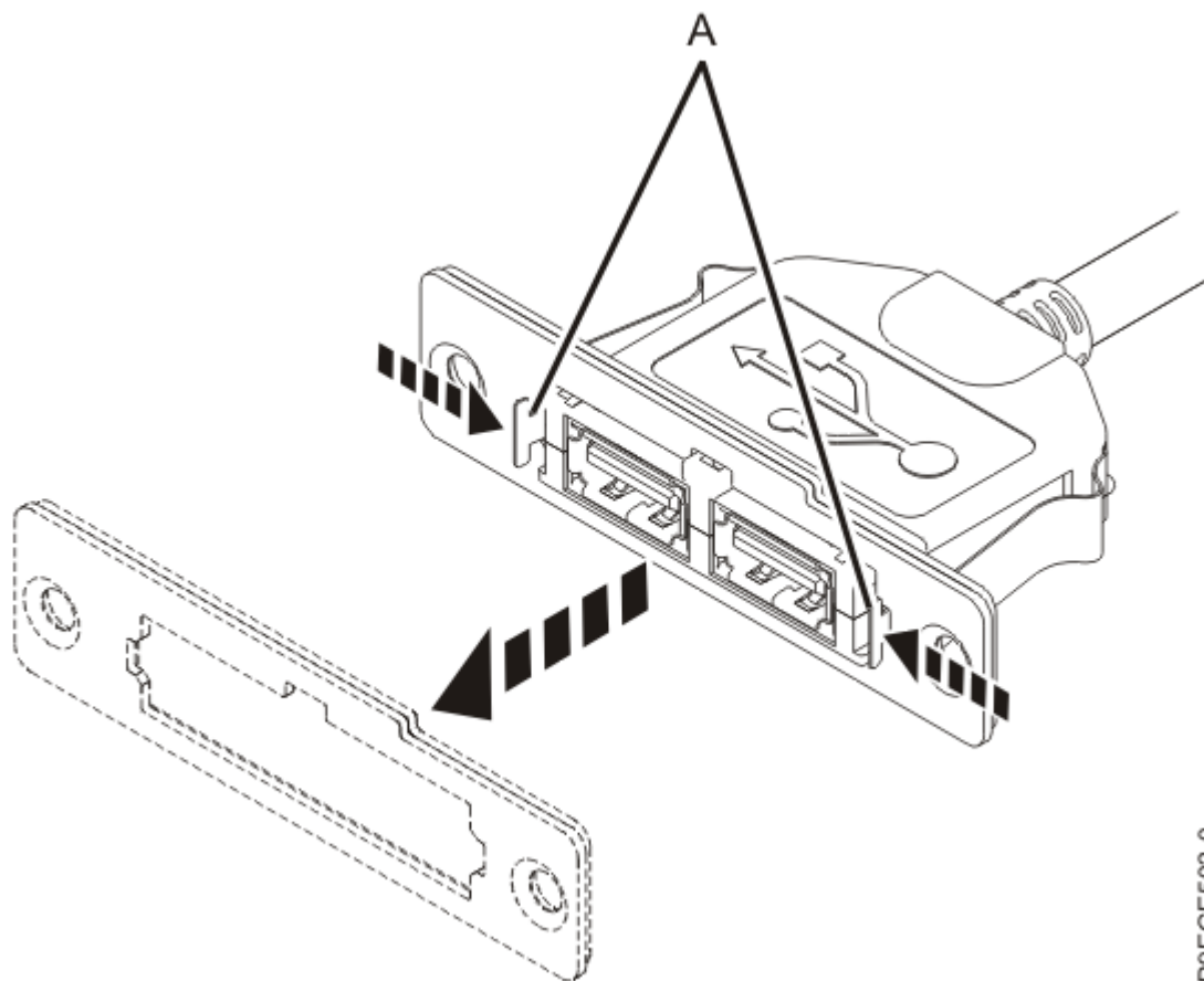
Abbildung 9. USB-Kabel an der Vorderseite und Buchse am vorderen USB-Halter ausbauen
