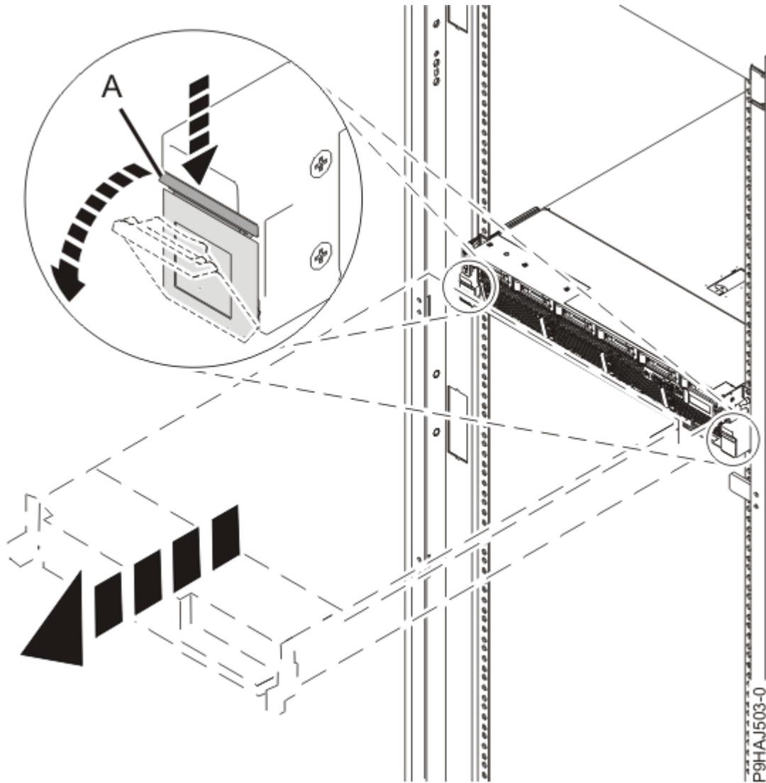
Abbildung 3. Seitliche Verriegelungen entriegeln
