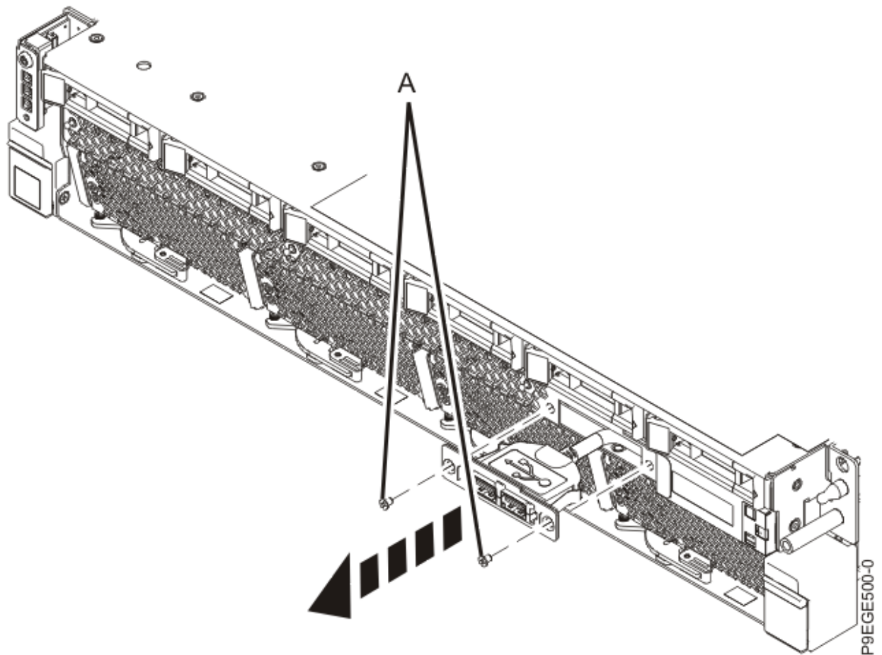
Abbildung 8. Zwei Schrauben vom vorderen USB-Halter entfernen
