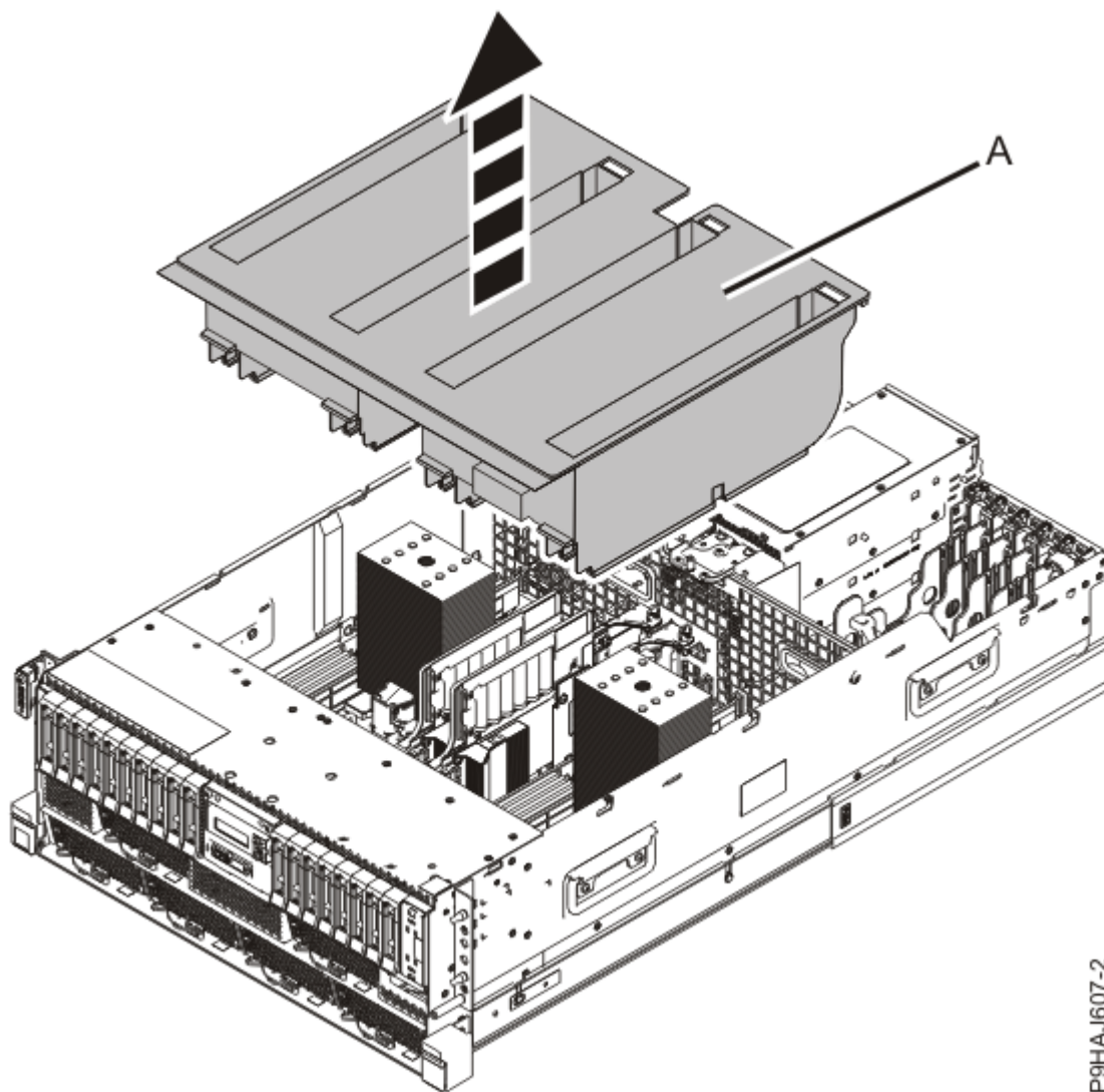
Abbildung 11. Luftführung aus einem Einschubsystem ausbauen
