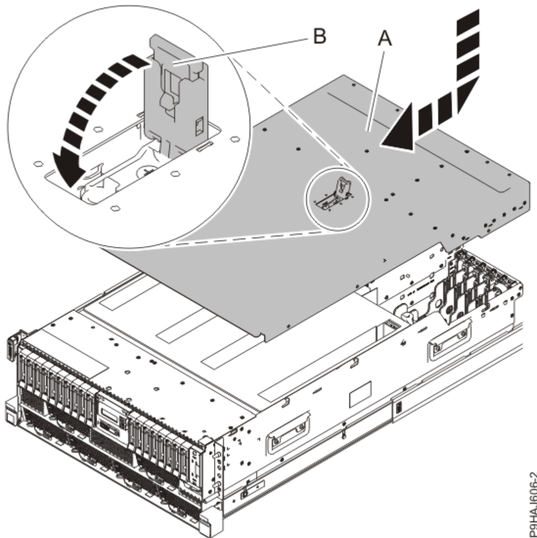
Abbildung 32. Serviceabdeckung installieren
