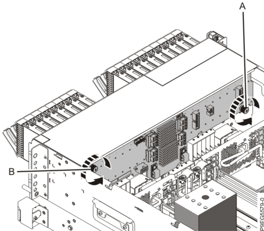
Abbildung 17. Schrauben der Plattenlaufwerk-Rückwandplatine lösen
