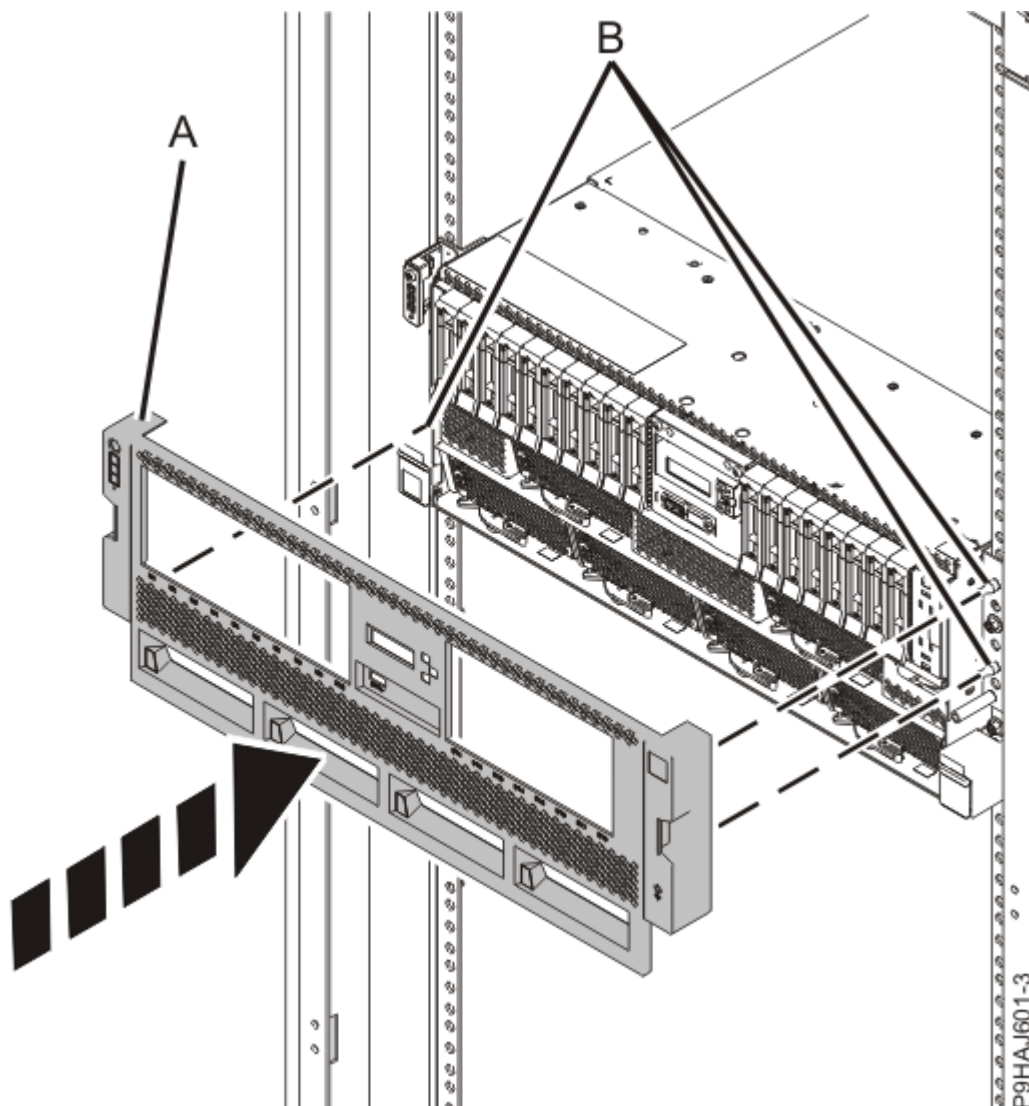
Abbildung 35. Vordere Abdeckung installieren
