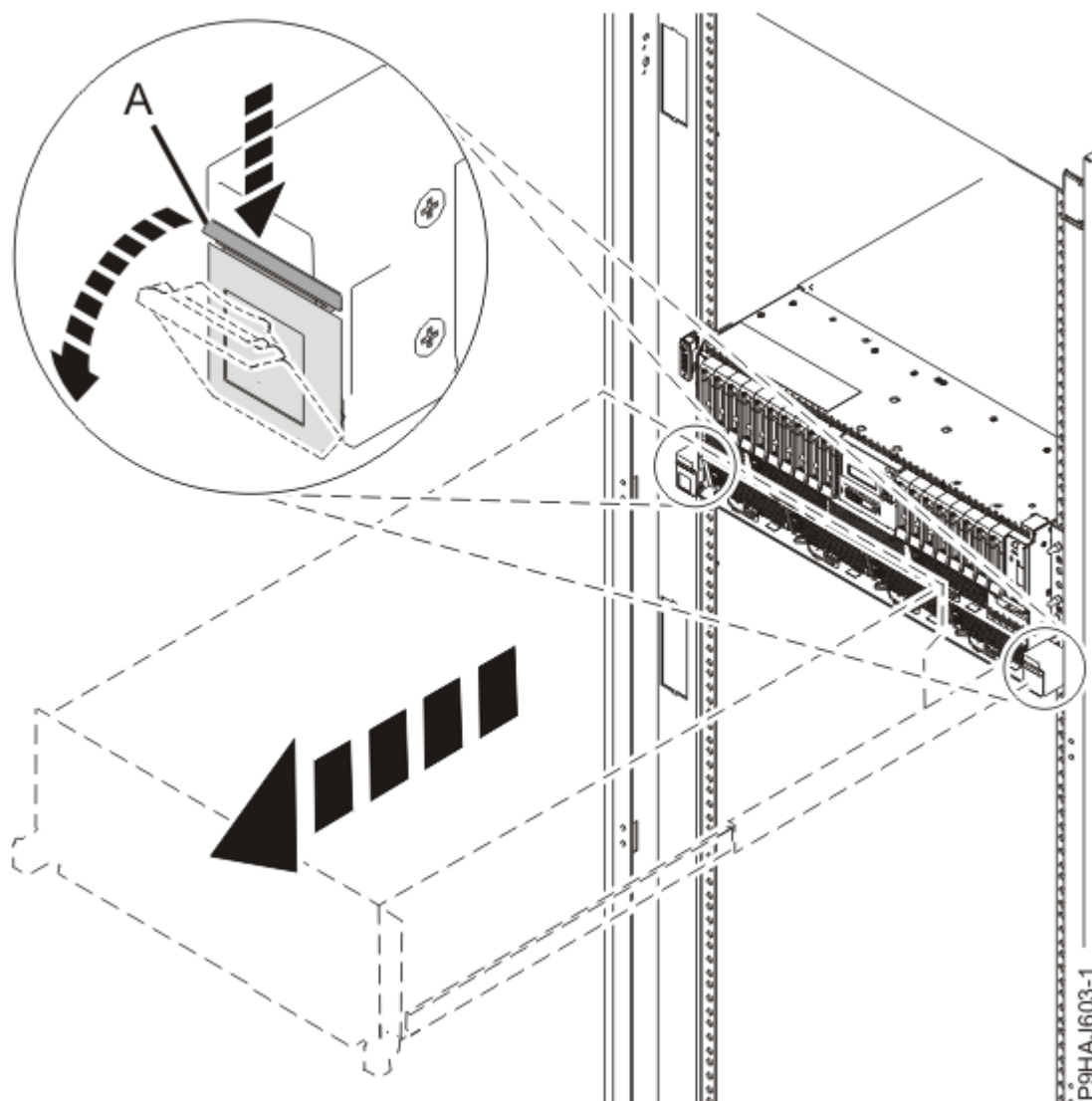
Abbildung 7. Seitliche Verriegelungen entriegeln
