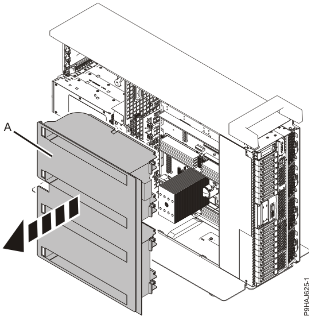
Abbildung 12. Luftführung aus einem Standalone-System ausbauen
