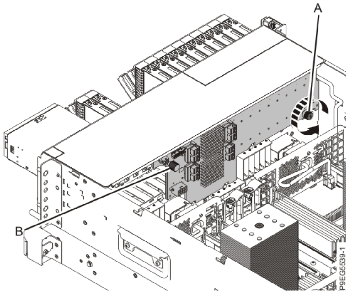
Abbildung 16. Schrauben der Plattenlaufwerk-Rückwandplatine lösen
