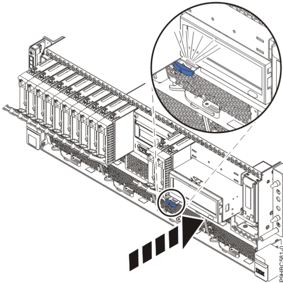
Abbildung 30. RDX-Andockstation austauschen
