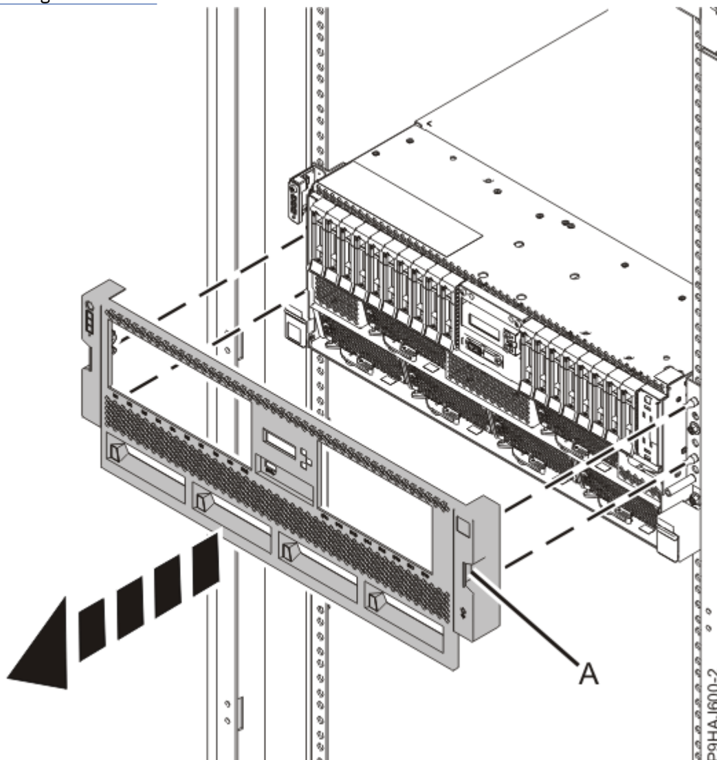
Abbildung 3. Vordere Abdeckung ausbauen
