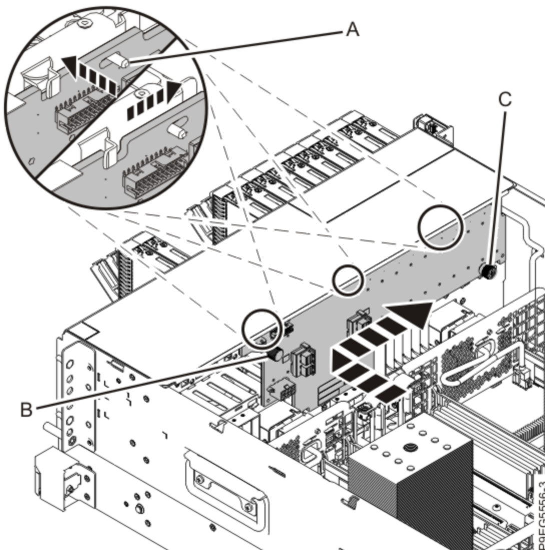
Abbildung 27. Mit Ausrichtungsstiften die Plattenlaufwerk-Rückwandplatine austauschen
