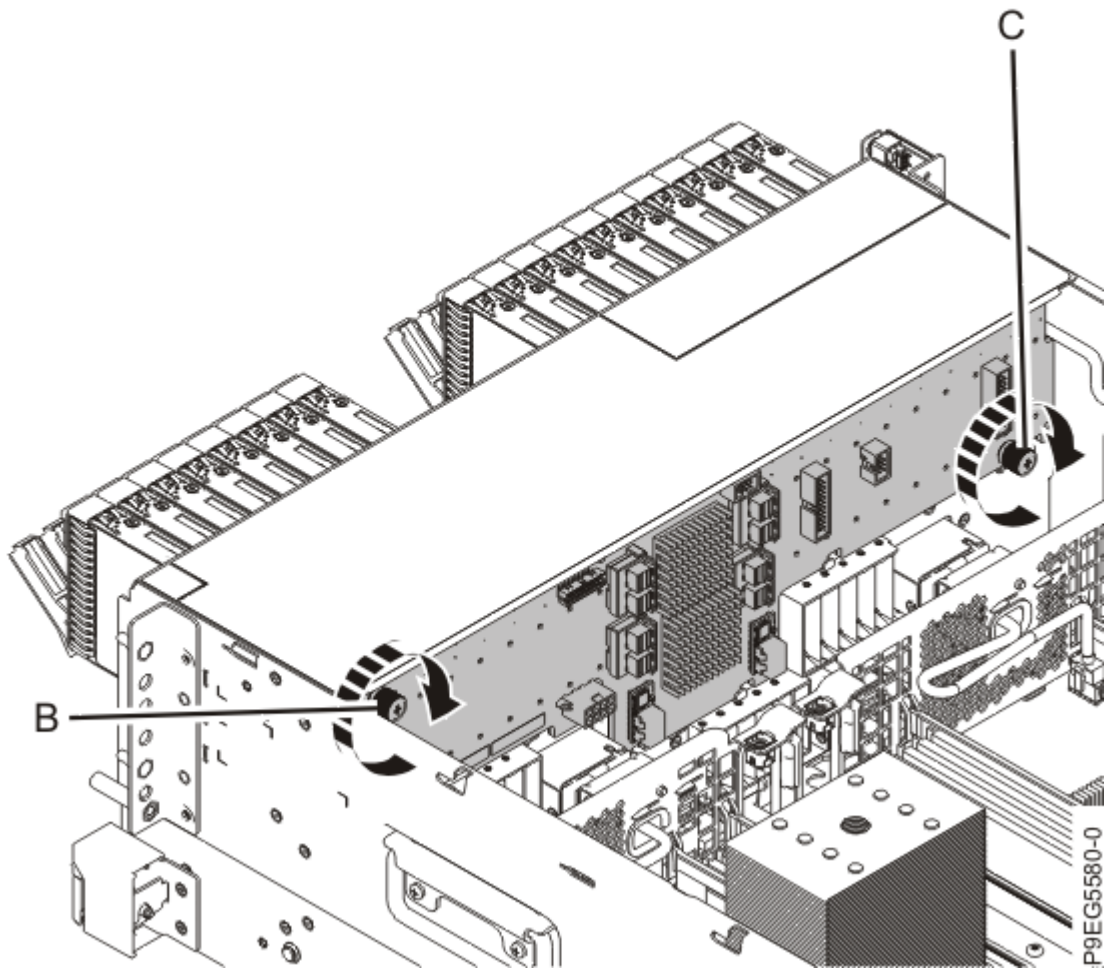
Abbildung 29. Plattenlaufwerk-Rückwandplatine austauschen
