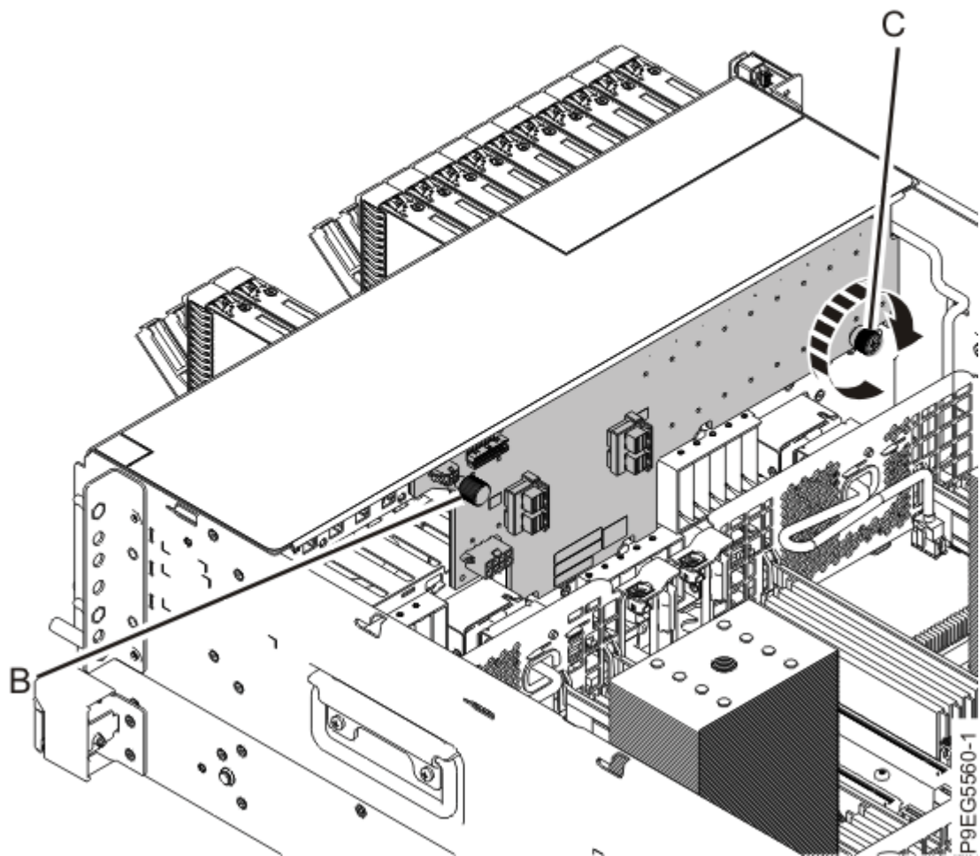
Abbildung 28. Plattenlaufwerk-Rückwandplatine austauschen
