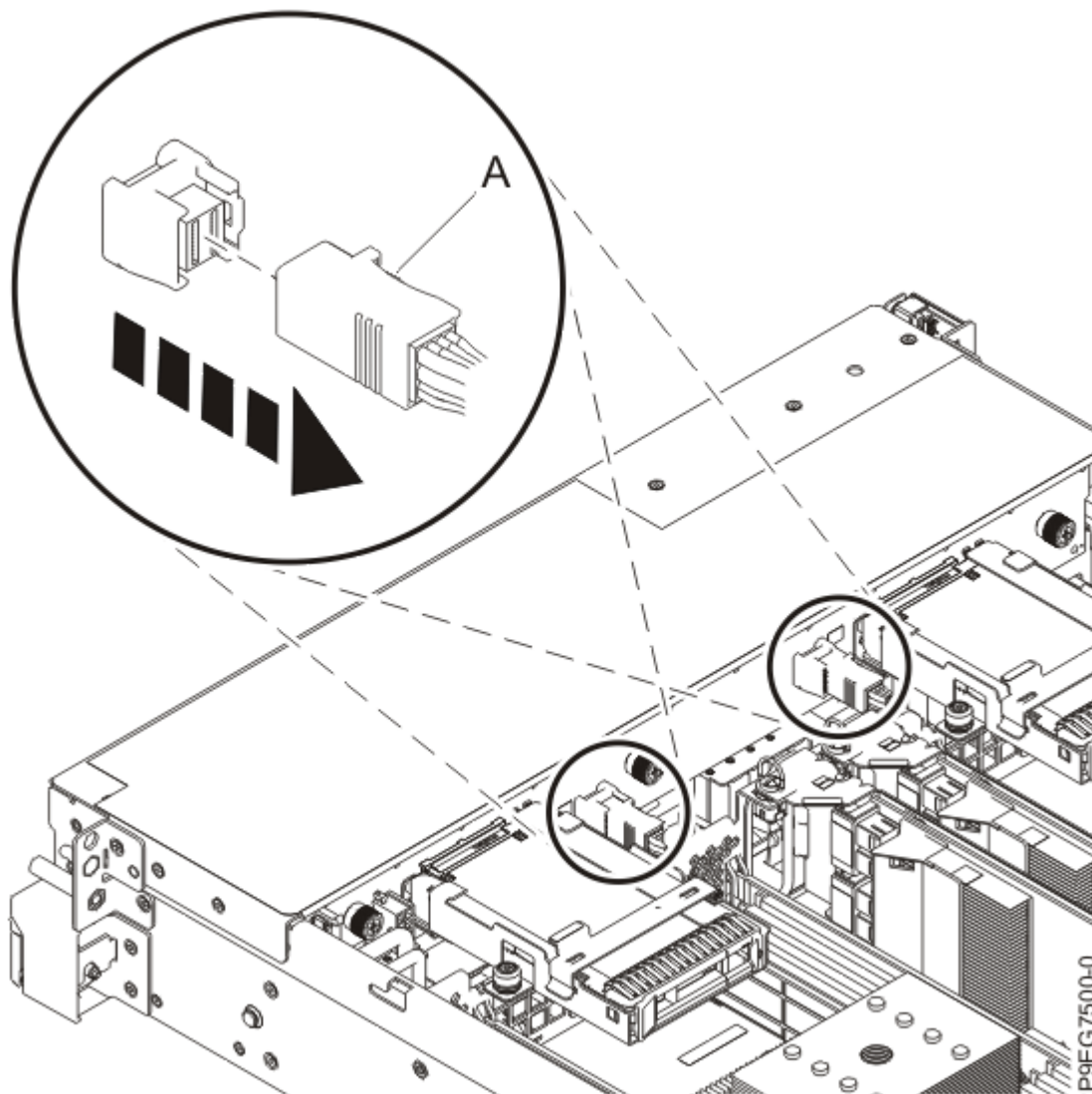
Abbildung 6. Vorderes SAS-Kabel herausziehen
