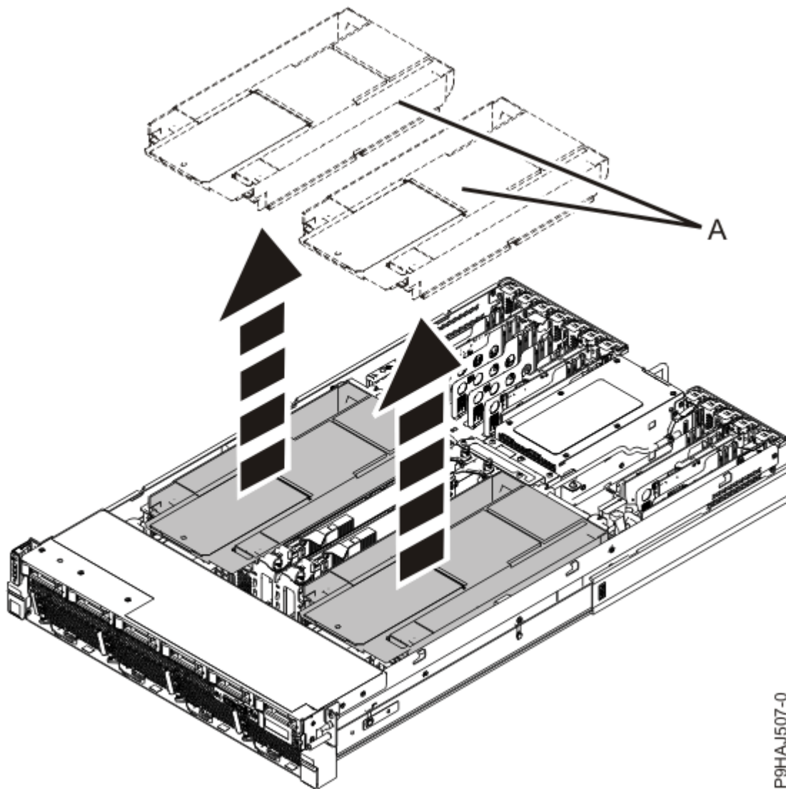
Abbildung 5. Luftführung ausbauen
