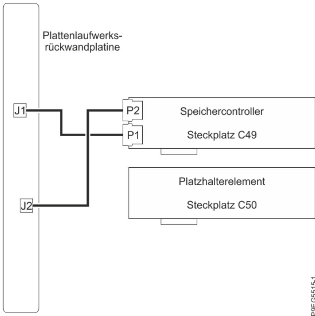
Abbildung 9. SAS-Kabel in einer Basisspeicherkonfiguration wieder anschließen
