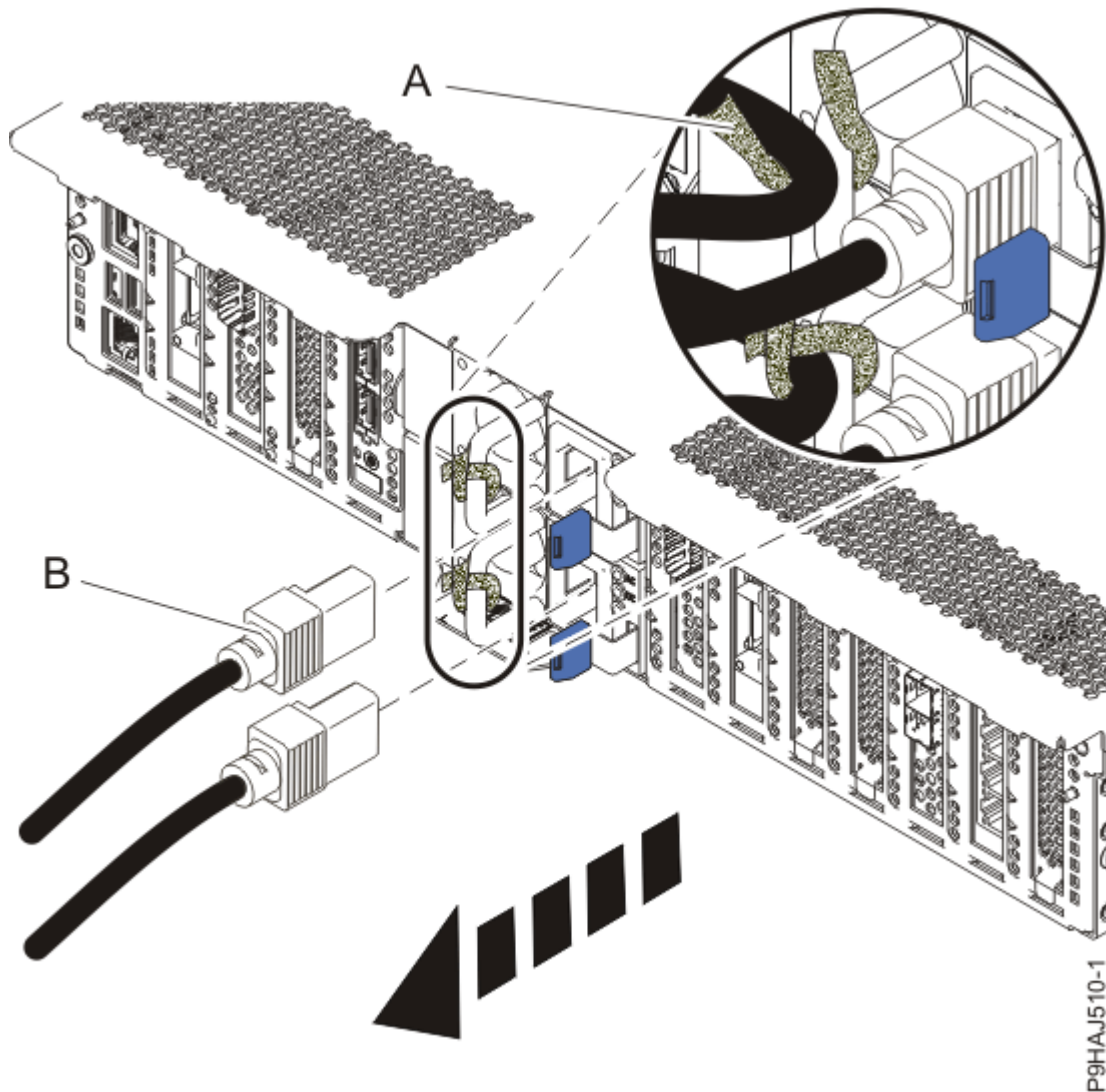
Abbildung 1. Netzkabel abziehen
