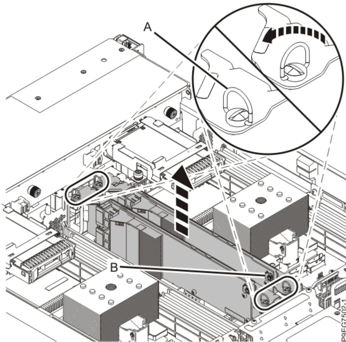
Abbildung 7. SAS-RAID-Adapter entfernen
