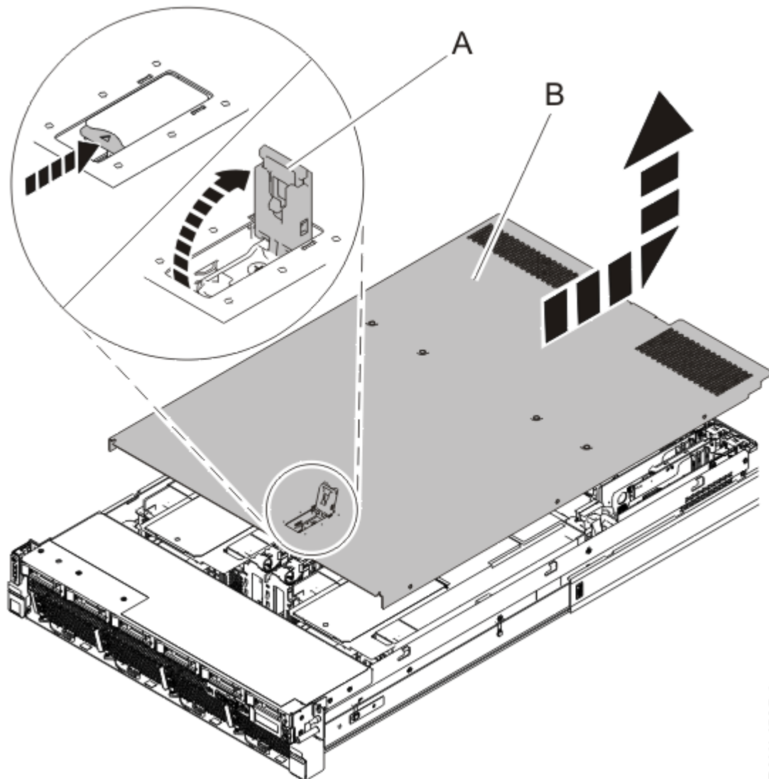
Abbildung 4. Serviceabdeckung ausbauen
