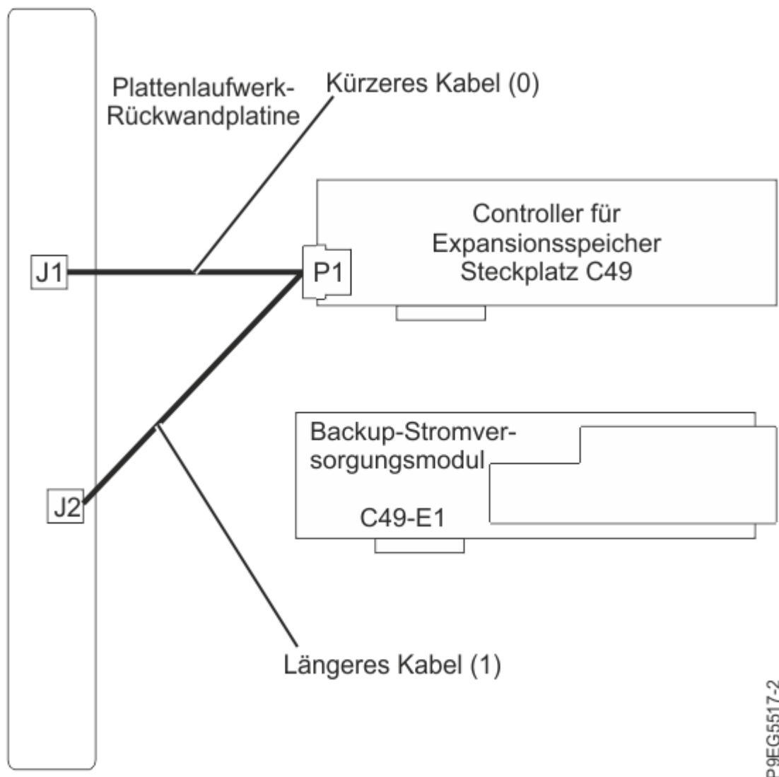
Abbildung 11. "Y"-SAS-Kabel in einer Konfiguration mit einem Hochleistungs-Speichercontroller wieder anschließen
