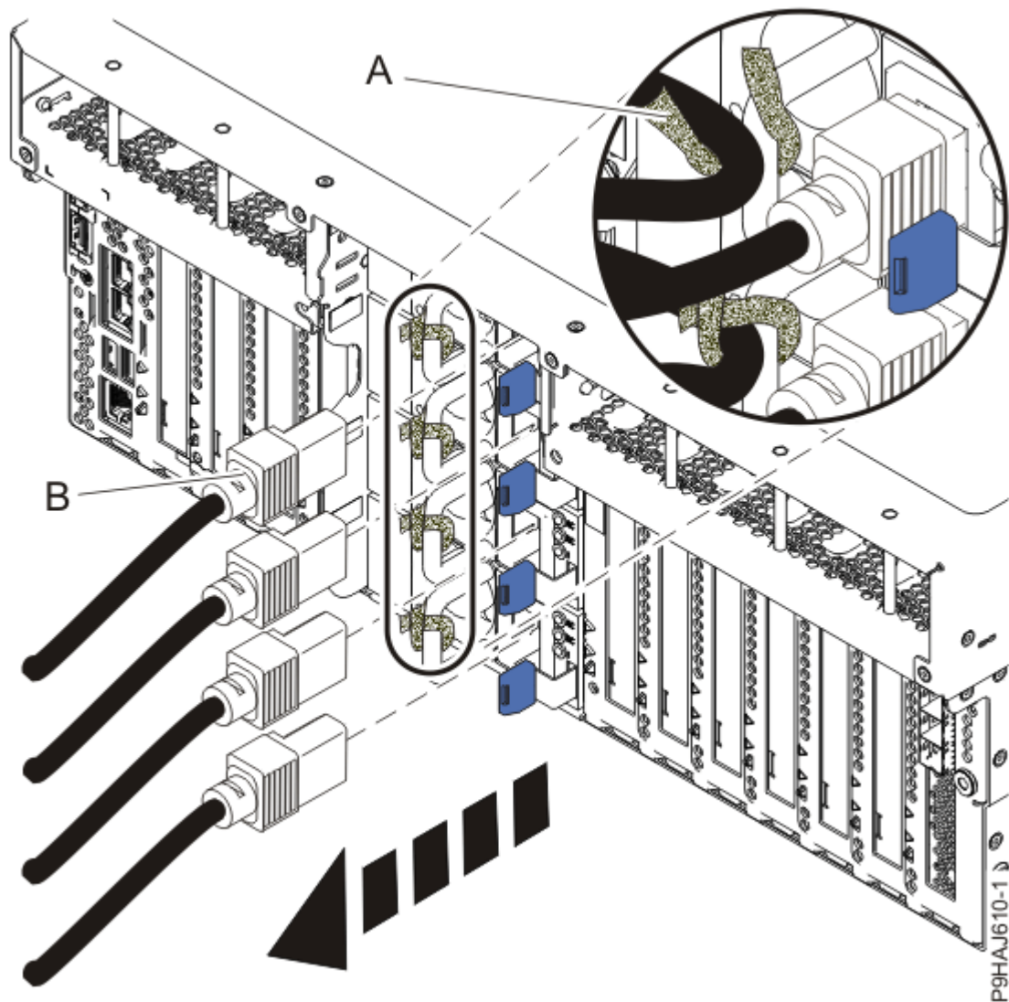
Abbildung 1. Netzkabel von einem Einschubserver entfernen
