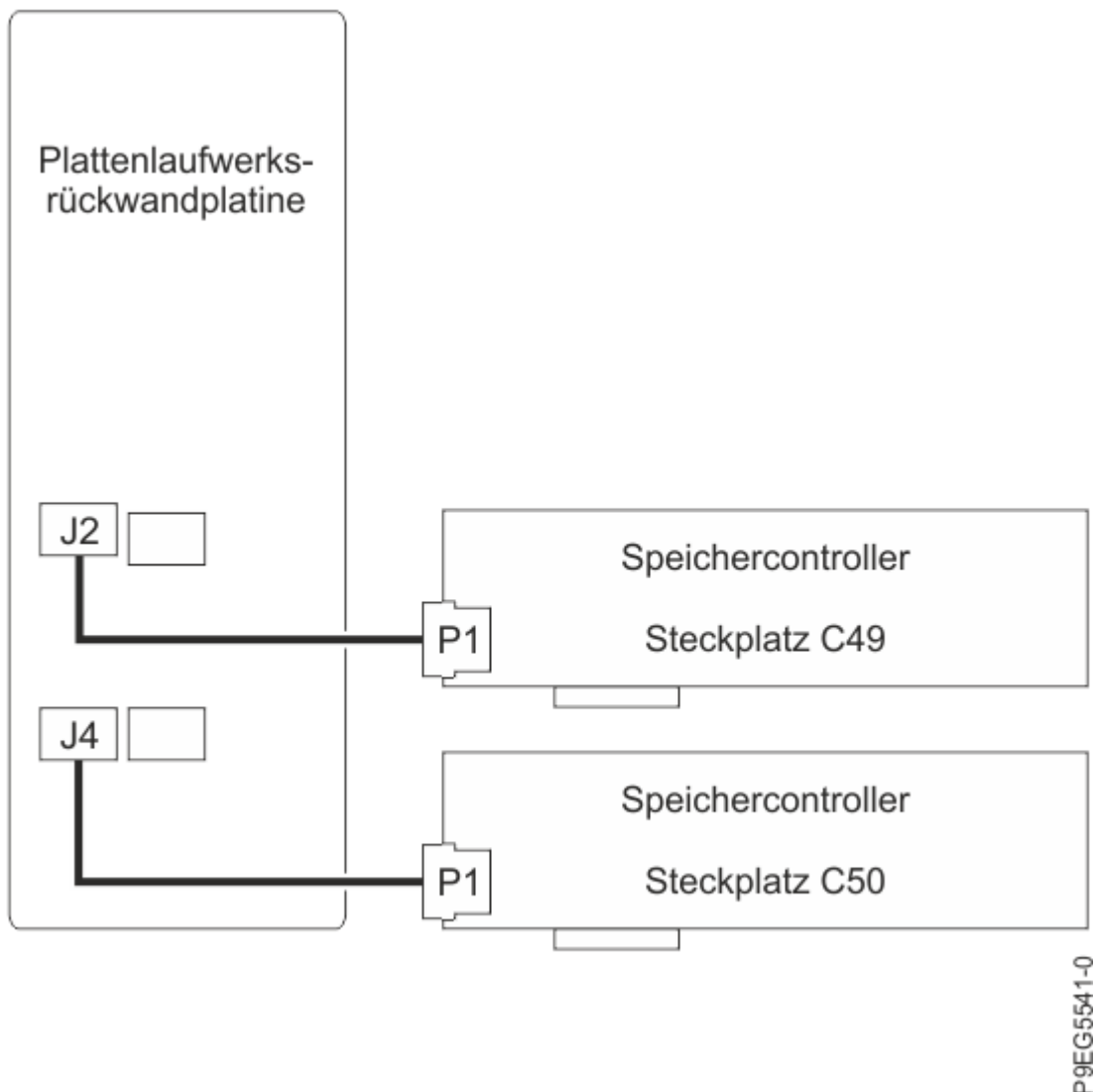
Abbildung 15. SAS-Kabel in einer Konfiguration vom Typ "12-Laufwerk mit erweiterter Funktion" wieder anschließen
