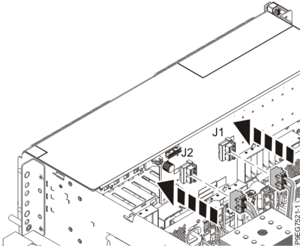
Abbildung 11. Vordere SAS-Kabel an der Plattenlaufwerk-Rückwandplatine mit Basisfunktion wieder anschließen
