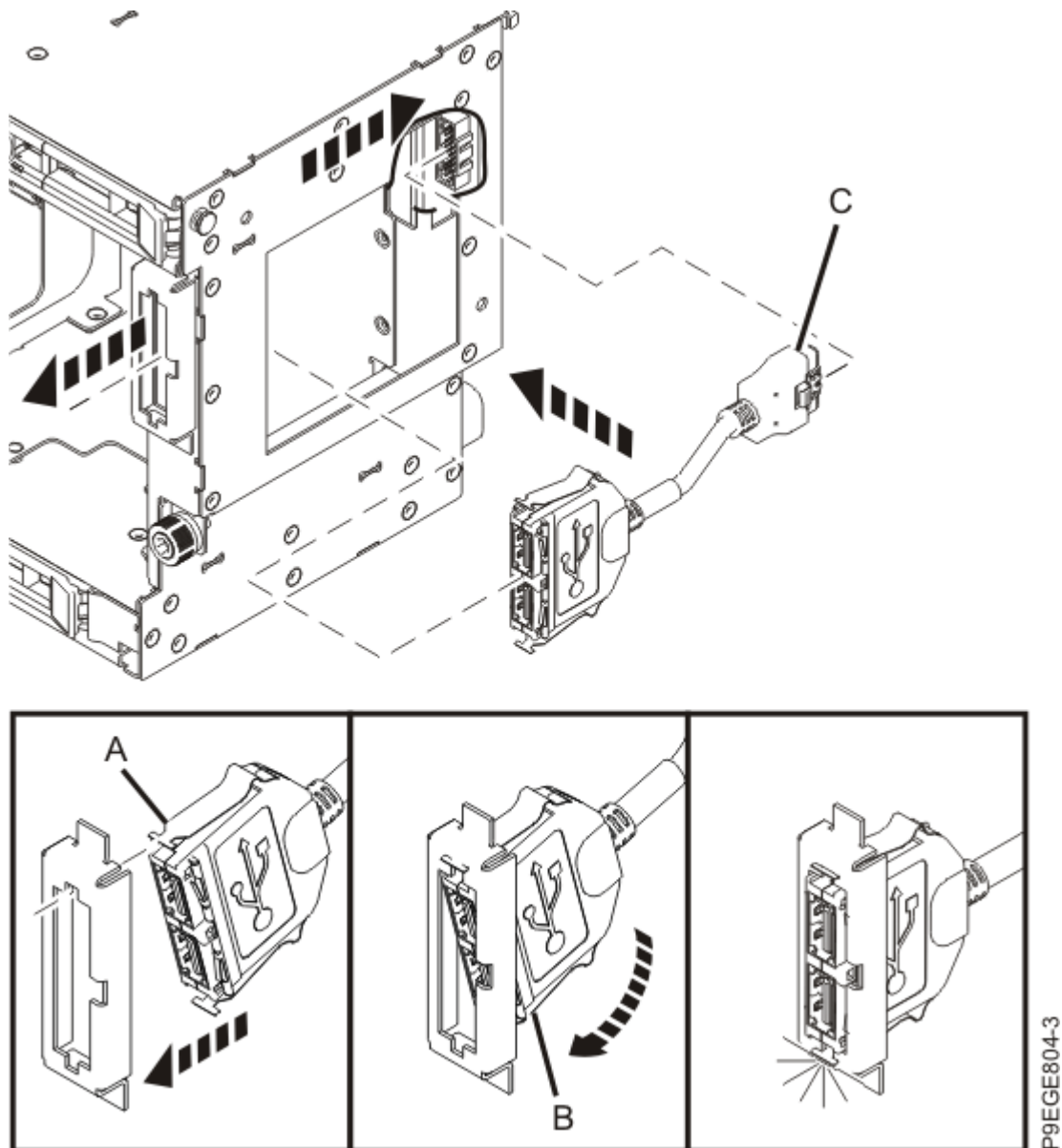
Abbildung 18. USB-Anschlusstecker an der Vorderseite austauschen
