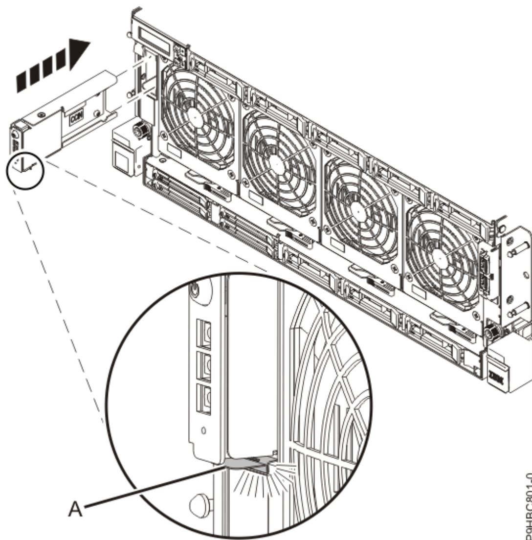
Abbildung 27. Steuerkonsole wiedereinbauen
