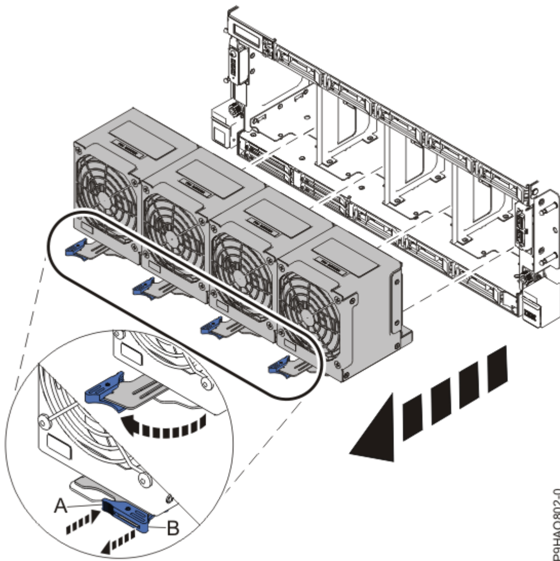
Abbildung 10. Lüfter ausbauen
