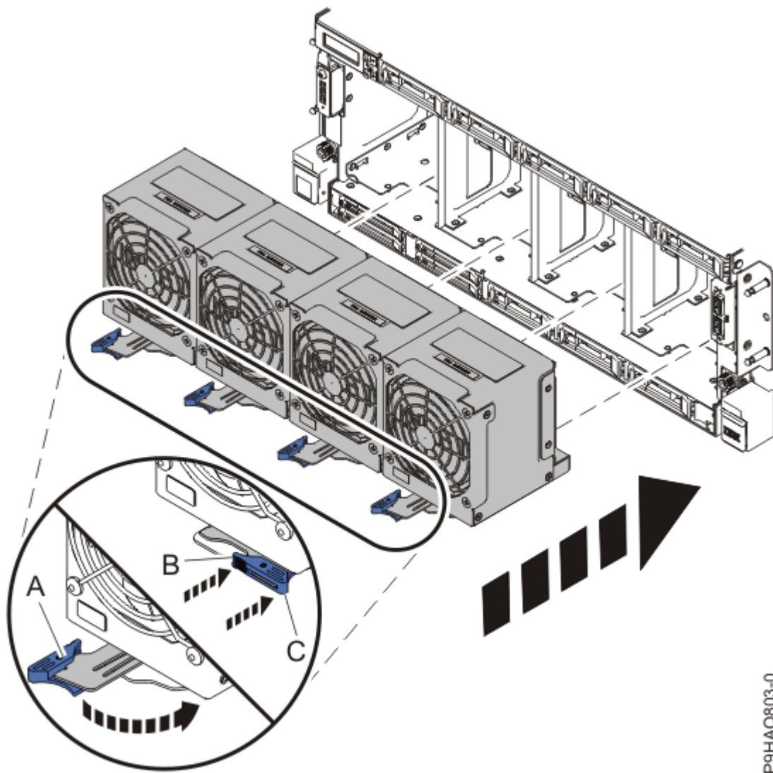
Abbildung 26. Lüfter wiedereinbauen
