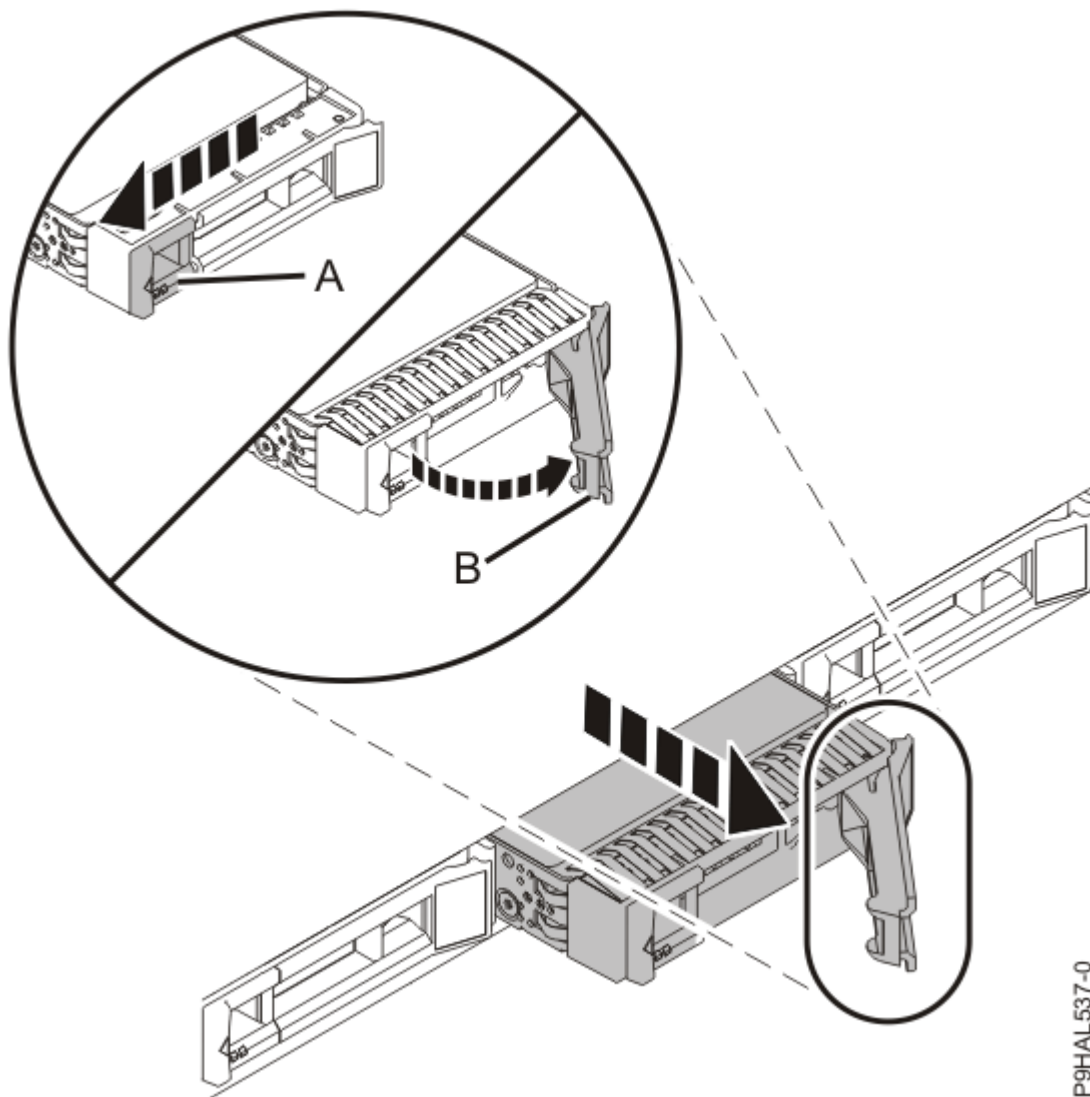
Abbildung 6. Laufwerk entriegeln und ausbauen
