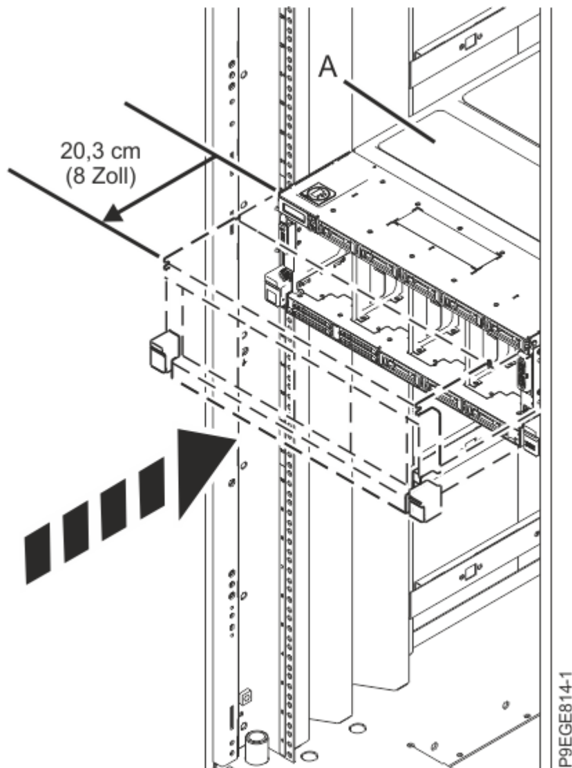
Abbildung 24. System in die Betriebsposition bringen
