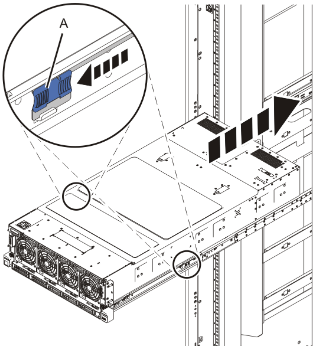
Abbildung 33. System in die Betriebsposition bringen
