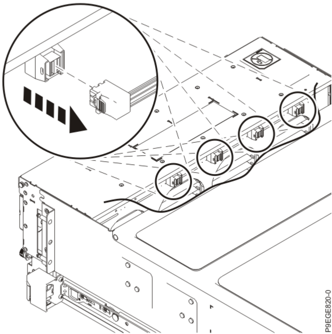
Abbildung 15. SAS-Kabel von der Rückwandplatine des erweiterten Plattenlaufwerks abziehen f) Ziehen Sie die Plattenlaufwerksrückwandplatine mit beiden aus dem System.
