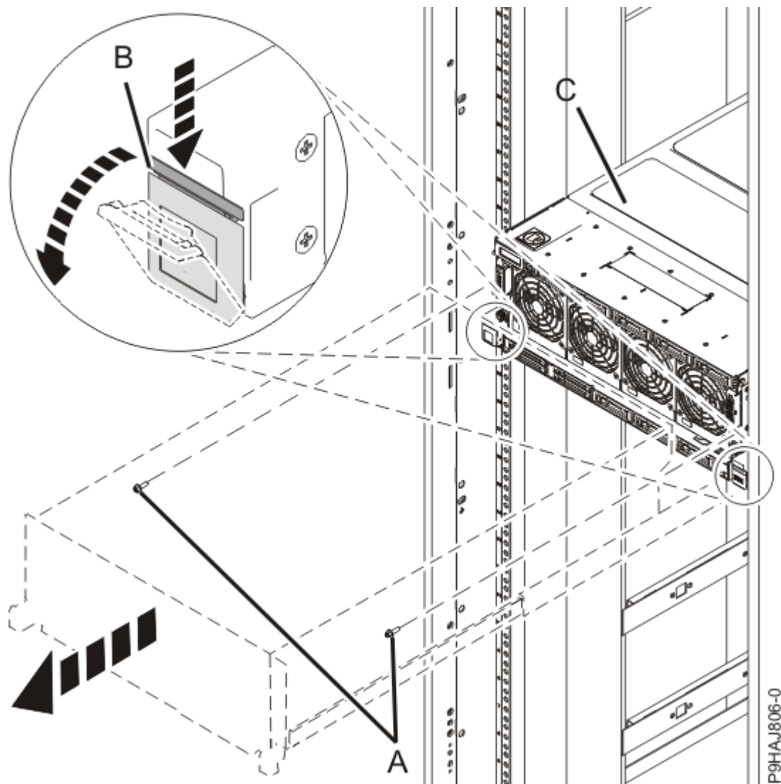
Abbildung 3. System in die Serviceposition bringen
