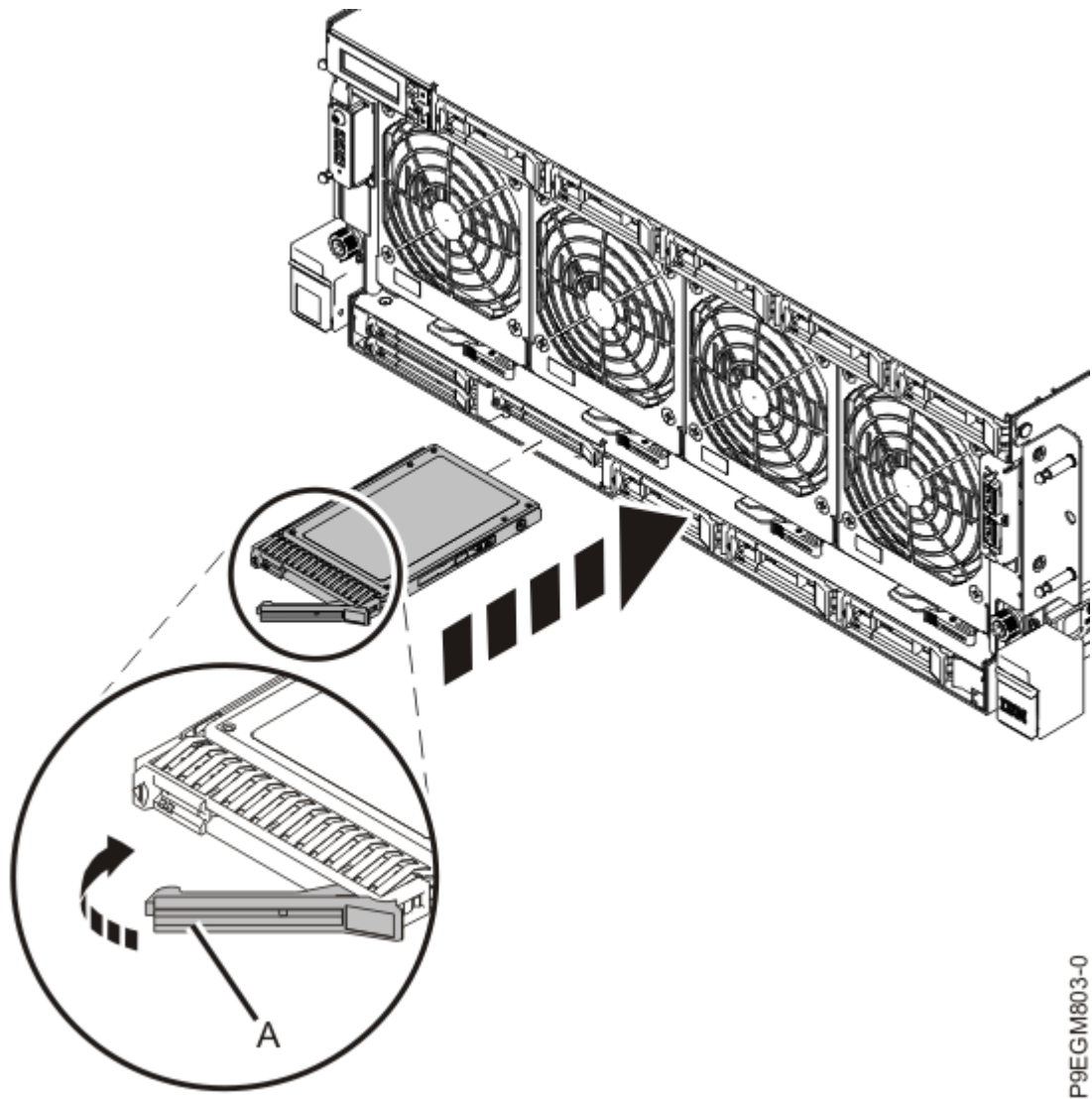
Abbildung 29. NVMe-U.2-Laufwerk im System vom Typ 9040-MR9 installieren oder wiedereinbauen
