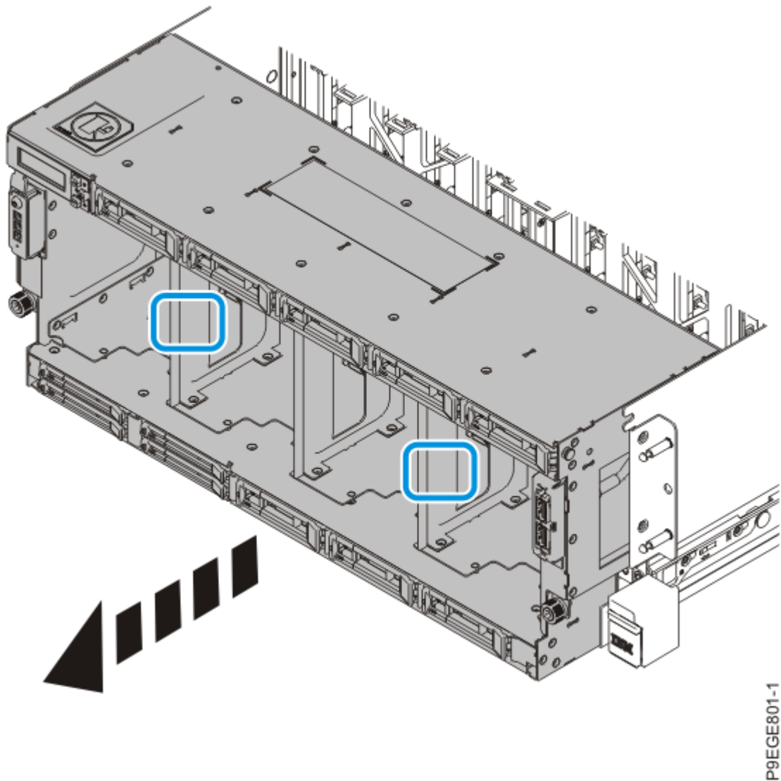
Abbildung 12. Plattenlaufwerksrückwandplatte teilweise ausbauen
