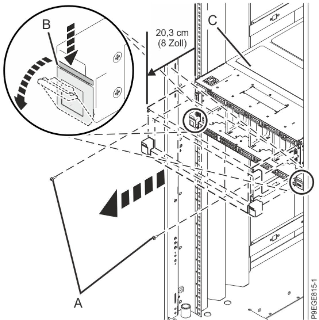
Abbildung 13. System teilweise aus dem Rack schieben
