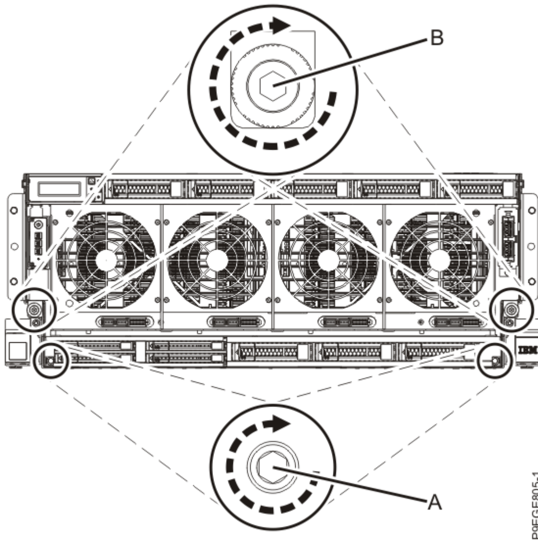
Abbildung 25. Schrauben für die Plattenlaufwerksrückwandplatine festziehen
