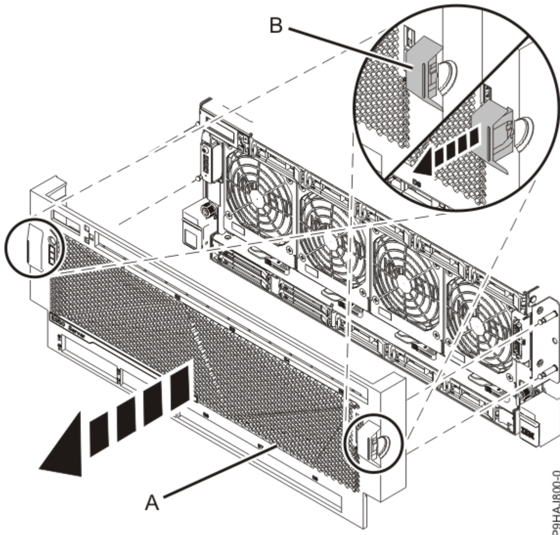
Abbildung 2. Vordere Abdeckung ausbauen
