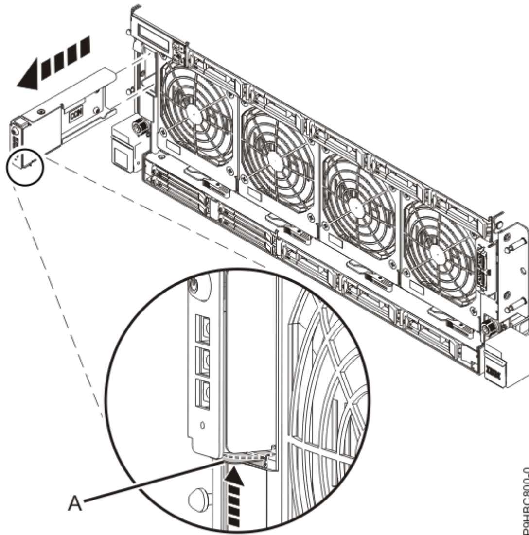
Abbildung 8. Steuerkonsole ausbauen
