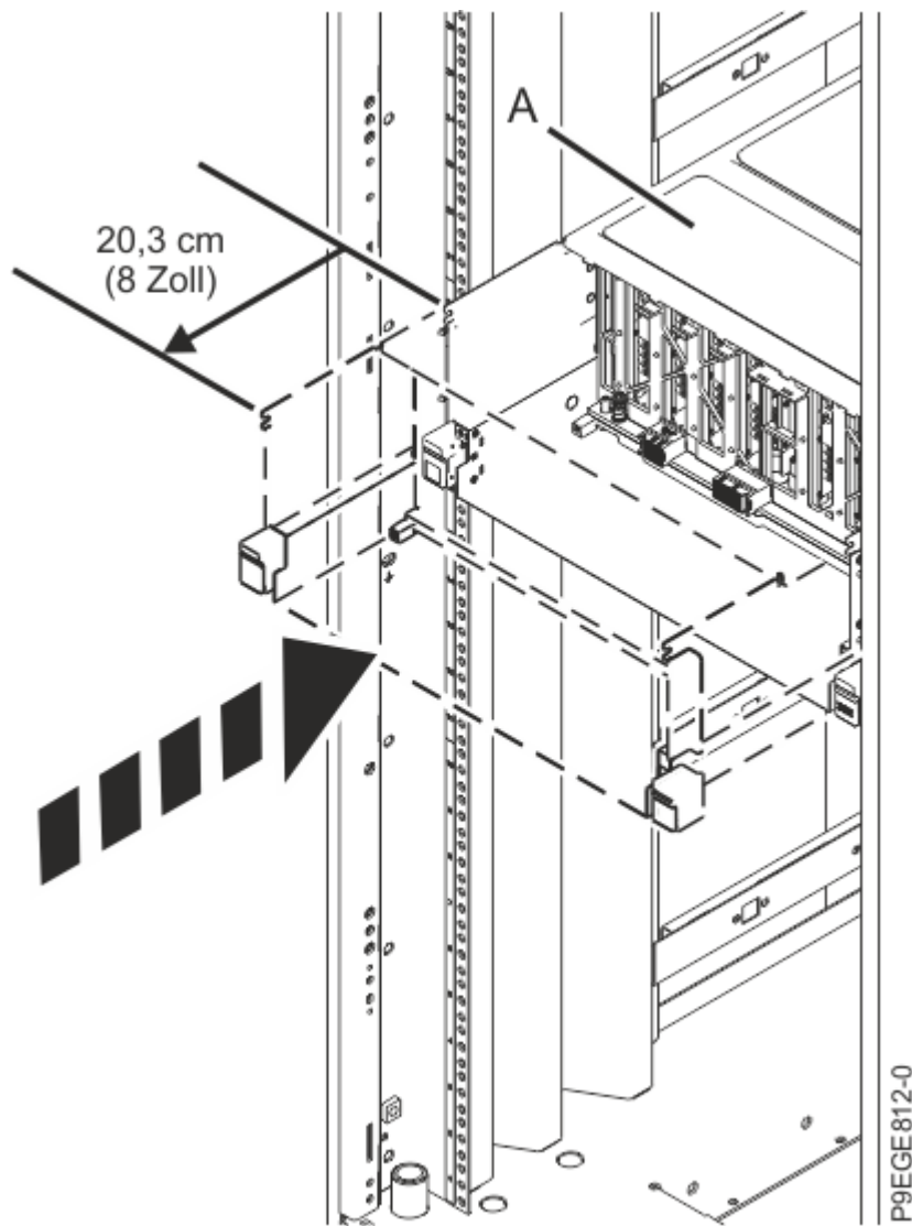
Abbildung 20. System teilweise in das Rack schieben
