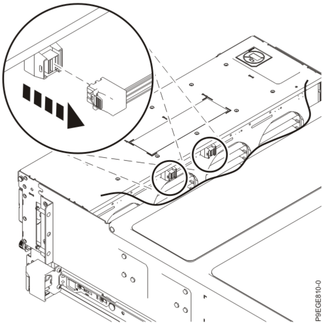
Abbildung 14. SAS-Kabel von der Rückwandplatine des Basisplattenlaufwerks abziehen
