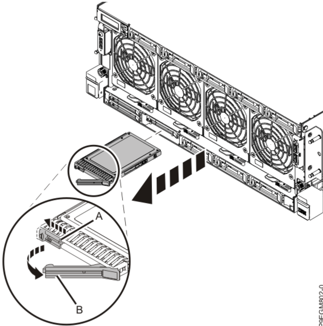
Abbildung 7. NVMe-U.2-Laufwerk aus dem System vom Typ 9040-MR9 ausbauen
