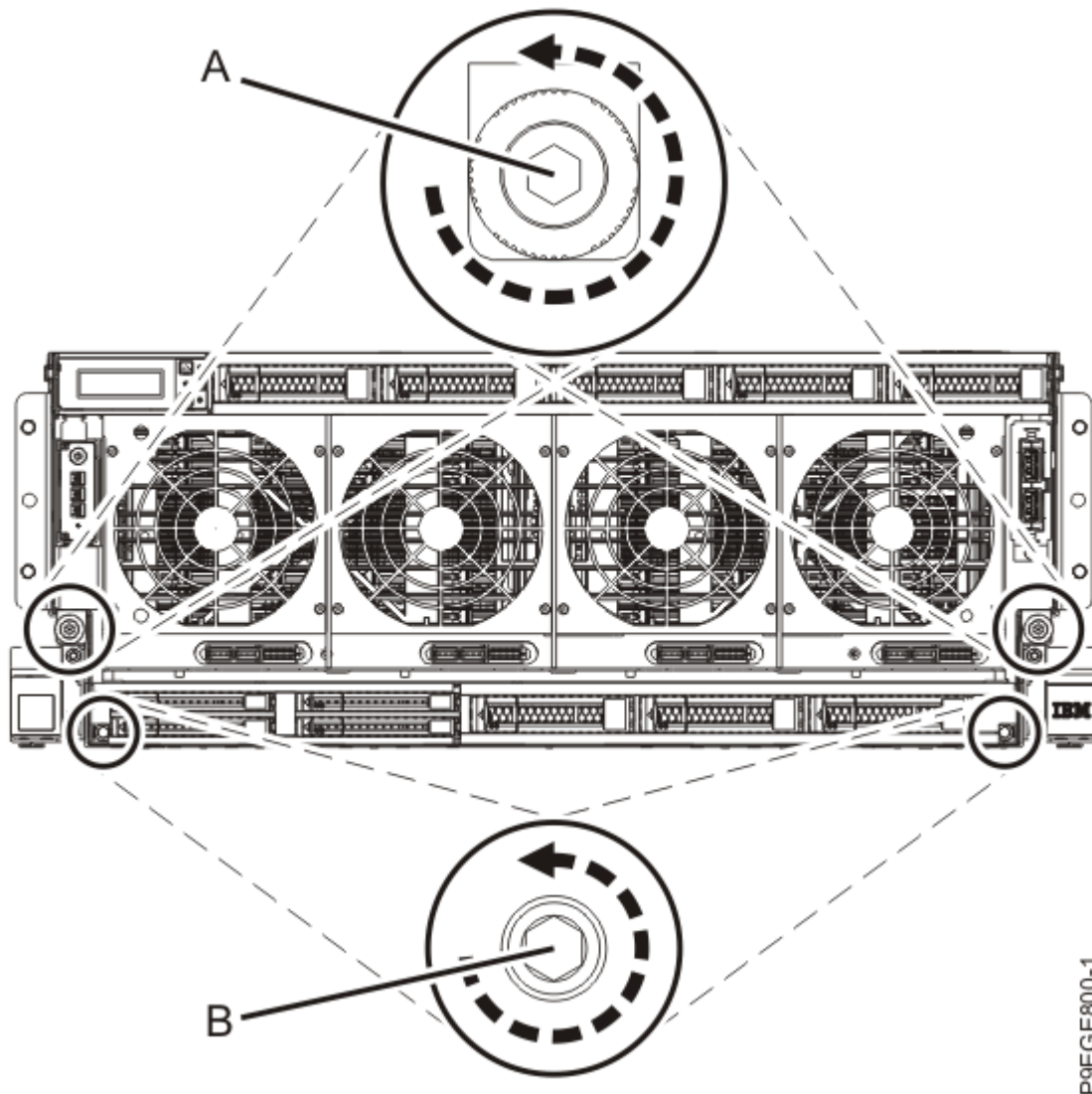
Abbildung 11. Schrauben der Plattenlaufwerksrückwandplatine lösen
