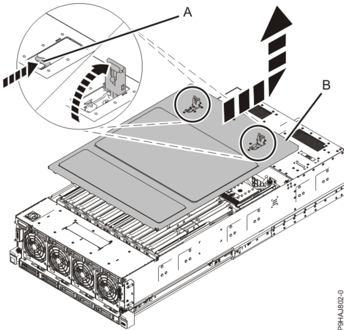
Abbildung 4. Serviceabdeckung ausbauen
