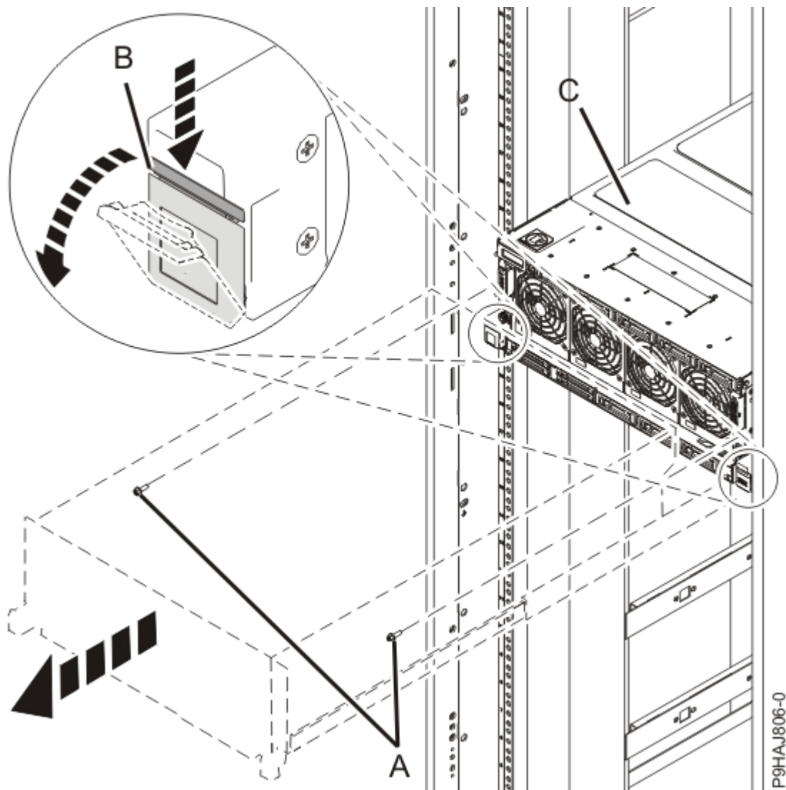
Abbildung 31. System in die Serviceposition bringen
