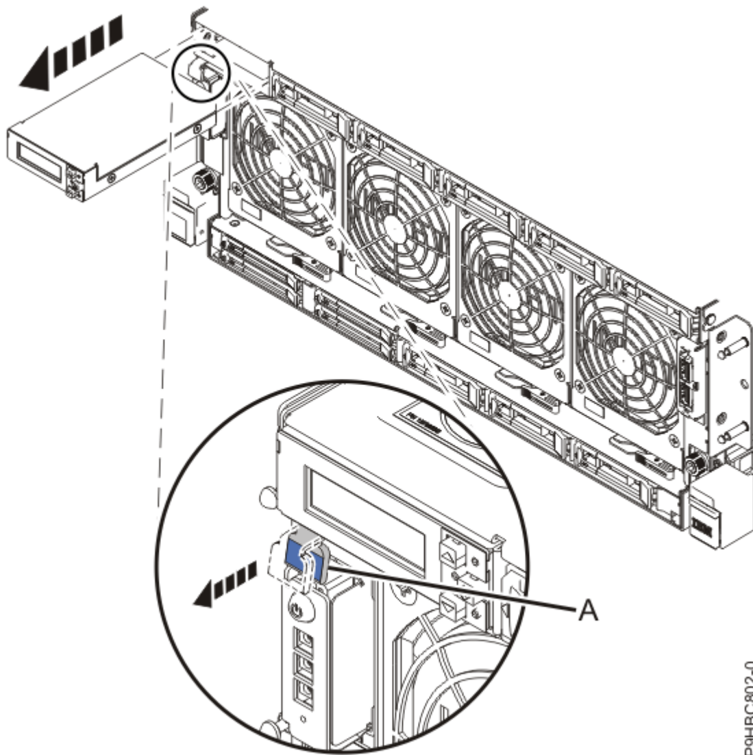
Abbildung 9. Steuerkonsolenanzeige ausbauen
