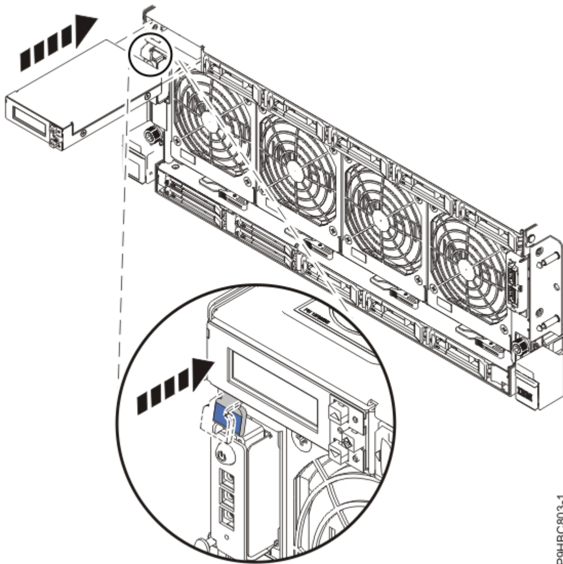
Abbildung 28. Steuerkonsolenanzeige wiedereinbauen
