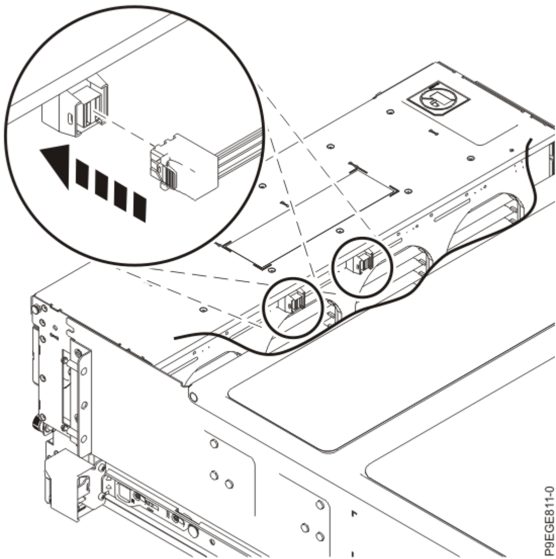
Abbildung 21. SAS-Kabel an die Plattenlaufwerksrückwandplatine (Basisfunktion) anschließen
