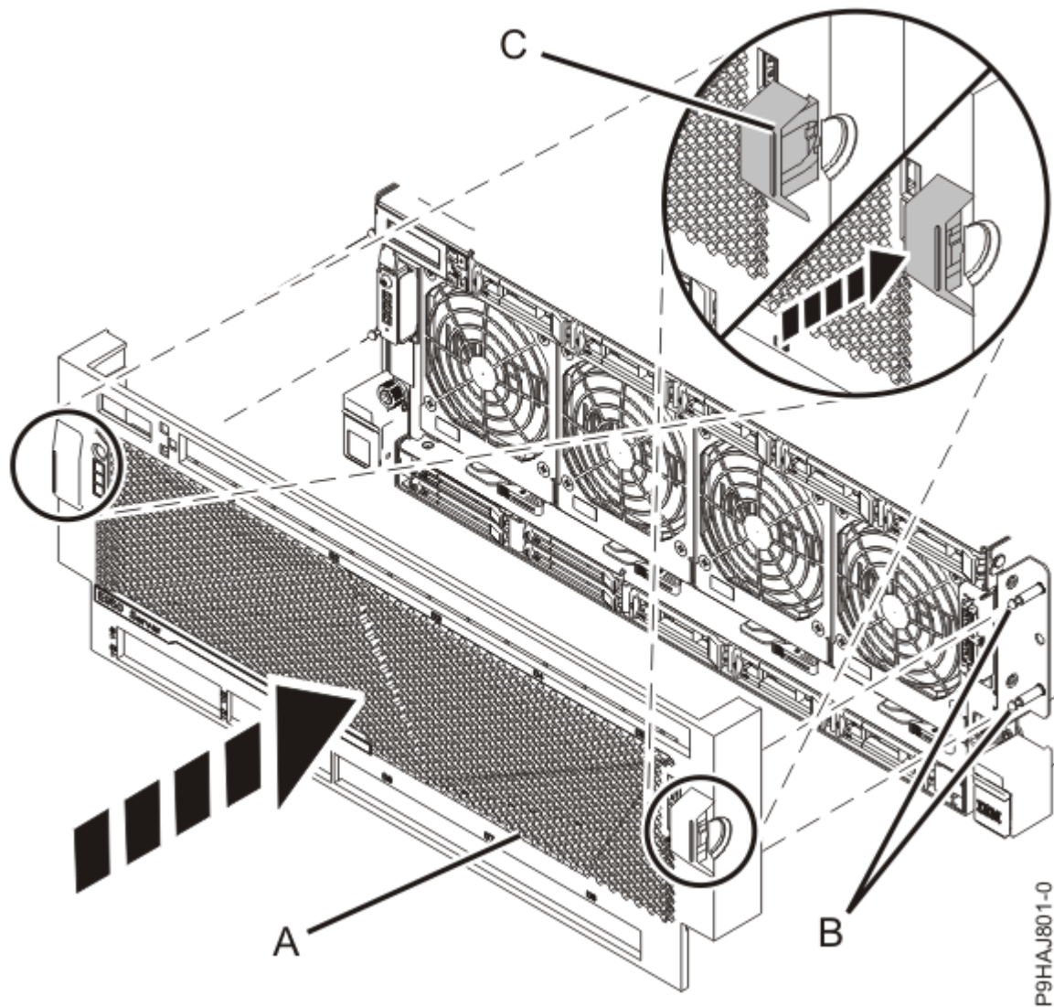
Abbildung 34. Vordere Abdeckung installieren
