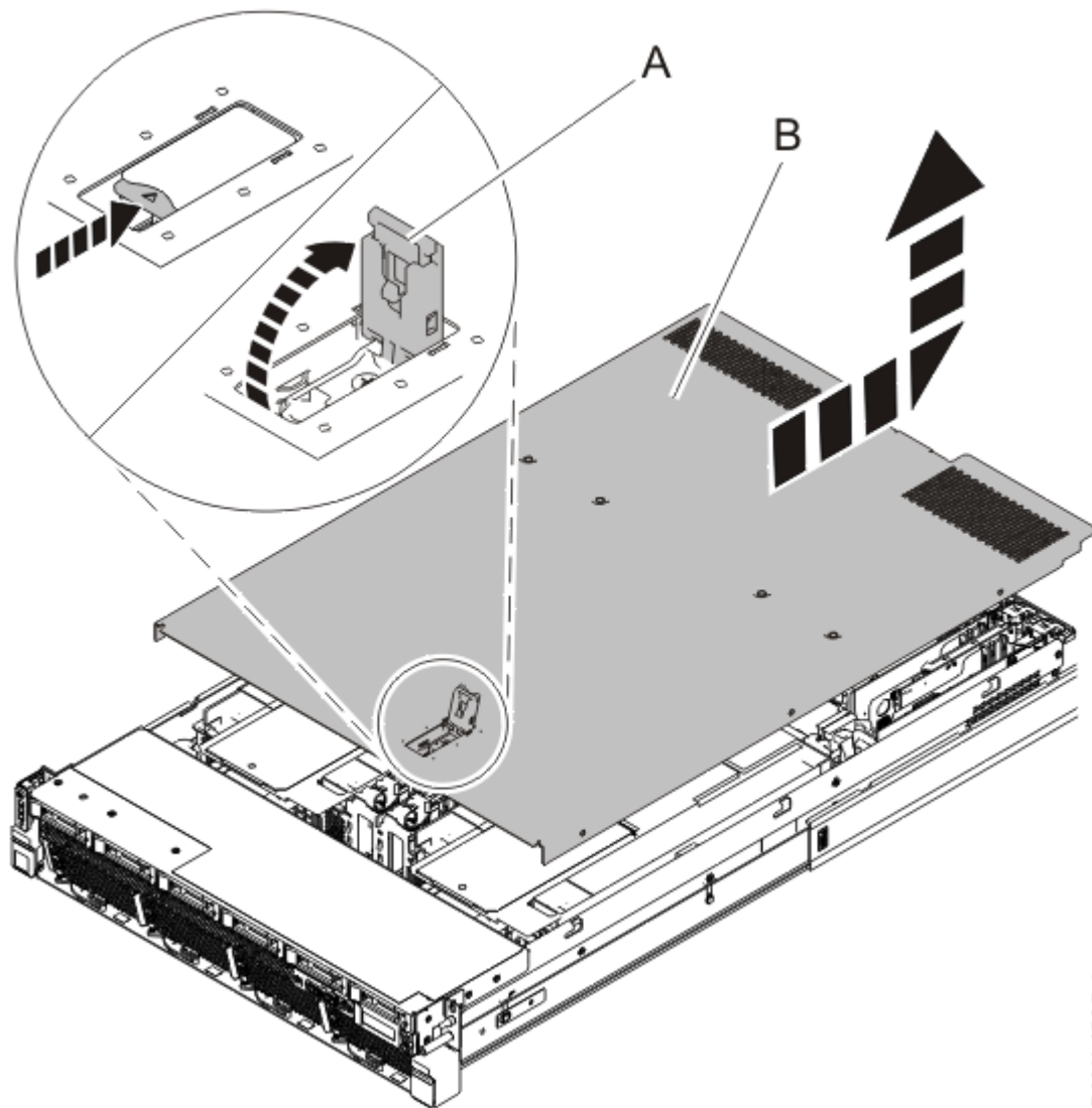
Abbildung 39. Serviceabdeckung ausbauen
