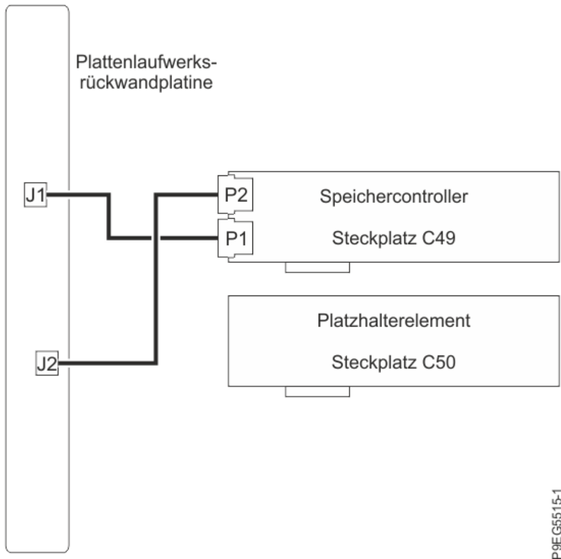
Abbildung 17. SAS-Kabel bei der Konfiguration mit Basisspeicher wieder anschließen
