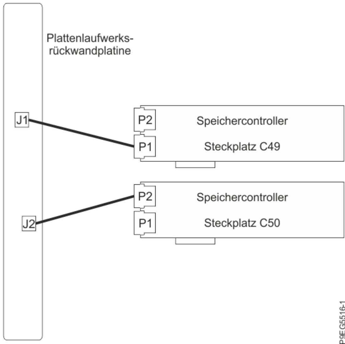
Abbildung 18. SAS-Kabel bei einer Konfiguration mit unterteilter Festplatte wieder anschließen
