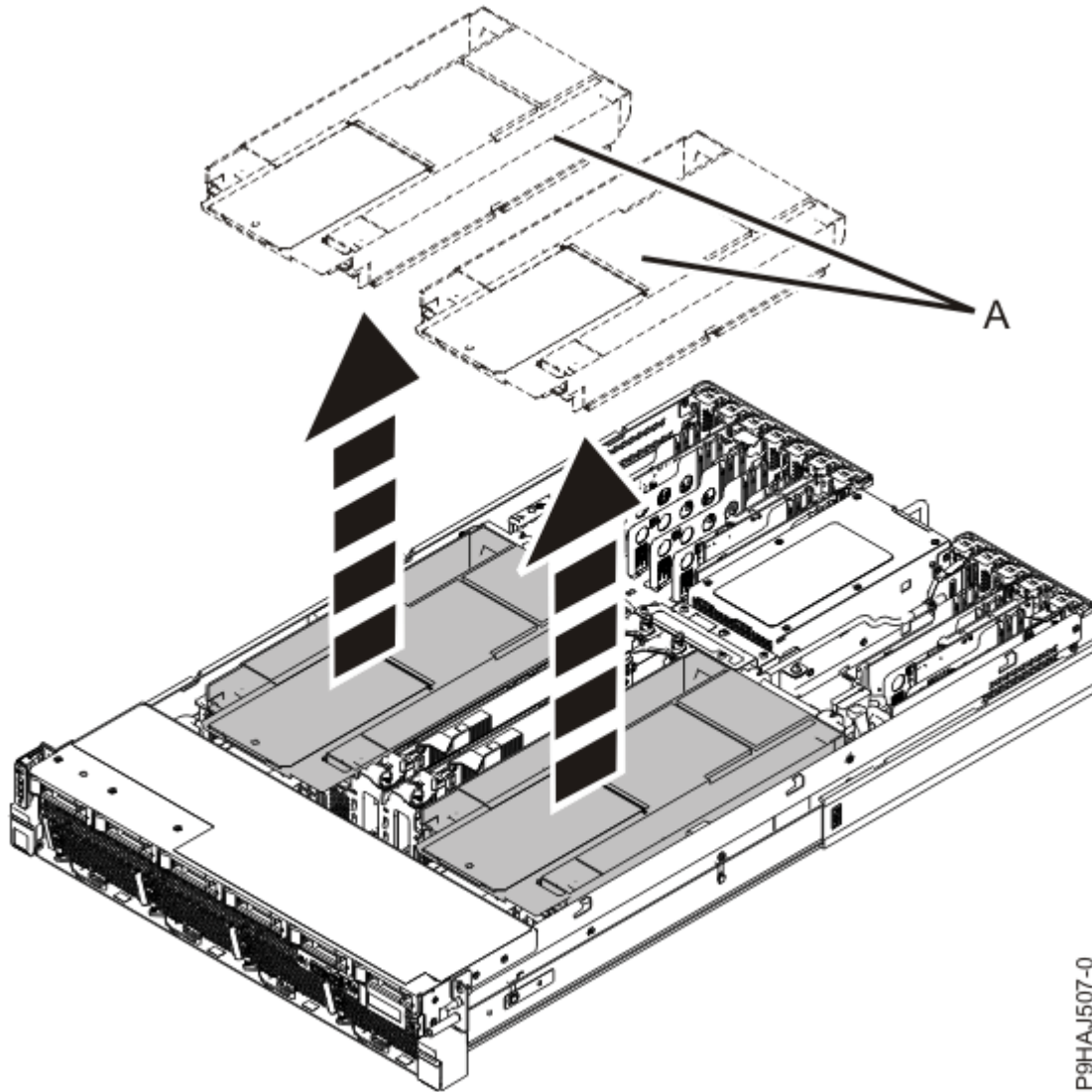
Abbildung 31. Luftführung ausbauen
