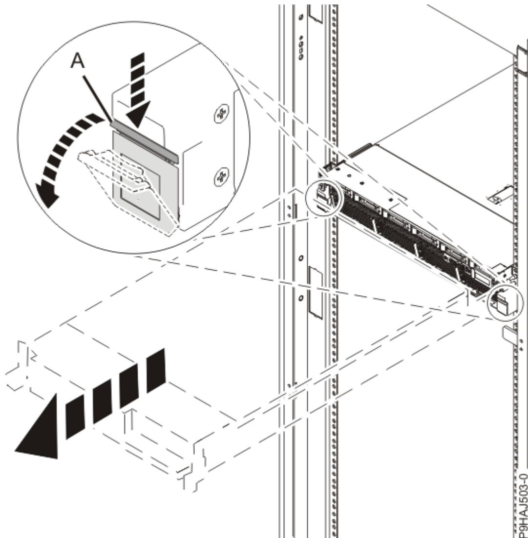
Abbildung 28. Seitliche Verriegelungen entriegeln
