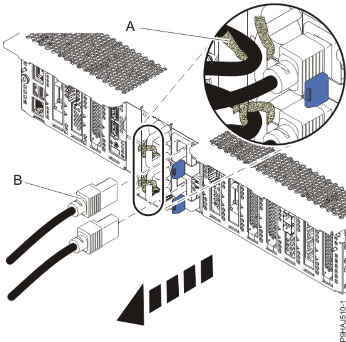
Abbildung 27. Netzkabel abziehen
