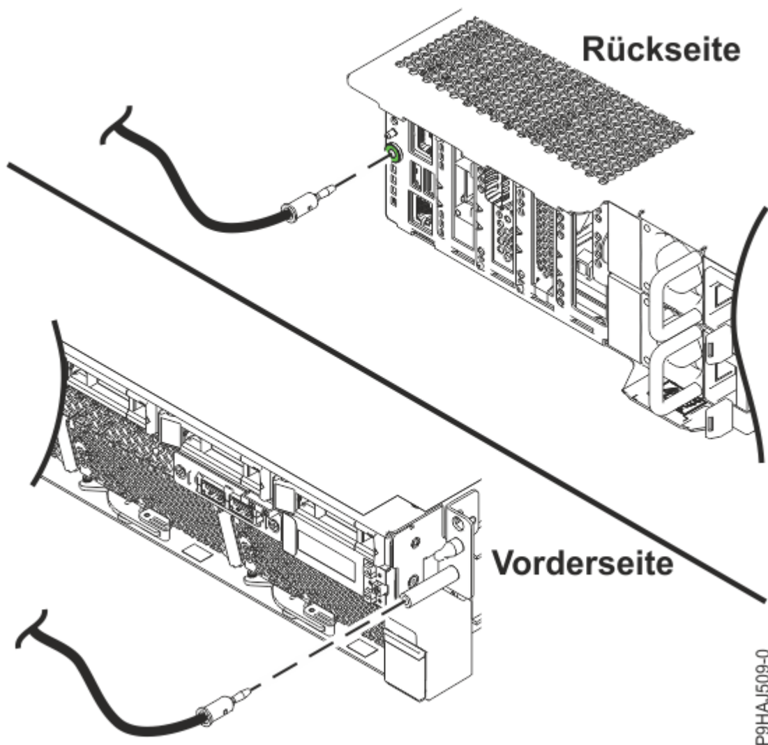
Abbildung 29. Position der ESD-Stecker
