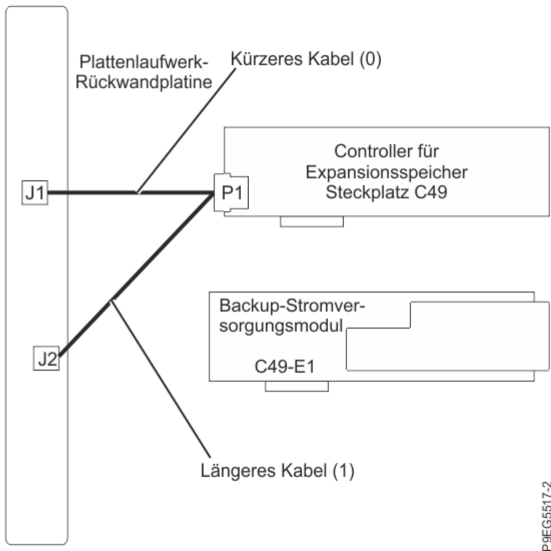
Abbildung 19. SAS-Kabel "Y" bei einer Konfiguration des leistungsfähigen Speichercontrollers wieder anschließen
