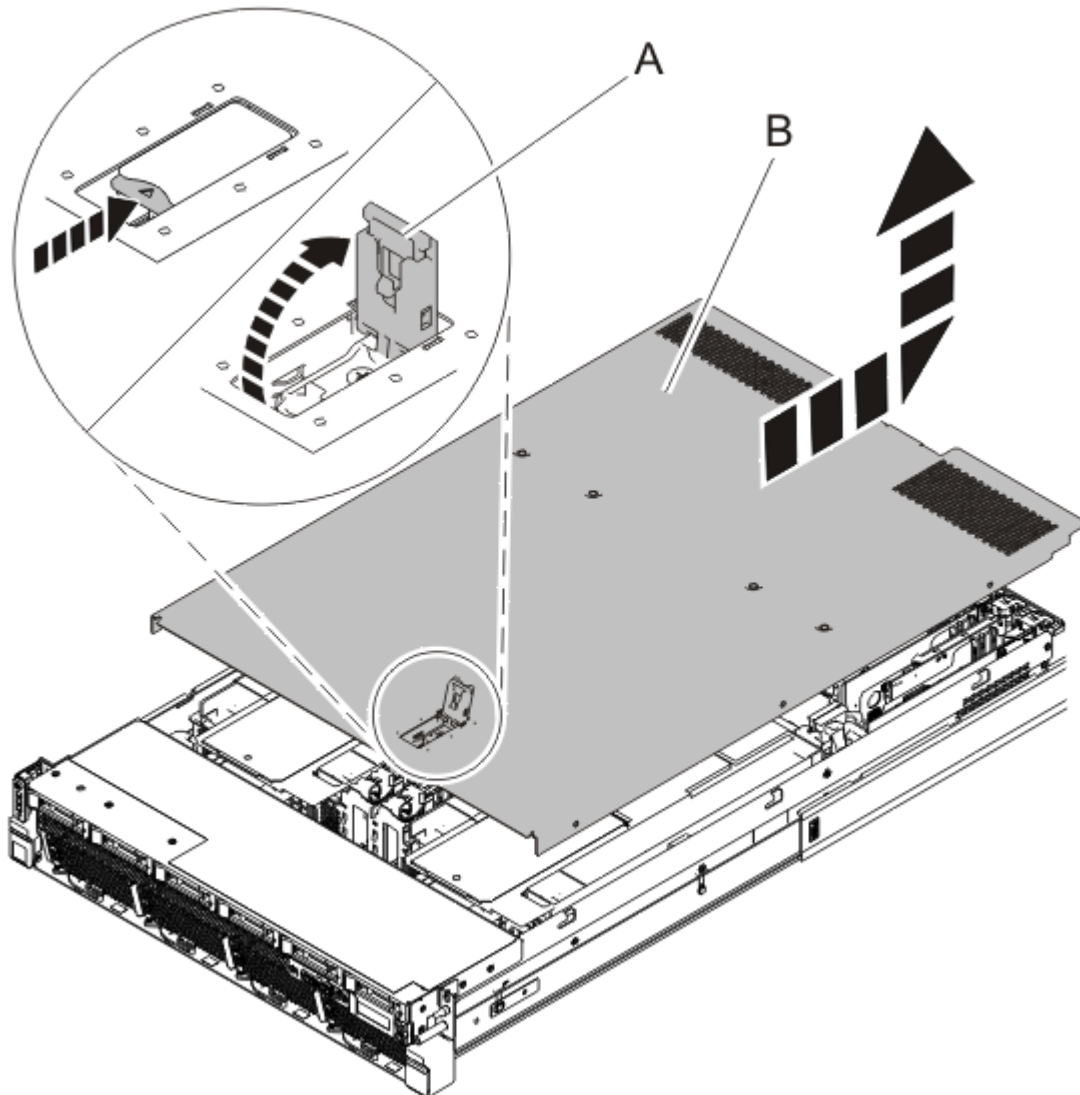
Abbildung 30. Serviceabdeckung ausbauen
