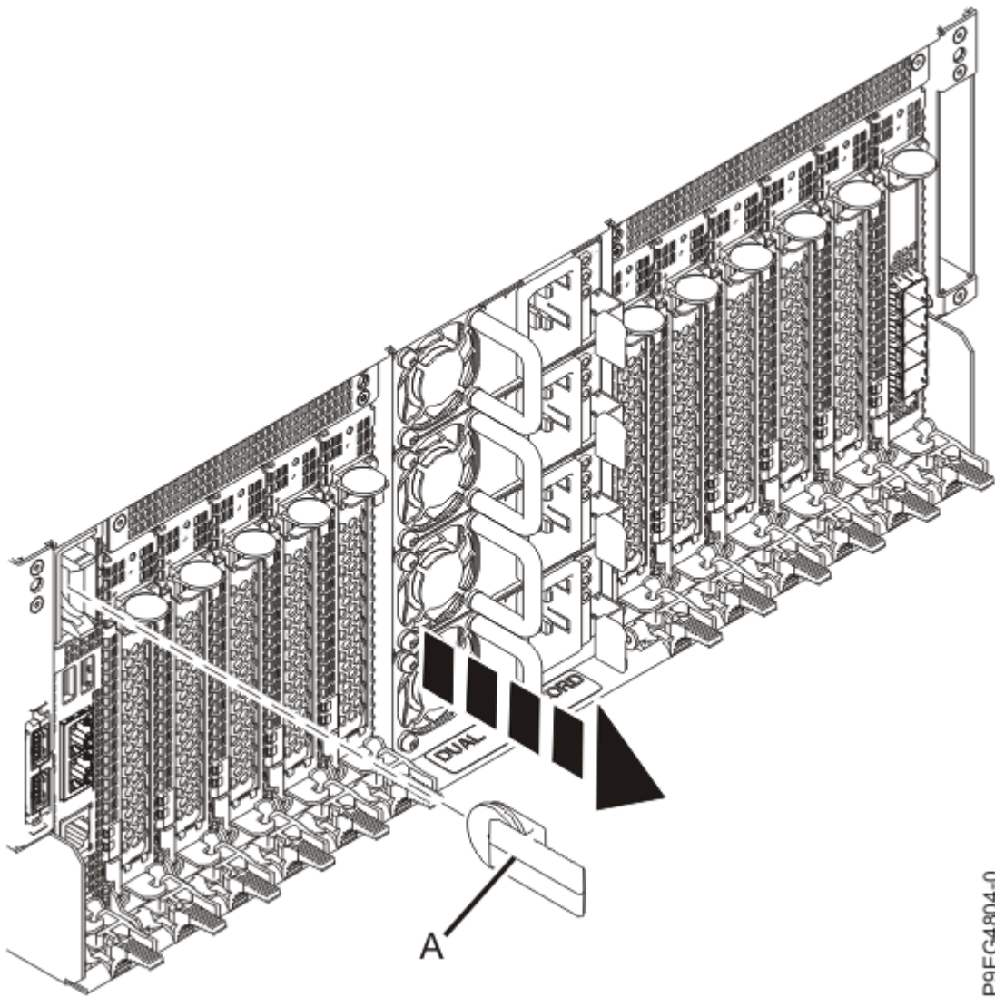
Abbildung 3. Uhrzeitbatterie entfernen
