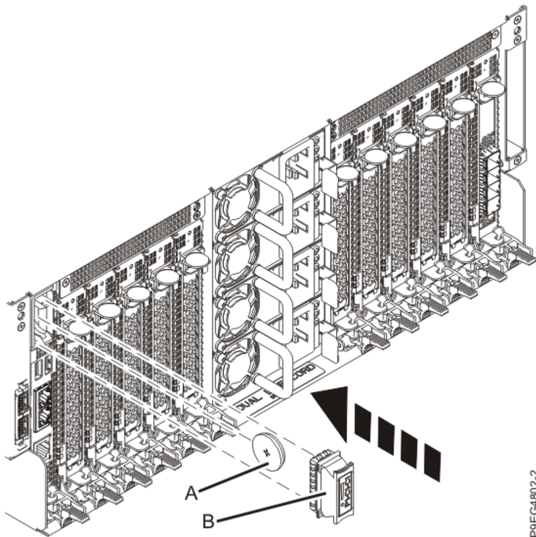
Abbildung 4. Uhrzeitbatterie einsetzen
