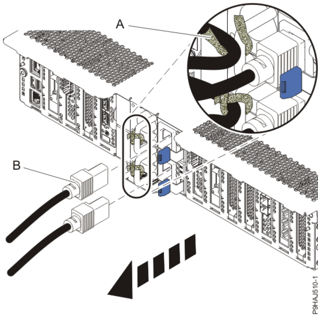
Abbildung 1. Netzkabel abziehen
