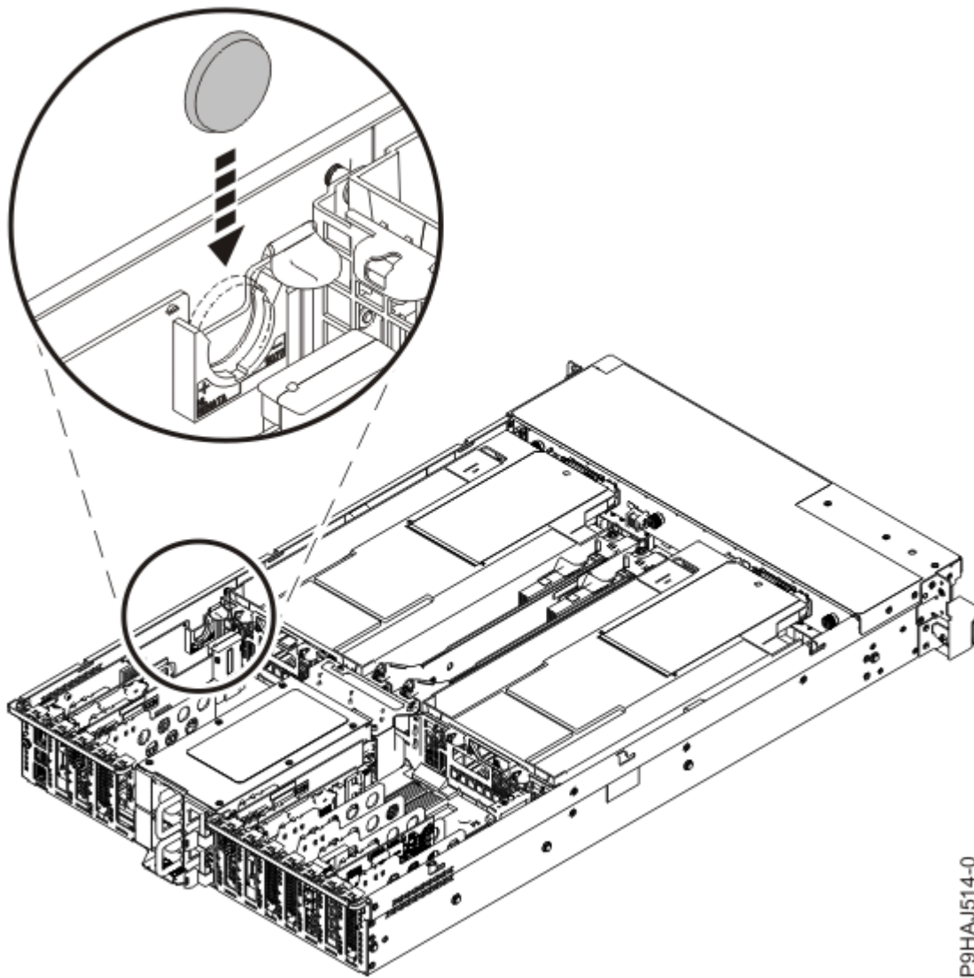
Abbildung 6. Uhrzeitbatterie einsetzen
