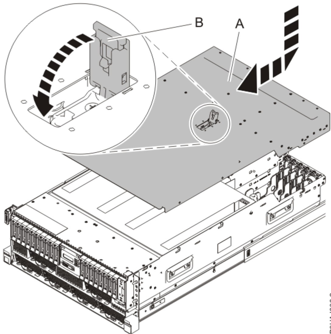
Abbildung 11. Serviceabdeckung installieren
