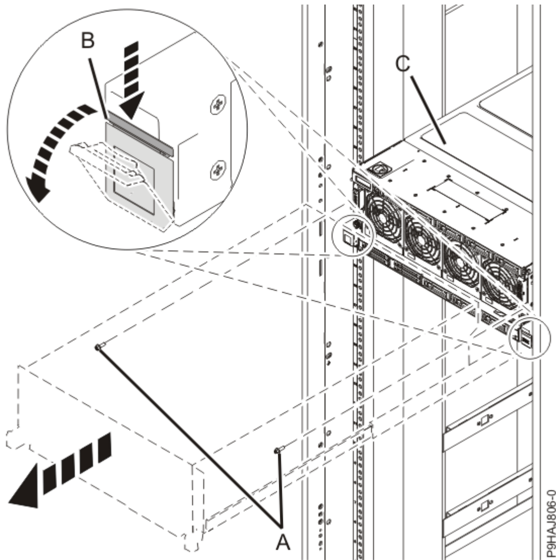
Abbildung 2. System in Serviceposition bringen
