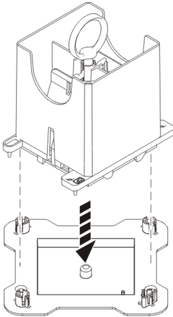
Abbildung 11. Werkzeug um 45 Grad gedreht auf der oberen Abdeckung der Verpackung platzieren
