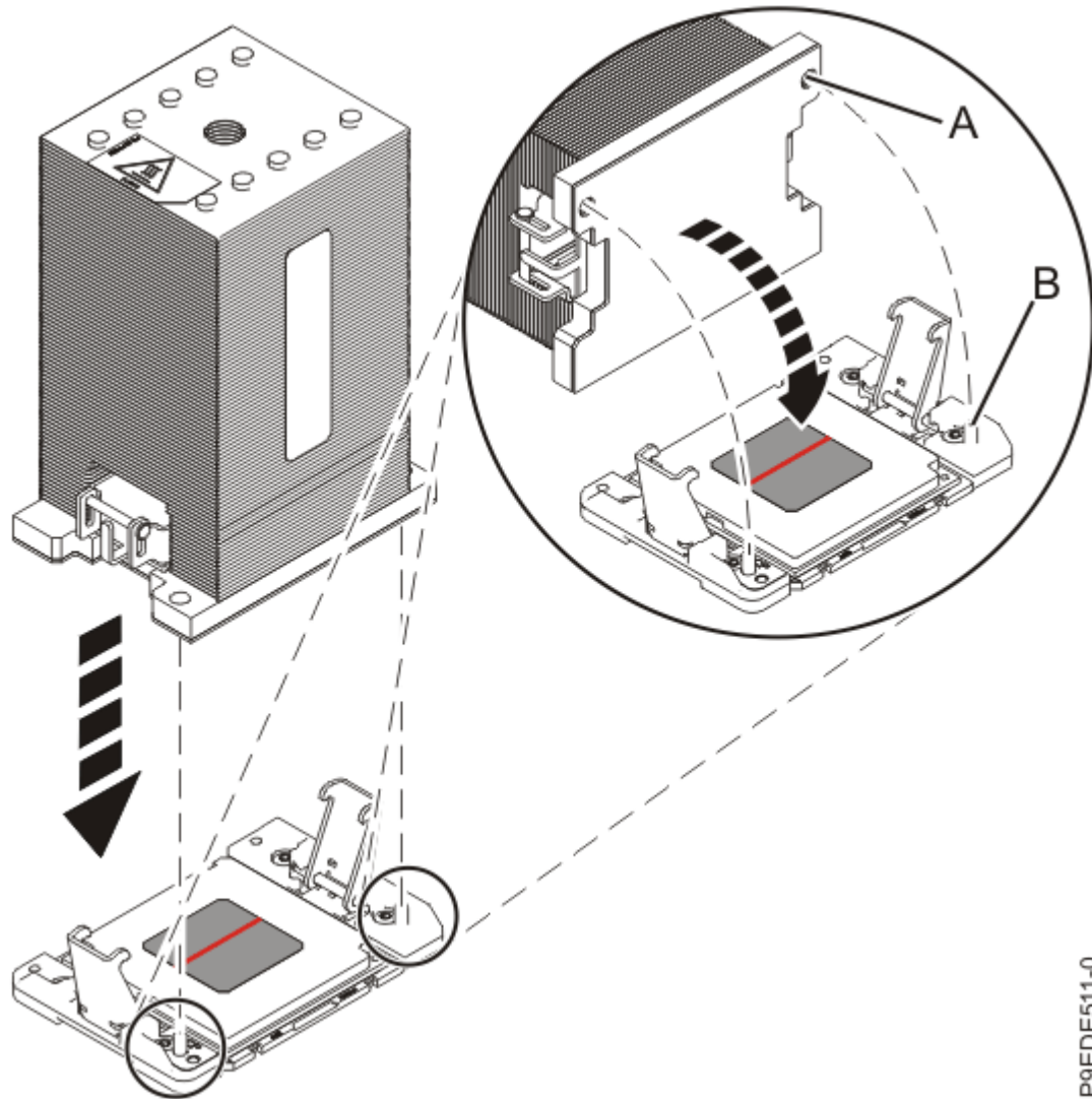
Abbildung 20. Kühlblech auf dem silberfarbenen TIM installieren
