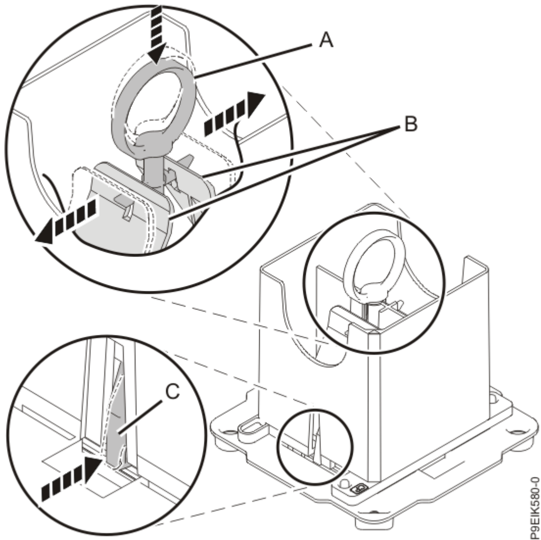
Abbildung 15. Systemprozessormodul im Werkzeug einrasten lassen
