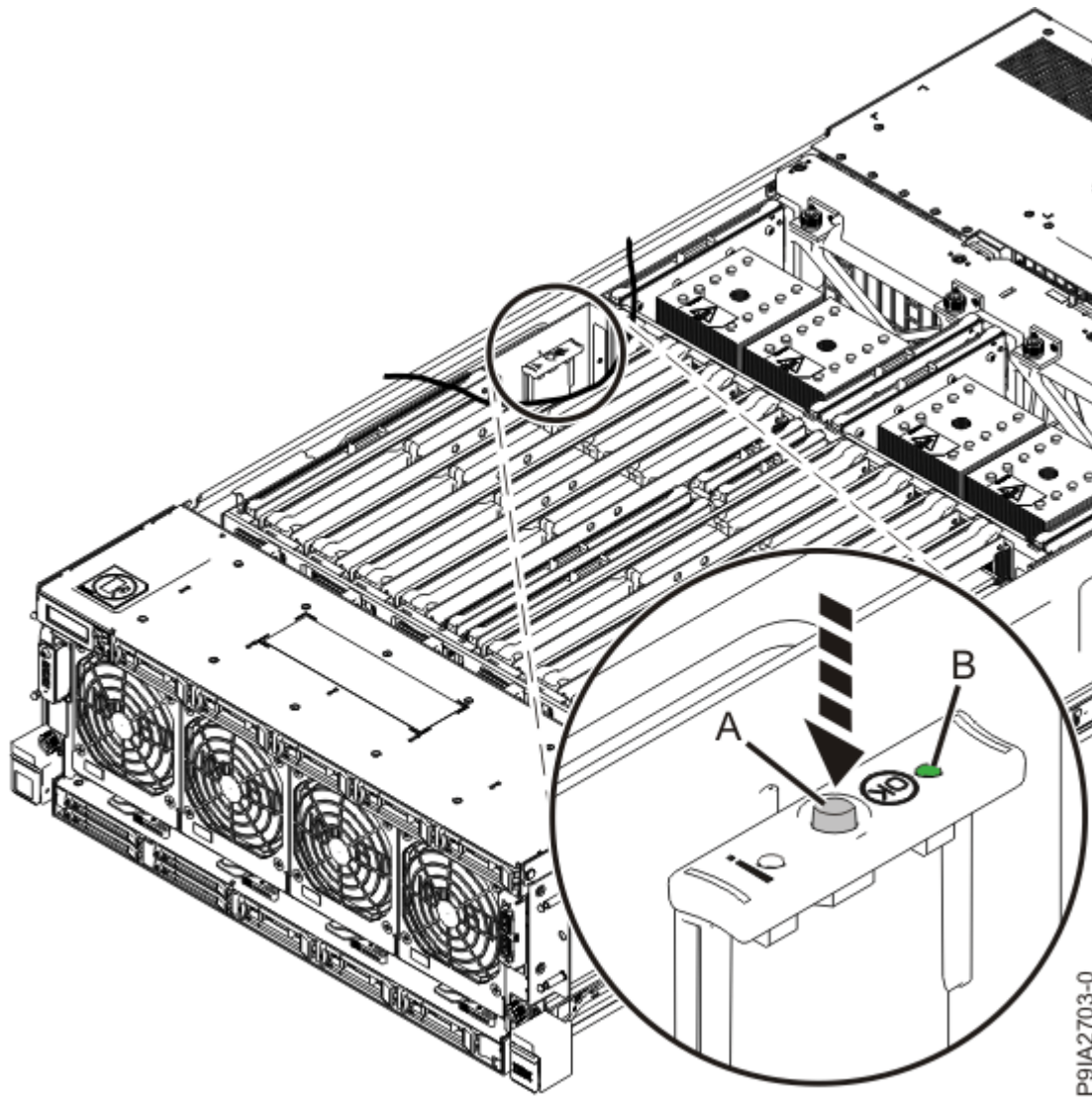
Abbildung 4. Kennzeichnungs-LED aktivieren
