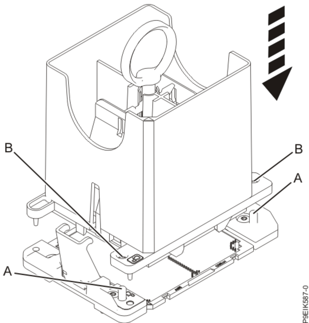
Abbildung 17. Systemprozessormodul installieren
