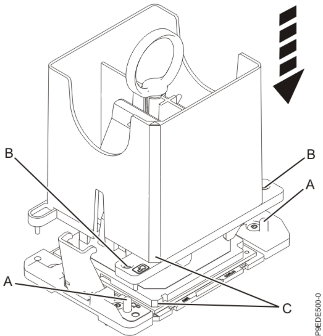
Abbildung 9. Ausbauwerkzeug auf das Systemprozessormodul herabsenken
