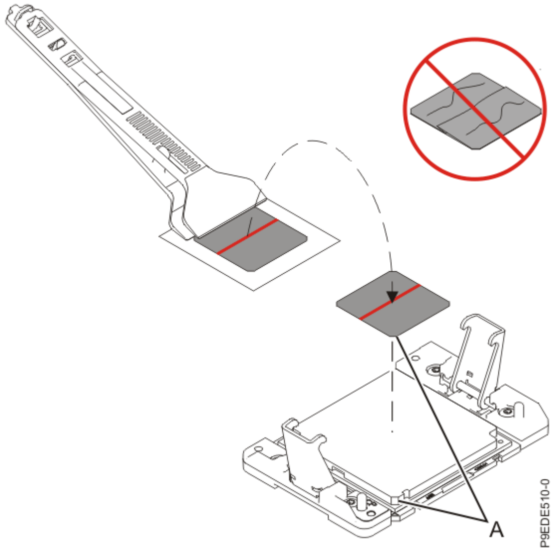
Abbildung 19. Installieren des silberfarbenen TIM auf dem Systemprozessormodul
