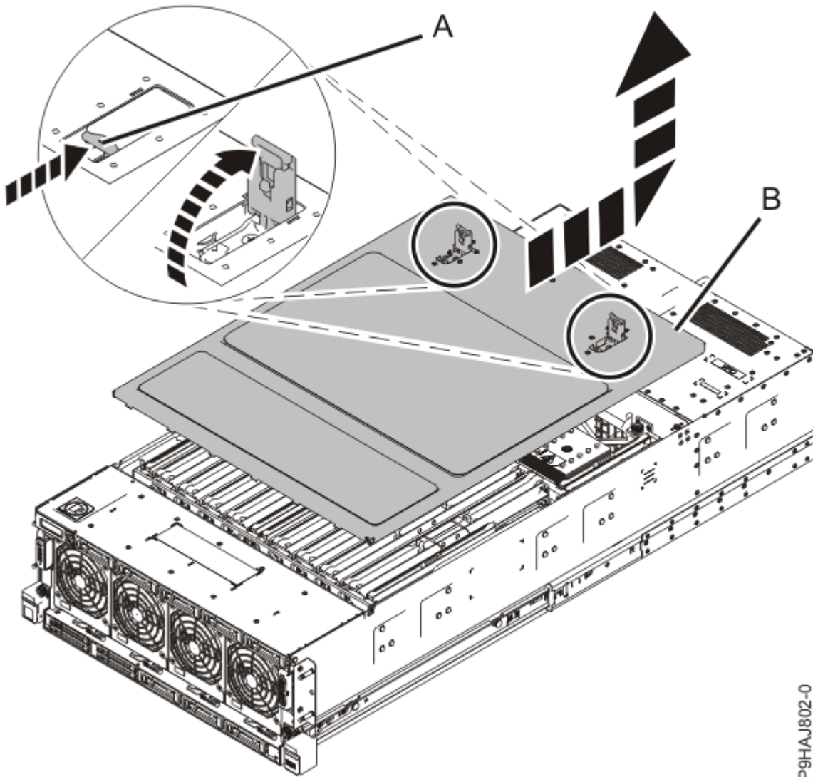
Abbildung 3. Serviceabdeckung ausbauen
