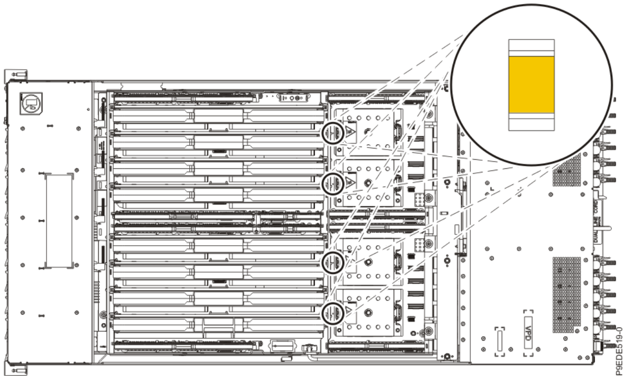
Abbildung 5. LEDs für ein Systemprozessormodul
