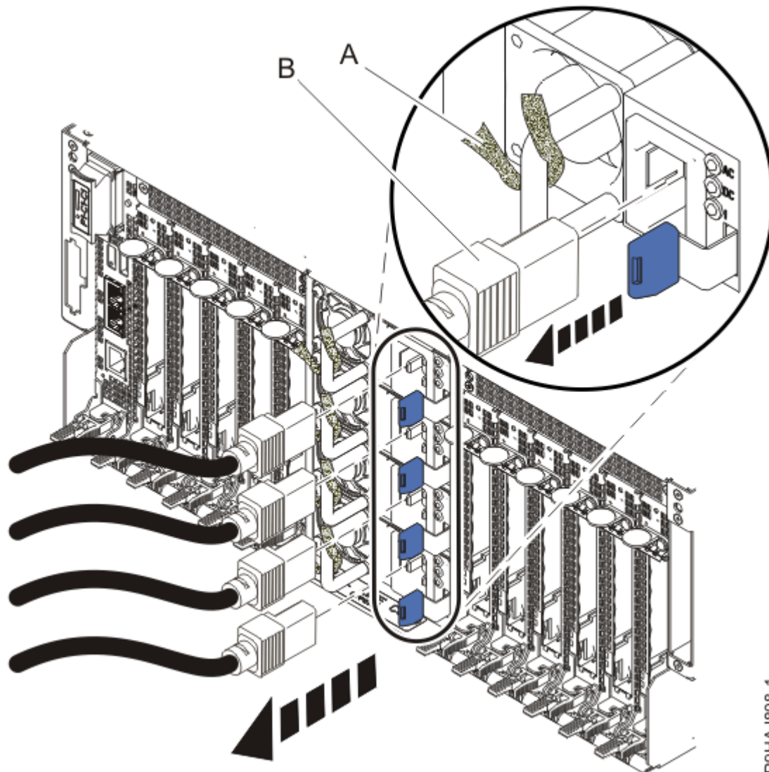
Abbildung 1. Netzkabel abziehen
