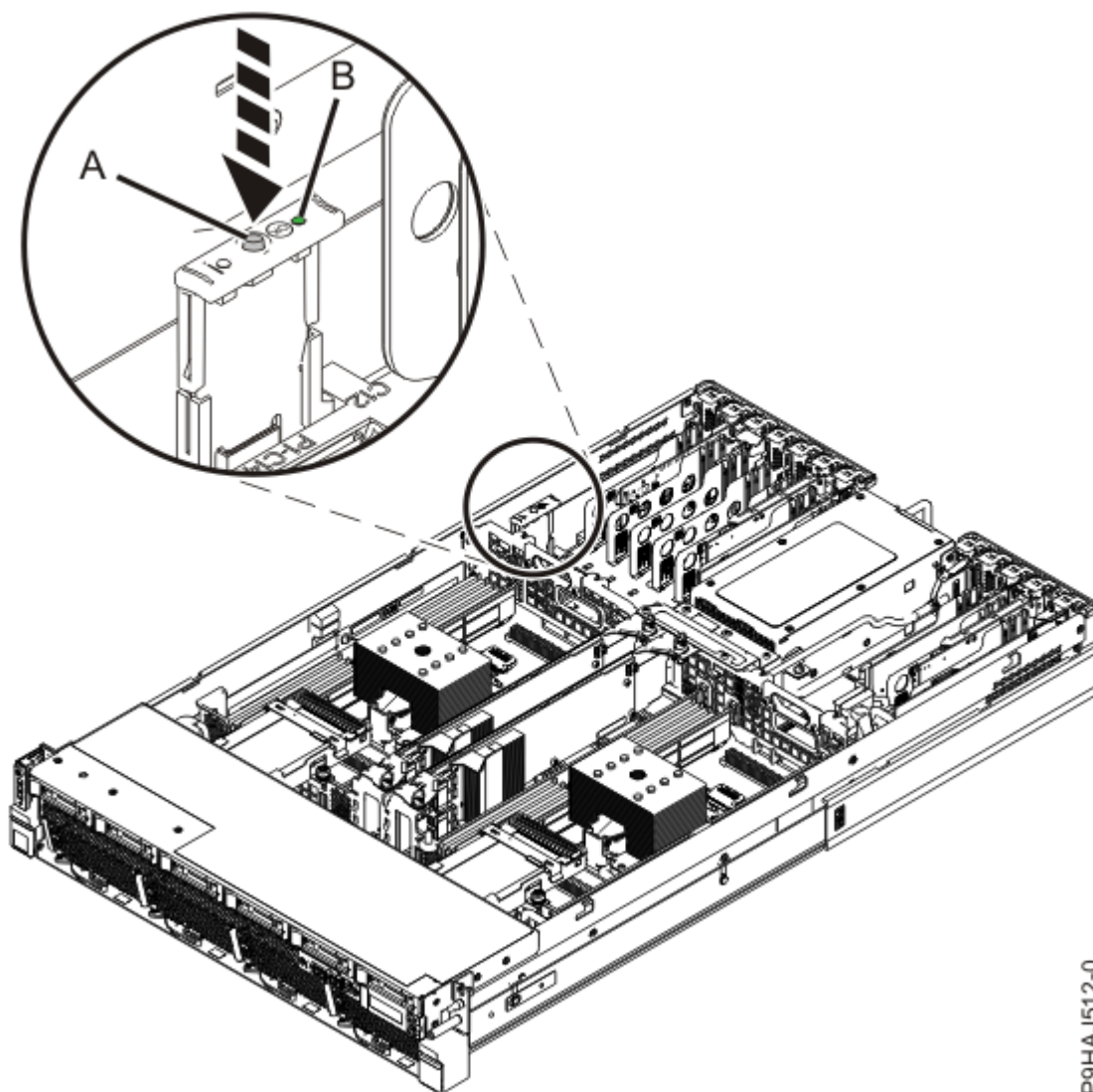
Abbildung 5. Kennzeichnungs-LED aktivieren
