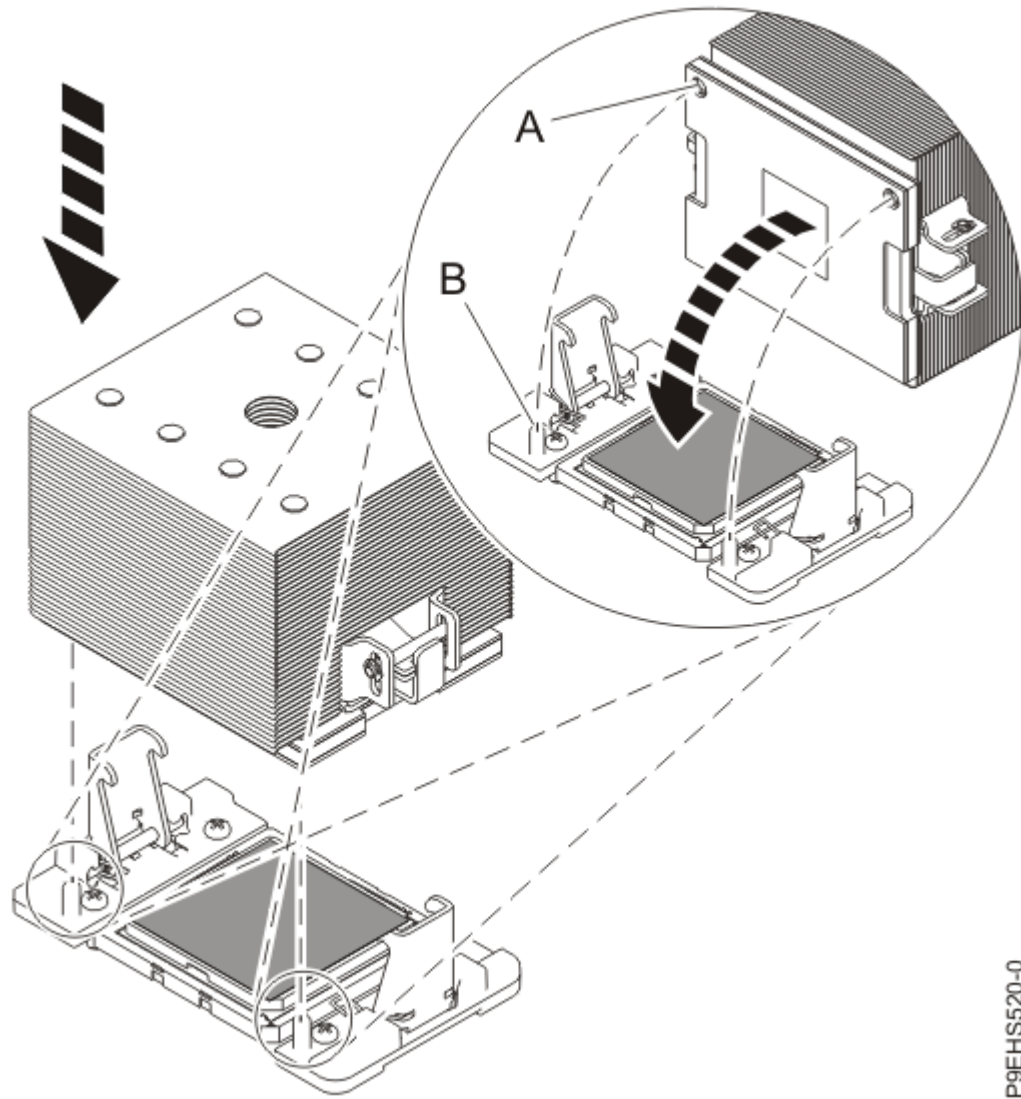
Abbildung 22. Kühlblech auf dem TIM installieren
