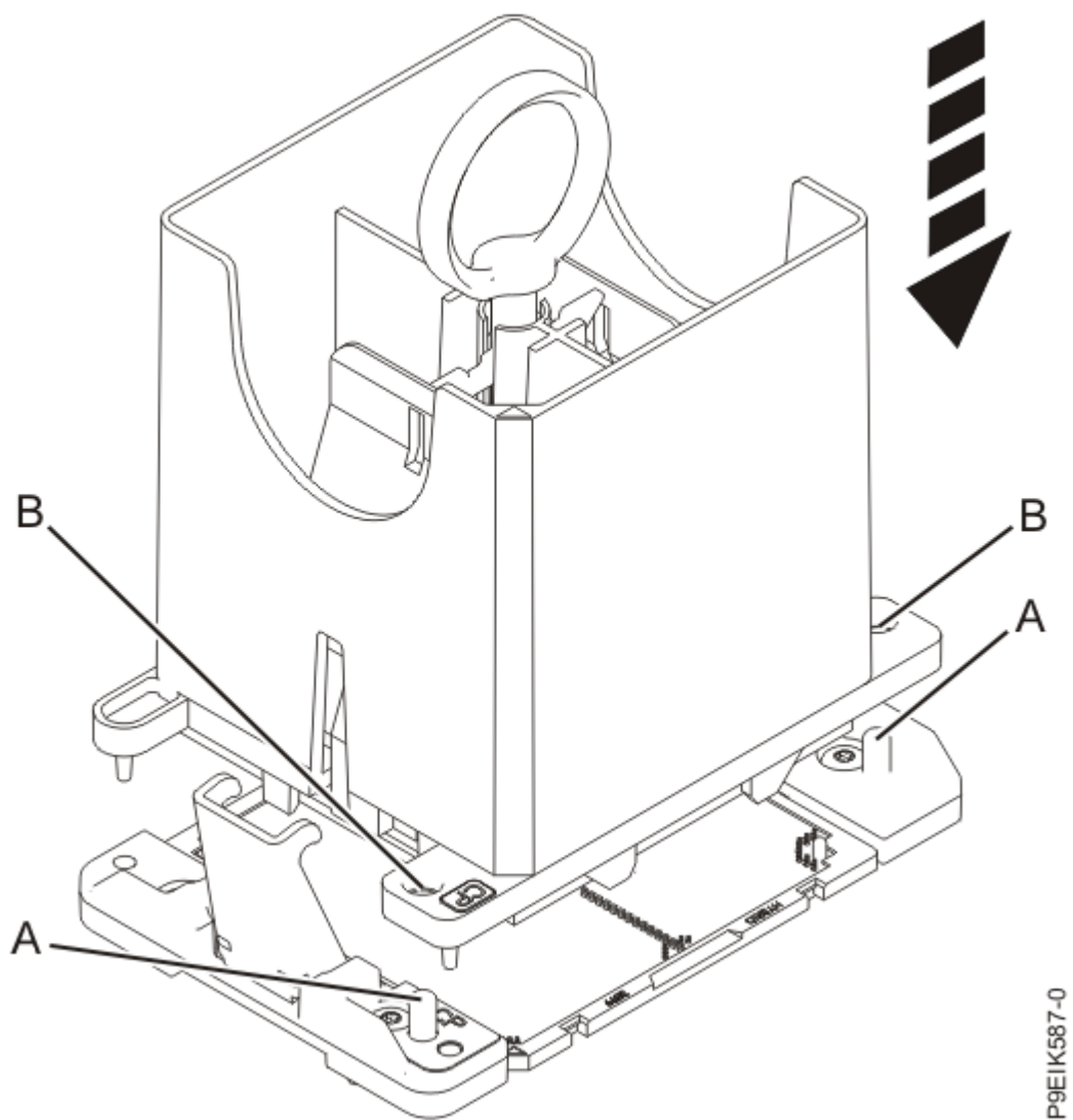
Abbildung 18. Systemprozessormodul installieren
