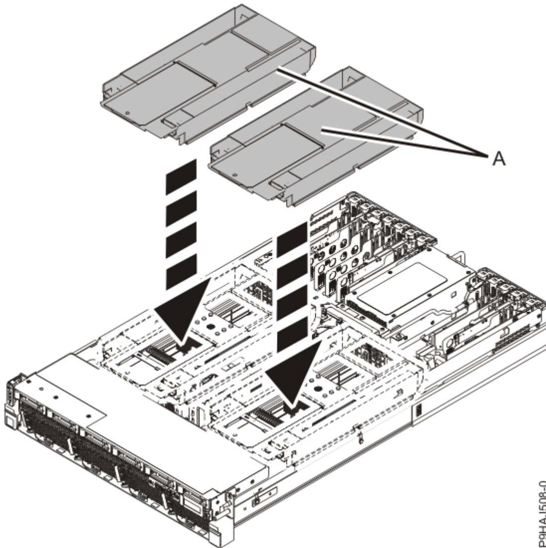
Abbildung 27. Luftführung wiedereinbauen
