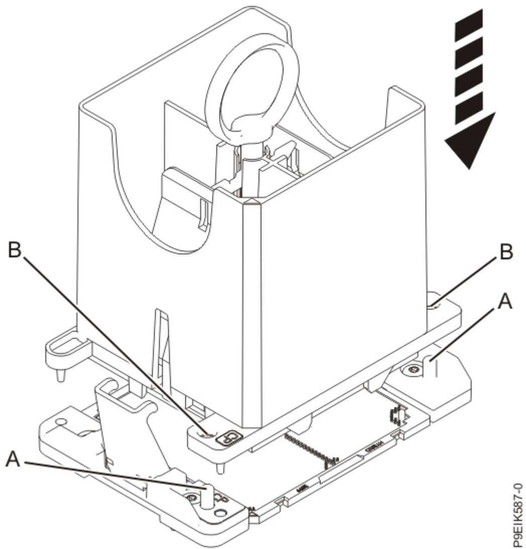
Abbildung 24. Systemprozessormodul installieren
