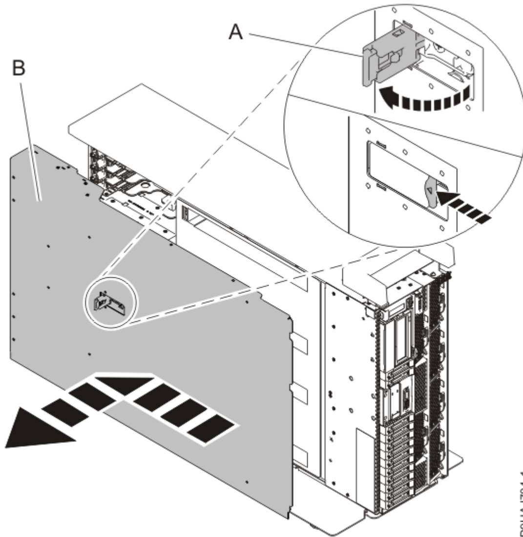
Abbildung 5. Serviceabdeckung ausbauen
