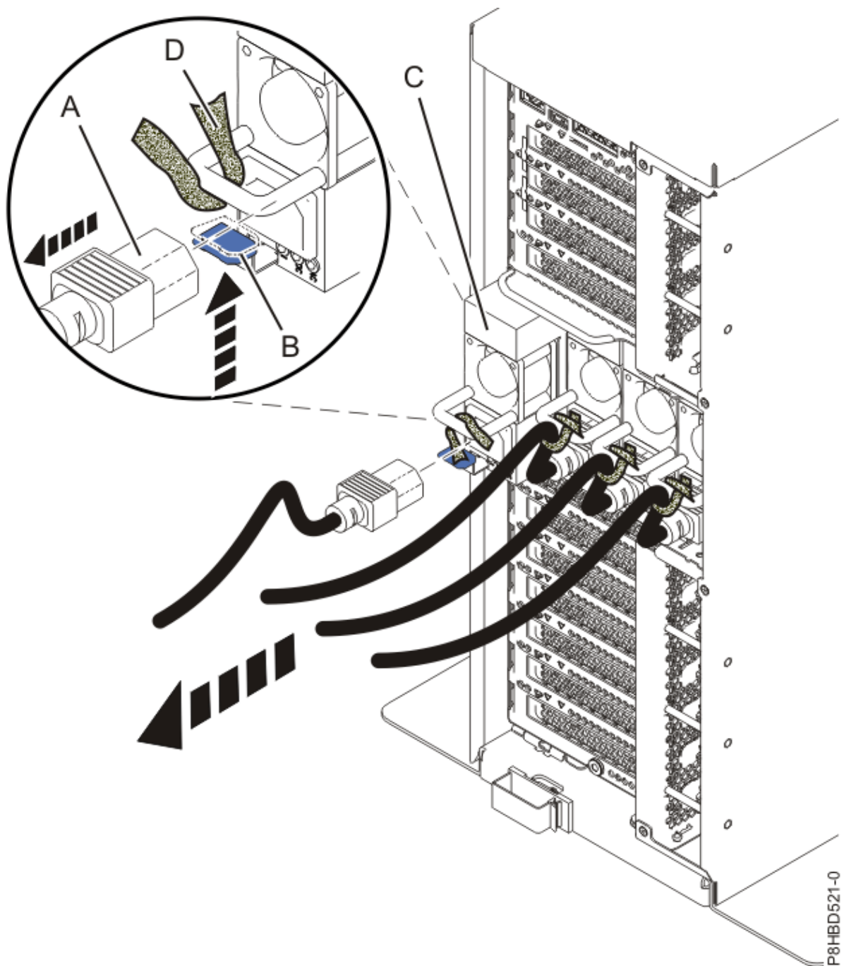
Abbildung 6. Netzteile entfernen
