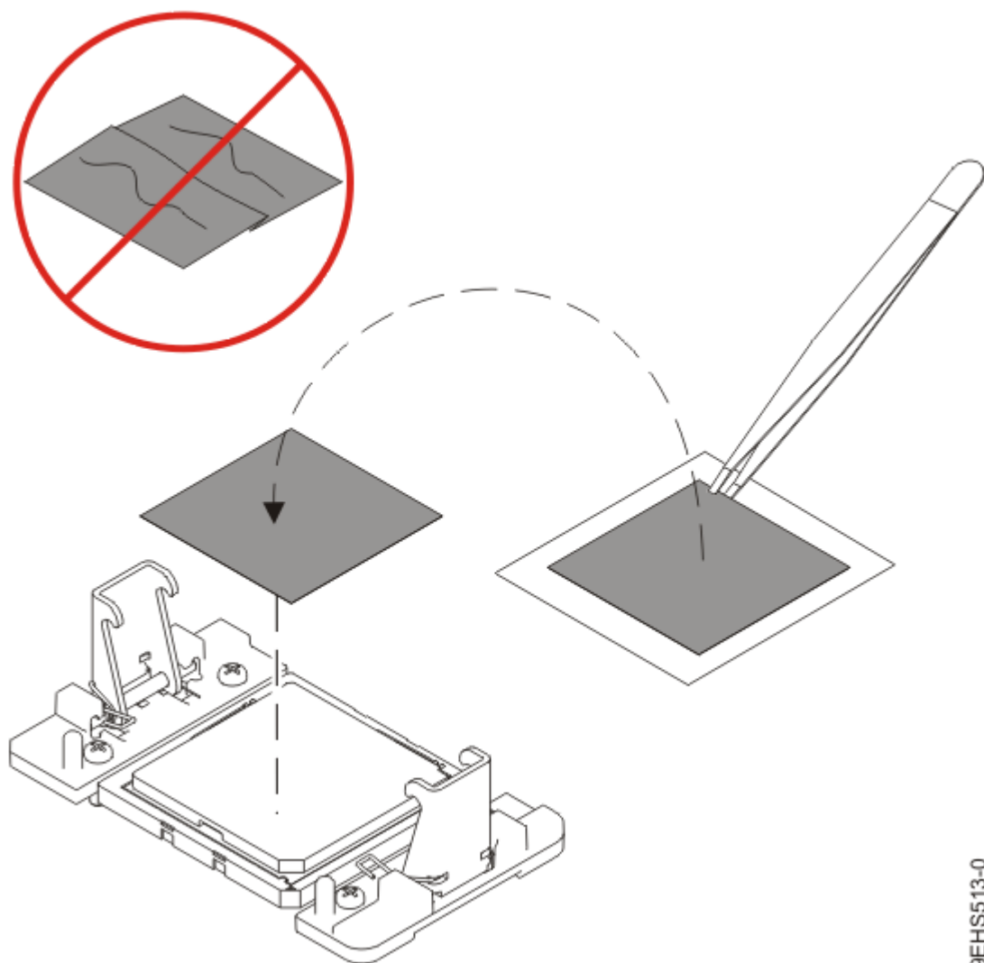
Abbildung 29. TIM auf dem Systemprozessormodul platzieren
