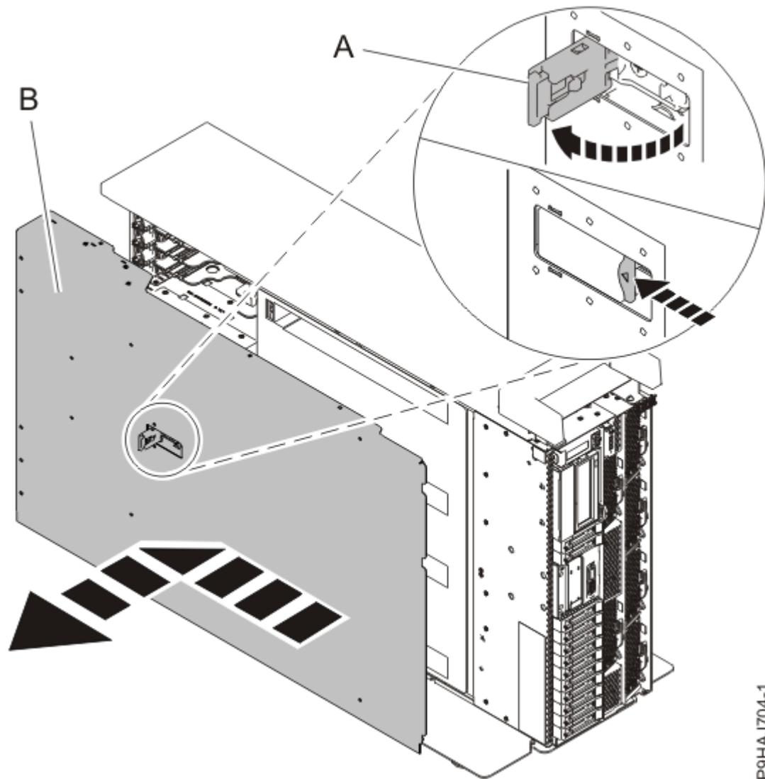
Abbildung 7. Serviceabdeckung ausbauen
