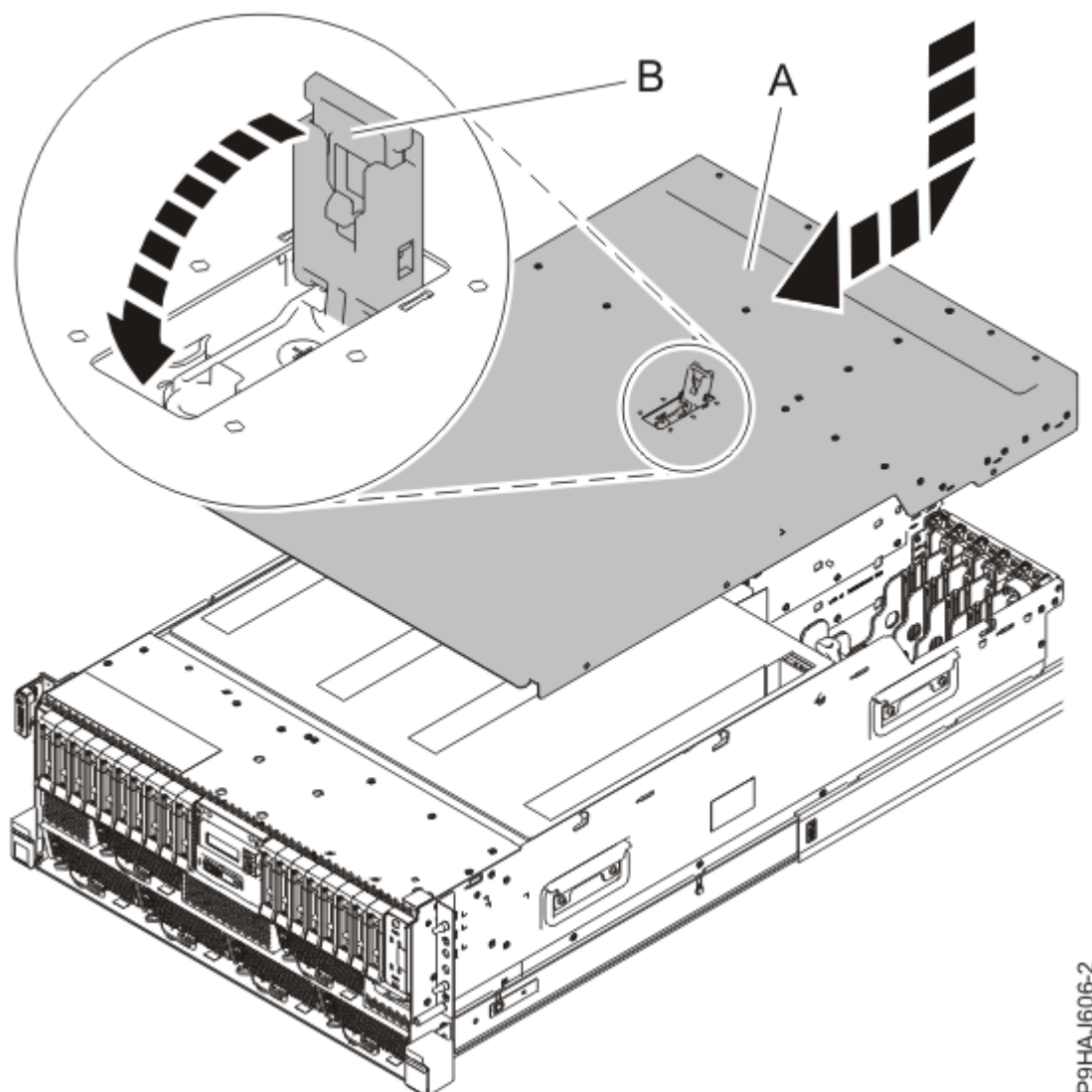
Abbildung 37. Serviceabdeckung installieren
