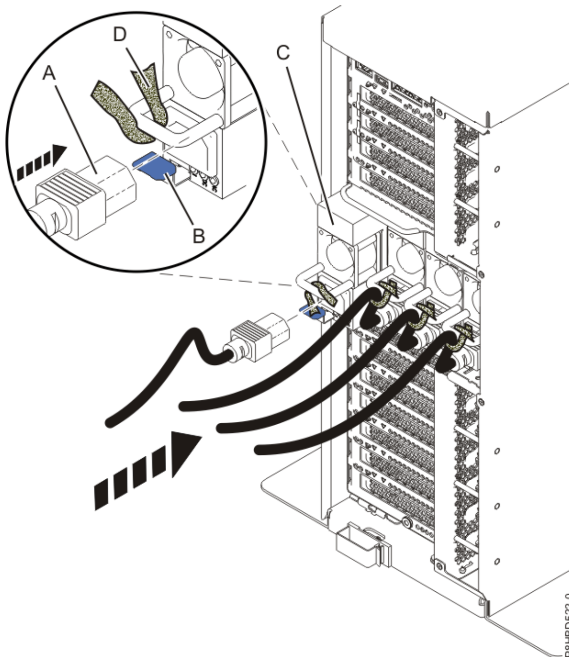
Abbildung 36. Netzteil austauschen
