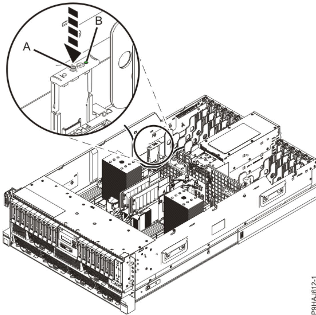
Abbildung 10. Aktivieren der Kennzeichnungs-LED für ein Einschubsystem
