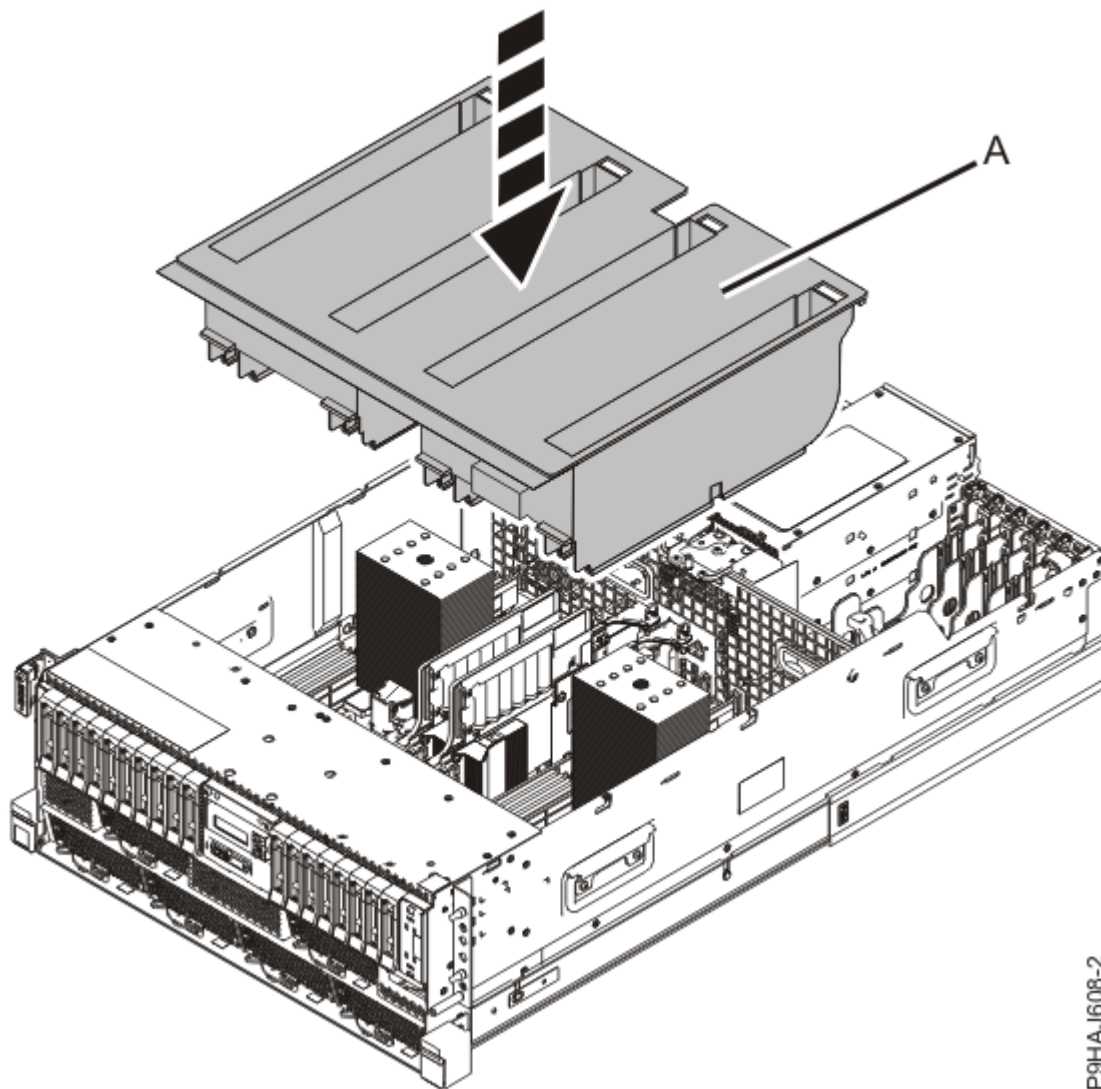
Abbildung 33. Luftführung bei einem Einschubsystem oder Standalone-System wiedereinbauen
