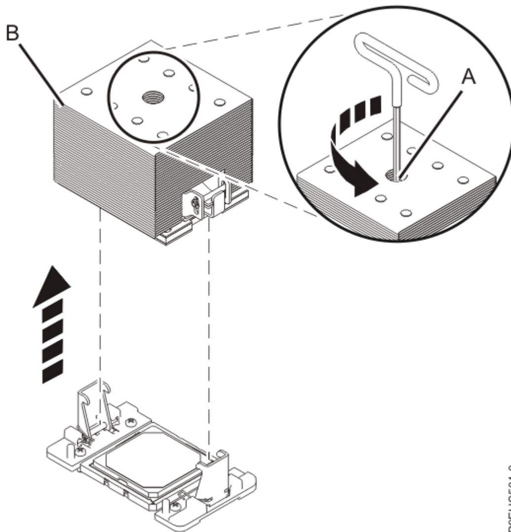
Abbildung 13. Kühlblech ausbauen
