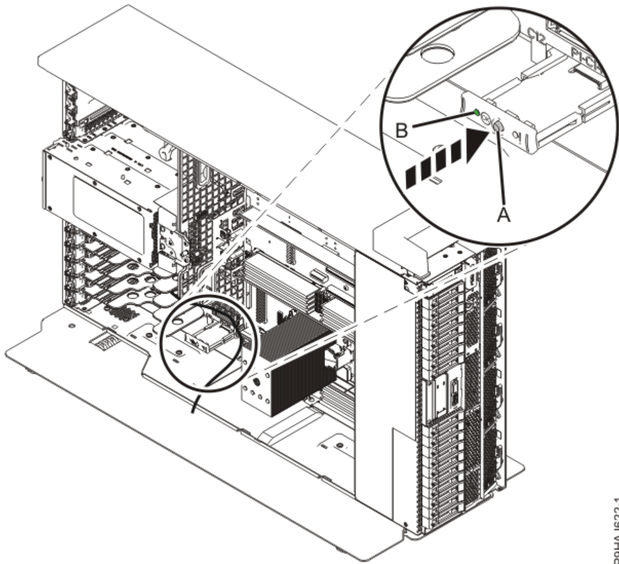
Abbildung 11. Aktivieren der Kennzeichnungs-LED für ein Standalone-System
