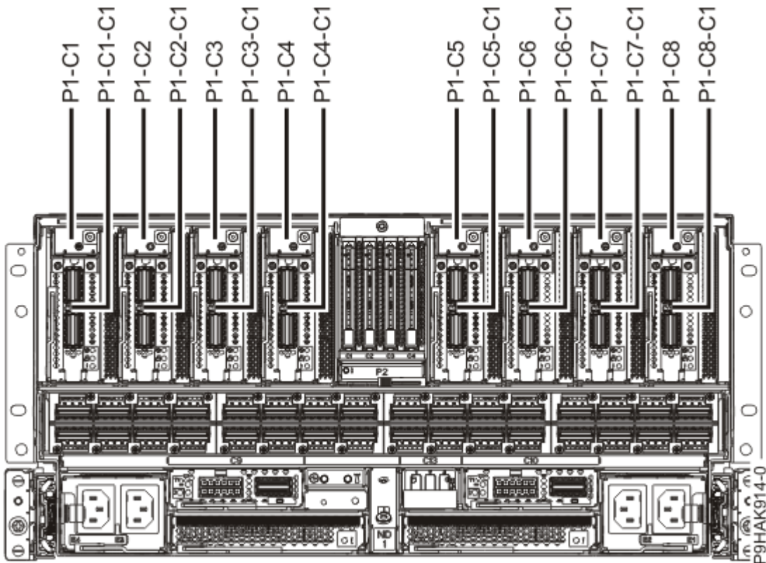
Abbildung 1. Rückansicht des Einschubsystems 9080-M9S mit Positionscodes der PCIe-Steckplätze
