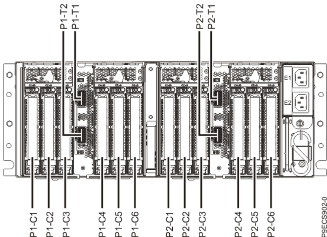
Abbildung 2. Rückansicht eines Einschubs für EMX0-PCIe3-Erweiterungen mit Positionscode der PCIe-Steckplätze
