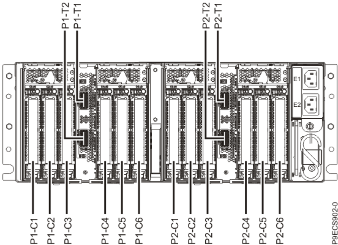
Abbildung 3. Rückansicht eines Einschubs für EMX0-PCIe3-Erweiterungen mit Positionscodes der PCIe-Steckplätze
