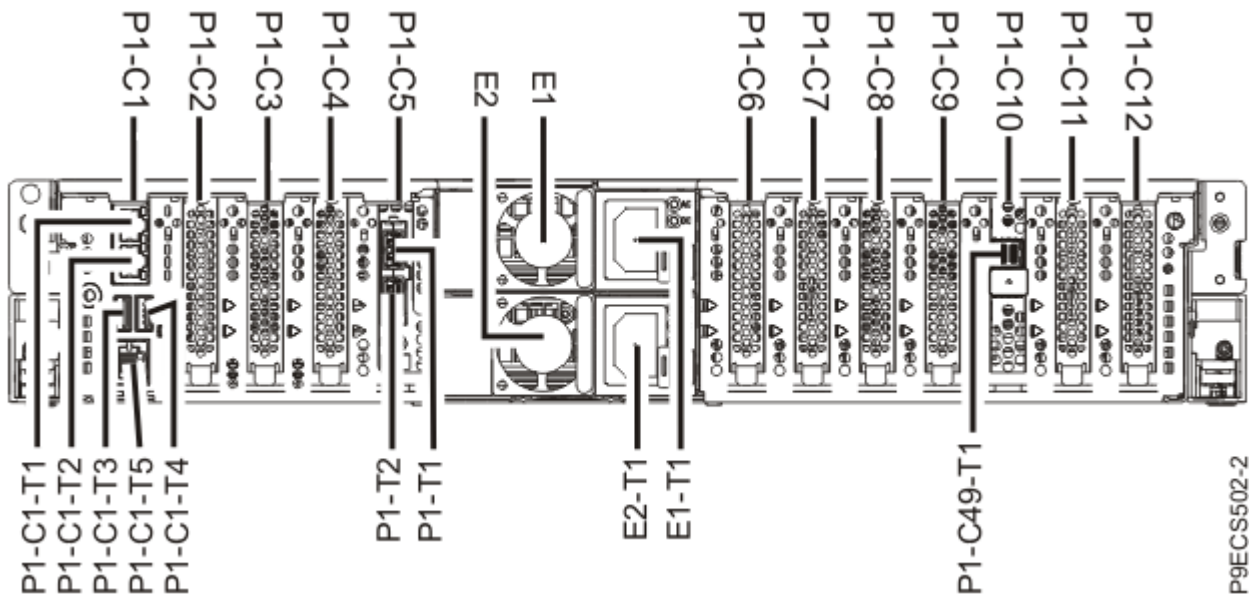
Abbildung 1. Rückansicht eines Einschubsystems vom Typ 5105-22E, 9009-22G oder 9223-22S mit Positionscodes der Steckplätze
