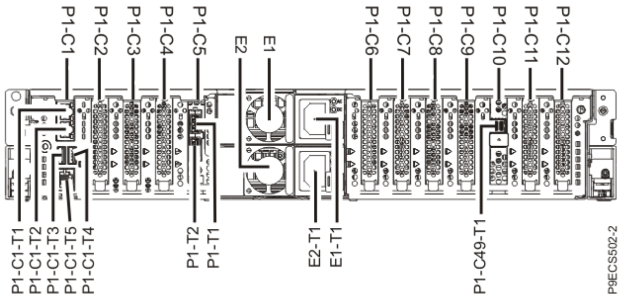
Abbildung 2. Rückansicht eines Einschubsystems vom Typ 9008-22L, 9009-22A oder 9223-22H mit Positionscodes der PCIe-Steckplätze
