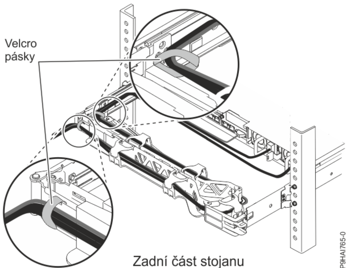
Obrázek 23. Upínací smyčka
