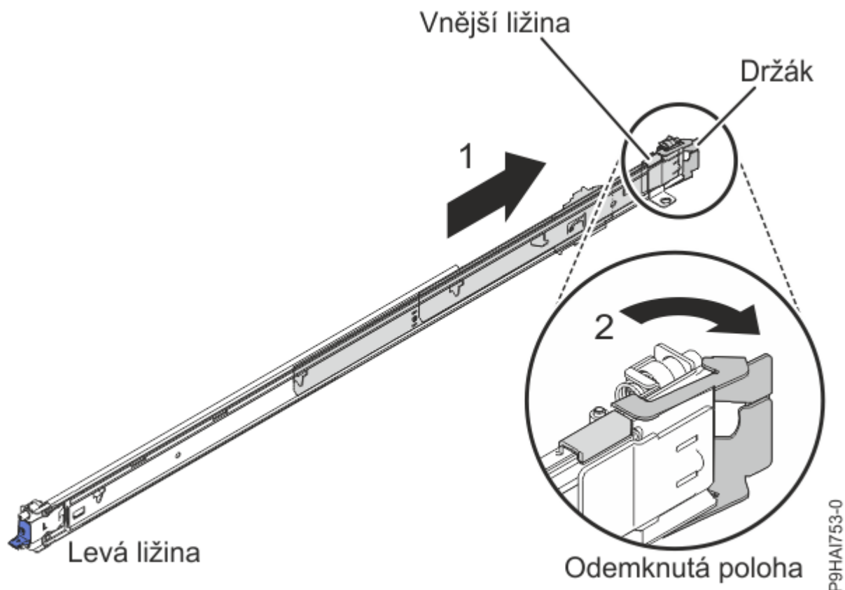
Obrázek 12. Výsuvná kolejnice a člen vnějšího výsuvu
