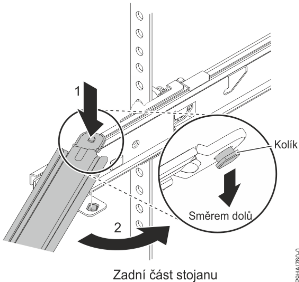
Obrázek 18. Připojení podpůrného ramene
