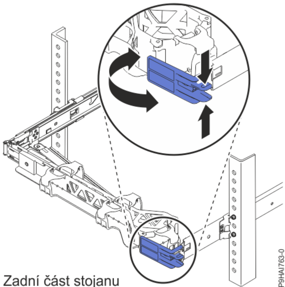
Obrázek 21. Držák zarážky podpory vedení kabelů
