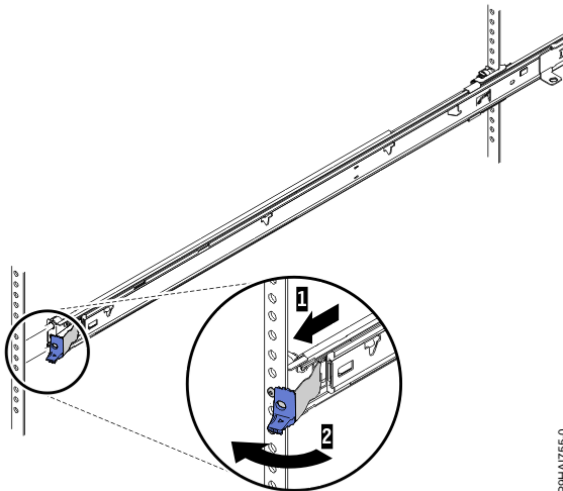
Obrázek 14. Přední západka výsuvné kolejnice
