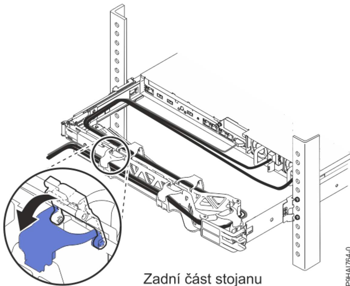
Obrázek 22. Připojení napájecího kabelu produktu Power a vedení kabelu
