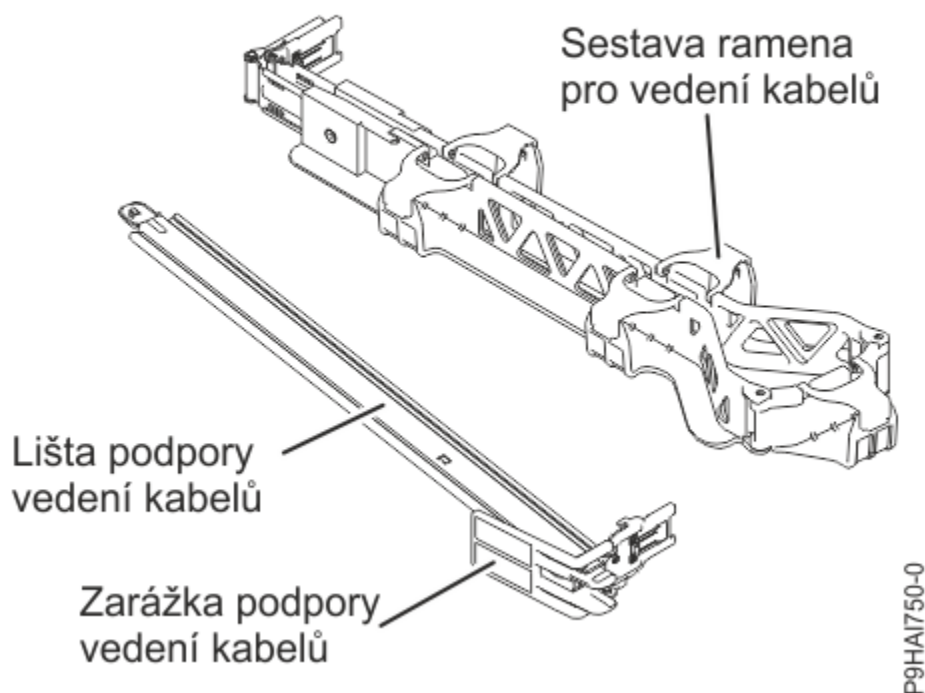
Obrázek 9. Obsah balení ramena pro vedení kabelů
