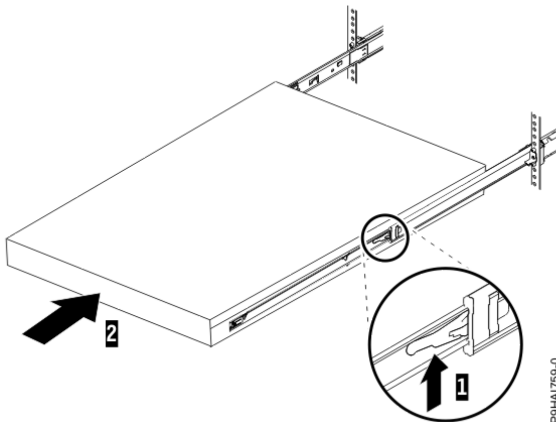
Obrázek 17. Uvolňovací západky a server
