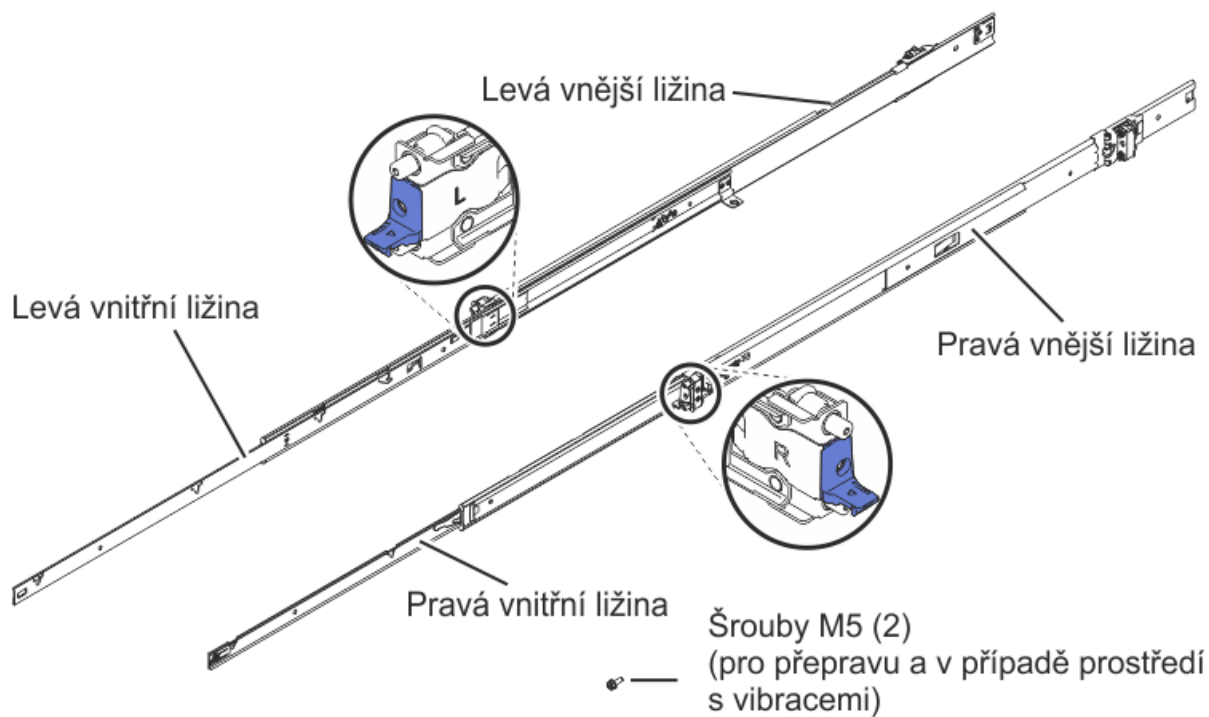
Obrázek 10. Obsah balení kolejnic
