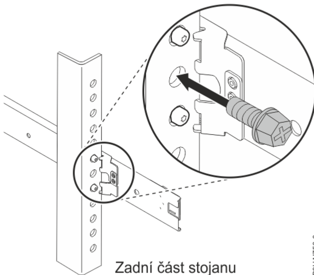
Obrázek 24. Zabezpečení serveru pro přepravu
