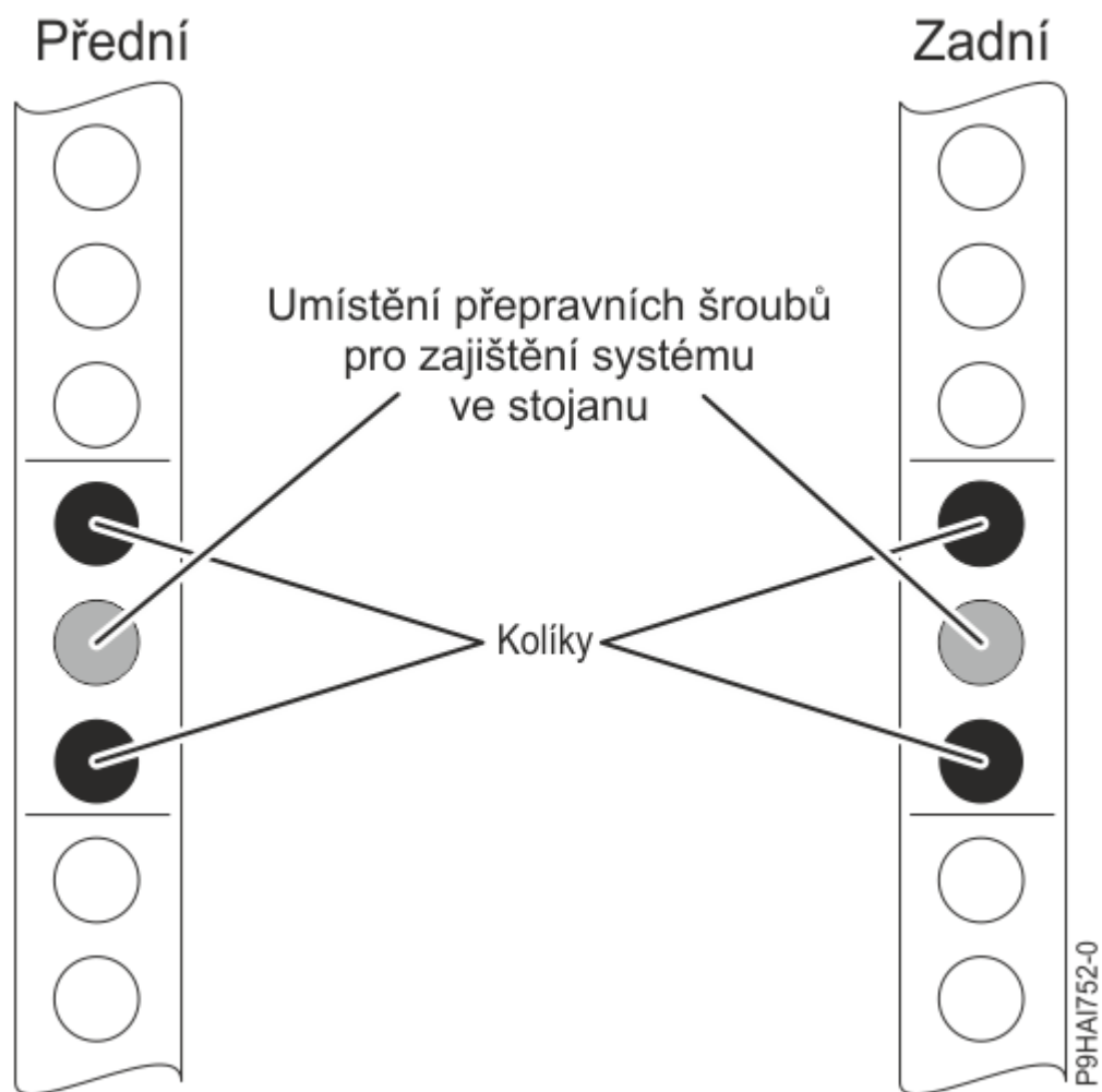
Obrázek 11. Identifikace místa ve stojanu
