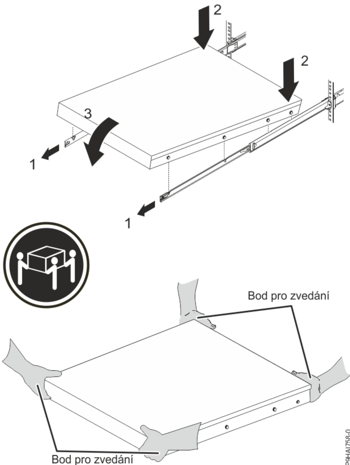
Obrázek 16. Vysunuté kolejnice, hlavice na serveru zarovnané s otvory v kolejích a body zvedání
