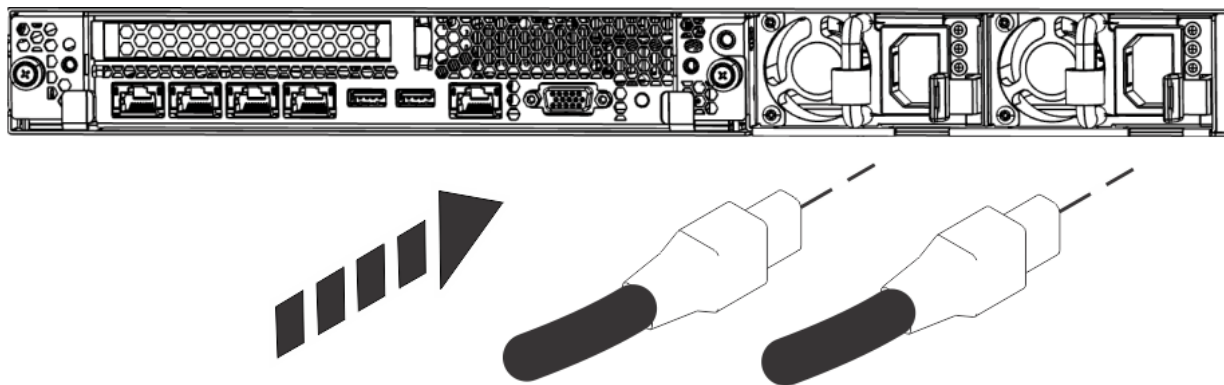
Obrázek 2. Zapojení napájecích kabelů do napájecích zdrojů
