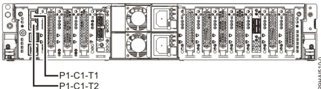
Obrázek 26. Umístění portů konzoly HMC 5105-22E, 9008-22L, 9009-22A, 9009-22G, 9223-22H a 9223-22S
