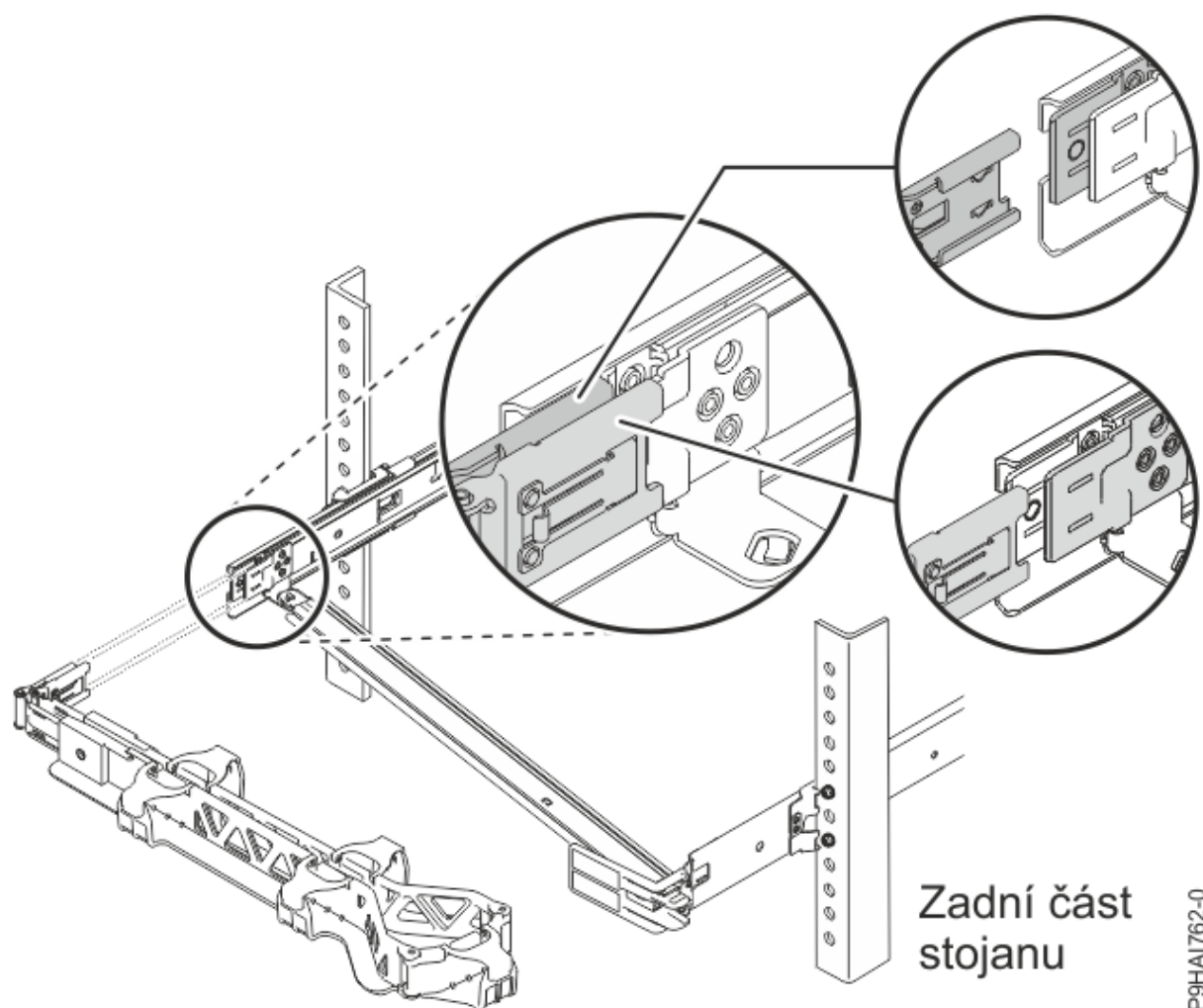
Obrázek 20. Připojení ramena pro vedení kabelů
