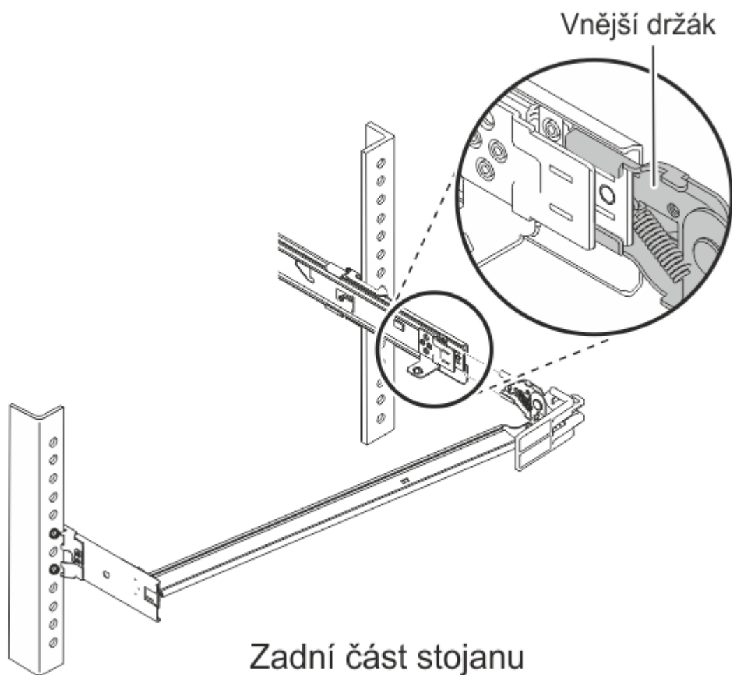
Obrázek 19. Připojení zarážky na výsuvnou kolejnici
