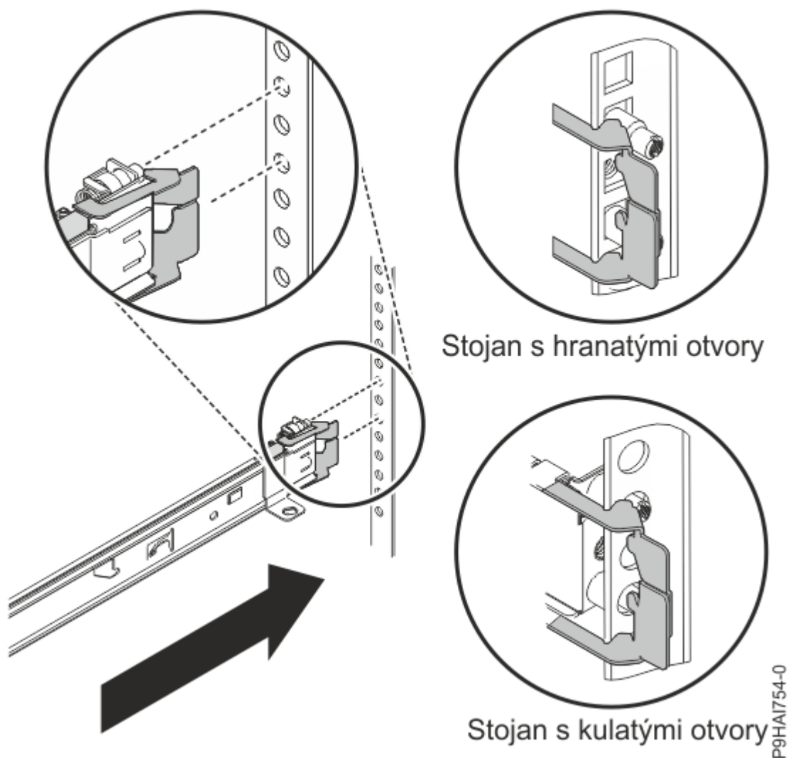
Obrázek 13. Vyrovnání kolíků s otvory v zadní části stojanu
