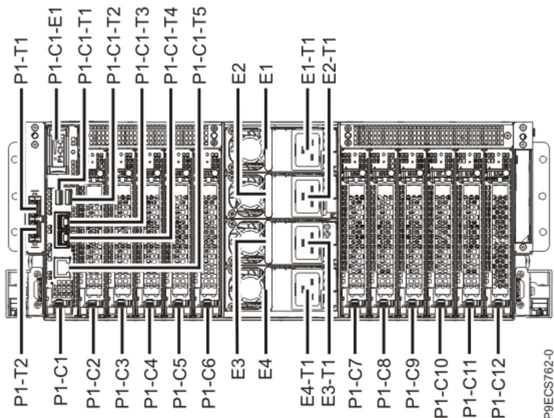
Obrázek 1. Pohled na zadní část systému 9040-MR9 montovaného do stojanu s kódy umístění slotů PCIe
