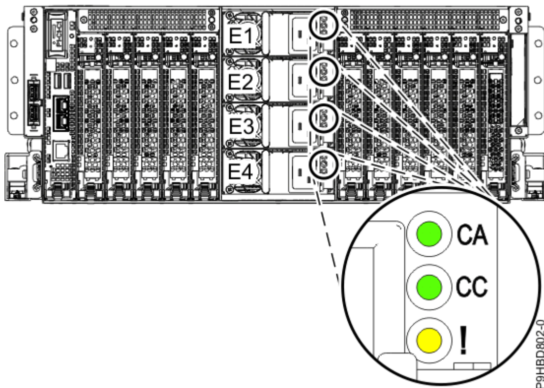
Figura 1. Ubicació de les fonts d'alimentació i dels LED
