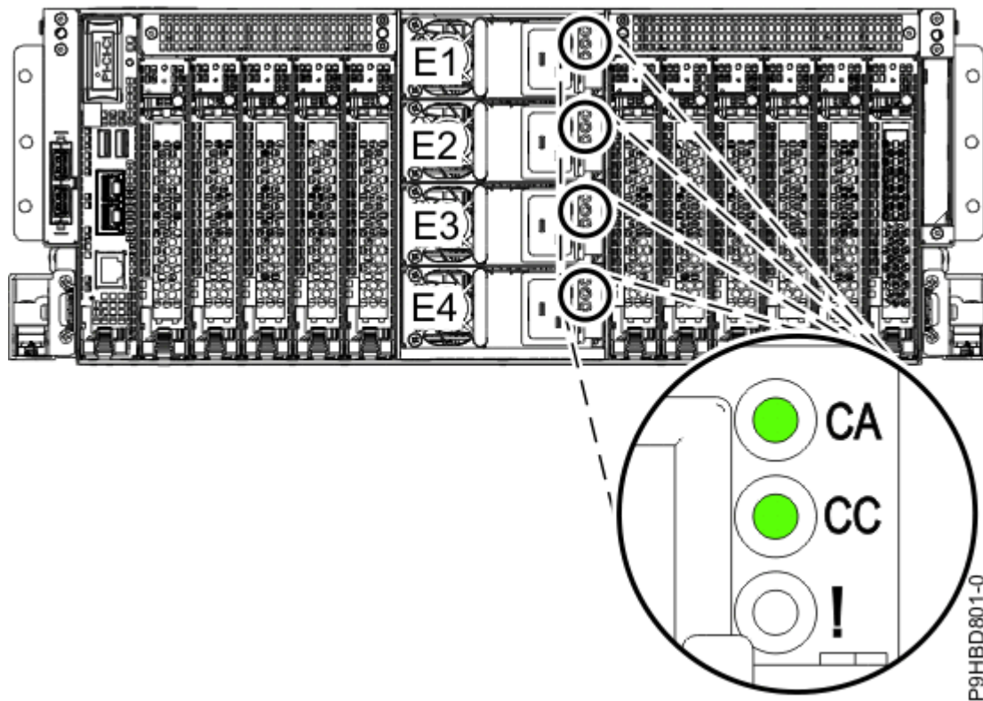
Figura 6. LED d'una font d'alimentació en funcionament
