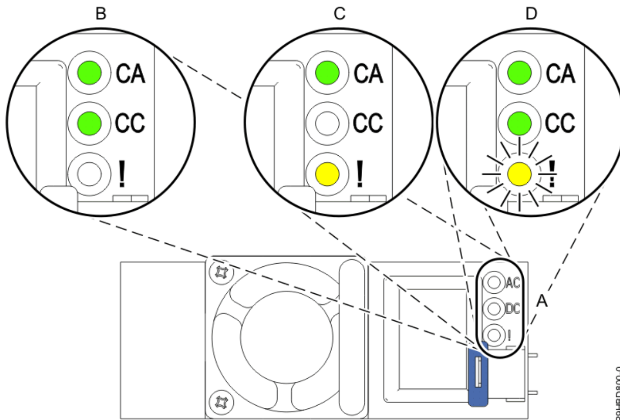
Figura 2. LED per a una font d'alimentació en funcionament (B) i amb error (C, D) en un sistema muntat en bastidor
