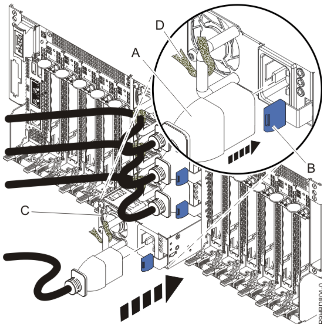
Figura 5. Substitució d'una font d'alimentació
