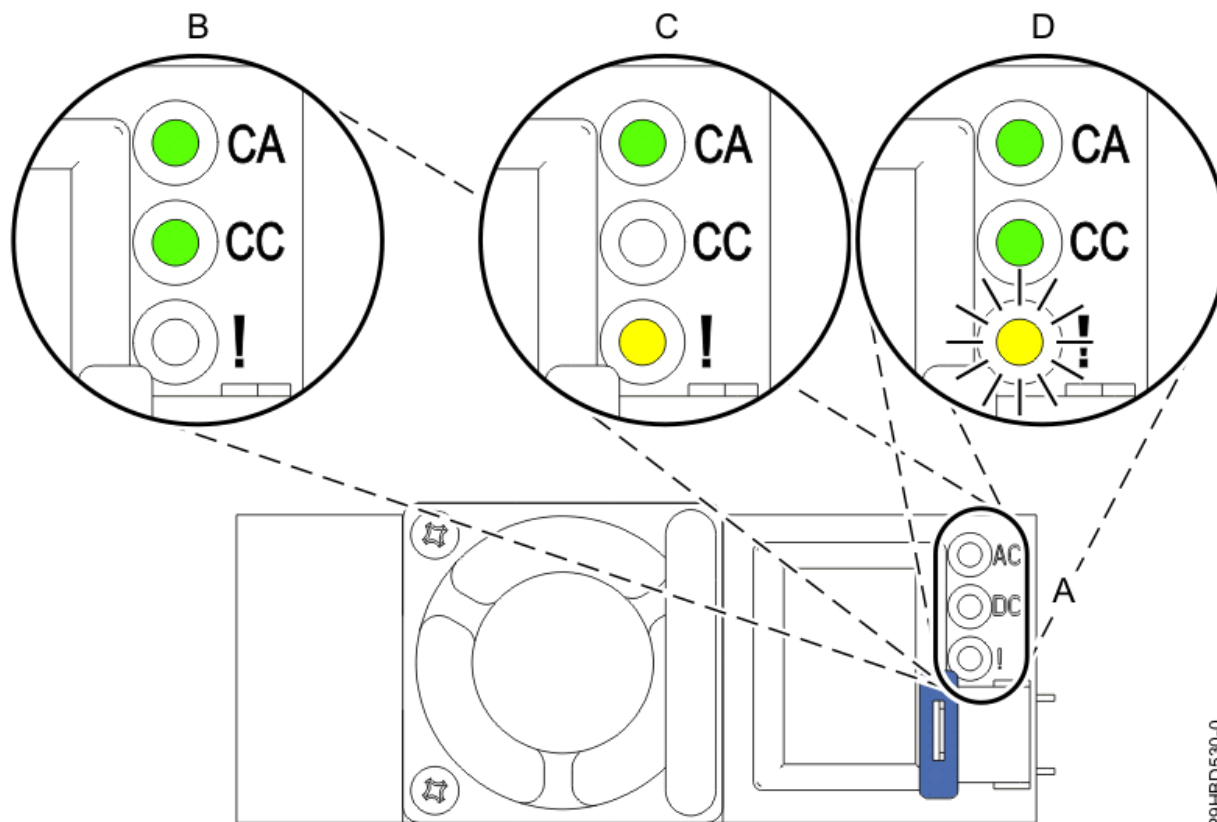
Figura 2. LED per a una font d'alimentació en funcionament (B) i amb error (C, D)
