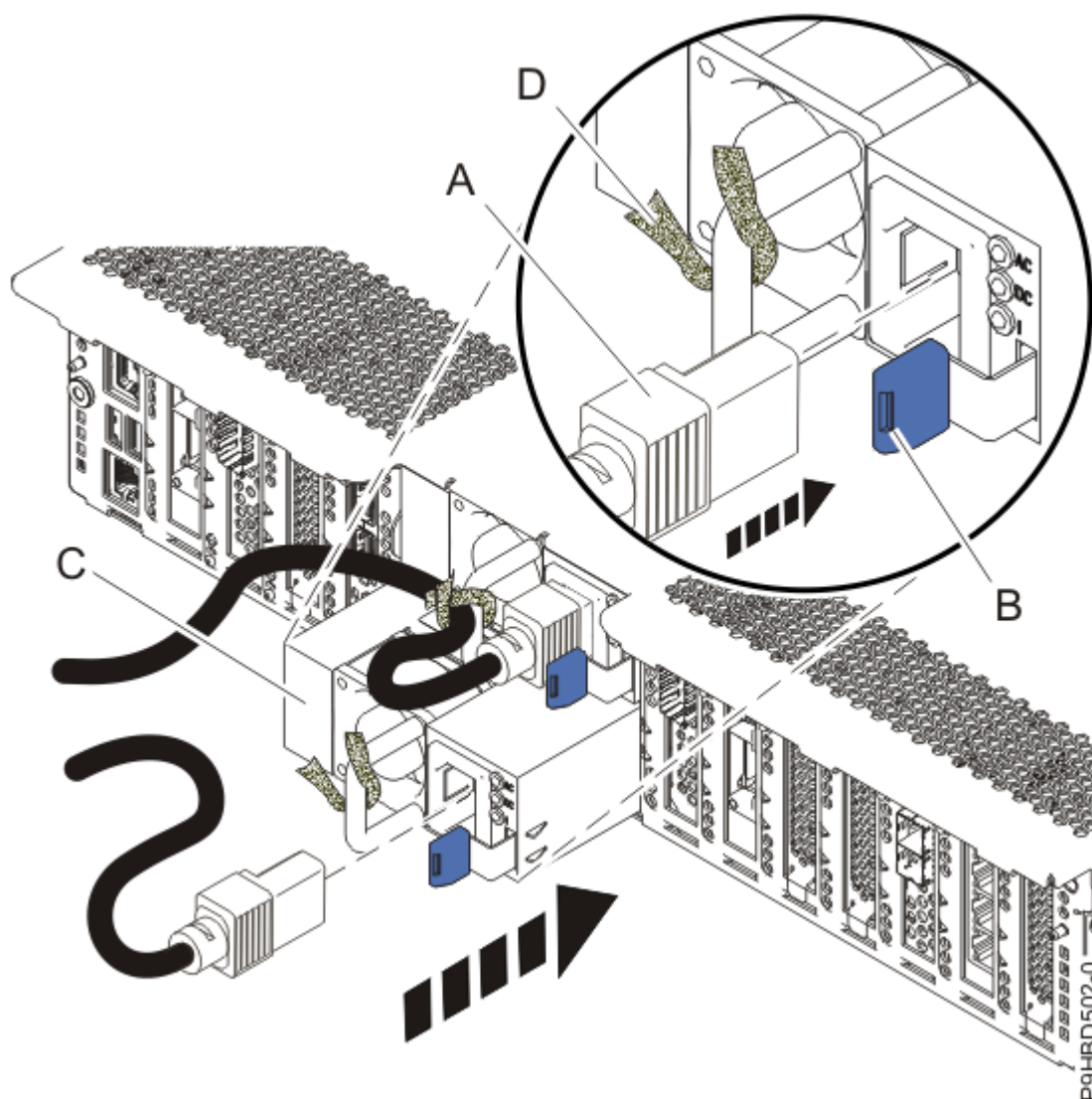
Figura 6. Substitució d'una font d'alimentació
