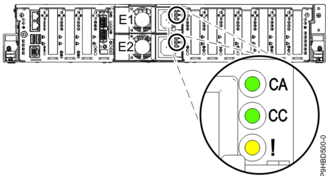
Figura 1. Ubicació de les fonts d'alimentació i dels LED del sistema
