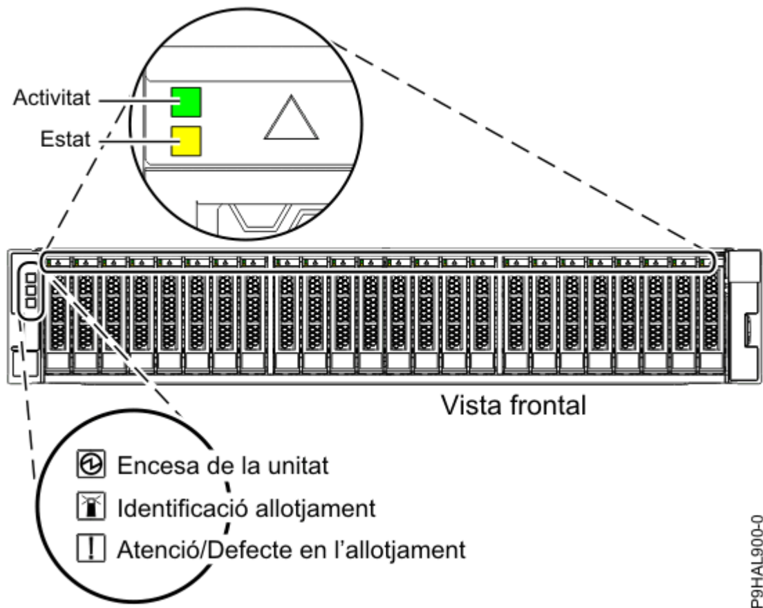
Figura 12. Vista frontal de l'allotjament d'emmagatzematge que mostra els indicadors de servei
