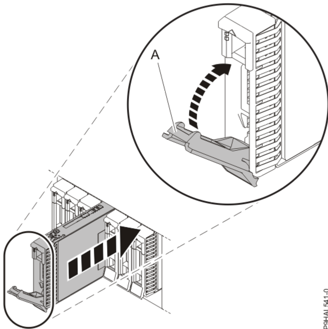
Figura 18. Substitució d'una unitat en un allotjament
