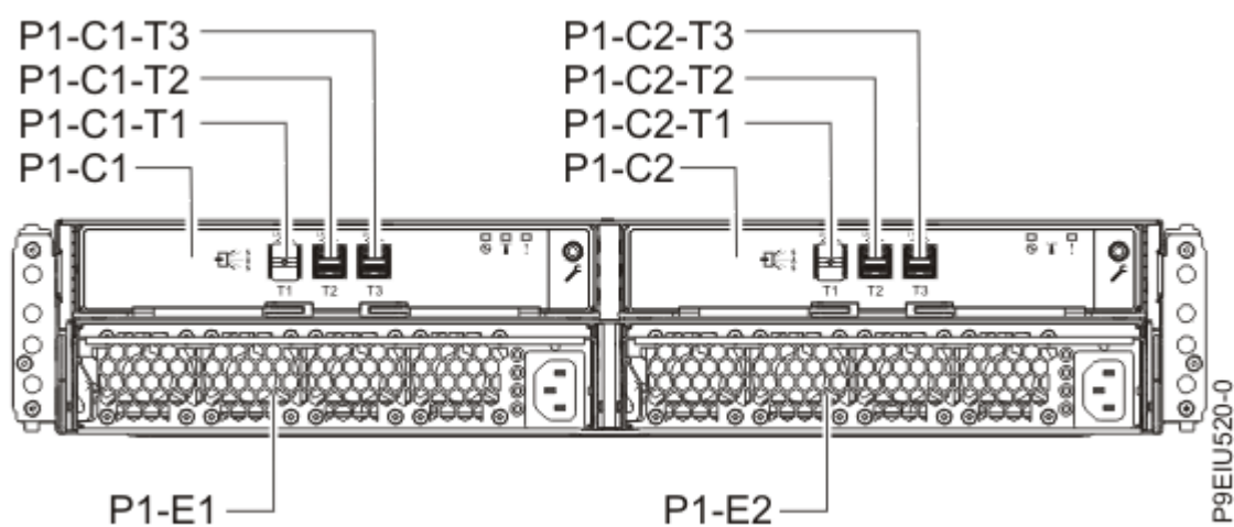
Figura 3. Vista posterior dels allotjaments d'emmagatzematge
