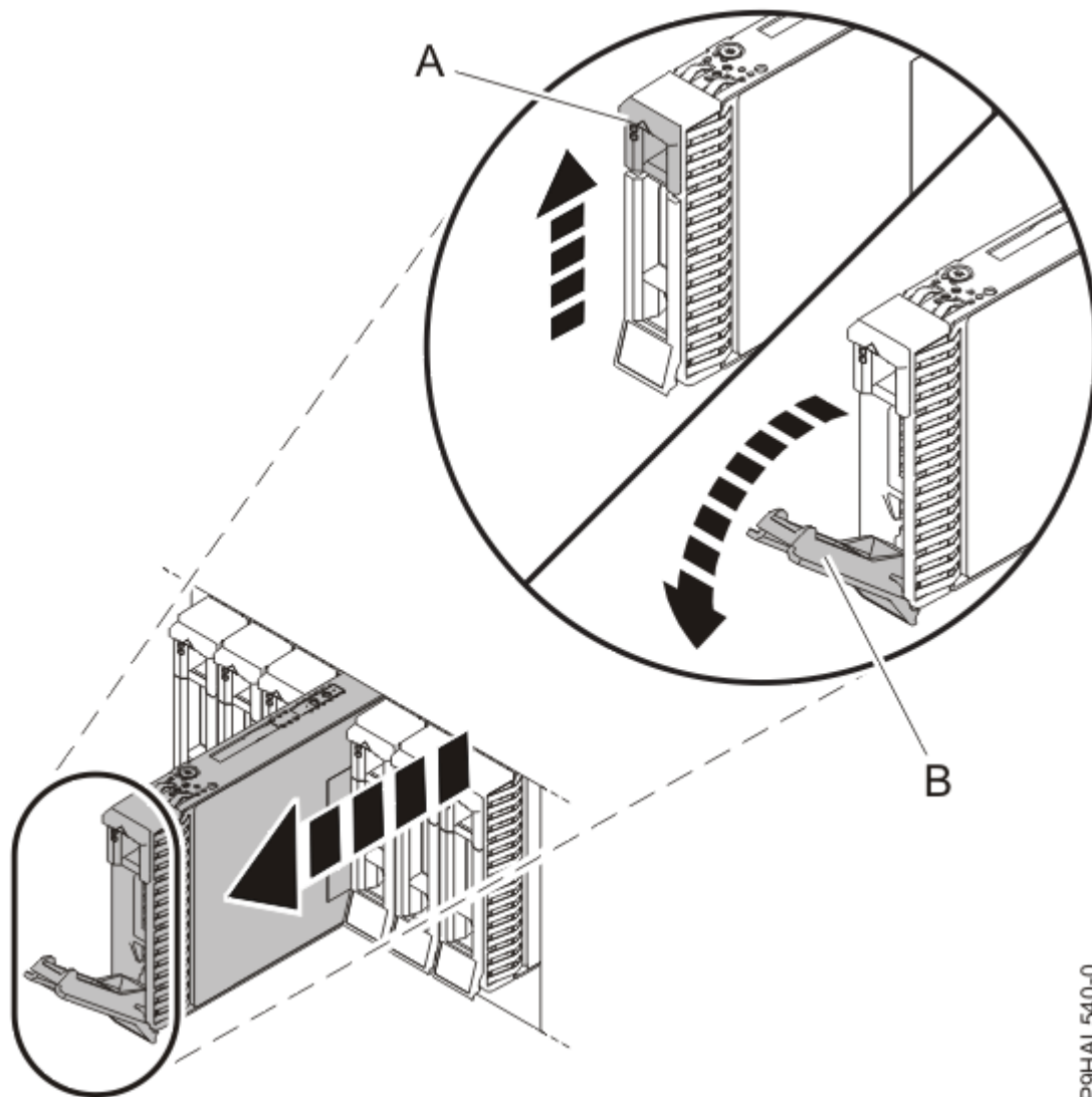
Figura 17. Desbloqueig i extracció de la unitat
