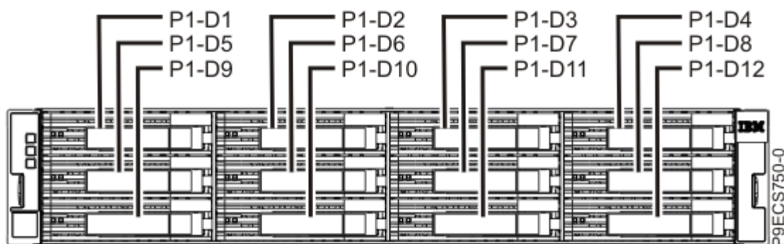
Figura 1. Vista frontal de l'allotjament d'emmagatzematge ESLL que mostra les ubicacions de les unitats
