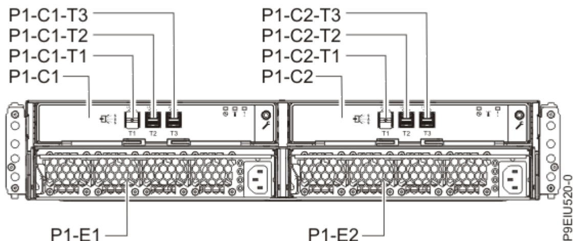
Figura 11. Vista posterior dels allotjaments d'emmagatzematge
