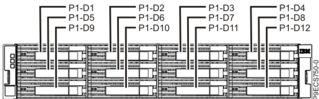
Figura 9. Vista frontal de l'allotjament d'emmagatzematge ESLL que mostra les ubicacions de les unitats
