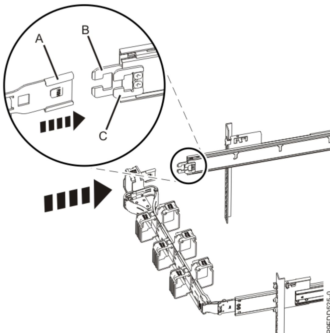
Figura 29. Tancament del braç portacables
