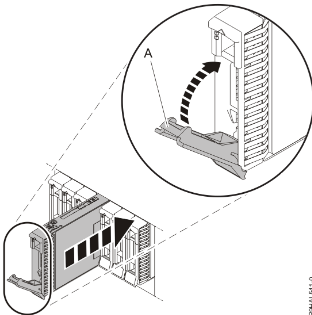
Figura 10. Instal·lació d'una unitat en un sistema
