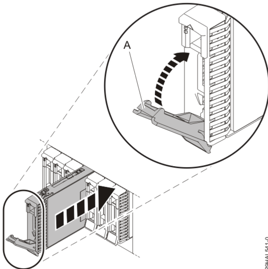
Figura 7. Instal·lació d'una unitat en un sistema
