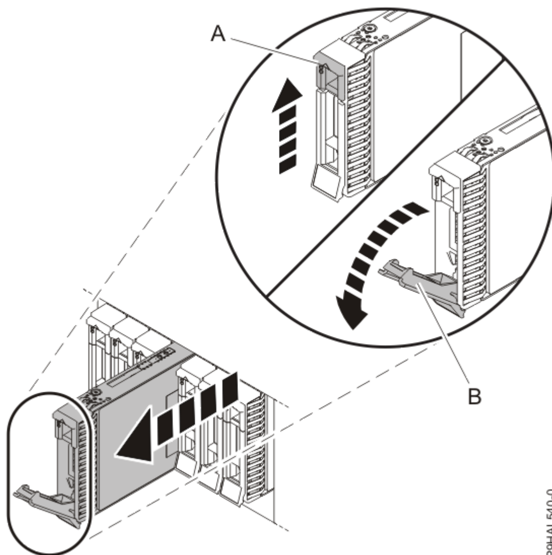
Figura 20. Desbloqueig i extracció de la unitat
