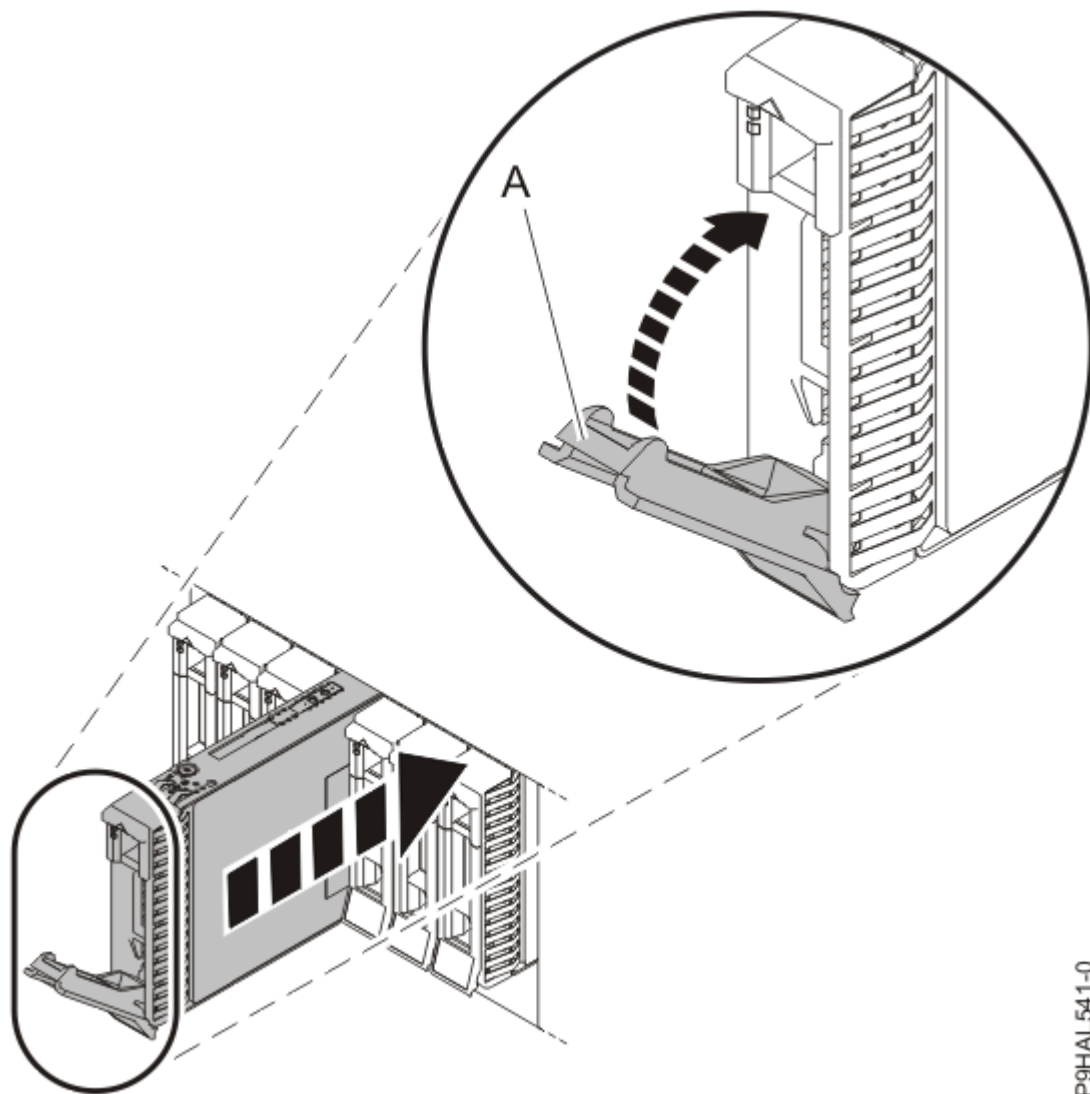
Figura 22. Instal·lació d'una unitat en un sistema
