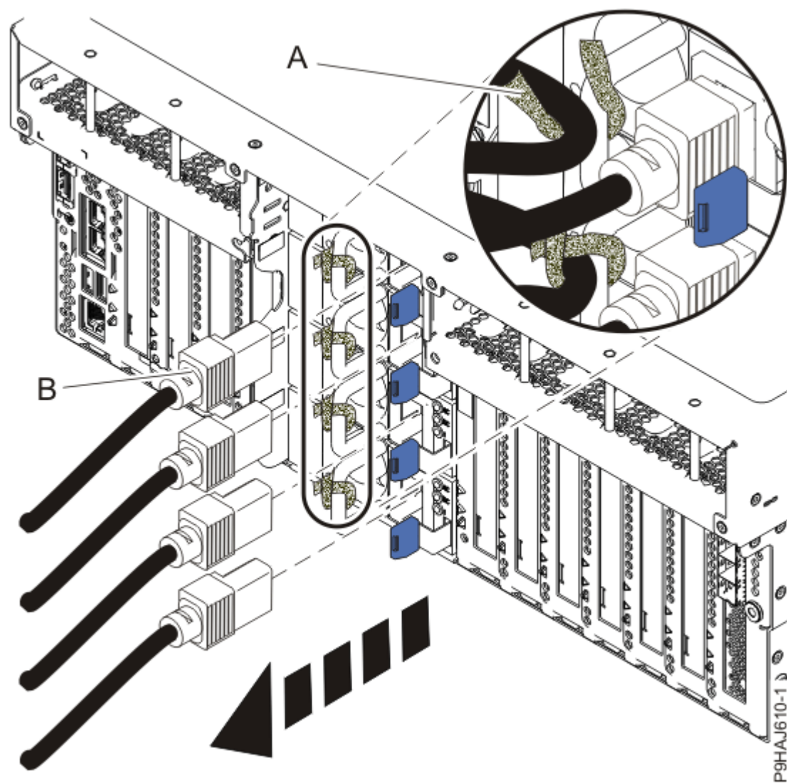
Figura 15. Extracció dels cables d'alimentació d'un servidor muntat en bastidor
