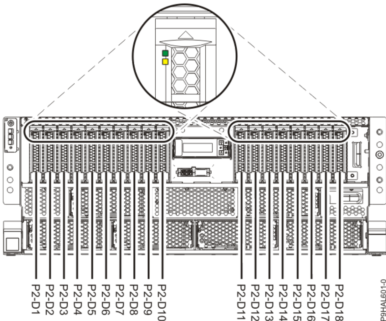
Figura 30. Ubicacions de les unitats de disc o unitats d'estat sòlid i dels indicadors de servei en un sistema 9009-41A, 9009-42A o 9223-42H muntat en bastidor
