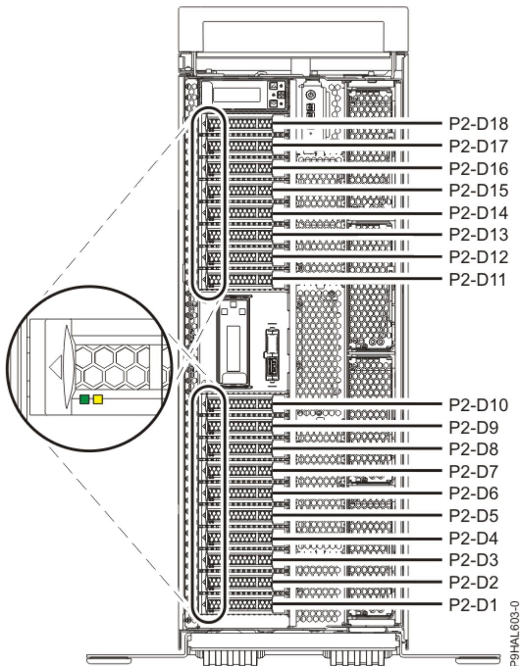
Figura 14. Ubicacions de les unitats de disc o unitats d'estat sòlid i dels indicadors de servei en un sistema 9009-41A, 9009-42A o 9223-42H autònom
