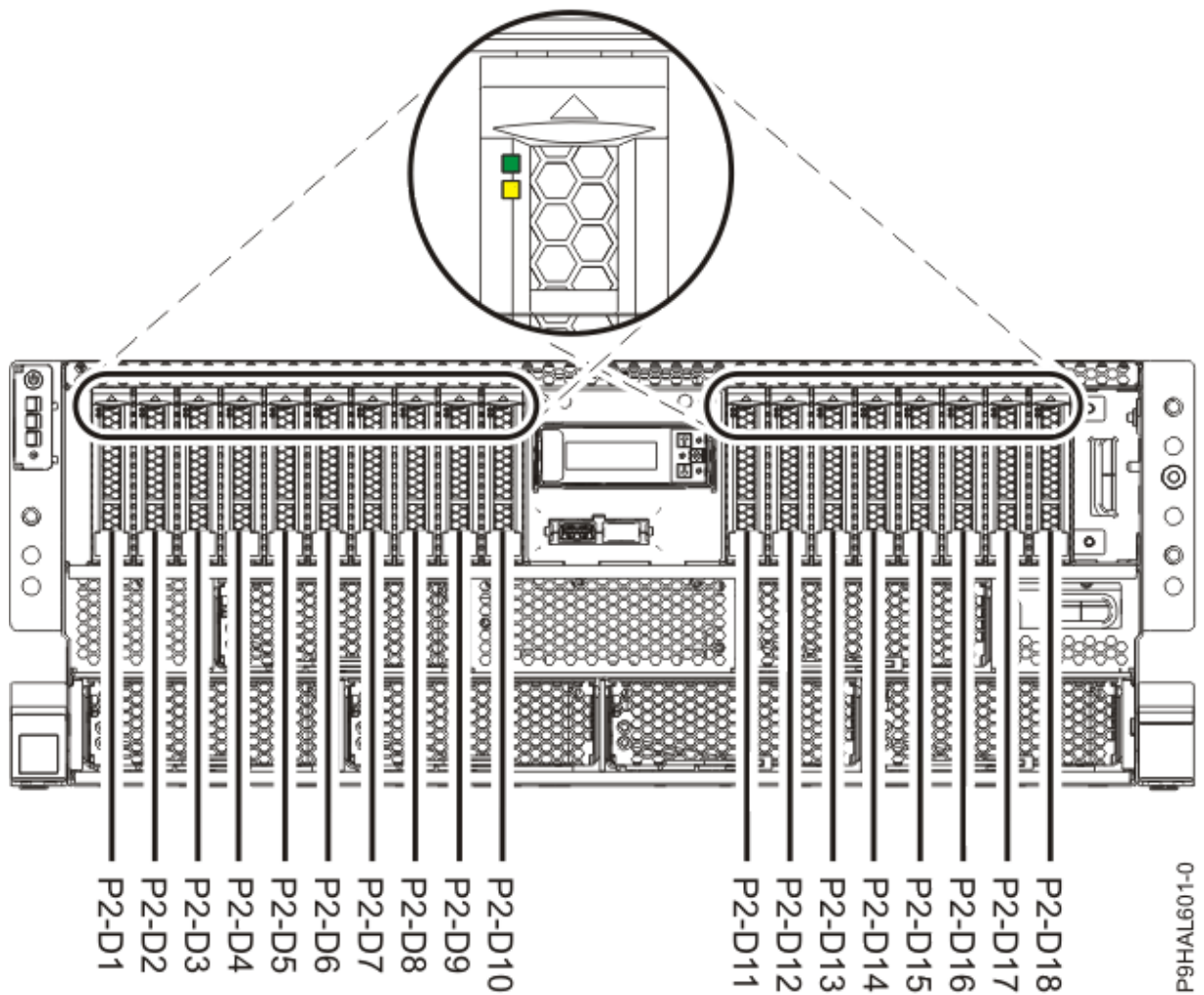
Figura 1. Ubicacions de les unitats de disc o unitats d'estat sòlid i dels indicadors de servei en un sistema 9009-41A, 9009-42A o 9223-42H muntat en bastidor
