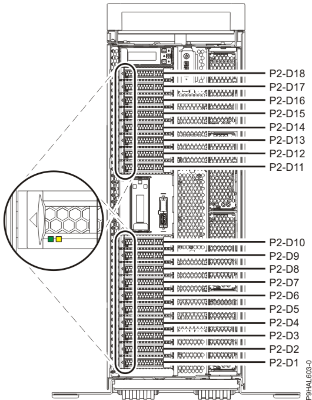
Figura 2. Ubicacions de les unitats de disc o unitats d'estat sòlid i dels indicadors de servei en un sistema 9009-41A, 9009-42A o 9223-42H autònom
