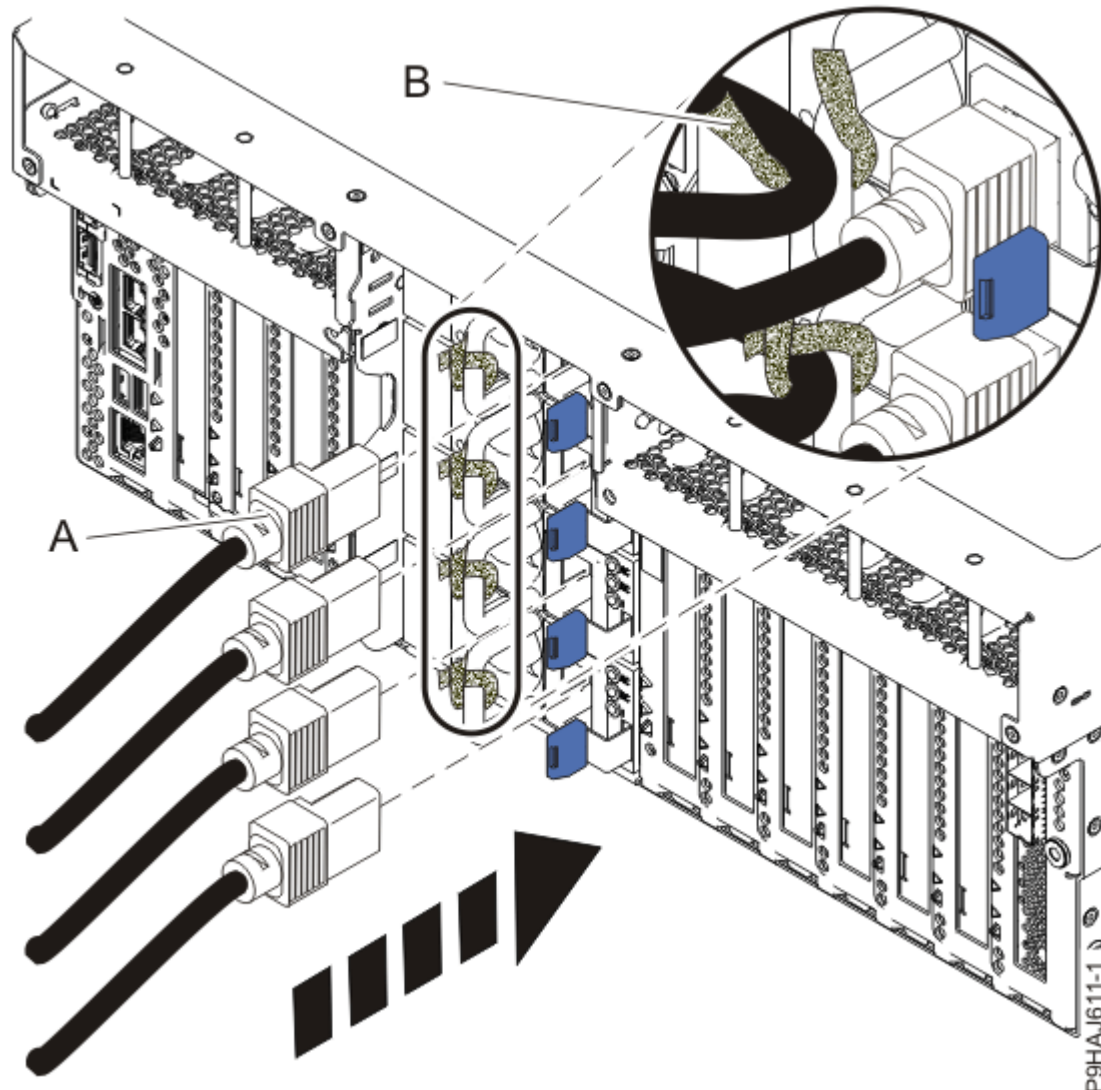
Figura 11. Connexió dels cables d'alimentació a un sistema muntat en bastidor
