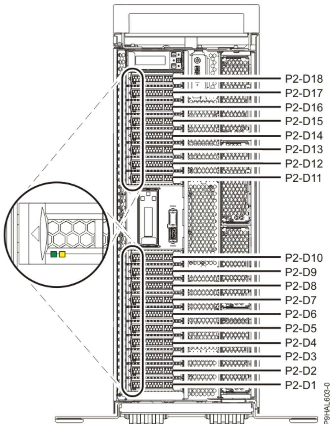
Figura 31. Ubicacions de les unitats de disc o unitats d'estat sòlid i dels indicadors de servei en un sistema 9009-41A, 9009-42A o 9223-42H autònom
