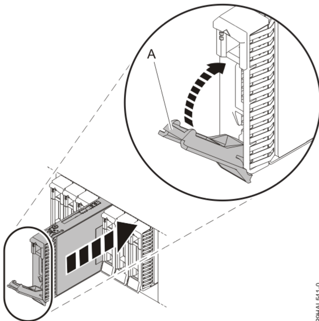
Figura 9. Instal·lació d'una unitat en un sistema
