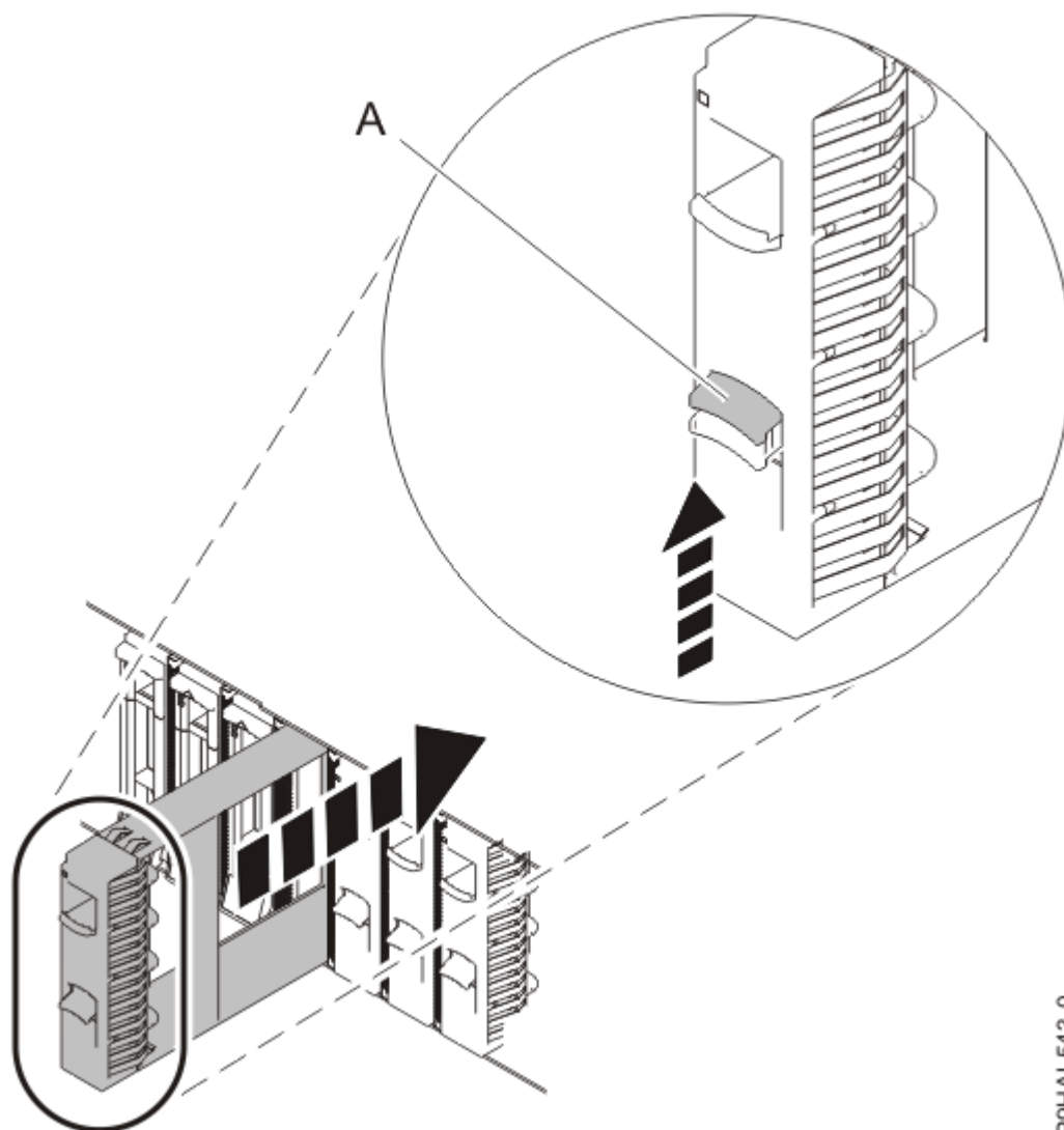
Figura 35. Instal·lació d'un panell de rebliment d'una unitat en un sistema
