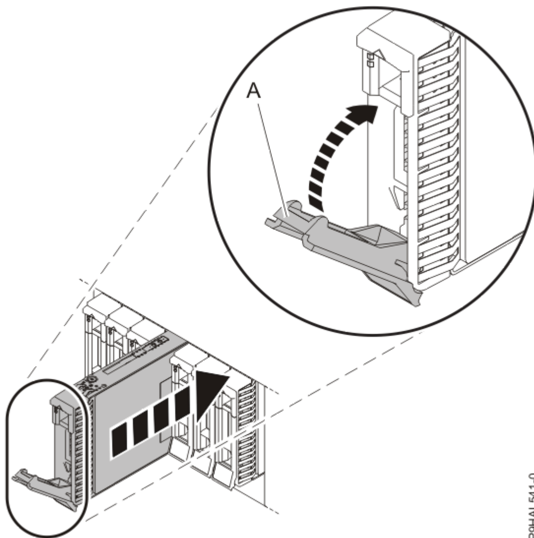
Figura 25. Instal·lació d'una unitat en un sistema
