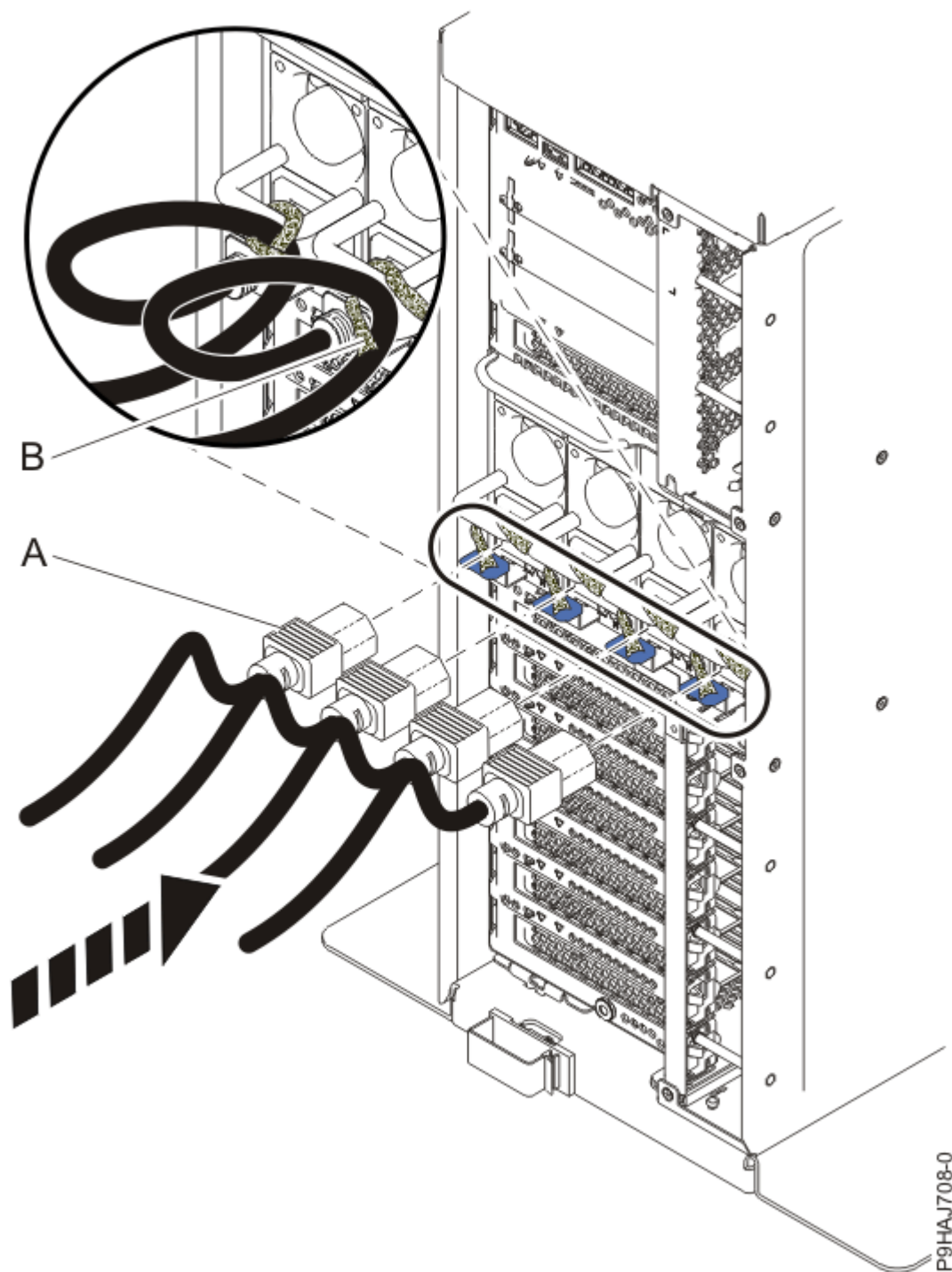
Figura 12. Connexió dels cables d'alimentació en un sistema autònom
