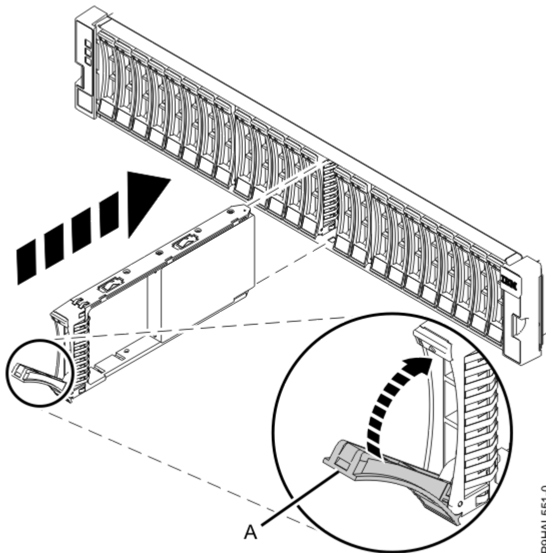
Figura 6. Instal·lació o substitució d'una unitat en un allotjament
