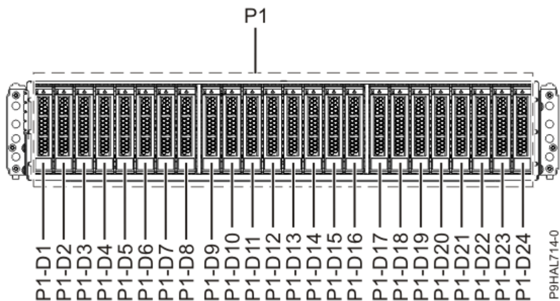
Figura 1. Vista frontal del model 5887 allotjament d'unitat de disc que mostra les ubicacions de les unitats de disc
