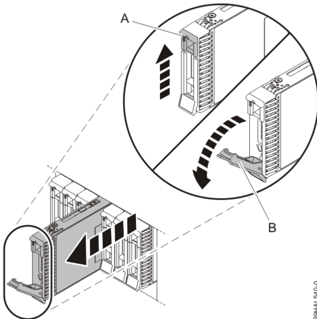
Figura 14. Desbloqueig i extracció de la unitat
