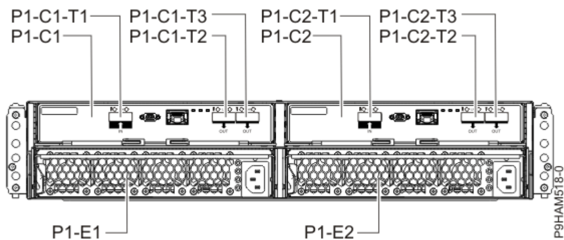
Figura 2. Vista posterior de l'5887 allotjament d'unitat de disc
