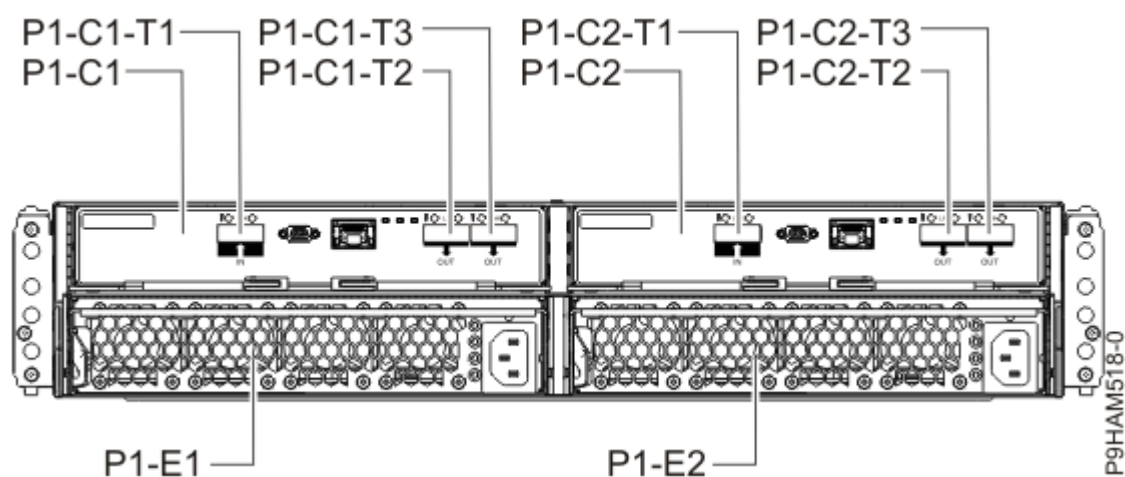
Figura 10. Vista posterior de l'5887 allotjament d'unitat de disc
