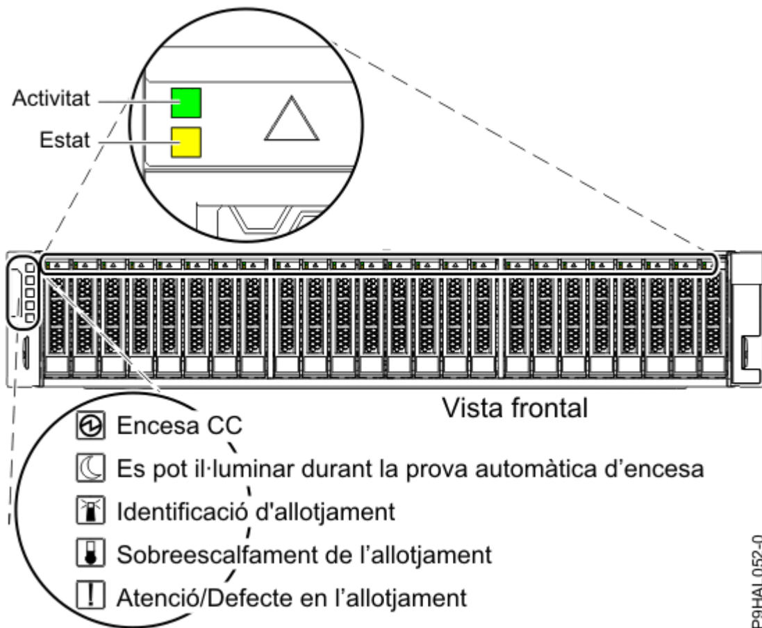
Figura 3. Vista frontal de l'5887 allotjament d'unitat de disc que mostra els indicadors de servei
