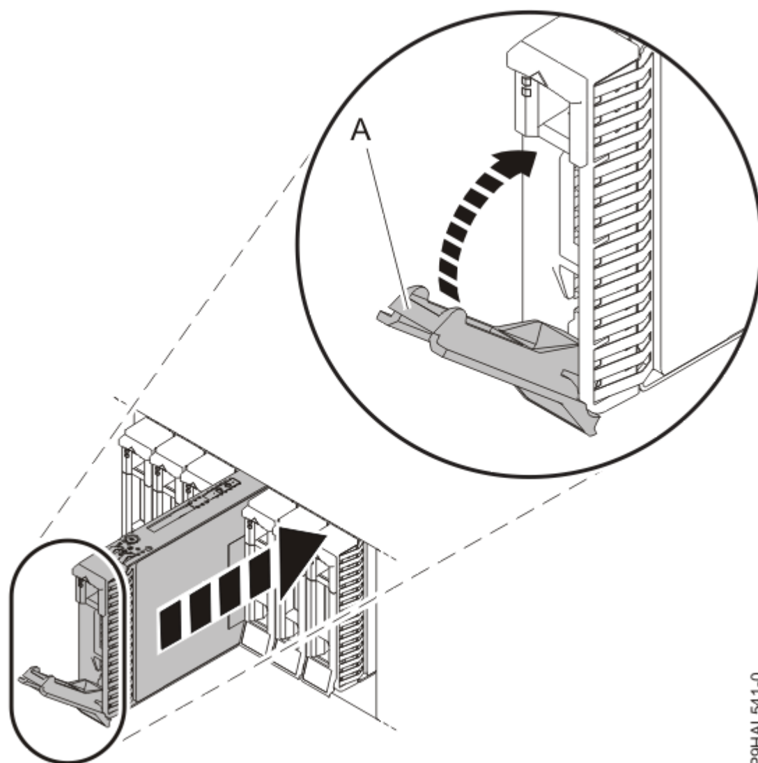
Figura 19. Instal·lació d'una unitat en un sistema
