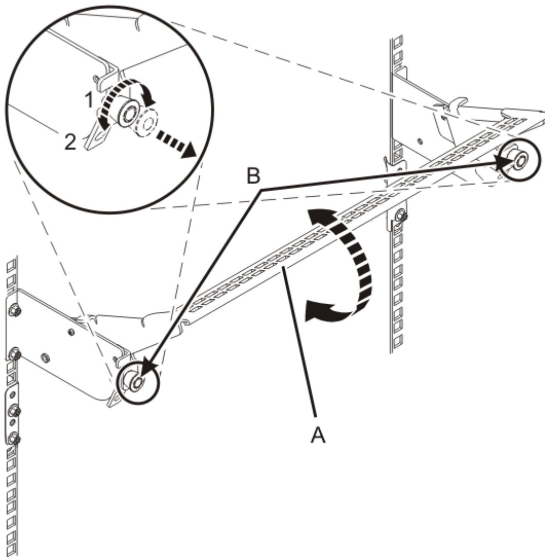
Figura 25. Col·locació de la peça de subjecció portacables en la posició operativa més baixa
