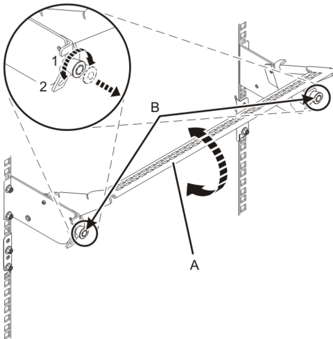
Figura 35. Col·locació de la peça de subjecció portacables en la posició operativa més baixa
