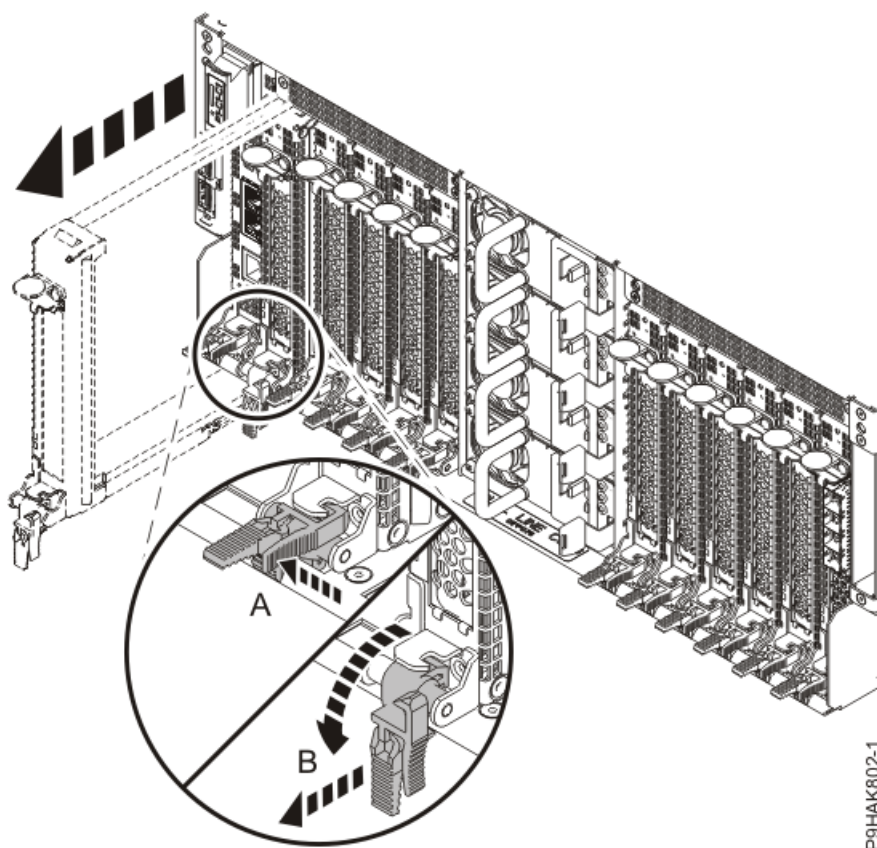
Figura 4. Extracció d'una casset d'adaptador del sistema 9040-MR9
