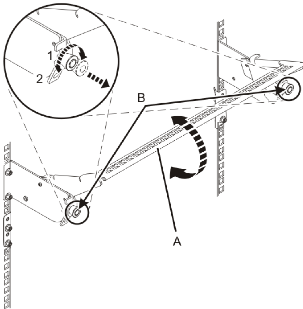
Figura 16. Col·locació de la peça de subjecció portacables en la posició de servei elevada
