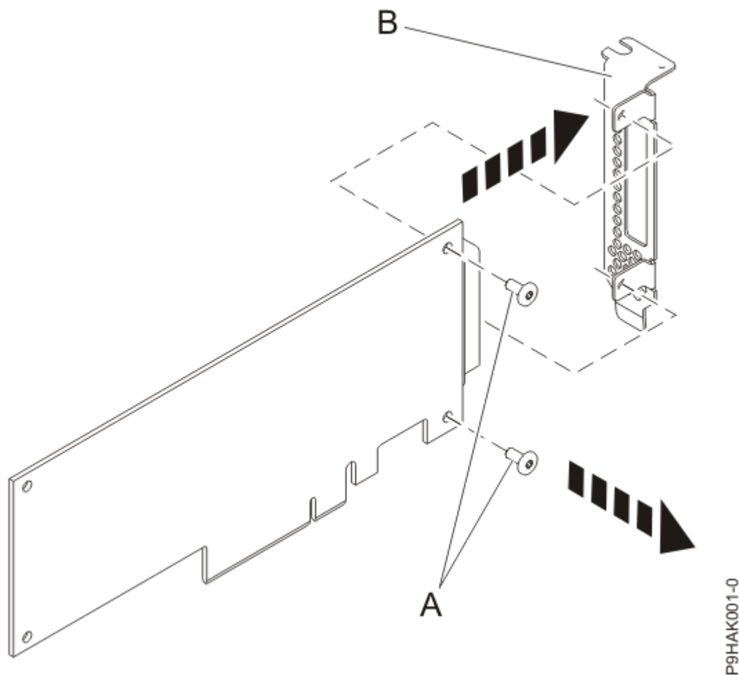
Figura 36. Extracció de la contrapunta de perfil baix d'un adaptador
