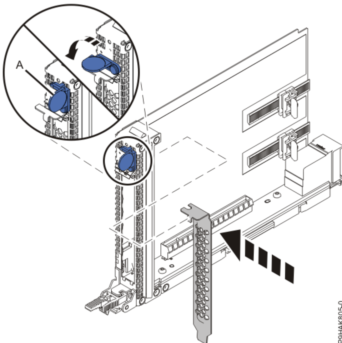
Figura 32. Substitució d'un adaptador a una casset per al sistema 9040-MR9
