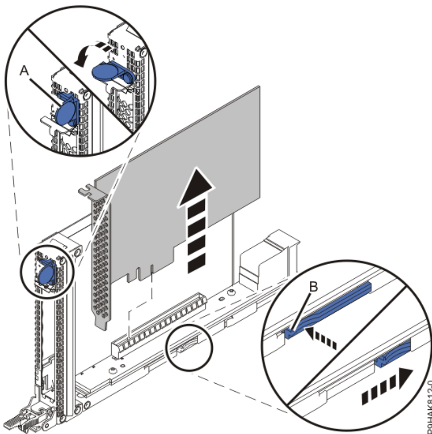
Figura 19. Extracció d'un adaptador d'una casset per al sistema 9040-MR9
