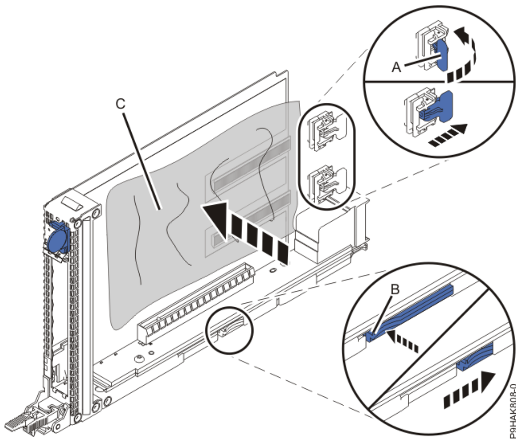
Figura 6. Col·locació d'un full de seguretat de descàrrega electrostàtica damunt les bandes de la casset del model 9040-MR9
