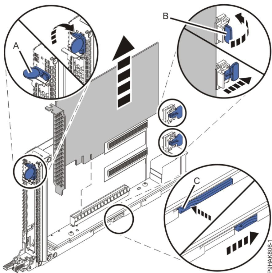
Figura 30. Extracció d'un adaptador d'una casset per al sistema 9040-MR9
