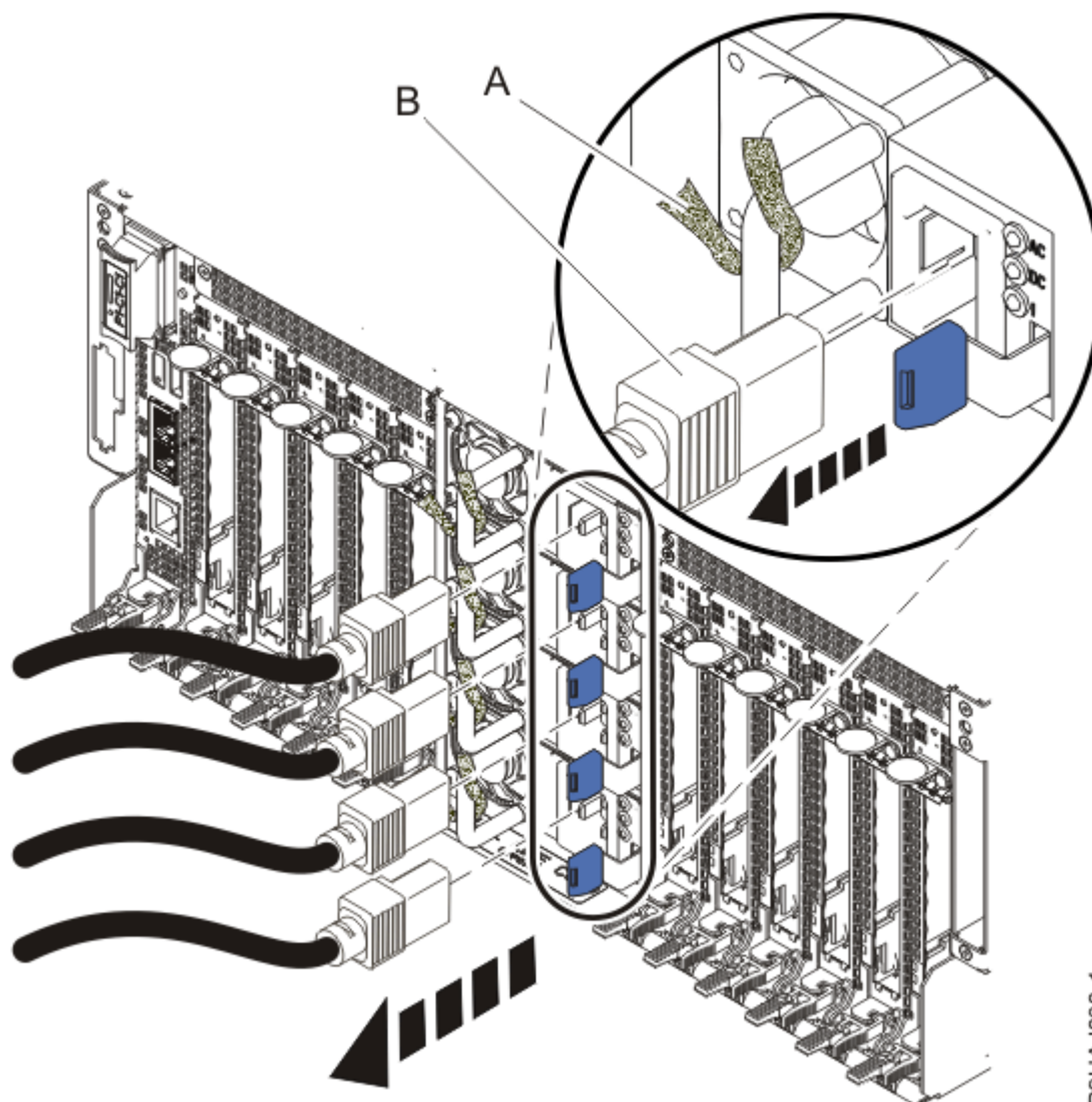
Figura 27. Extracció dels cables d'alimentació
