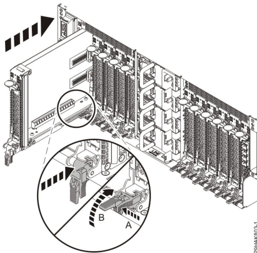
Figura 24. Instal·lació d'una casset al model 9040-MR9
