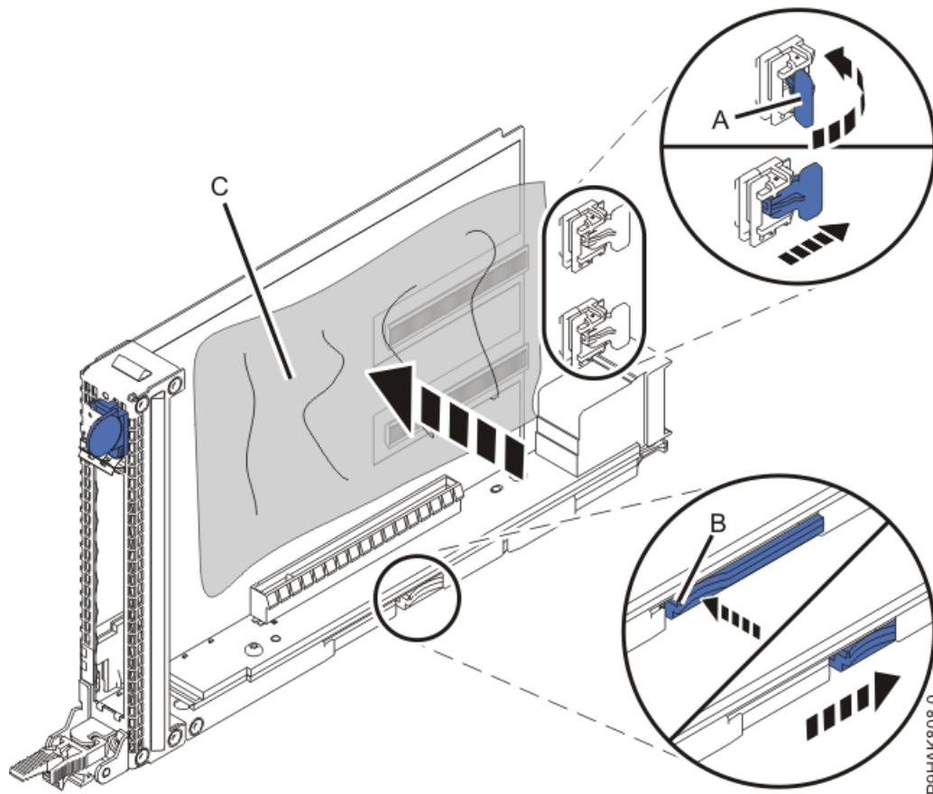
Figura 20. Col·locació d'un full de seguretat de descàrrega electrostàtica damunt les bandes de la casset del model 9040-MR9
