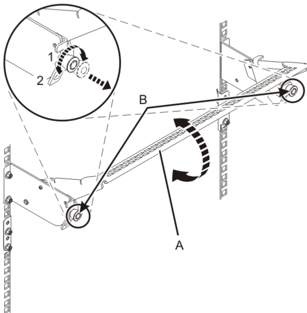
Figura 28. Col·locació de la peça de subjecció portacables en la posició de servei elevada
