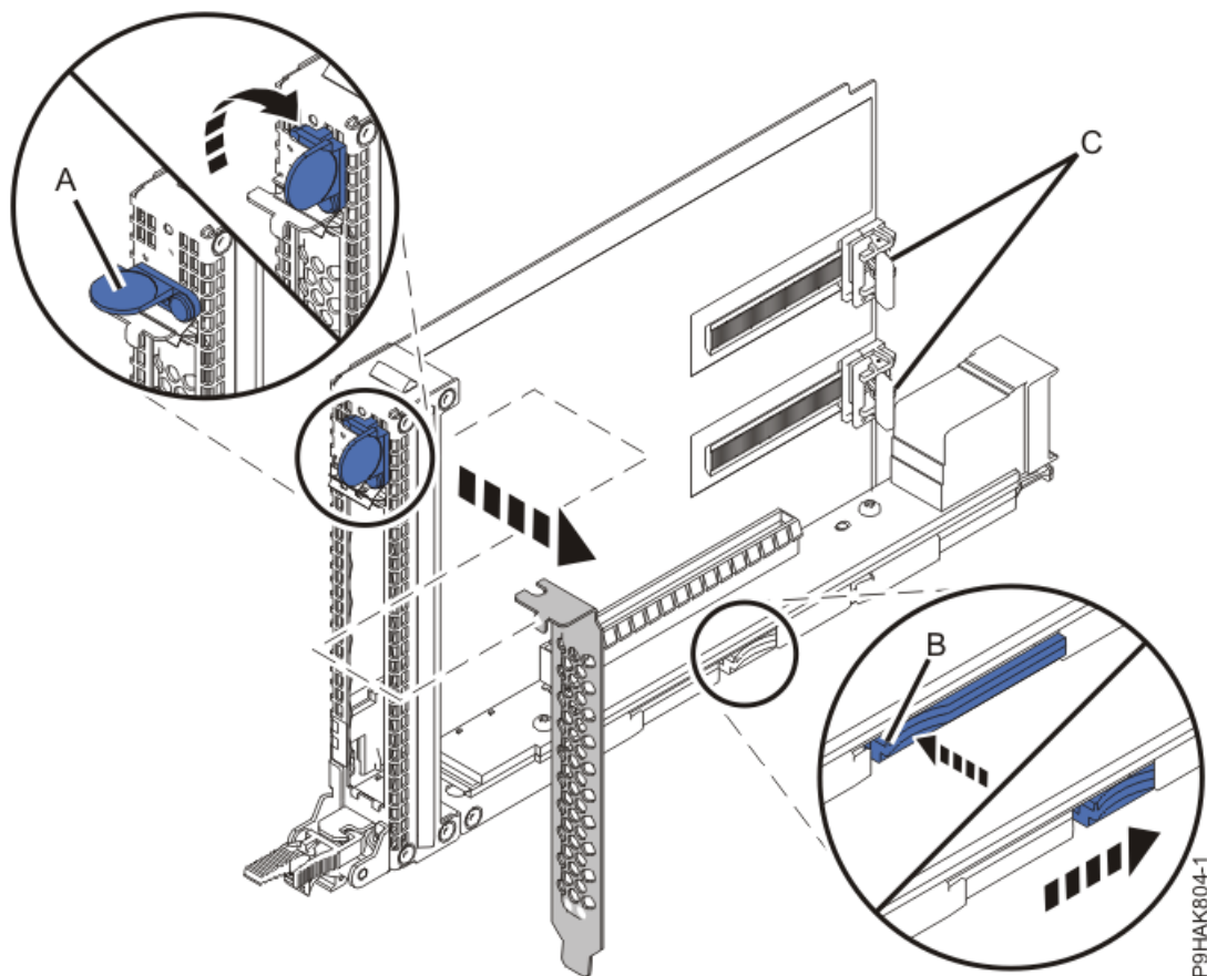
Figura 5. Extracció de la casset d'un panell de reblliment de contrapunta per al sistema 9040-MR9
