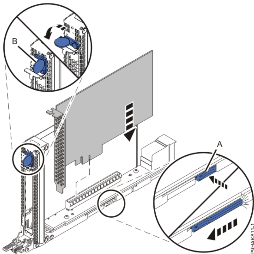
Figura 9. Instal·lació d'un adaptador a la casset per al sistema 9040-MR9
