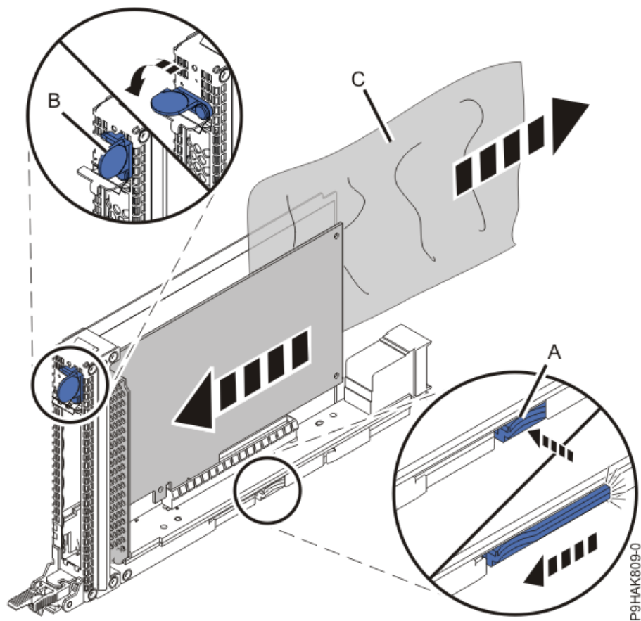
Figura 21. Instal·lació d'un adaptador a la casset per al sistema 9040-MR9
