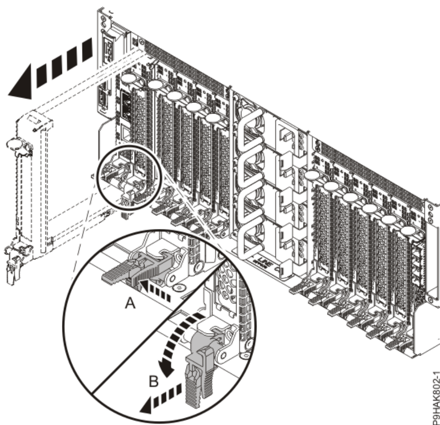
Figura 17. Extracció d'una casset d'adaptador del sistema 9040-MR9
