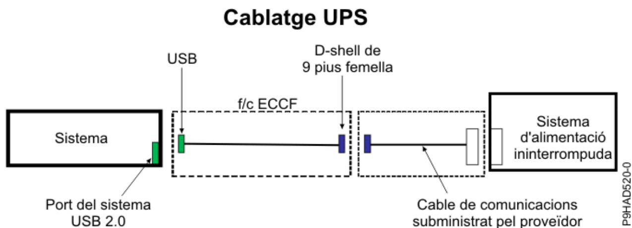
Figura 38. Cablatge UPS per al
