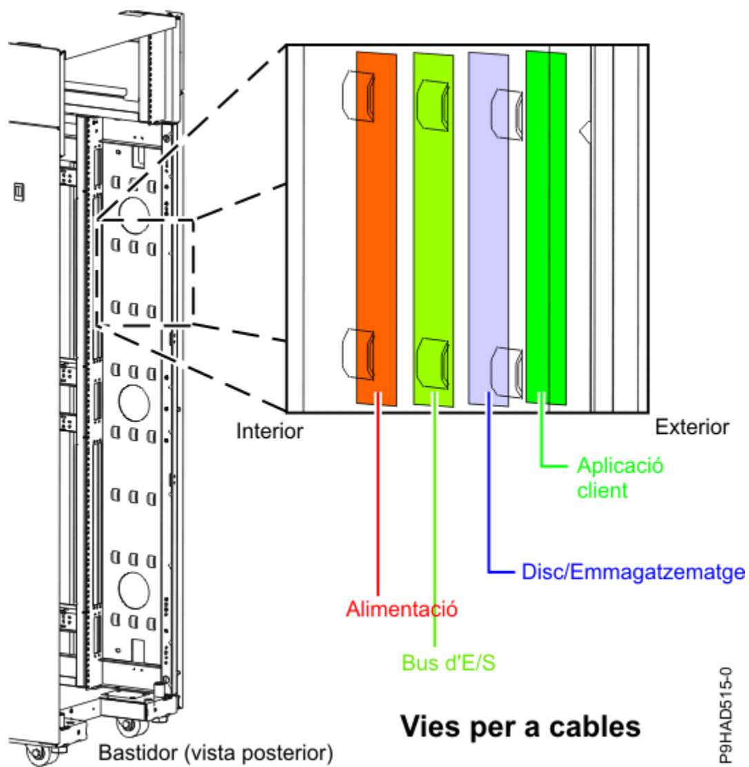
Figura 43. Ponts portacables
