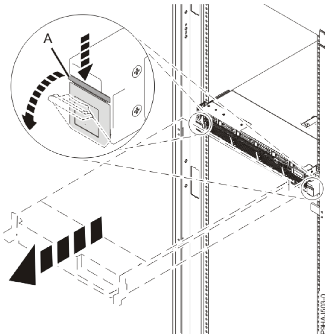
Figura 2. Alliberament dels pestells laterals
