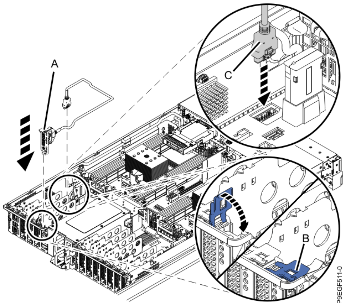
Figura 6. Substitució del cable posterior USB
