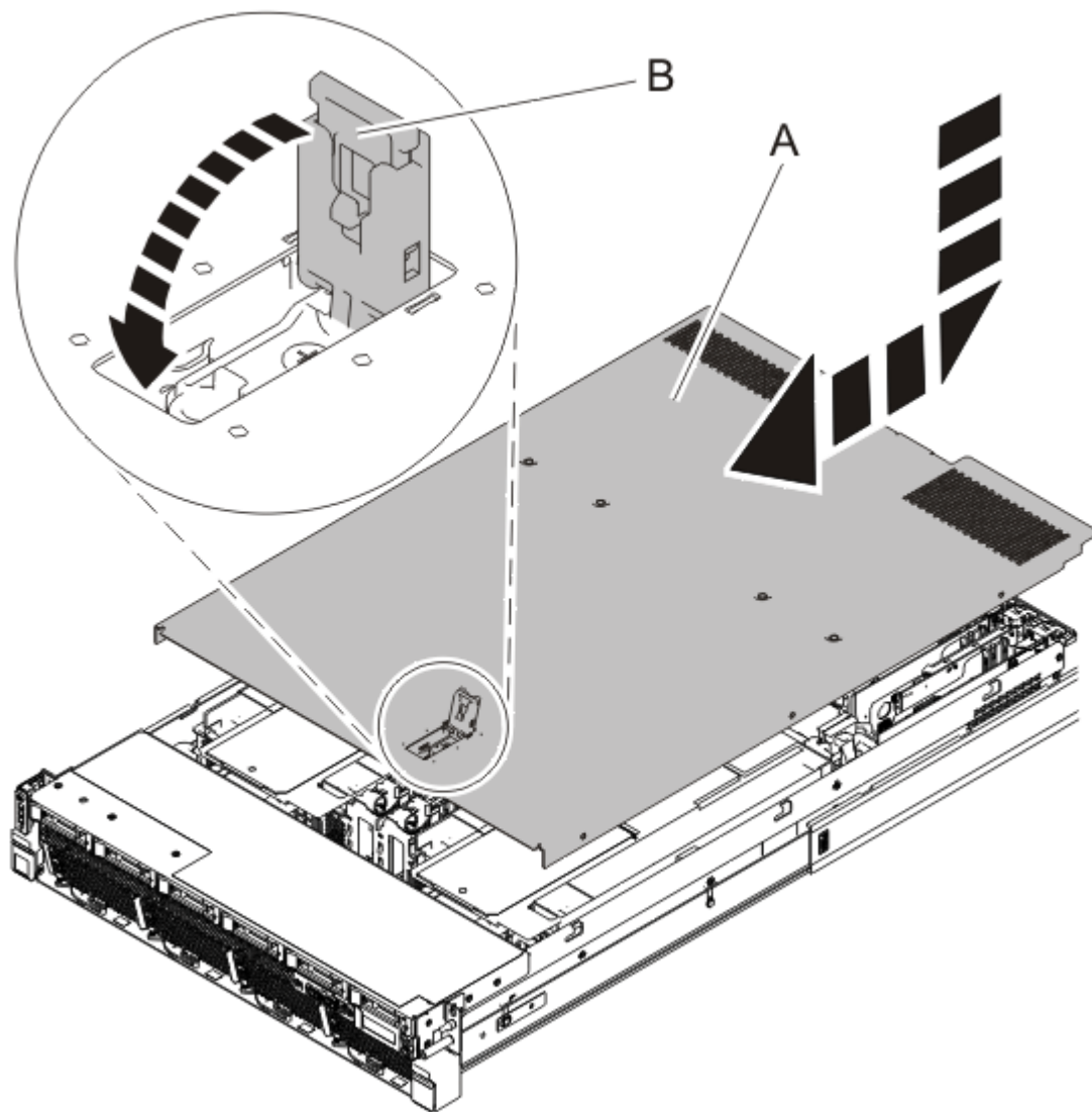
Figura 7. Instal·lació de la coberta d'accés de servei
