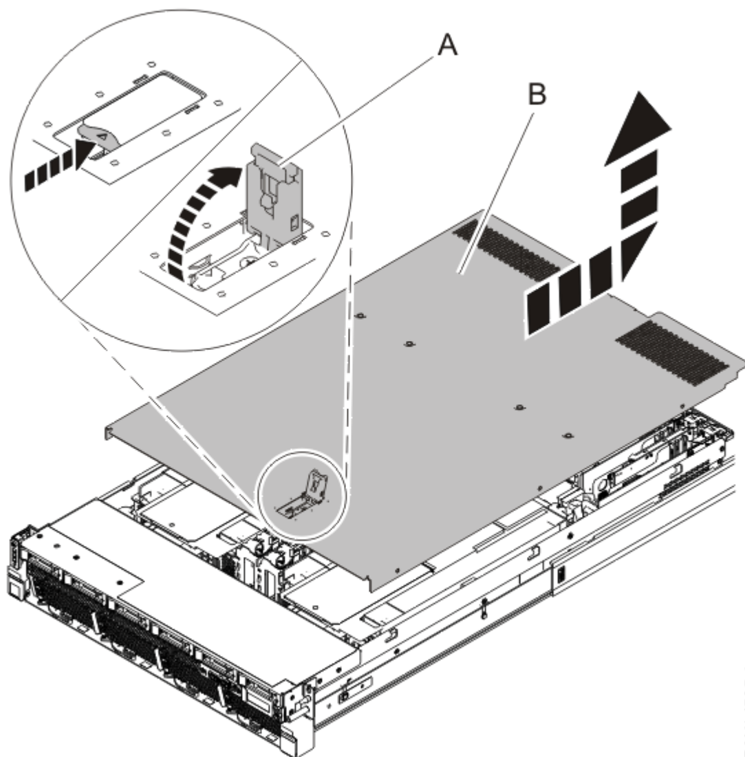
Figura 4. Extracció de la coberta d'accés de servei
