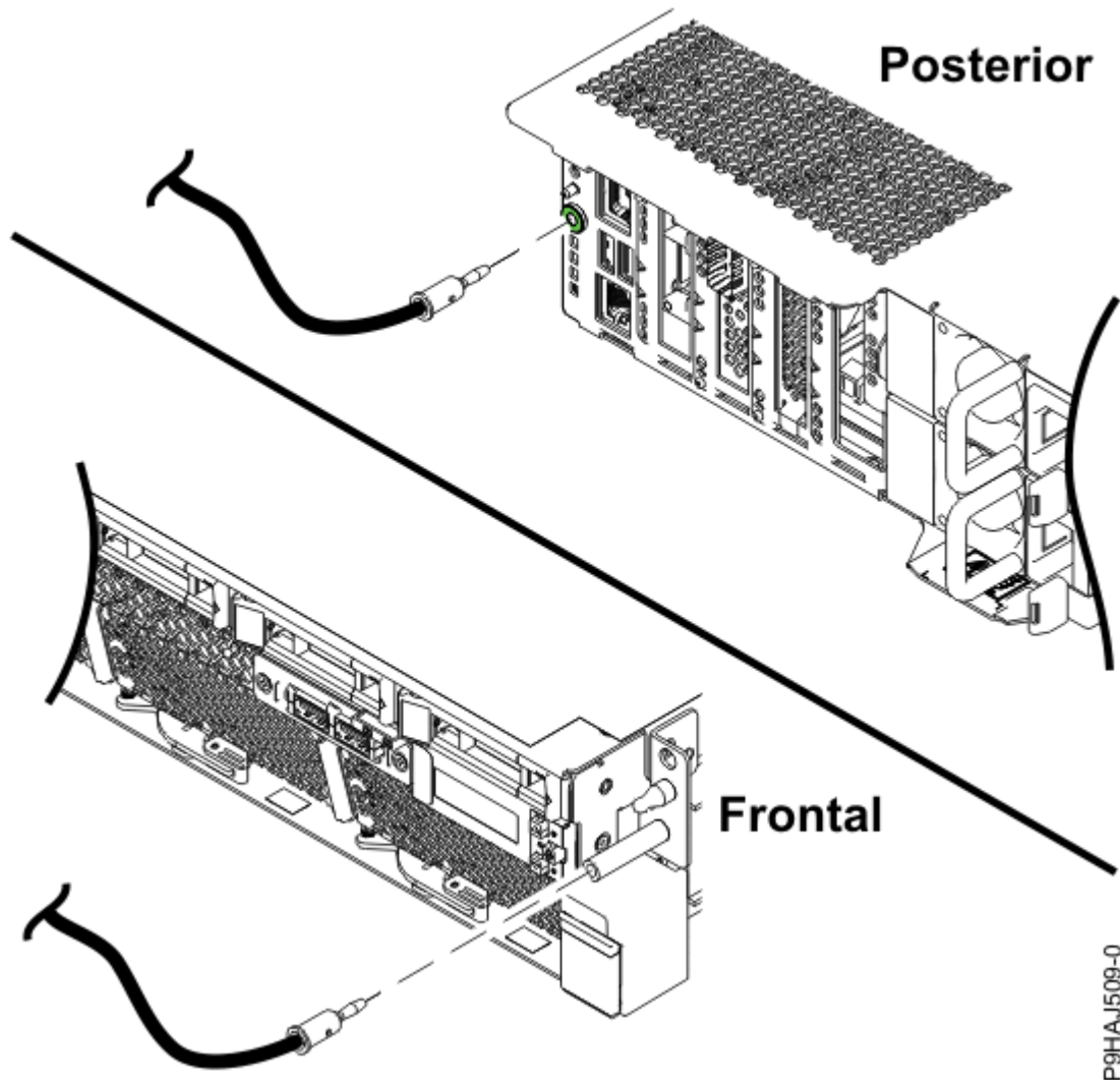
Figura 3. Ubicació dels endolls ESD
