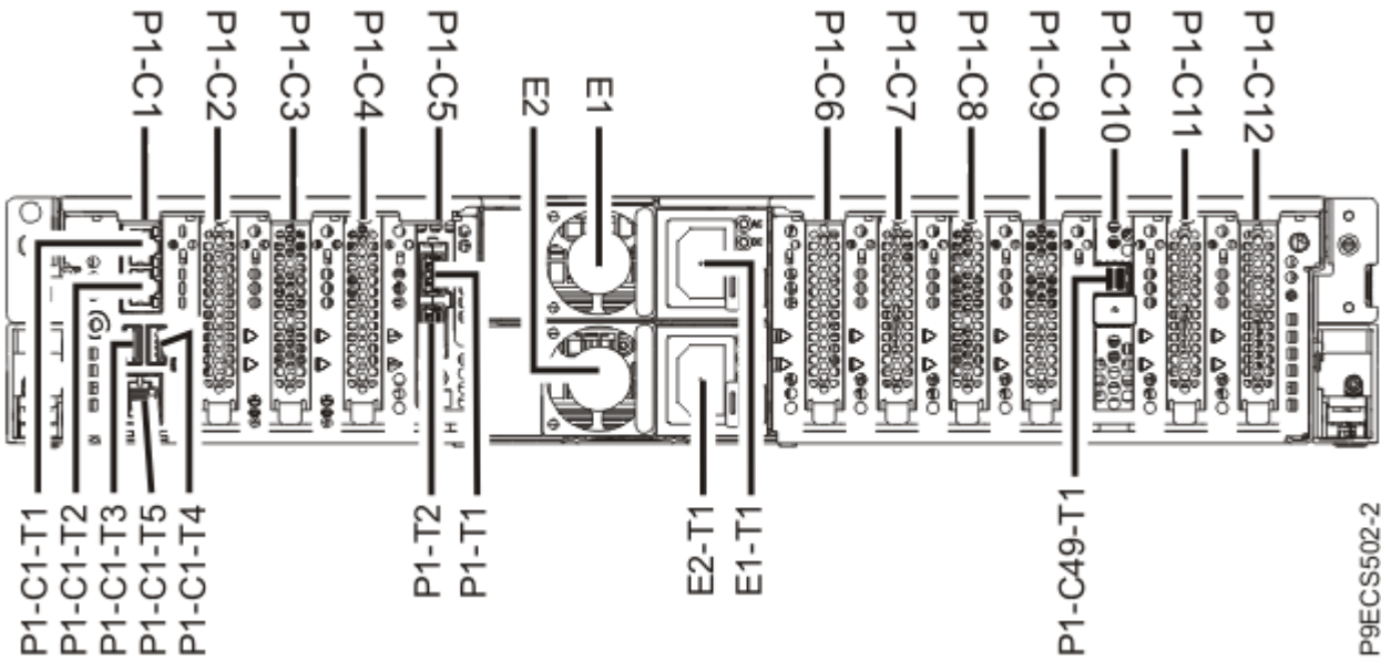
Figura 1. Vista posterior d'un sistema 5105-22E, 9009-22G o 9223-22S muntat en bastidor amb els codis d'ubicació de les ranures PCIe4
