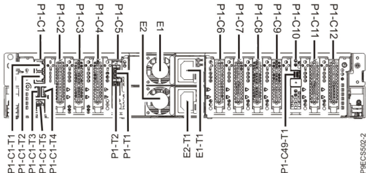
Figura 2. Vista posterior d'un sistema 9008-22L, 9009-22A o 9223-22H muntat en bastidor amb els codis d'ubicació de les ranures PCIe
