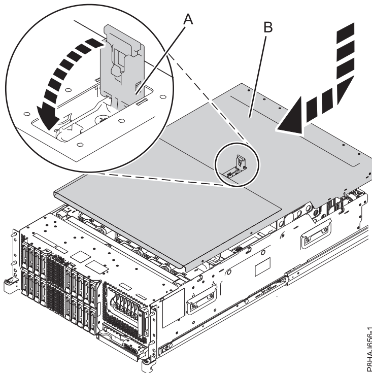
รูปที่ 25. การติดตั้ง ฝาครอบการเข้าถึงเซอรัวิส
