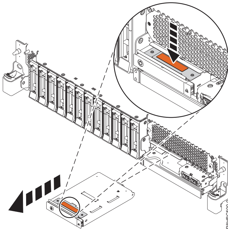
รูปที่ 1. การถอดคอนโทรลพาเนล
