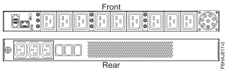
รูปที่ 36. PDU สำหรับระบบ 8408-44E
