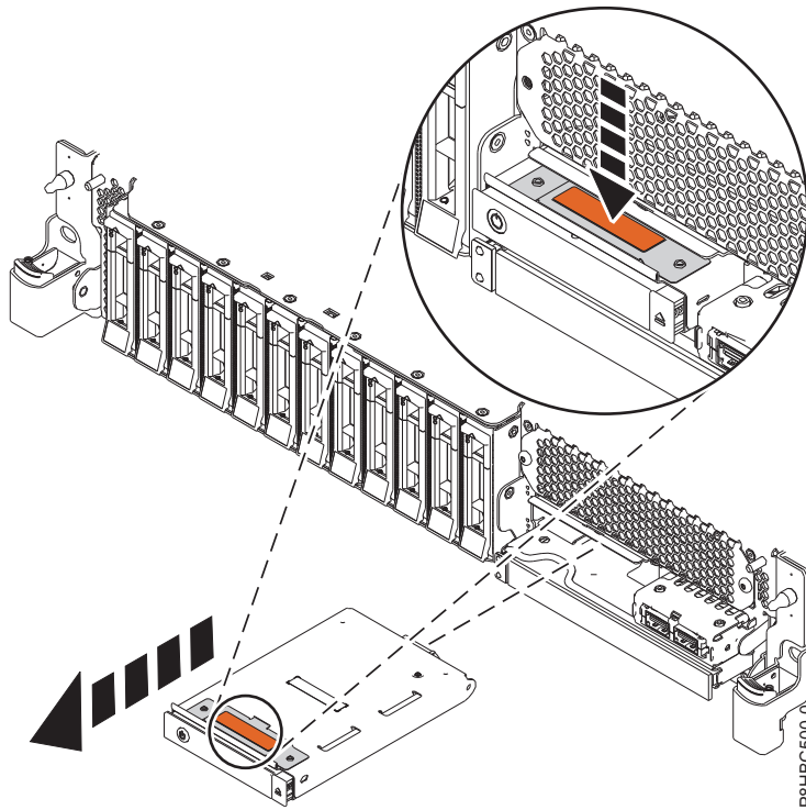
รูปที่ 4. การถอดคอนโทรลพาเนล
