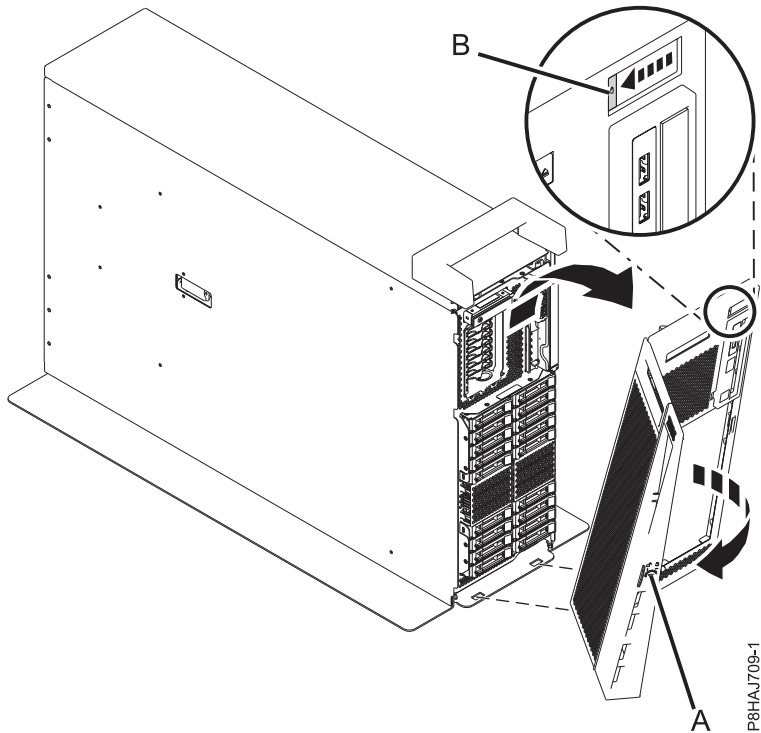
รูปที่ 10. การถอดฝาครอบด้านหน้า
