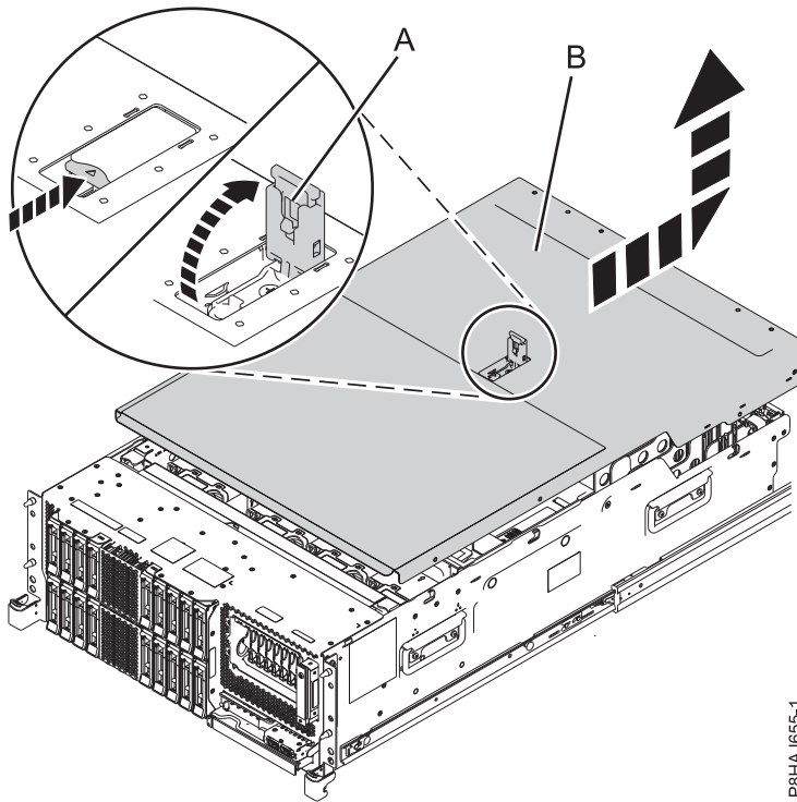
รูปที่ 23. การถอดฝาครอบการเข้าถึงเซอร์วิส
