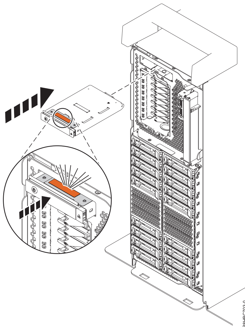
รูปที่ 9. การเปลี่ยนคอนโทรลพาเนลสำหรับระบบแบบสแตนด์อะโลน
