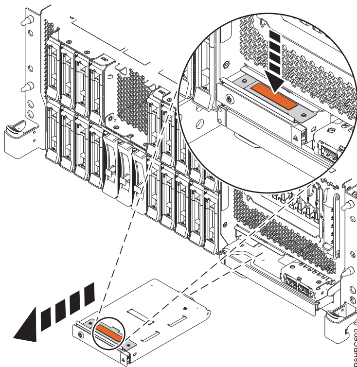
รูปที่ 1. การถอดคอนโทรลพาเนล ออกจากระบบแบบติดตั้งบนชั้นวาง
