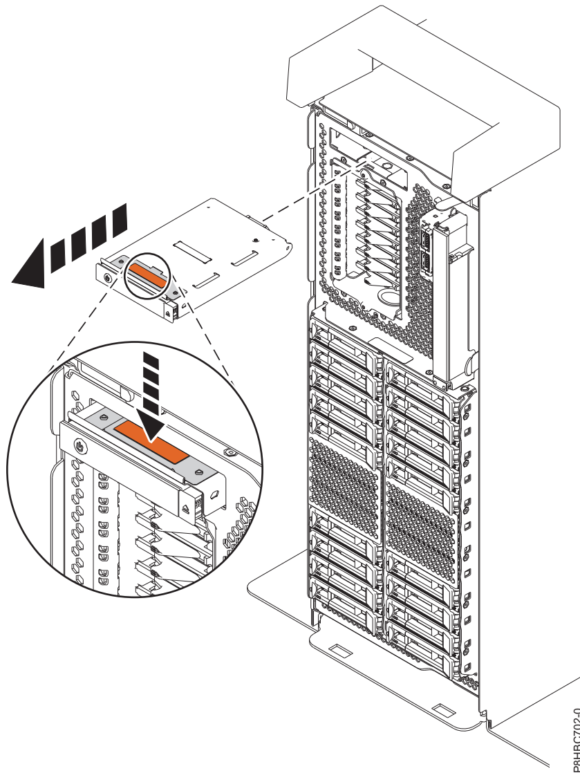
รูปที่ 2. การถอดคอนโทรลพANELออกจากระบบแบบสแตนด์เอโลน
