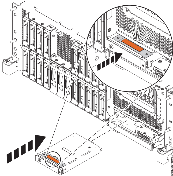
รูปที่ 3. การเปลี่ยนคอนโทรลพาเนลในระบบแบบติดตั้งบนชั้นวาง
