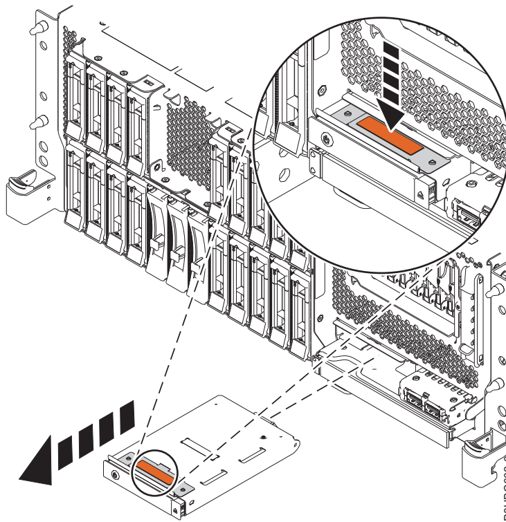
รูปที่ 6. การถอดคอนโทรลพาเนลออกจากระบบแบบติดตั้งบนชั้นวาง
