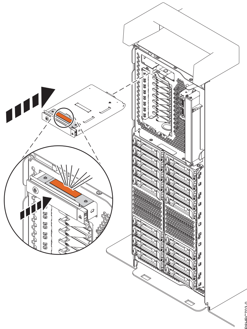
รูปที่ 4. การเปลี่ยนคอนโทรลพาเนลสำหรับระบบแบบสแตนด์อะโลน
