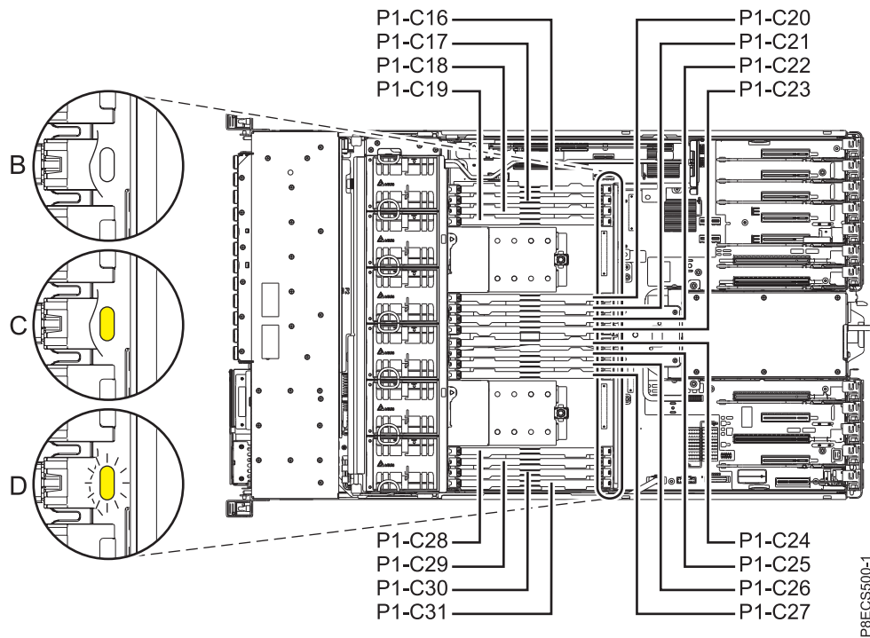
รูปที่ 4. ตำแหน่งสำหรับ โมดูลหน่วยความจำ และตัวบ่งชี้การให้บริการในระบบ 5148-21L, 5148-22L, 8247-21L, 8247-22L, 8284-21A, or 8284-22A
