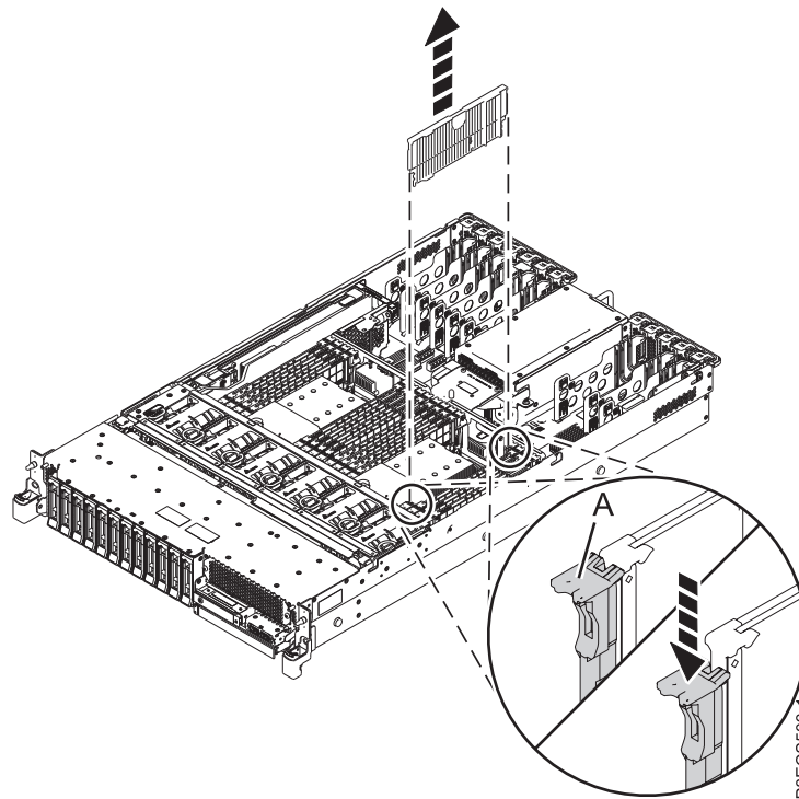
รูปที่ 7. การถอดฟิลเลอร์โมดูลหน่วยความจำออกจาก โมดูลหน่วยความจำ สล็อตในระบบ 5148-21L, 5148-22L, 8247-21L, 8247-22L, 8284-21A, or 8284-22A
