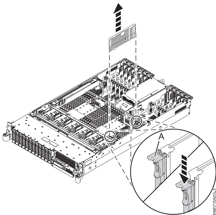
รูปที่ 2. การถอดฟิลเลอร์ โมดูลหน่วยความจำออกจาก โมดูลหน่วยความจำ สล็อตในระบบ 5148-21L, 5148-22L, 8247-21L, 8247-22L, 8284-21A, or 8284-22A
