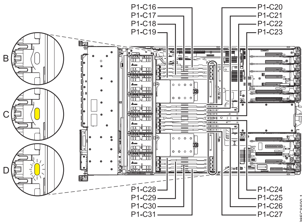
รูปที่ 1. ตำแหน่งสำหรับ โมดูลหน่วยความจำ และตัวบ่งชี้การให้บริการในระบบ 5148-21L, 5148-22L, 8247-21L, 8247-22L, 8284-21A, or 8284-22A
