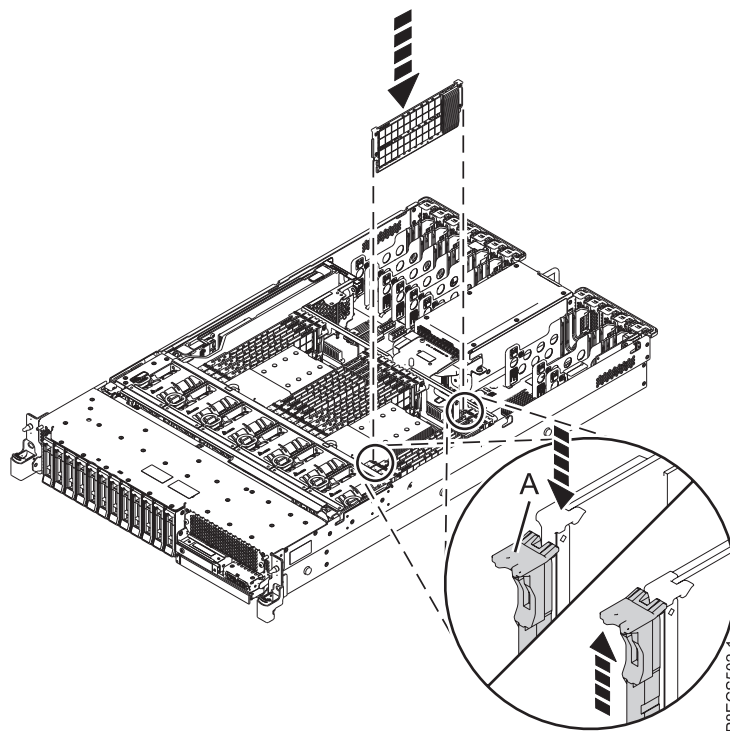
รูปที่ 8. การติดตั้งหรือการเปลี่ยน โมดูลหน่วยความจำ ในระบบ 5148-21L, 5148-22L, 8247-21L, 8247-22L, 8284-21A, or 8284-22A
