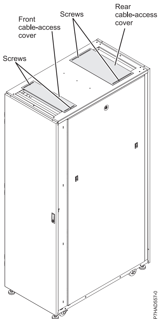
รูปที่ 34. ฝาครอบ การเข้าถึงสายเคเบิล
