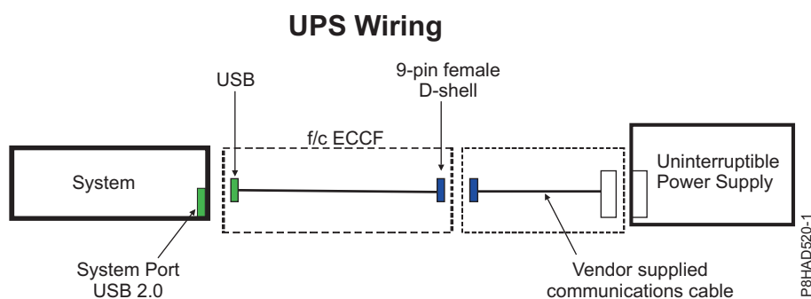
รูปที่ 58. การเดินสาย UPS สำหรับ 5148-21L, 5148-22L, 8247-21L, 8247-21L, 8247-22L, 8247-42L, 8284-22A, 8286-41A และ 8286-42A
