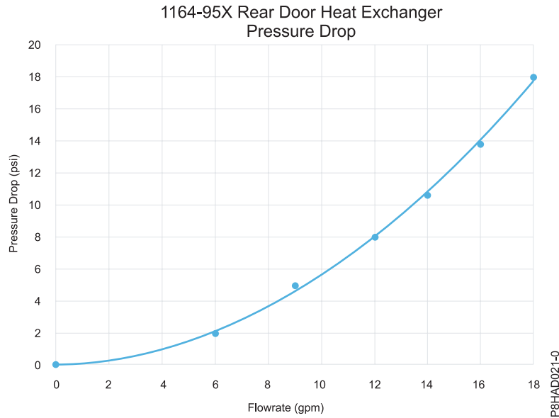
รูปที่ 39. ความดันลด (หน่วยมาตรฐาน)
