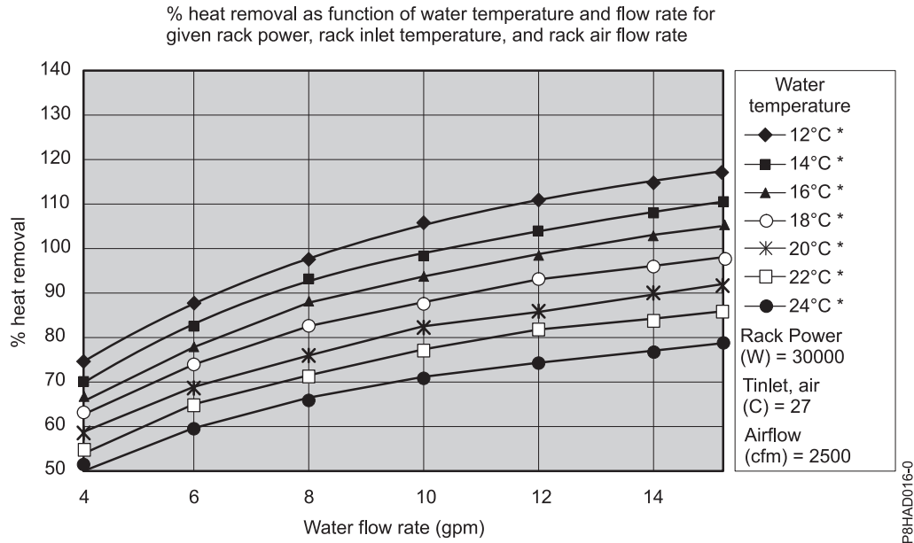
รูปที่ 54. ประสิทธิภาพการทำงานปกติของตัวแลกเปลี่ยนความร้อน โหลดความร้อน 30 kW
