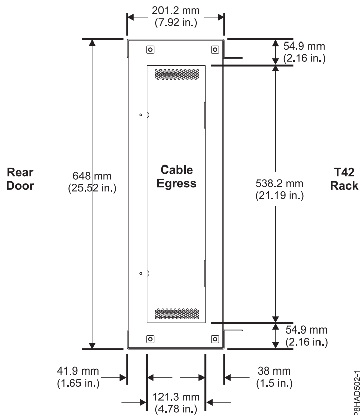
รูปที่ 29. ส่วนขยายชั้นวางด้านหลัง FC ERGO (มองจากด้านบน)
