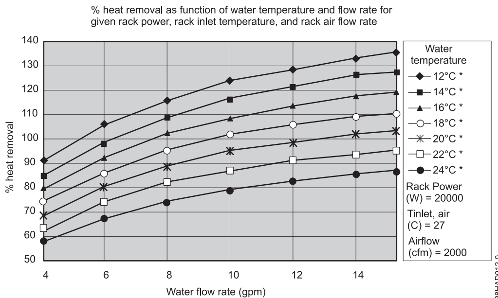
รูปที่ 53. ประสิทธิภาพการทำงานโดยปกติของตัวแลกเปลี่ยนความร้อน โหลดความร้อน 20 kW
