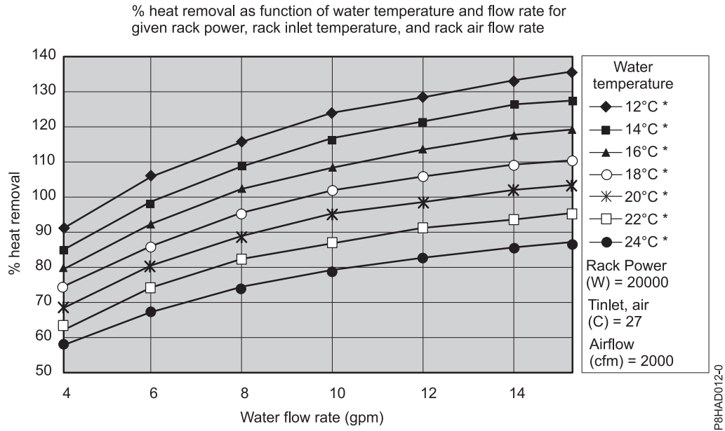
รูปที่ 37. ประสิทธิภาพการทำงานโดยปกติของตัวแลกเปลี่ยนความร้อน โหลดความร้อน 20 kW
