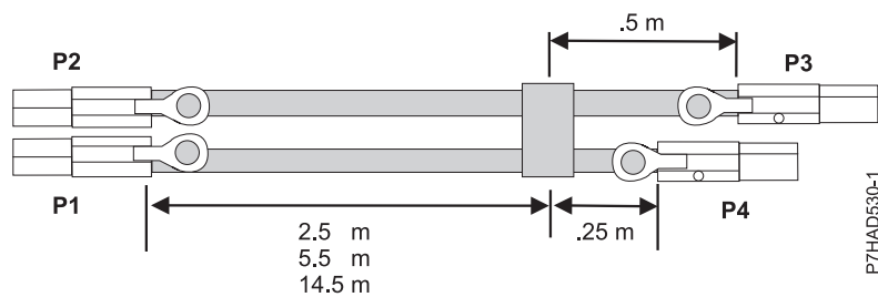
รูปที่ 66. ความยาวชุดสายเคเบิล SAS X ภายนอก
