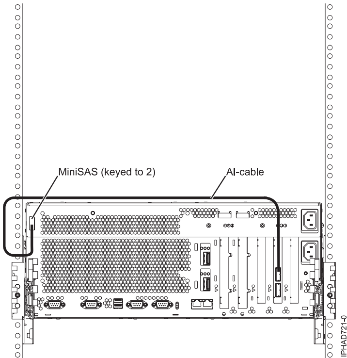
รูปที่ 76. จากอะแดปเตอร์ SAS ไปยังดิสก์สล็อต SAS ภายในผ่านทางพอร์ต SAS ภายนอกของระบบ
