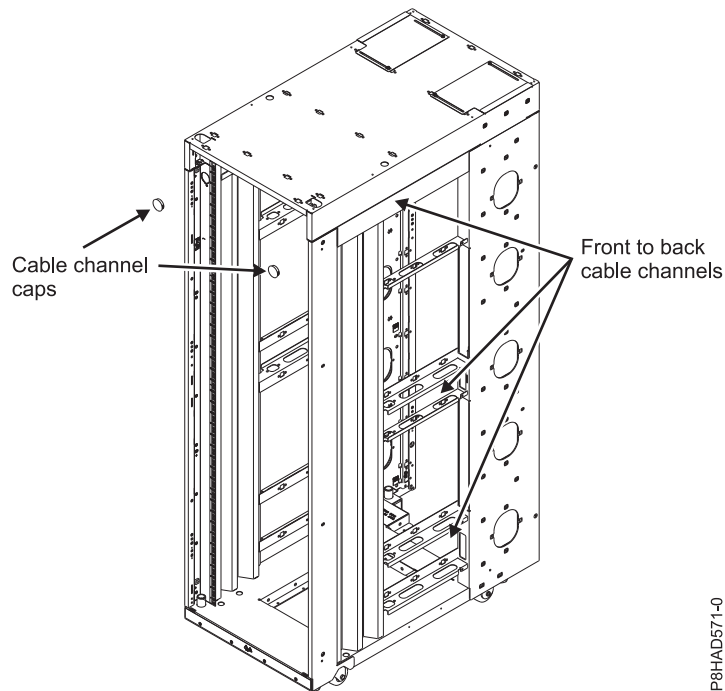
รูปที่ 49. การเดินสายภายในชั้นวาง
