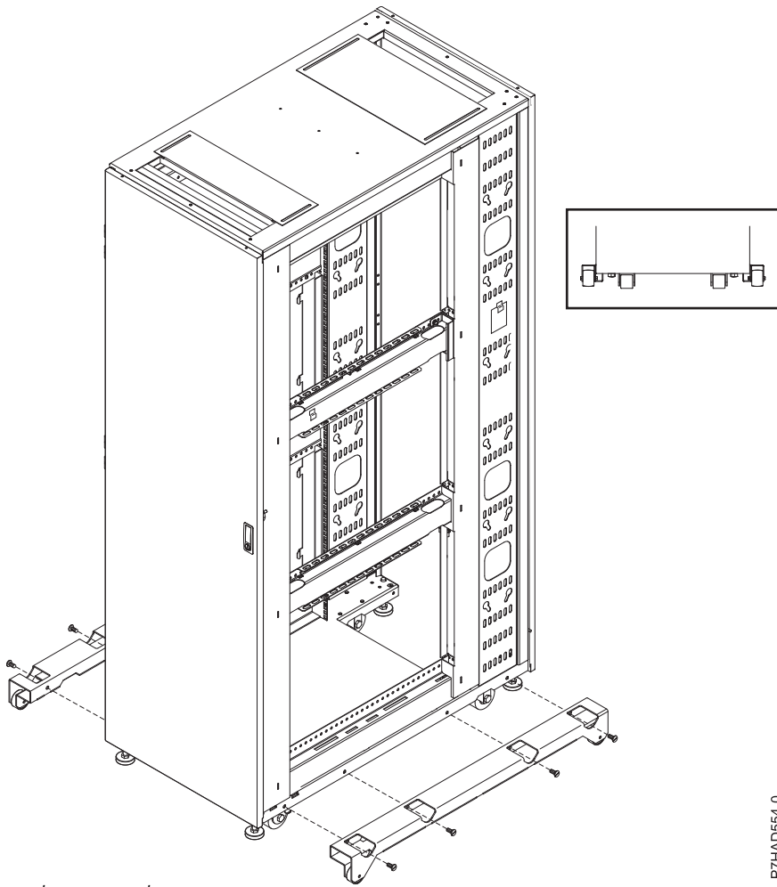
รูปที่ 35. ตำแหน่งของ Outtrigger
