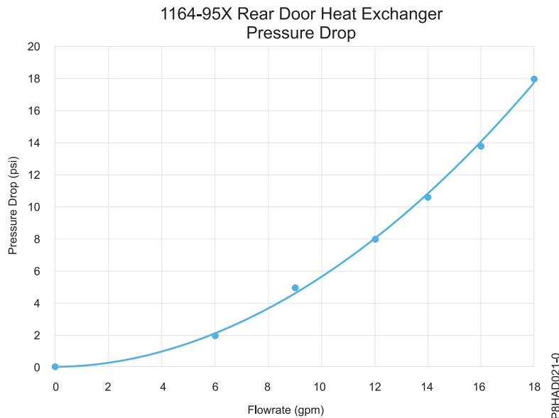
รูปที่ 55. ความดันลด (หน่วยมาตรฐาน)
