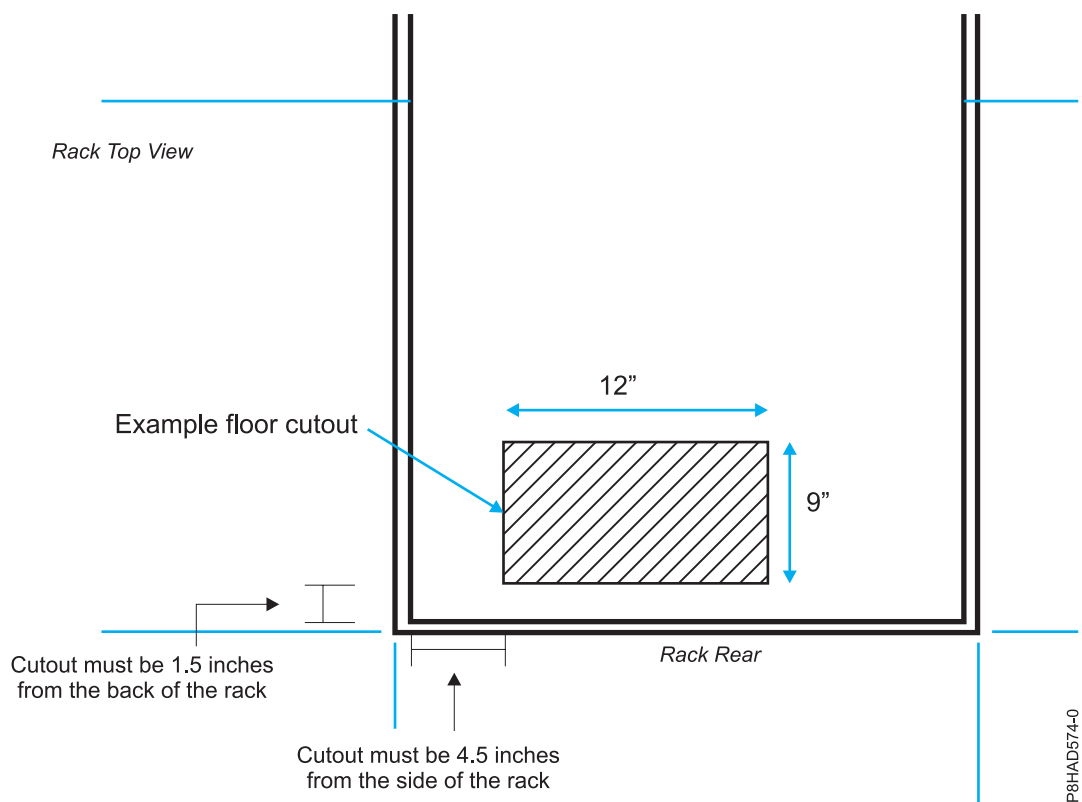
รูปที่ 48. ช่องเจาะที่พื้น
