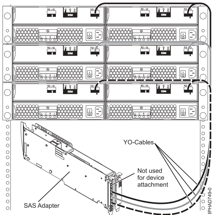
รูปที่ 72. จากอะแดปเตอร์ tri-port SAS ไปยังลิ้นชักส่วนขยายดิสก์
