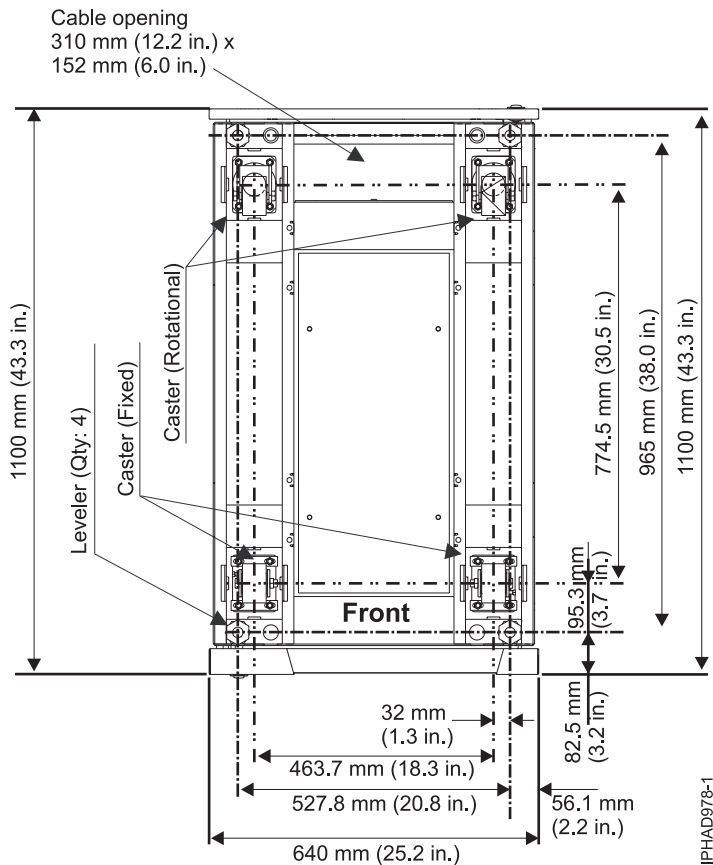
รูปที่ 9. ตำแหน่งลูกล้อและตัวปรับระดับ
