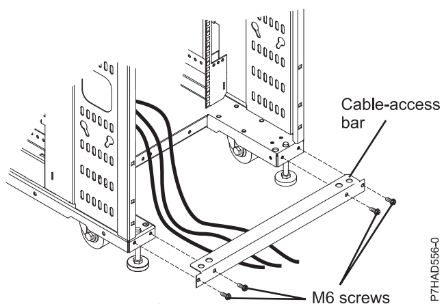
รูปที่ 33. แถบสำหรับเข้าถึงสายเคเบิล
