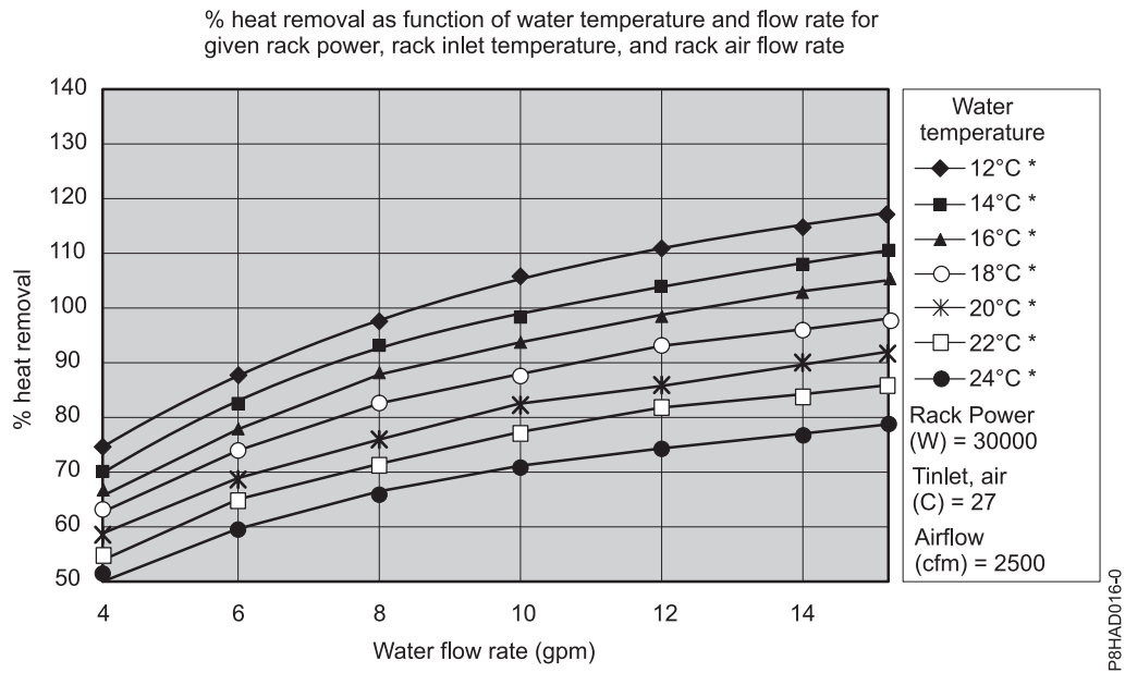
รูปที่ 38. ประสิทธิภาพการทำงานปกติของตัวแลกเปลี่ยนความร้อน โหลดความร้อน 30 kW
