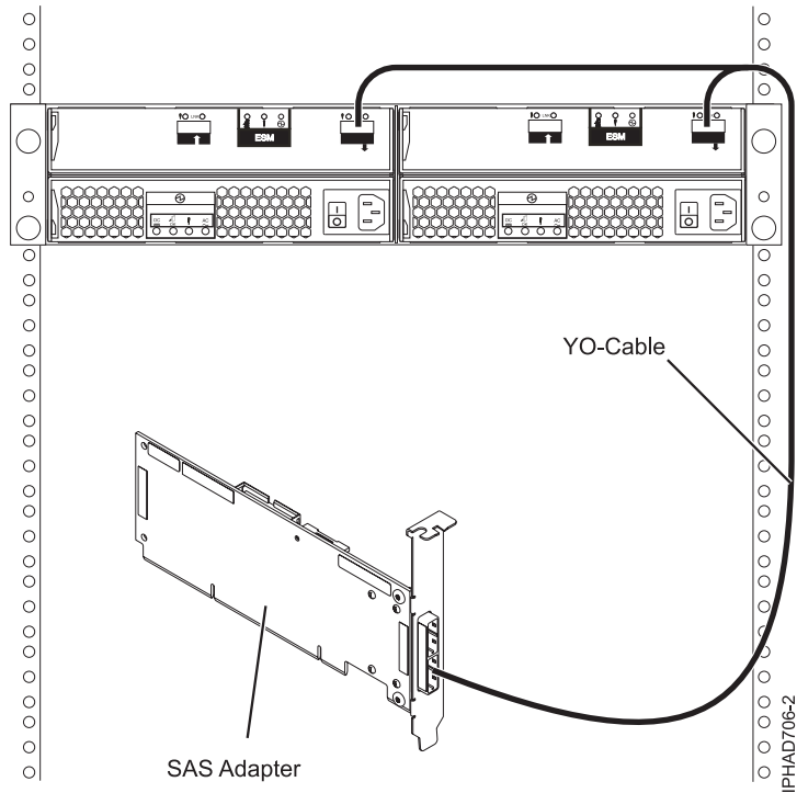
รูปที่ 69. จากอะแดปเตอร์ SAS ไปยังลิ้นชักส่วนขยายดิสก์หนึ่งลิ้นชัก
