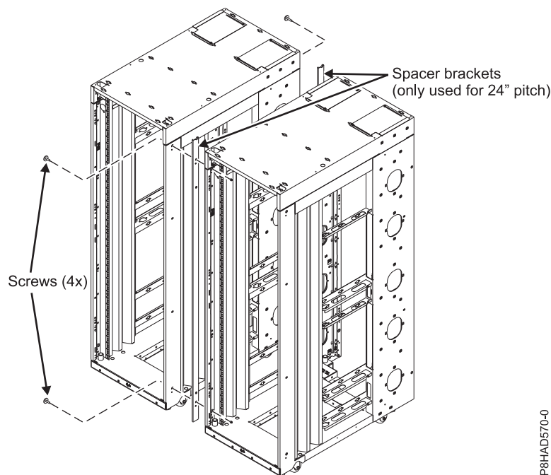
รูปที่ 52. การเชื่อมต่อชั้นวางหลายชั้น
