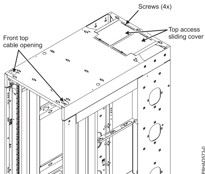
รูปที่ 51. การเดินสายด้านบน
