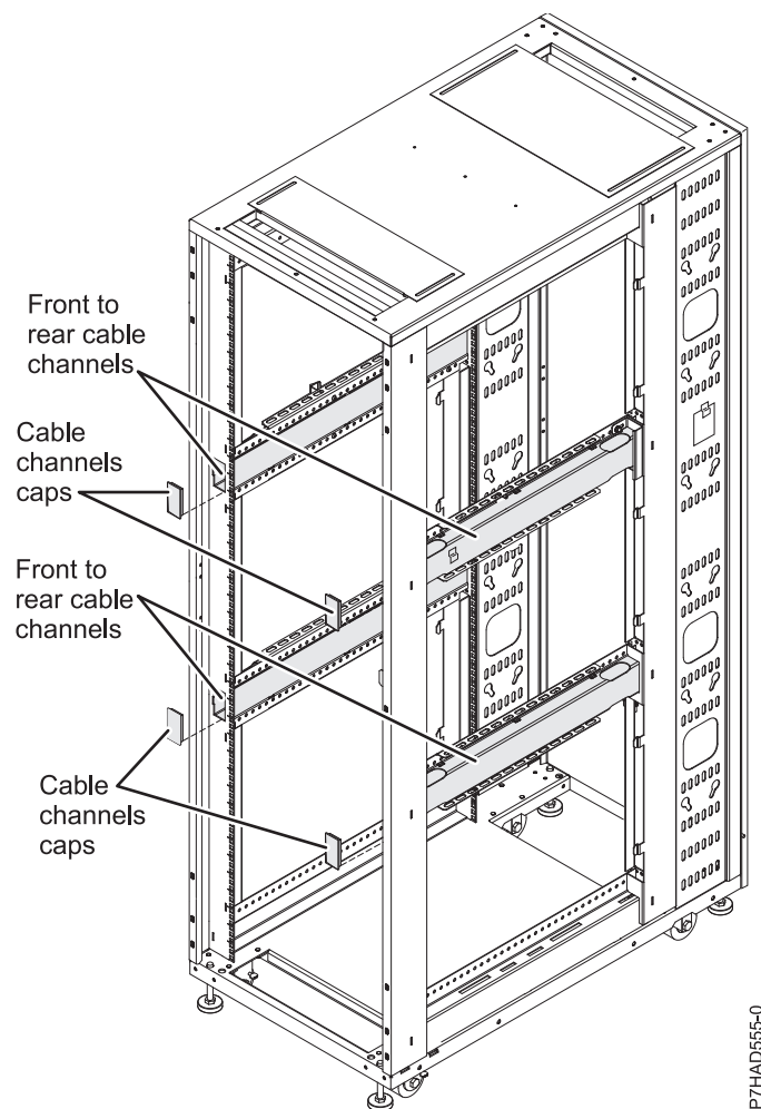
รูปที่ 32. การเดินสายภายในชั้นวาง
