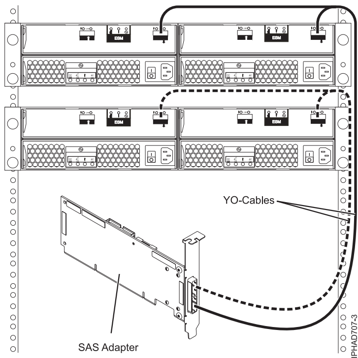
รูปที่ 70. จากอะแดปเตอร์ SAS ไปยังลิ้นชักส่วนขยายดิสก์ 2 ลิ้นชัก
