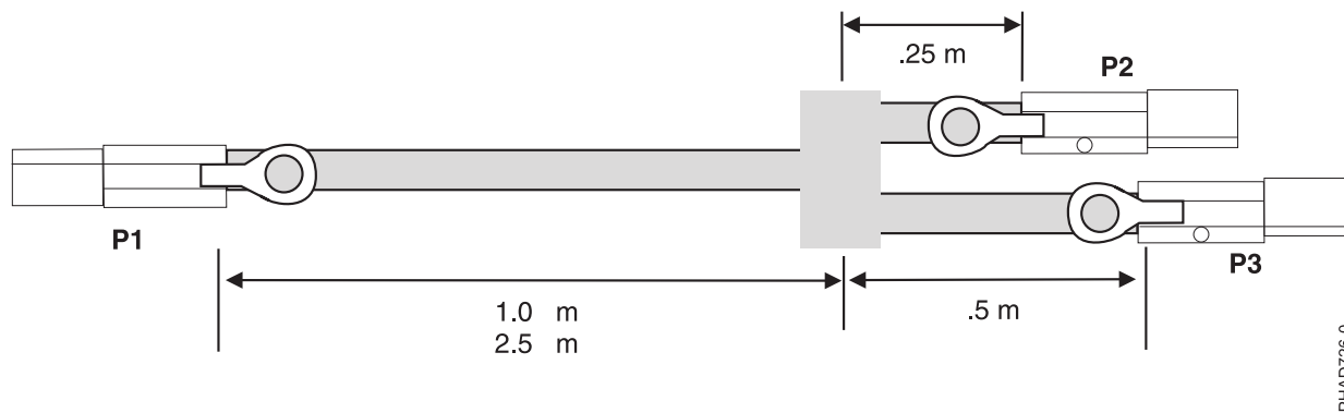
รูปที่ 68. ความยาวชุดสายเคเบิล SAS YI ภายนอก
