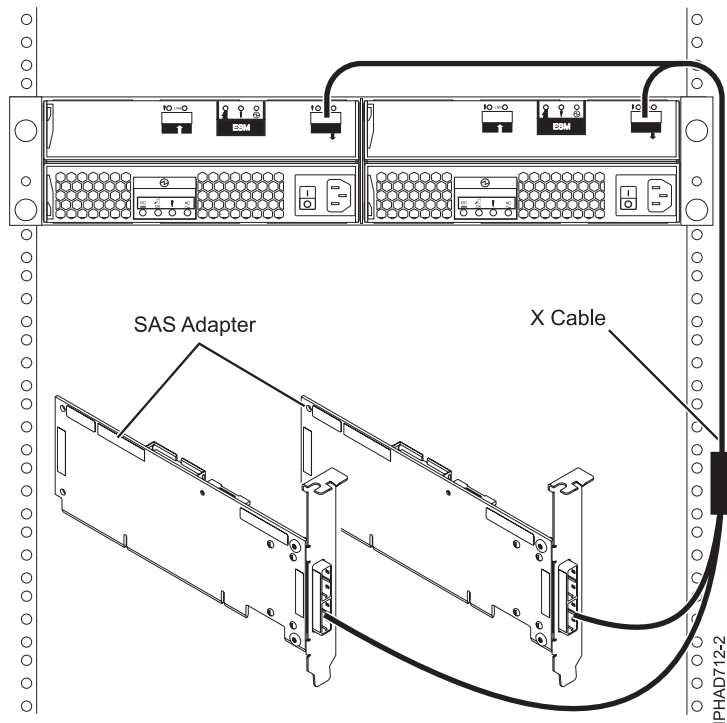
รูปที่ 78. จากอะแดปเตอร์ SAS RAID สองตัวไปยังลิ้นชักส่วนขยายดิสก์ในคอนฟิกรูเรชันแบบ multi-initiator HA RAID
