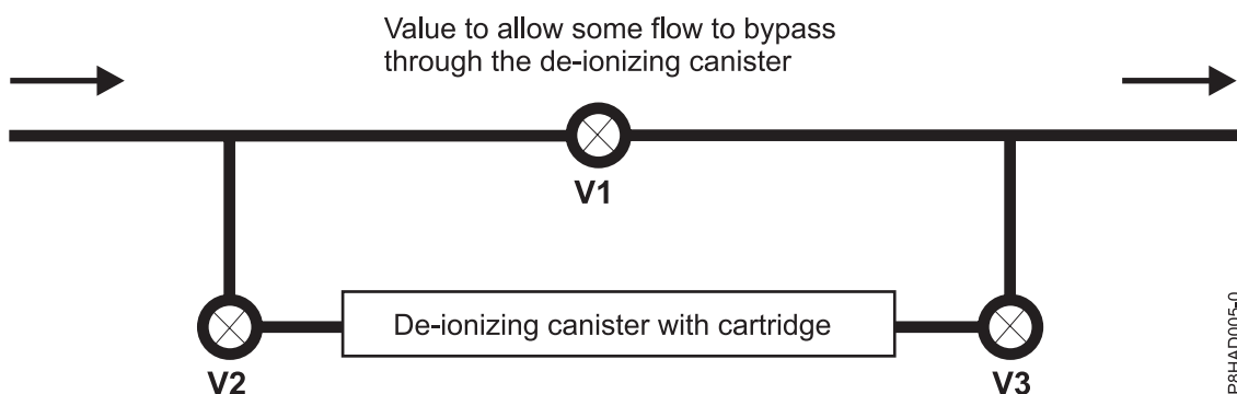
รูปที่ 88. กำจัดไอออนของน้ำโดยใช้กลไกการกำจัดไอออน ที่ติดตั้งในลูการระบายความร้อน
