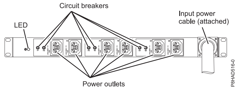
รูปที่ 62. HVDC PDU
