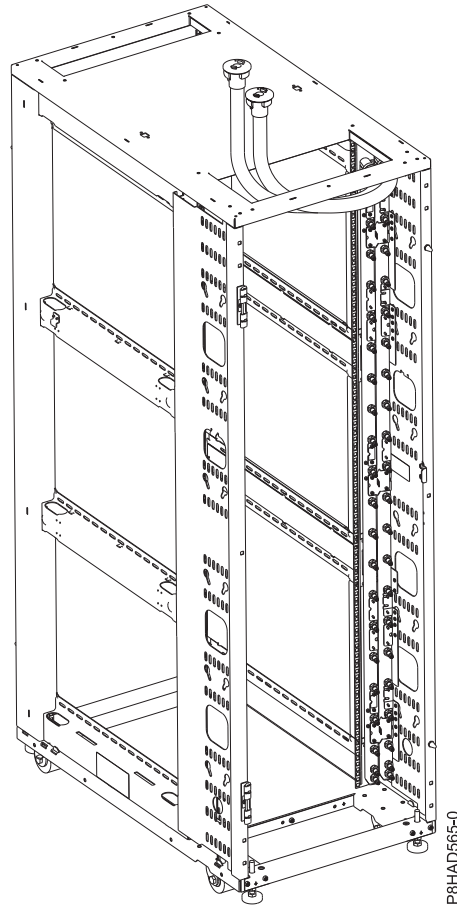
รูปที่ 40. ชั้นวางและท่อร่วมที่มีท่อจ่ายและท่อส่ง อยู่นอกชั้นวางด้านบน
