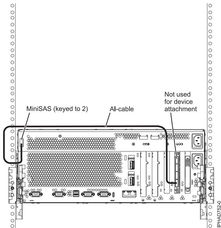
รูปที่ 77. อะแดปเตอร์ FC5904 หรือ FC5908 ที่เชื่อมต่อกับ ลินซ์ส่วนขยายดิสก์
