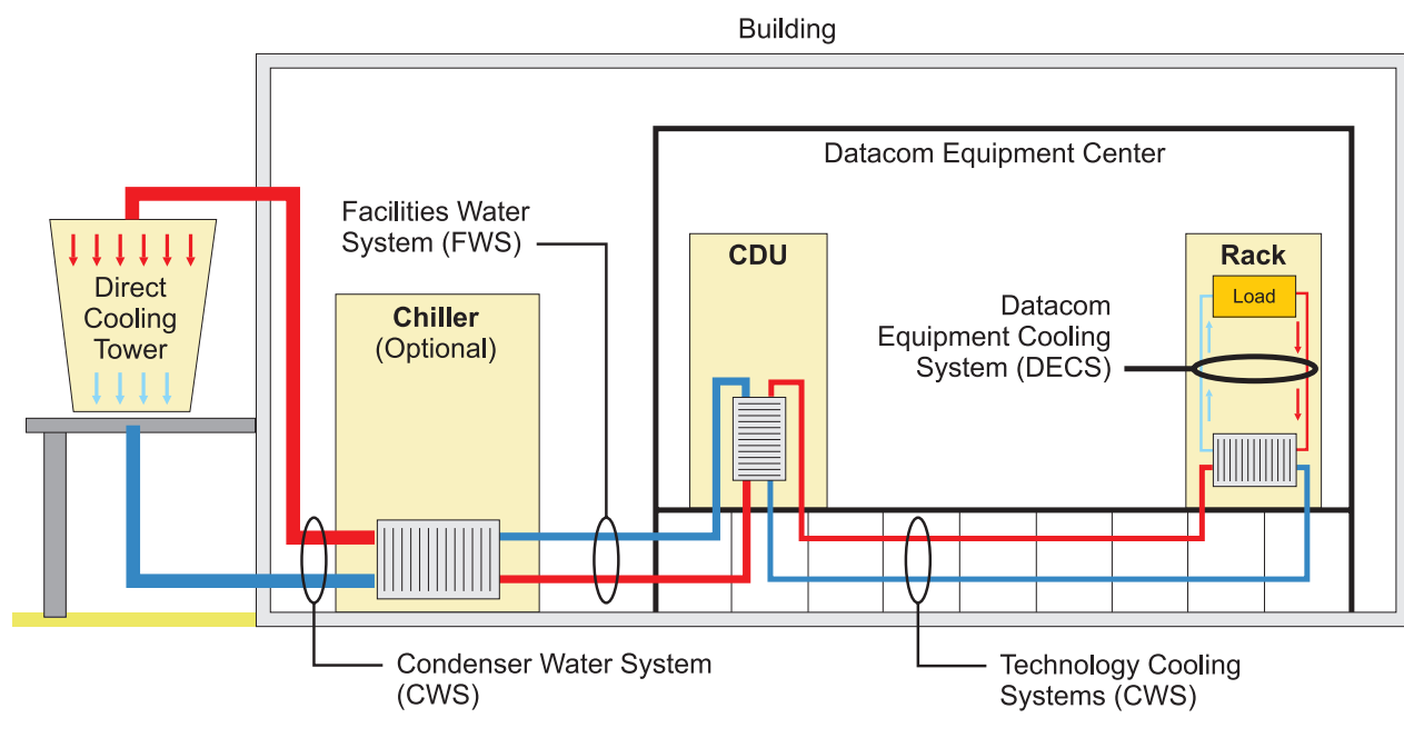
รูปที่ 87. ตัวอย่างของระบบการระบายความร้อน ของเหลวและลูบในศูนย์ข้อมูล
