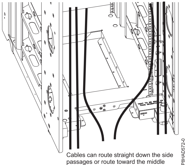
รูปที่ 50. การเดินสายใต้พื้น
