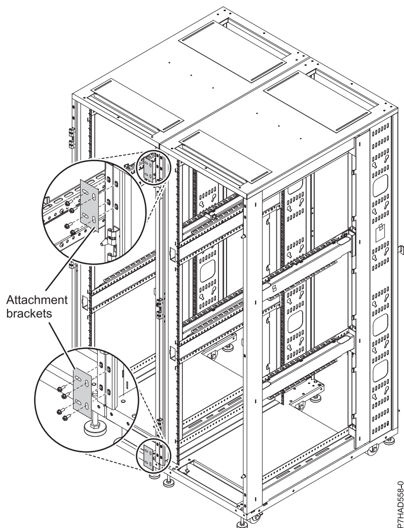
รูปที่ 36. กรอบยึด
