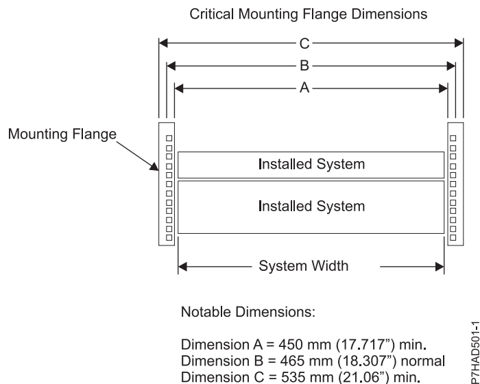
รูปที่ 56. มิติของขอบยึดที่สำคัญ
