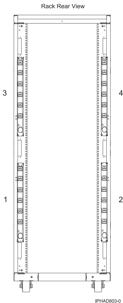
รูปที่ 59. ตำแหน่งในแนวตั้งของ Power distribution unit
