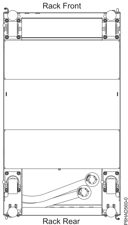
รูปที่ 45. ตำแหน่งทางออกของท่อด้านล่าง (เมื่อดูจากด้านล่าง)
