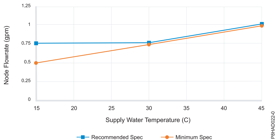
รูปที่ 2. อัตราโพล์น้ำที่ทำให้เย็นลงเทียบกับข้อกำหนดระบบน้ำ (ยูนิตมาตรฐาน)
