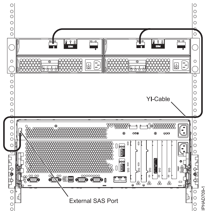
รูปที่ 75. จากพอร์ตของอะแดปเตอร์ SAS ภายนอกของระบบไปยังลิ้นชักส่วนขยายดิสก์
