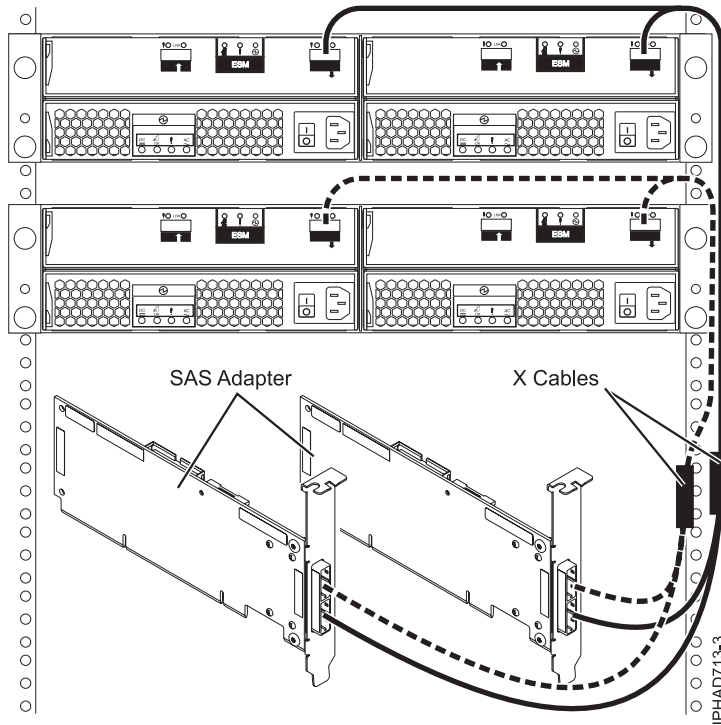
รูปที่ 79. จากอะแดปเตอร์ SAS RAID สองตัวไปยังลิ้นชัก ส่วนขยายดิสก์สองลิ้นชักในคอนฟิกรูเรชั่นแบบ multi-initiator HA RAID
