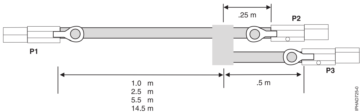
รูปที่ 67. ความยาวชุดสายเคเบิล SAS YO ภายนอก
