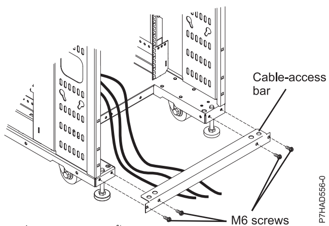
รูปที่ 28. แถบสำหรับเข้าถึงสายเคเบิล
