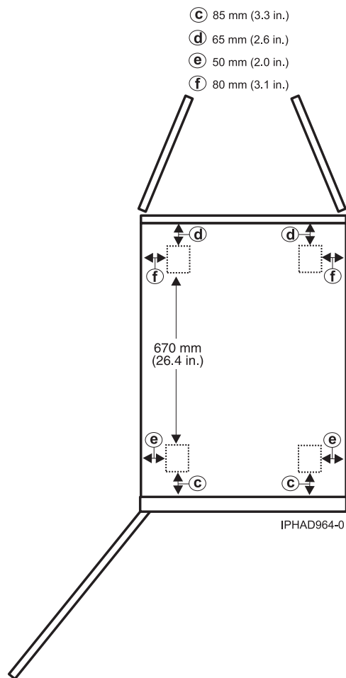
รูปที่ 20. ตำแหน่งลูกกลิ้งของโมเดล 0555 และ 7014-S25
