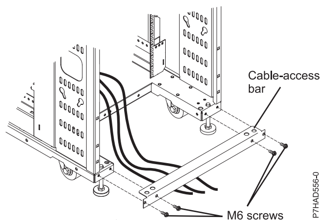
รูปที่ 28. แปกสำหรับเข้าถึงสายเคเบิล
