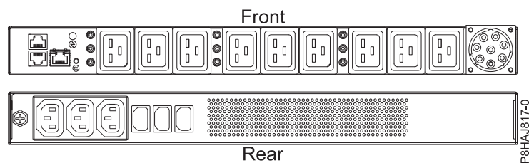
รูปที่ 48. PDU สำหรับระบบ 8408-44E
