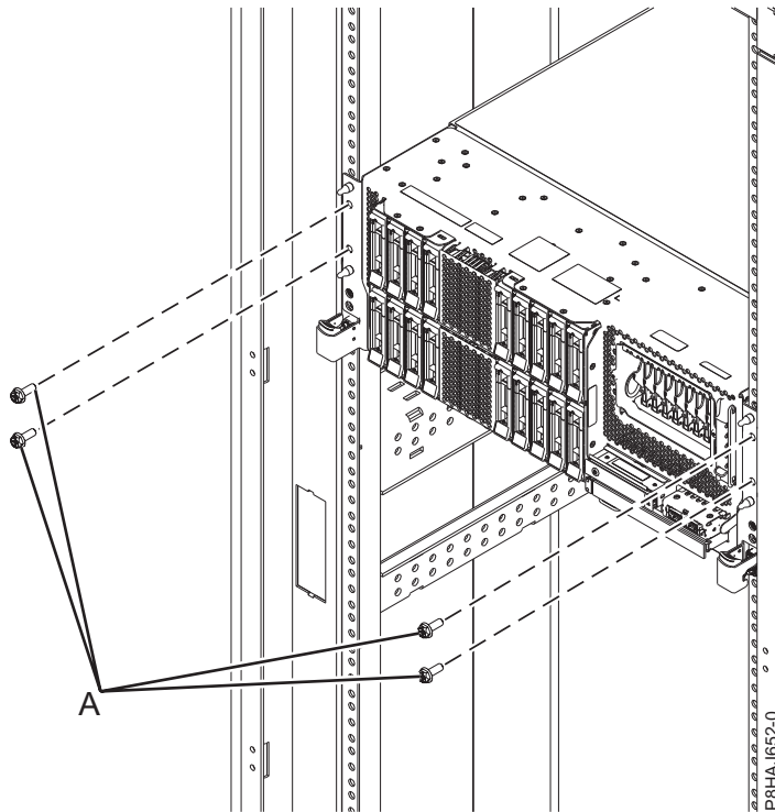
รูปที่ 43. การถอดฝาครอบด้านหน้า
