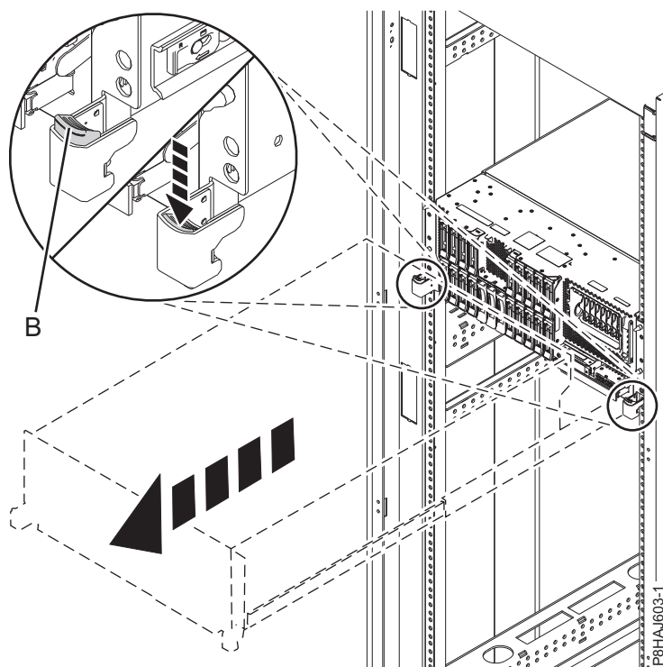
รูปที่ 44. การปลดแลตซ์ด้านข้าง
