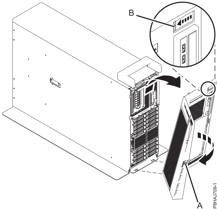
รูปที่ 22. การถอดฝาครอบด้านหน้า
