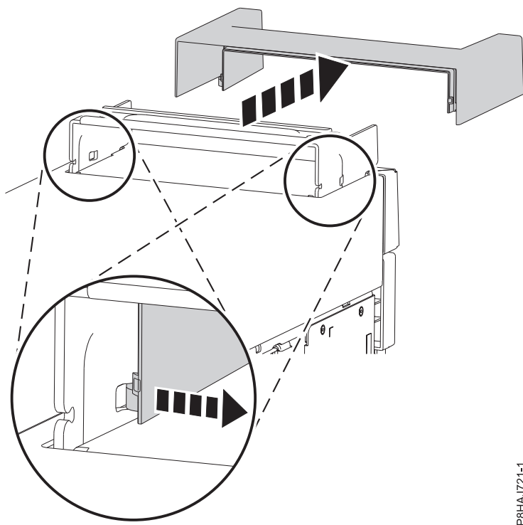
รูปที่ 24. การถอดฝาครอบด้านซ้ายออกจากระบบสแตนด์อะโลน 8286-41A
