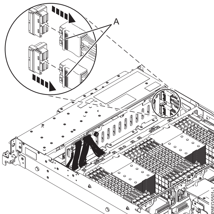
รูปที่ 1. การถอดสายเคเบิล SAS ด้านหน้าออกจากด้านหลังดิสก์ไดรฟ์
