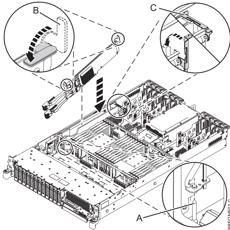
รูปที่ 13. การเปลี่ยนอะแดปเตอร์ภายใน PCIe3 x8 SAS RAID ขนาด 6 Gb
