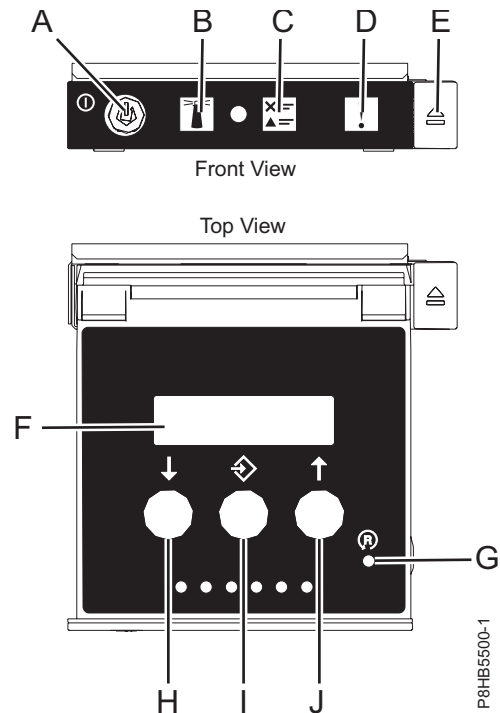
รูปที่ 19. แผงควบคุม
