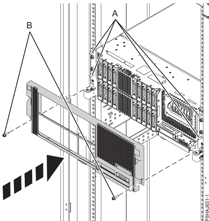
รูปที่ 28. การติดตั้งฝาครอบด้านหน้า
