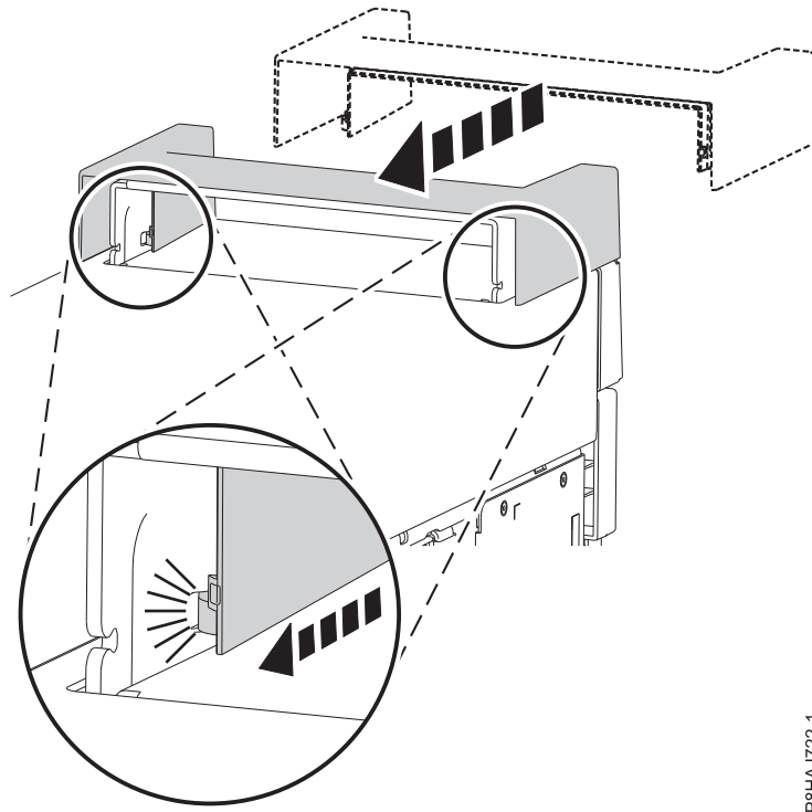
รูปที่ 31. การยึดฝาครอบด้านข้างในระบบสแตนด์อะโลน 8286-41A
