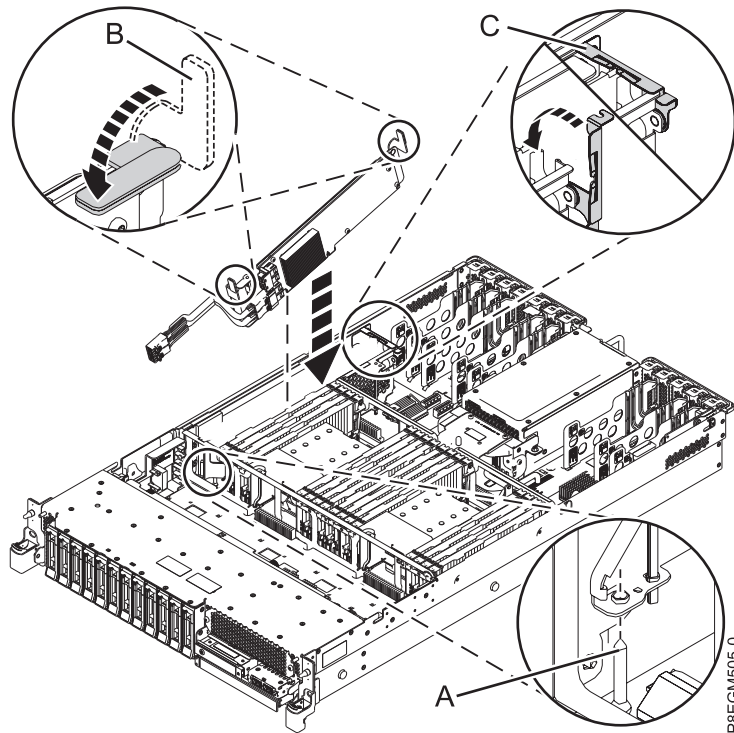
รูปที่ 5. การติดตั้งอะแดปเตอร์ภายใน PCIe3x8 SAS RAID ขนาด 6 Gb ในช่องเสียบ P1-C15
