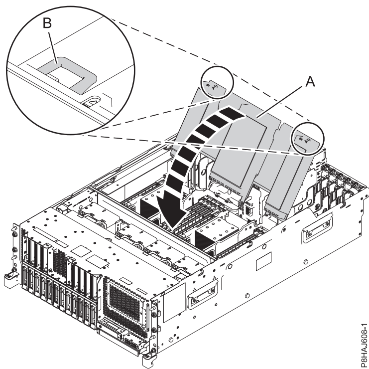
รูปที่ 40. การเปิด ตัวไลแวนอากาศ
