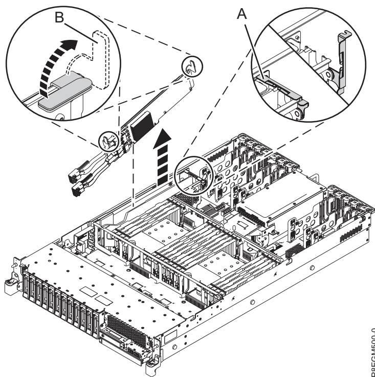
รูปที่ 12. การถอดอะแดปเตอร์ภายใน SAS RAID
