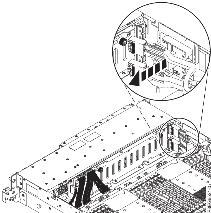
รูปที่ 2. การถอดสายเคเบิล SAS ด้านหน้าออกจากบล็อกนำทาง
