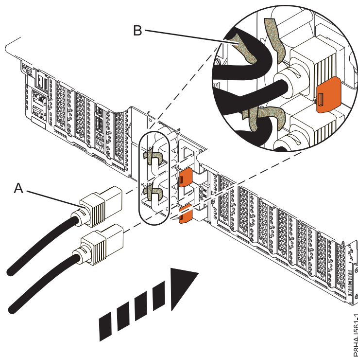
รูปที่ 56. การเชื่อมต่อสายไฟเข้ากับระบบ 5148-21L, 5148-22L, 8247-21L, 8247-22L, 8284-21A, or 8284-22A
