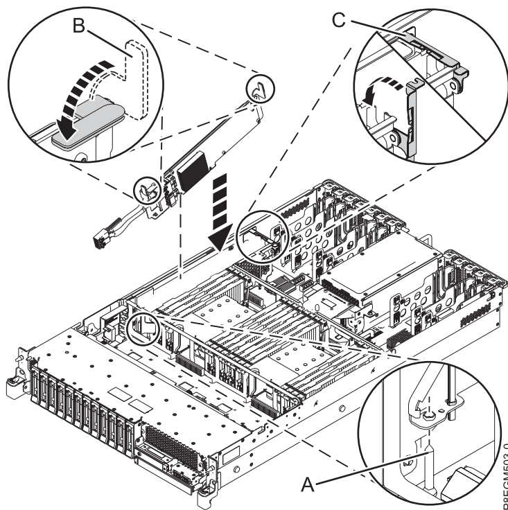
รูปที่ 4. การเปลี่ยน อะแดปเตอร์ภายใน PCIe3x8 SAS RAID ขนาด 6 Gb ในช่องเสียบ P1-C14
