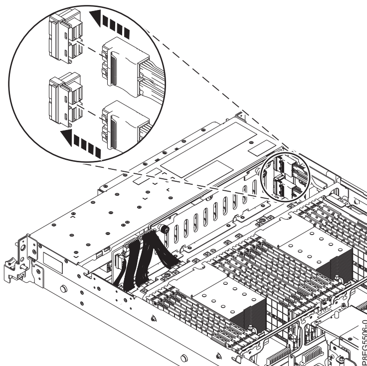
รูปที่ 15. การเสียบสายเคเบิล SAS ด้านหน้าที่ด้านหลัง ดิสก์ไดรฟ์อีกครั้ง
