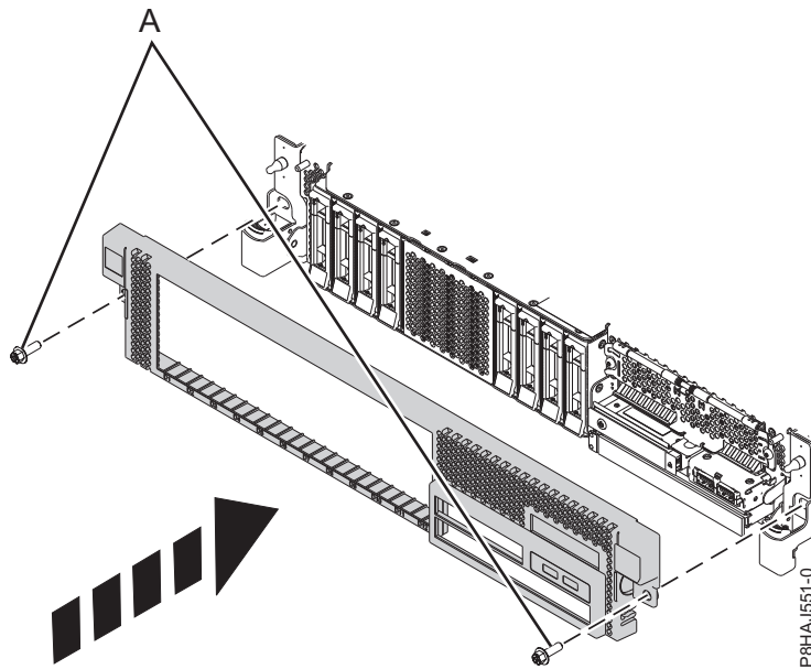
รูปที่ 27. การติดตั้งฝาครอบด้านหน้า
