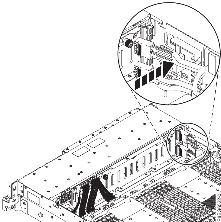
รูปที่ 14. การวางสายเคเบิล SAS ด้านหลังในบล็อกนำทาง
