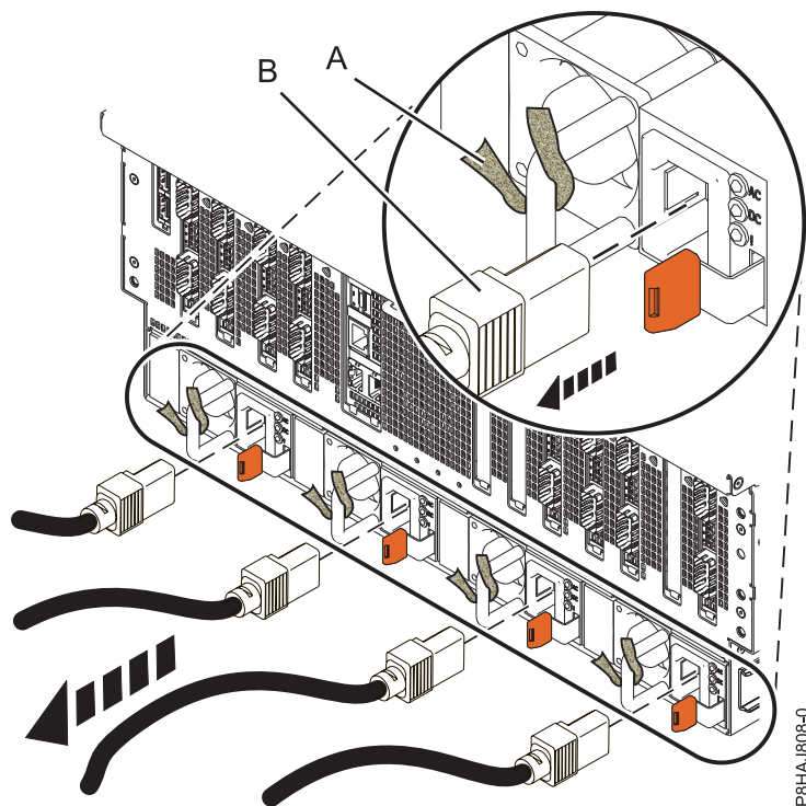
รูปที่ 51. การถอดสายไฟออกจากระบบ 8408-44E หรือ 8408-E8E
