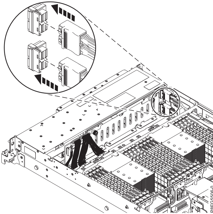
รูปที่ 7. การเชื่อมต่อสายเคเบิล SAS ด้านหน้าที่ด้านหลังดิสก์ไดรฟ์อีกครั้ง
