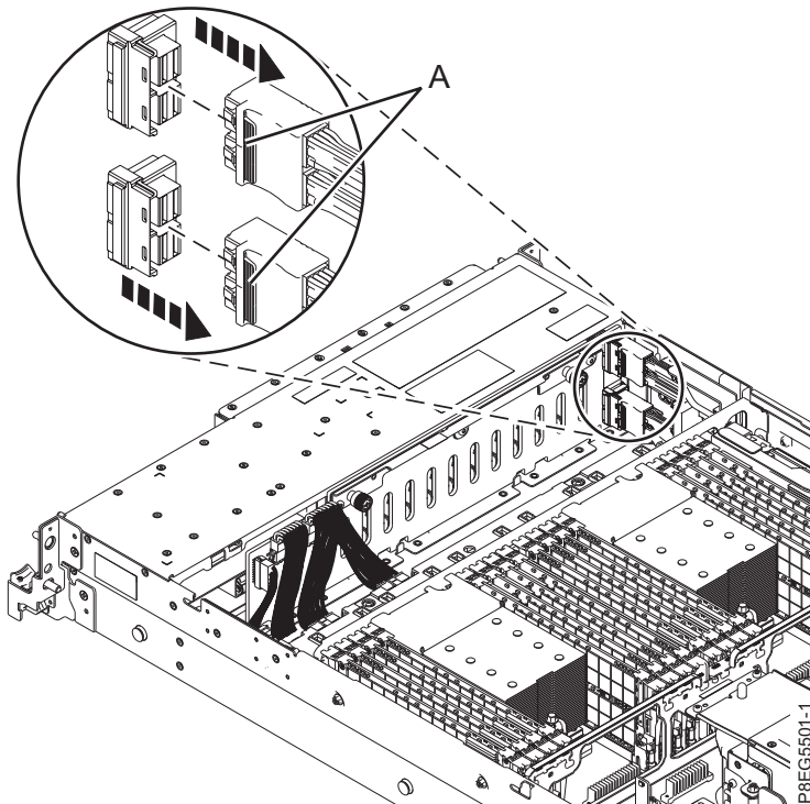
รูปที่ 10. การถอดสายเคเบิล SAS ด้านหน้าออกจาก ด้านหลังดิสก์ไดรฟ์
