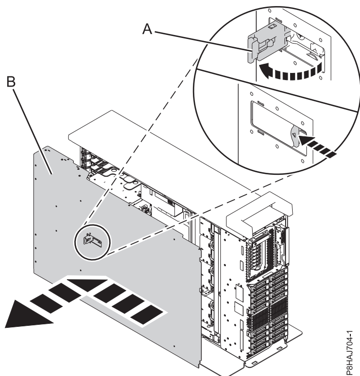
รูปที่ 36. การถอดฝาครอบการเข้าถึงเซิร์ฟเวอร์
