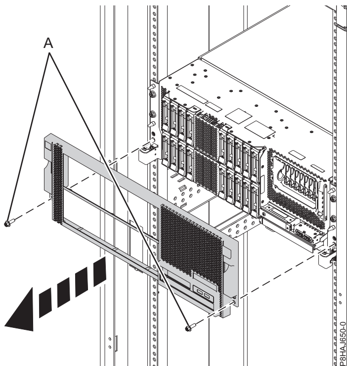
รูปที่ 21. การถอดฝาครอบด้านหน้า
