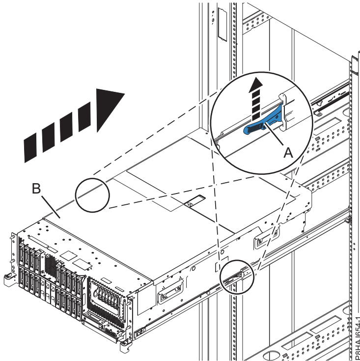
รูปที่ 45. การจัดตำแหน่งระบบในตำแหน่งการทำงาน
