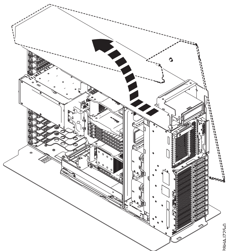
รูปที่ 26. การถอดฝาครอบด้านข้าง 8286-41A
