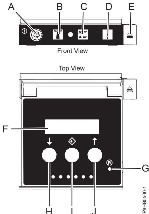
รูปที่ 18. คอนโทรลพาเนล LEDs
