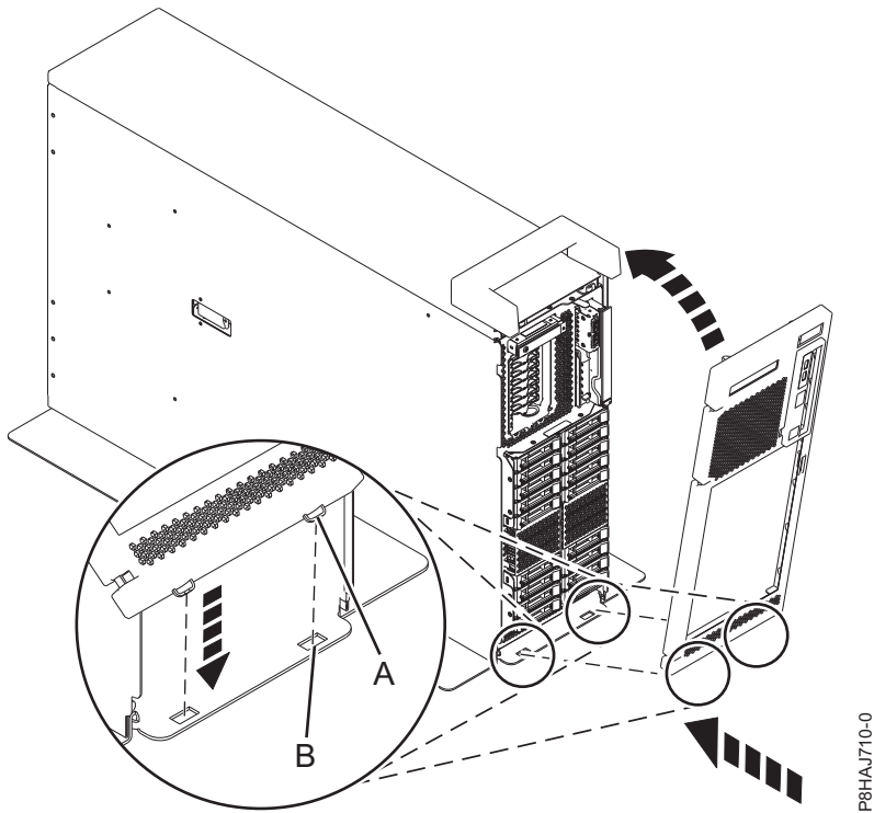
รูปที่ 29. ติดตั้งฝาครอบด้านหน้า
