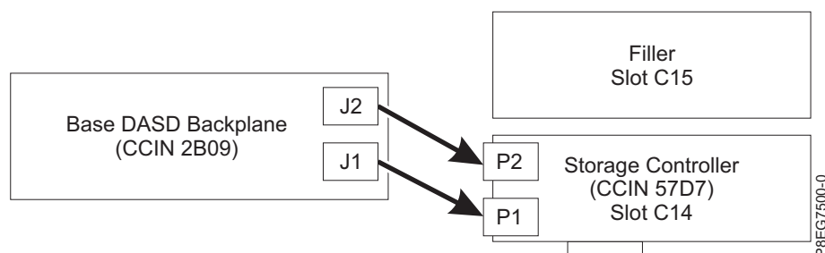
รูปที่ 16. การเสียบสายเคเบิล SAS อีกครั้งในกำหนดคอนฟิกที่เก็บพื้นฐาน
