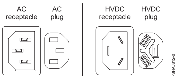
รูปที่ 52. ตัวเชื่อมต่อ AC และ HVDC
