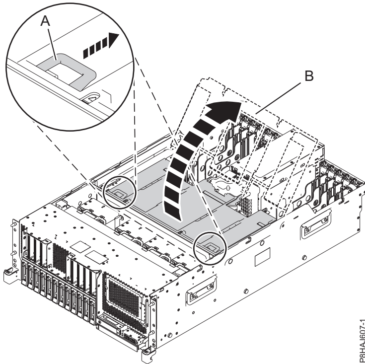
รูปที่ 39. การเปิดตัวไลเวยนอากาศ
