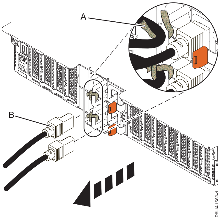
รูปที่ 50. การถอดสายไฟออกจากระบบ 5148-21L, 5148-22L, 8247-21L, 8247-22L, 8284-21A, or 8284-22A
