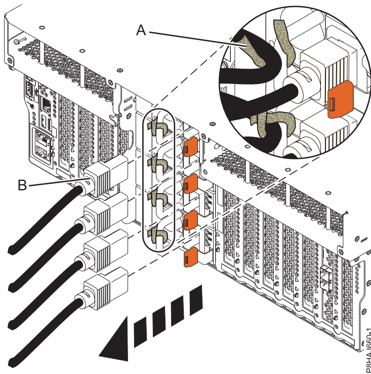
รูปที่ 49. การถอดสายไฟออกจากระบบ 8247-42L, 8286-41A หรือ 8286-42A
