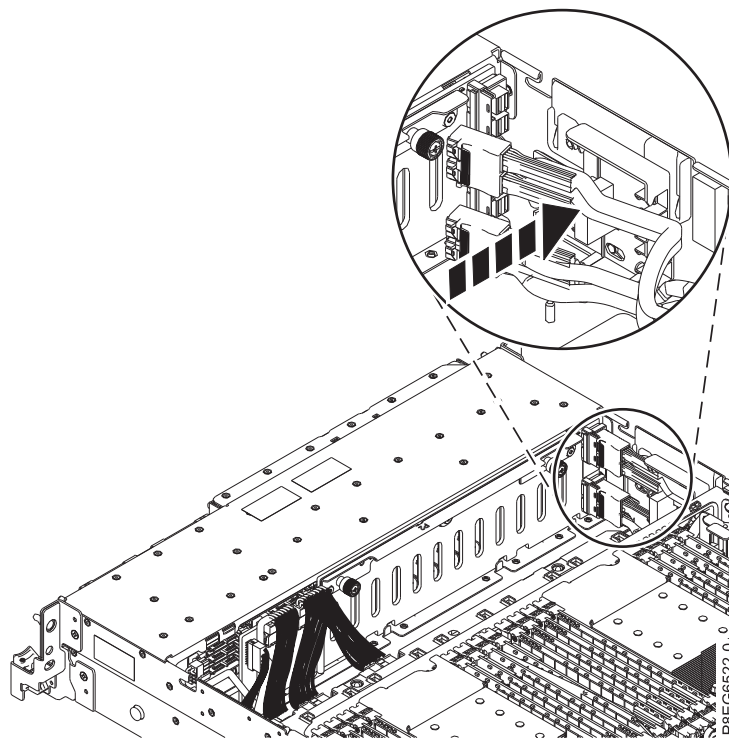
รูปที่ 6. การจัดวางสายเคเบิล SAS ด้านหน้า
