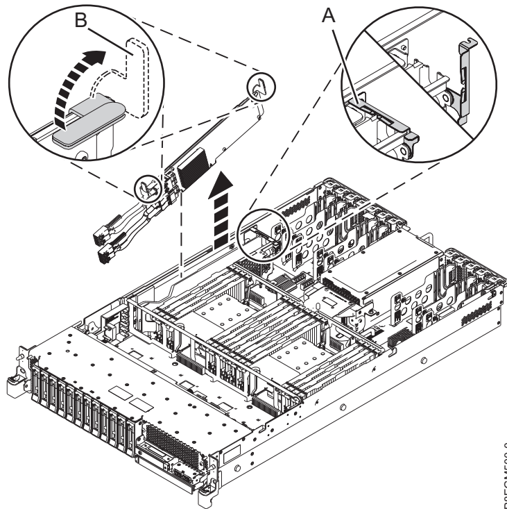
รูปที่ 3. การถอดอะแดปเตอร์ภายใน SAS RAID ในช่องเสียบ P1-C14
