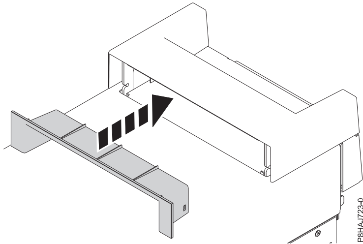
รูปที่ 32. การใส่ชิ้นส่วนภายในฝาครอบด้ามยึดบนระบบสแตนด์เอโลน 8286-41A
