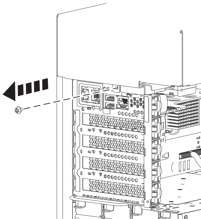
รูปที่ 25. การถอดสกรูออกจากฝาครอบด้านข้าง 8286-41A
