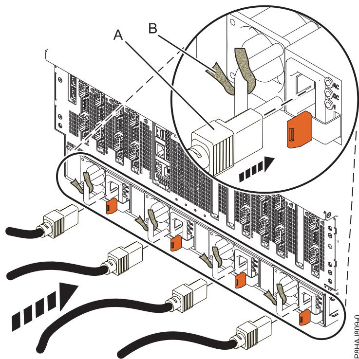
รูปที่ 57. การเชื่อมต่อสายไฟเข้ากับ ระบบ 8408-44E หรือ 8408-E8E
