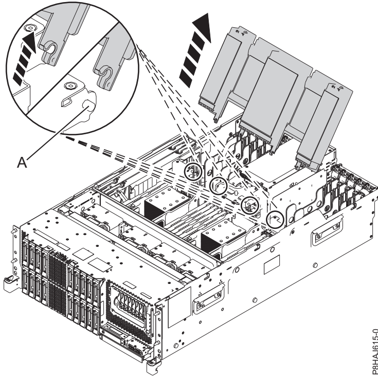
รูปที่ 41. การถอดตัวไหลเวียนอากาศ
