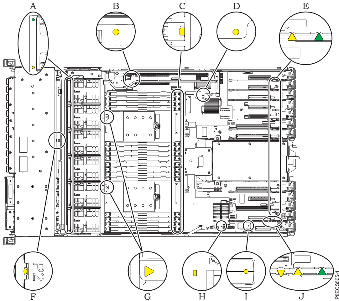
รูปที่ 9. LED ตัวบ่งชี้เซอวิส
