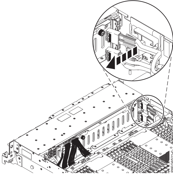
รูปที่ 11. การถอดสายเคเบิล SAS ด้านหน้าออกจากบล็อกนำทาง
