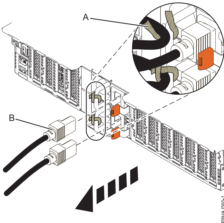
รูปที่ 53. การถอดสายไฟออกจากระบบ 5148-21L, 5148-22L, 8247-21L, 8247-22L, 8284-21A, or 8284-22A
