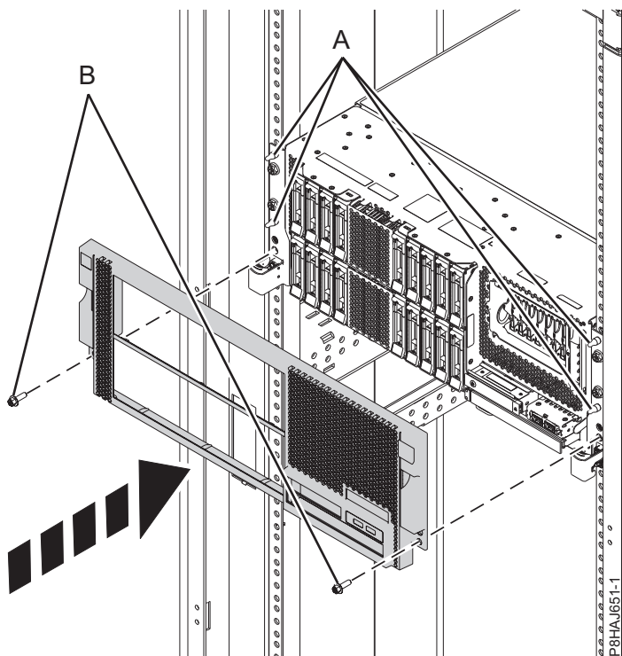
รูปที่ 31. การติดตั้งฝาครอบด้านหน้า
