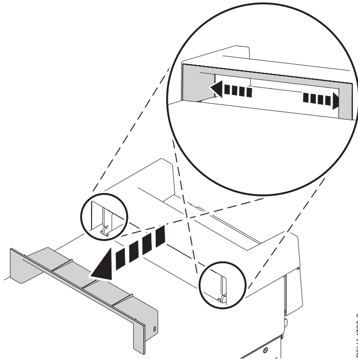
รูปที่ 26. การถอดชิ้นส่วนฝาครอบด้ามยึดบนระบบสแตนด์อะโลน 8286-41A
