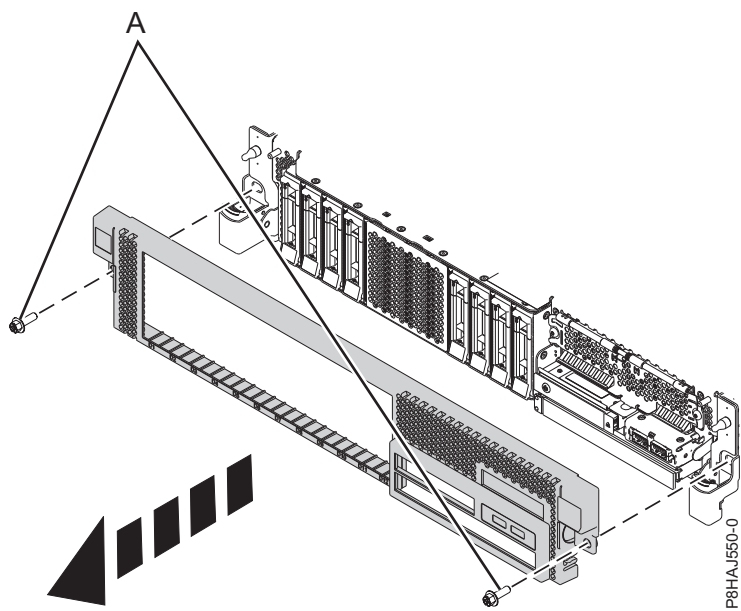
รูปที่ 23. การถอดฝาครอบด้านหน้า
