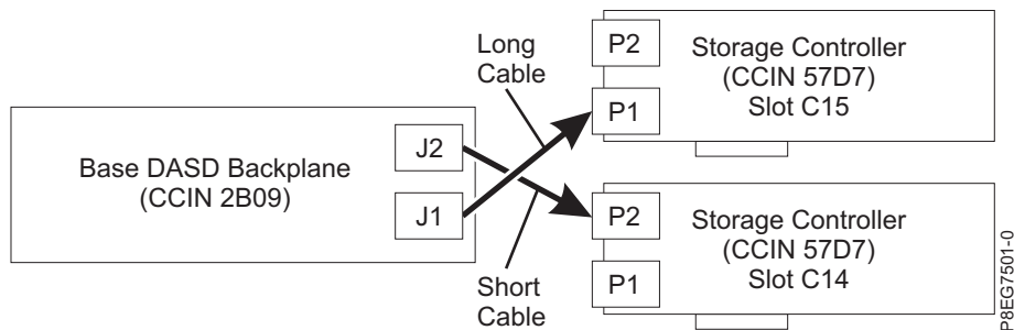
รูปที่ 8. การเชื่อมต่อสายเคเบิลสายเคเบิล SAS อีกครั้งในการกำหนดคอนฟิกการแบ่งดิสก์
