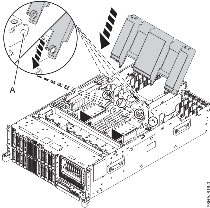
รูปที่ 45. การเปลี่ยนตัวไหลเวียนอากาศ
