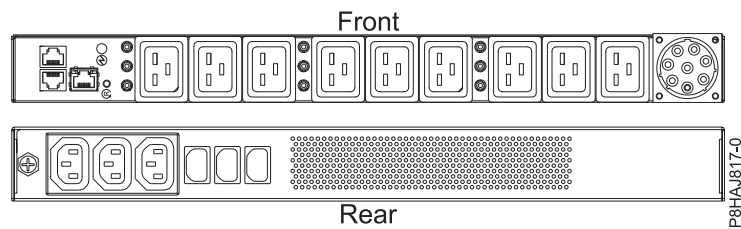
รูปที่ 51. PDU สำหรับระบบ 8408-44E
