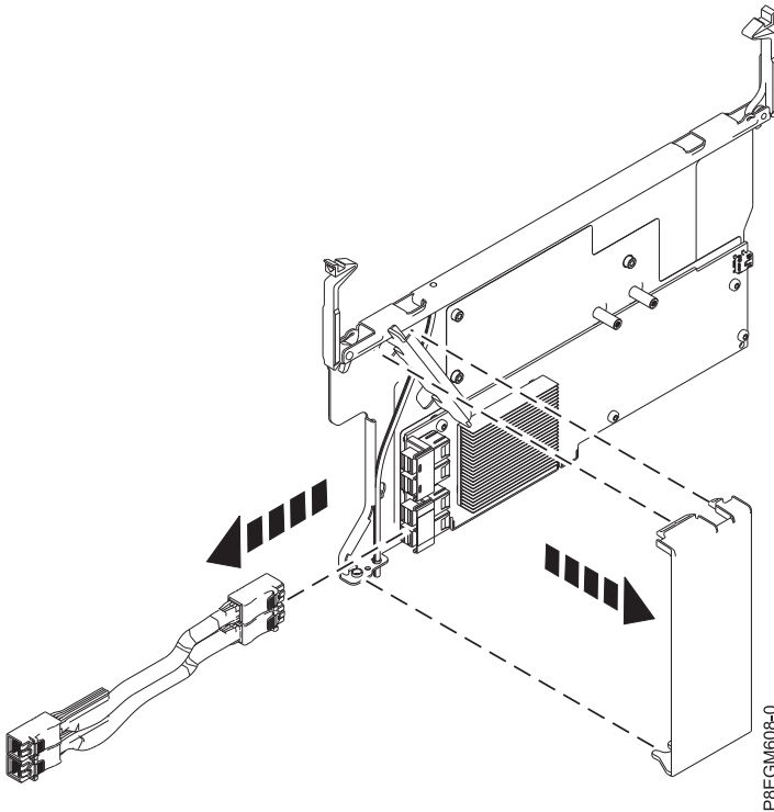
รูปที่ 14. การถอดฝาครอบ การไหลเวียนอากาศ
