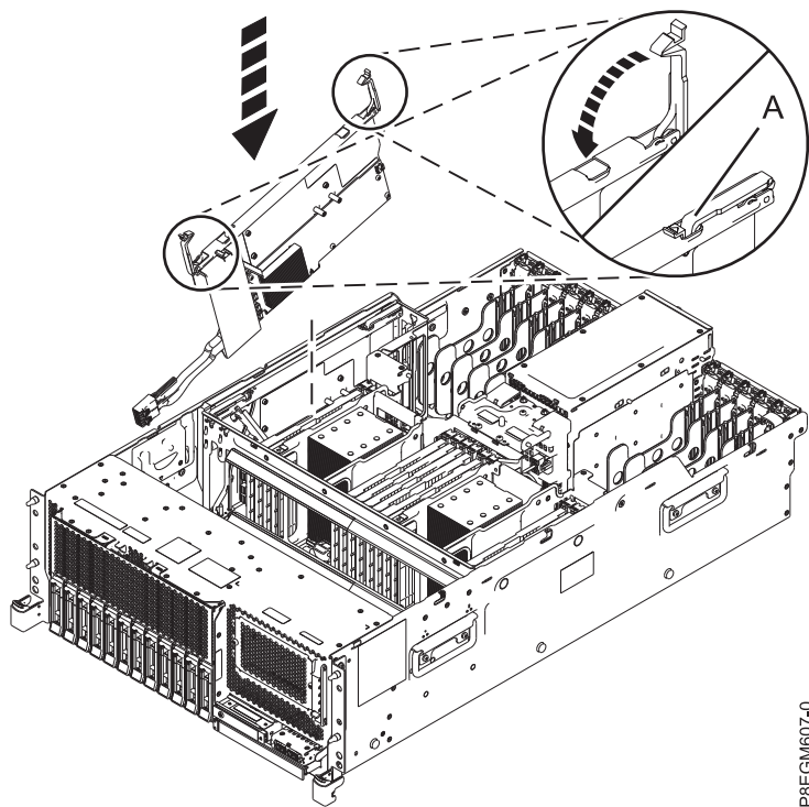
รูปที่ 6. การติดตั้งอะแดปเตอร์ภายใน SAS RAID ในช่องเสียบ P1-C15
