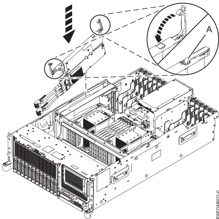
รูปที่ 16. การติดตั้งอะแดปเตอร์ภายในภายใน SAS RAID
