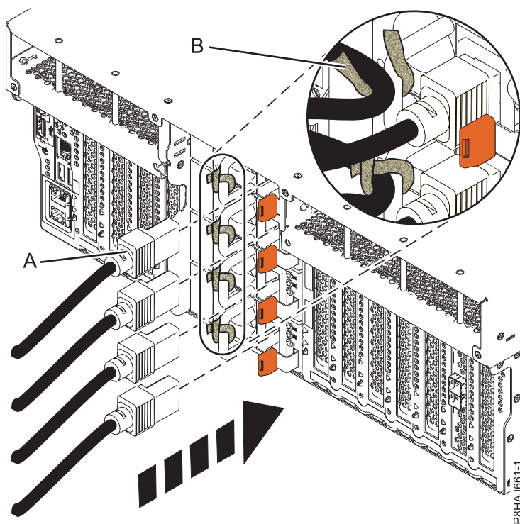
รูปที่ 58. การเชื่อมต่อสายไฟเข้ากับ ระบบ 8247-42L, 8286-41A หรือ 8286-42A
