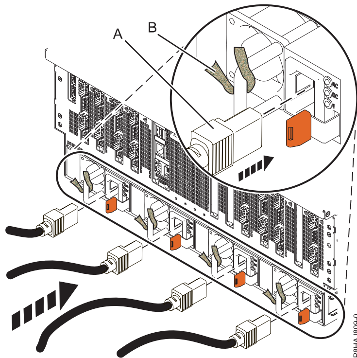
รูปที่ 60. การเชื่อมต่อสายไฟเข้ากับ ระบบ 8408-44E หรือ 8408-E8E
