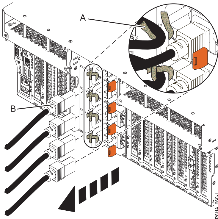
รูปที่ 52. การถอดสายไฟออกจากระบบ 8247-42L, 8286-41A หรือ 8286-42A
