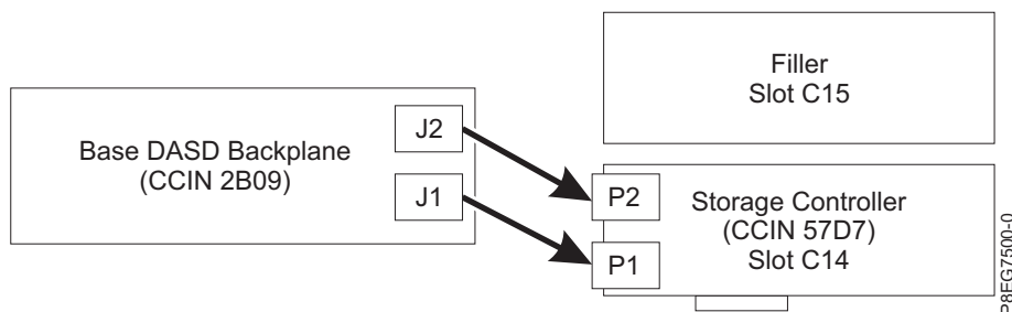
รูปที่ 18. การเสียบสายเคเบิล SAS อีกครั้งในกำหนดคอนฟิกที่เก็บพื้นฐาน
