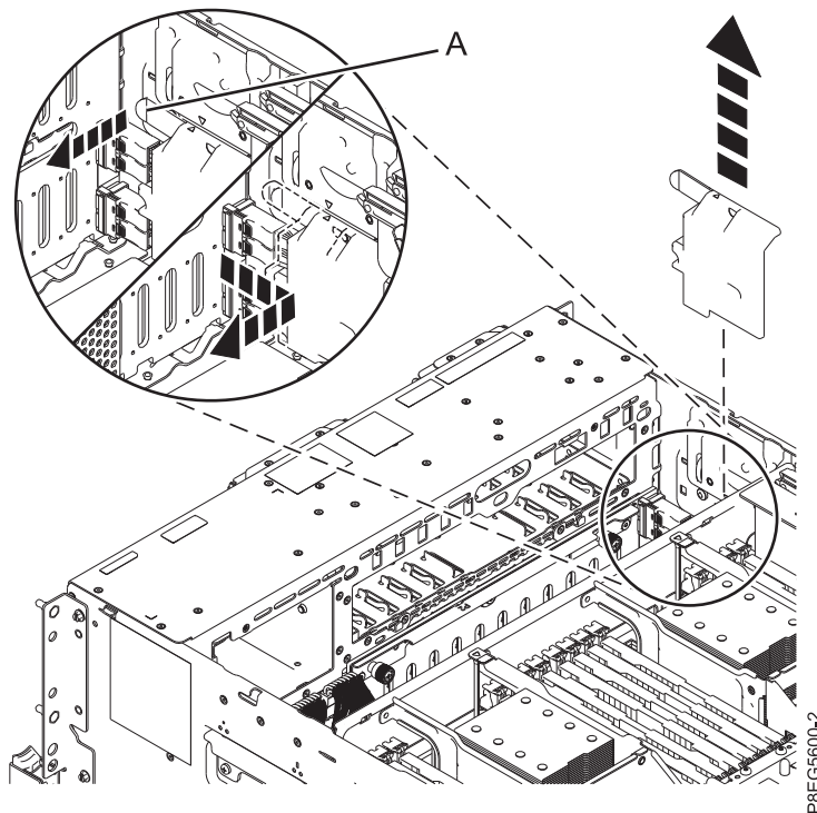
รูปที่ 11. การถอดฝาครอบสายเคเบิล SAS
