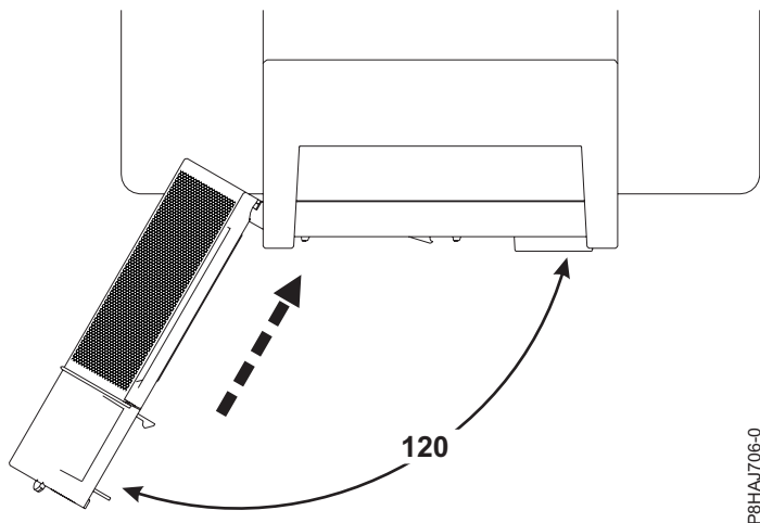
รูปที่ 33. การหมุนฝาครอบด้านหน้า
