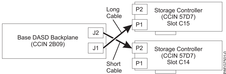
รูปที่ 19. การเชื่อมต่อสาย SAS อีกครั้งในคอนฟิกร์ระบบแบบแยก
