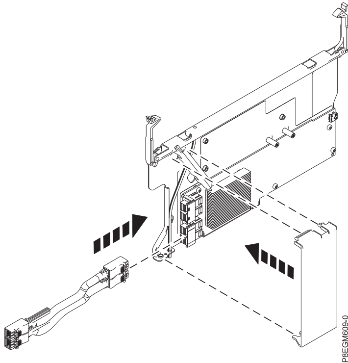
รูปที่ 5. การติดตั้ง ฝาครอบการไหลเวียนอากาศ
