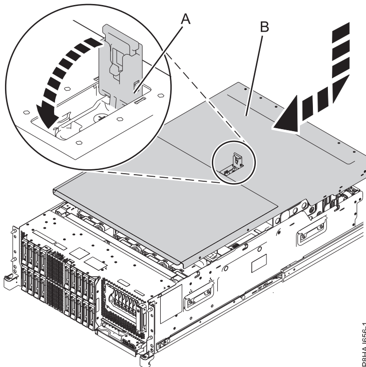
รูปที่ 40. การติดตั้ง ฝาครอบการเข้าถึงเซอว์วิส
