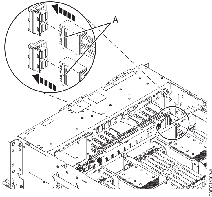
รูปที่ 17. การเชื่อมต่อสายเคเบิล SAS ด้านหน้าอีกครั้ง
