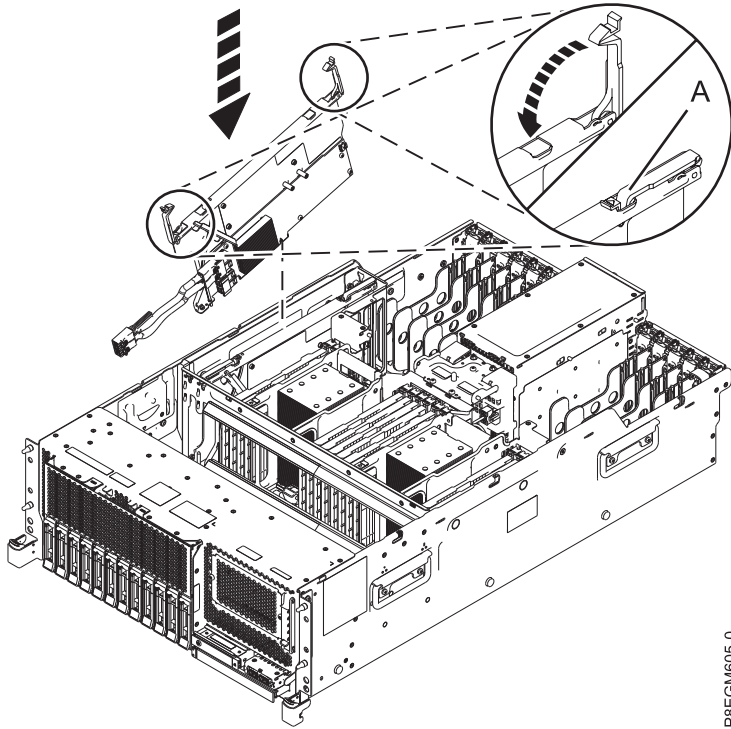
รูปที่ 4. การติดตั้งอะแดปเตอร์ภายใน SAS RAID ในช่องเสียบ slot P1-C14
