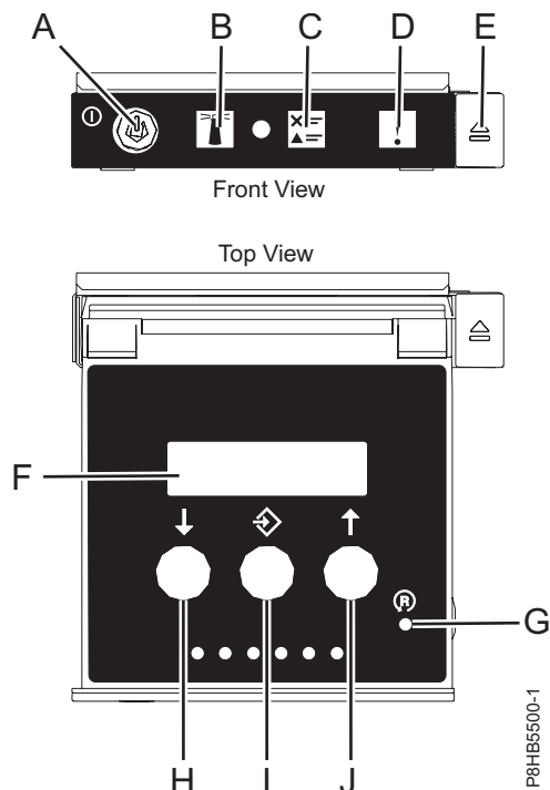
รูปที่ 21. คอนโทรลพาเนล LEDs
