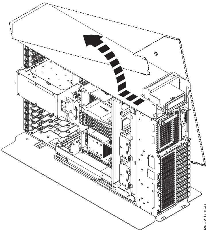
รูปที่ 29. การถอดฝาครอบด้านข้าง 8286-41A
