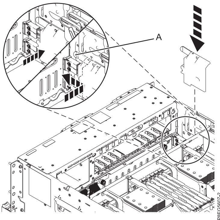
รูปที่ 20. การเปลี่ยนฝาครอบสายเคเบิล SAS
