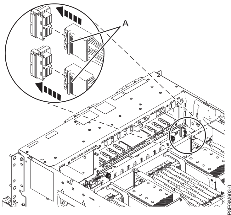
รูปที่ 7. การเชื่อมต่อสายเคเบิล SAS ด้านหน้าที่ด้านหลังดิสก์ไดรฟ์
