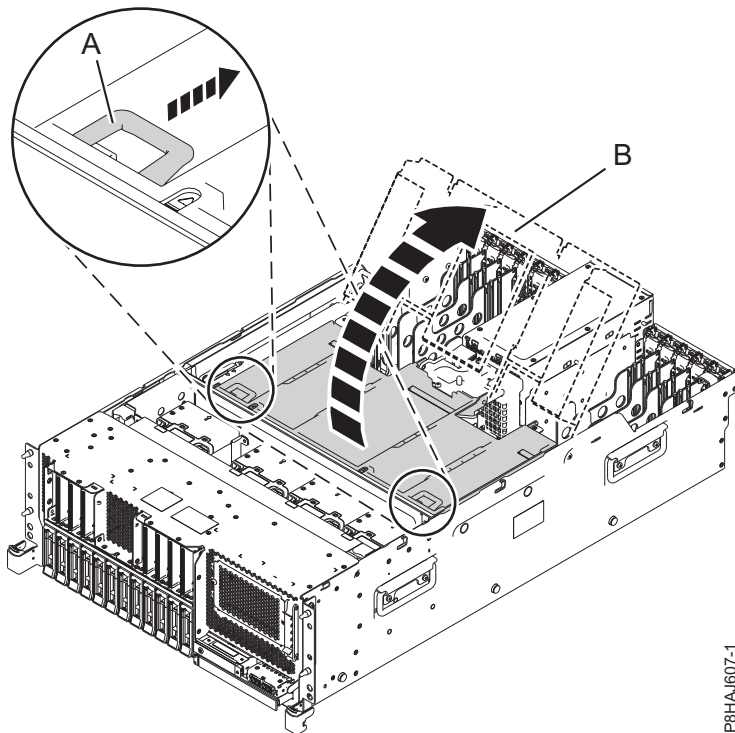
รูปที่ 42. การเปิดตัวโหลเวียนอากาศ
