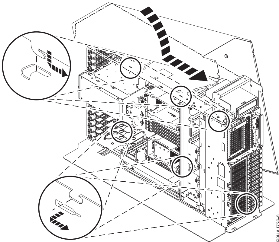
รูปที่ 36. การติดตั้งฝาครอบด้านข้าง 8286-41A
