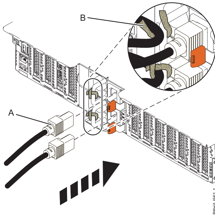
รูปที่ 59. การเชื่อมต่อสายไฟเข้ากับระบบ 5148-21L, 5148-22L, 8247-21L, 8247-22L, 8284-21A, or 8284-22A
