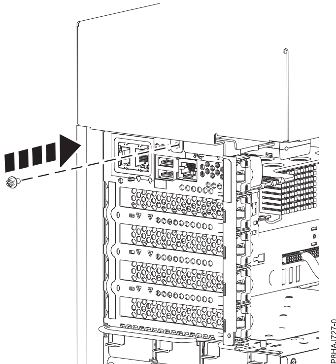
รูปที่ 37. การติดตั้งสกรูของฝาครอบด้านข้าง 8286-41A
