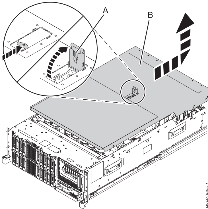
รูปที่ 38. การถอดฝาครอบการเข้าถึงเซิร์ฟเวอร์
