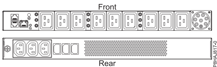
รูปที่ 57. PDU สำหรับระบบ 8408-44E
