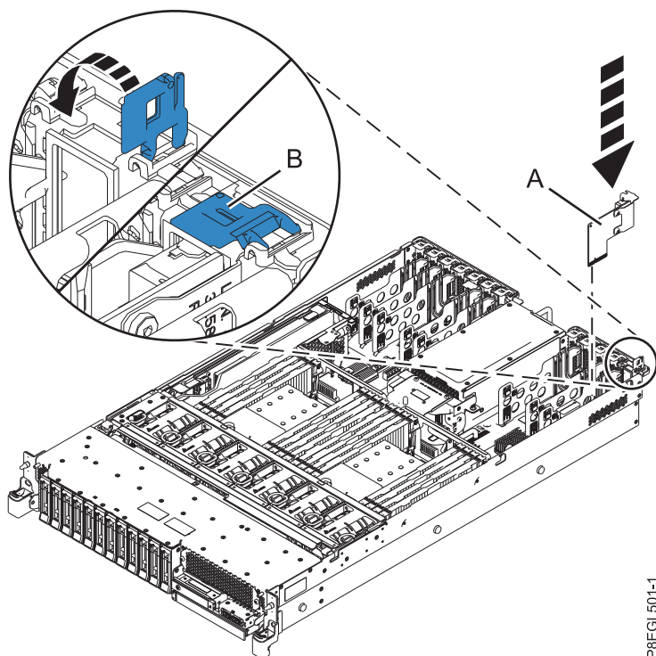
รูปที่ 2. การเปลี่ยน การ์ด I/O ระบบ ใน ระบบที่ติดตั้งบนชั้นวาง
