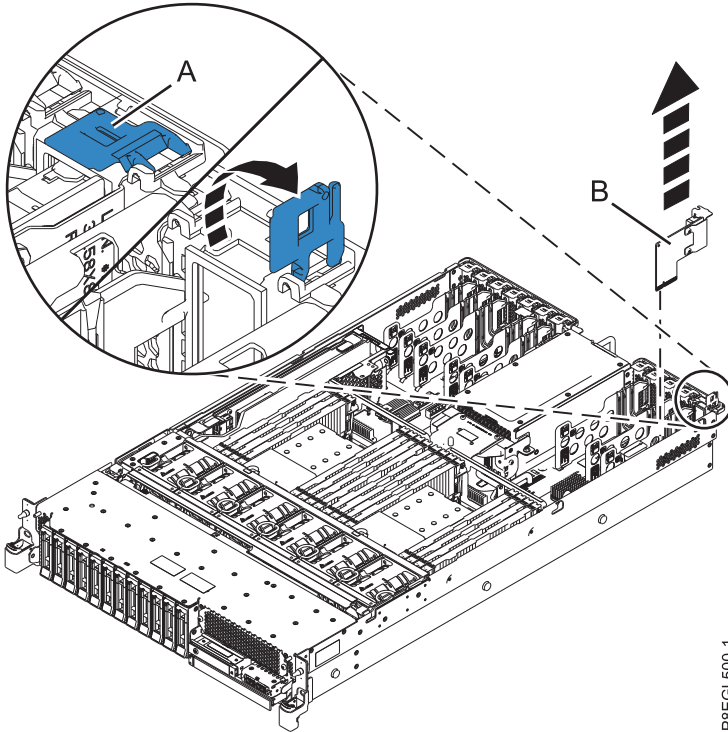
รูปที่ 1. การถอด การ์ด I/O ระบบ ออกจาก ระบบที่ติดตั้งบนแผง
