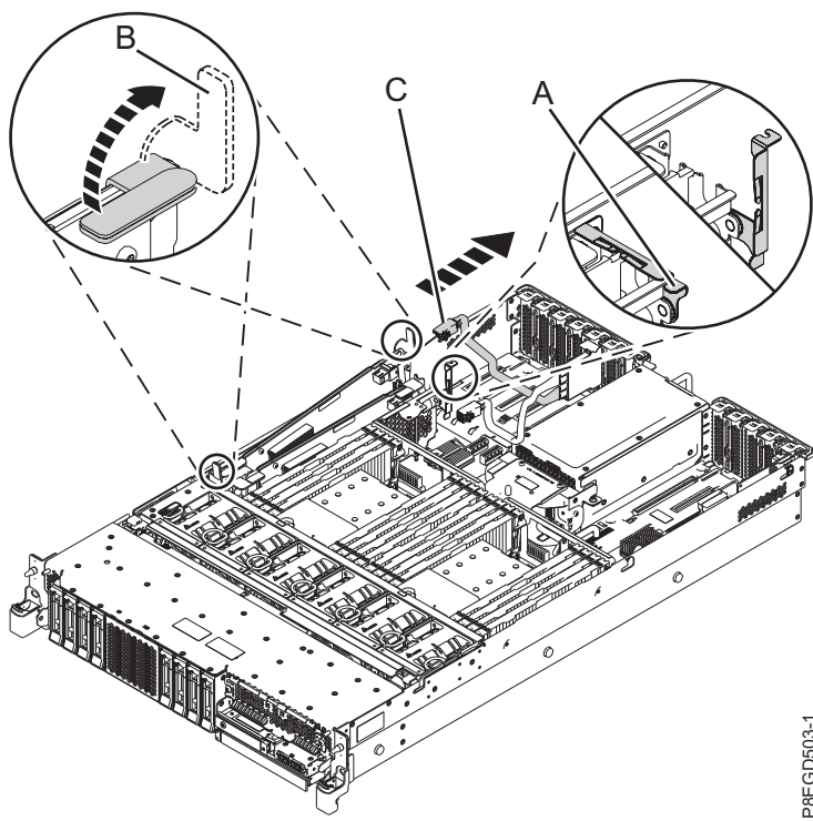
รูปที่ 3. การถอดสายเคเบิล SAS ด้านหลังออกจากอะแดปเตอร์ภายใน SAS RAID ในตำแหน่งช่องเสียบ P1-C14
