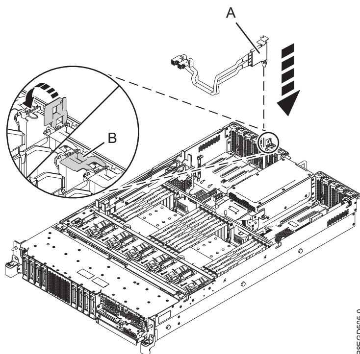
รูปที่ 5. การติดตั้งสายเคเบิล SAS ด้านหลัง
