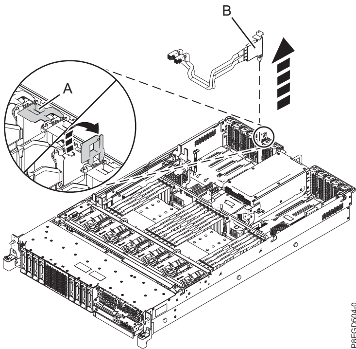
รูปที่ 4. การถอดสายเคเบิล SAS ด้านหลัง
