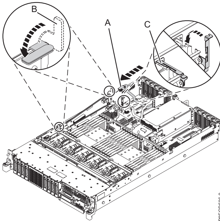
รูปที่ 6. การเปลี่ยนสายเคเบิล SAS ด้านล่างข้างหลังที่ตำแหน่งช่องเสียบ P1-C14
