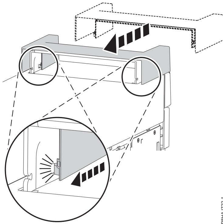
รูปที่ 23. การยึดฝาครอบด้านข้างในระบบ 8286-41A สแตนด์อะโลน
