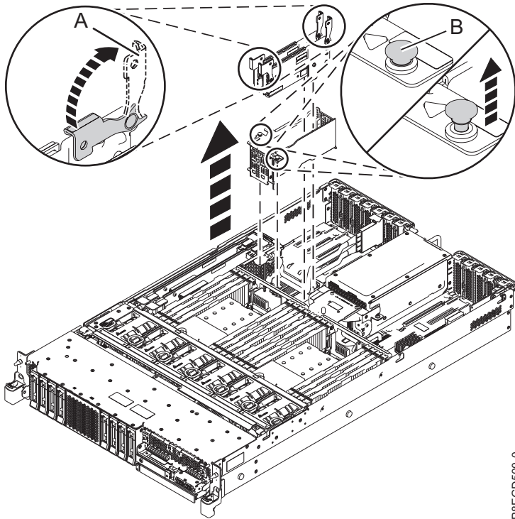
รูปที่ 1. การถอดการ์ดโมดูลไฟสำรอง และโครง
