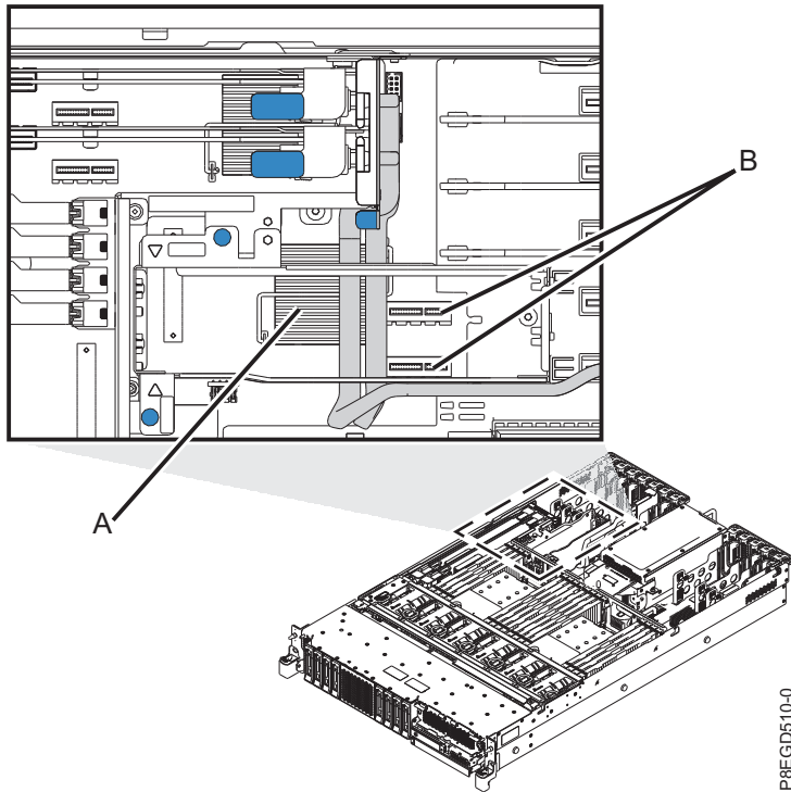
รูปที่ 8. การจัดเส้นทางสายเคเบิล SAS ด้านหลัง
