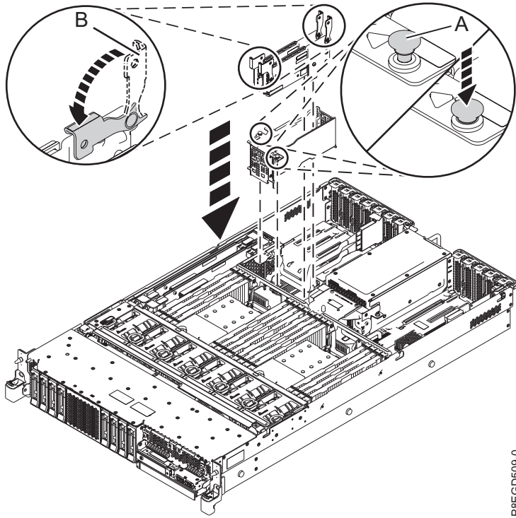
รูปที่ 9. การเปลี่ยนกล่องโมดูลไฟฟ้า
