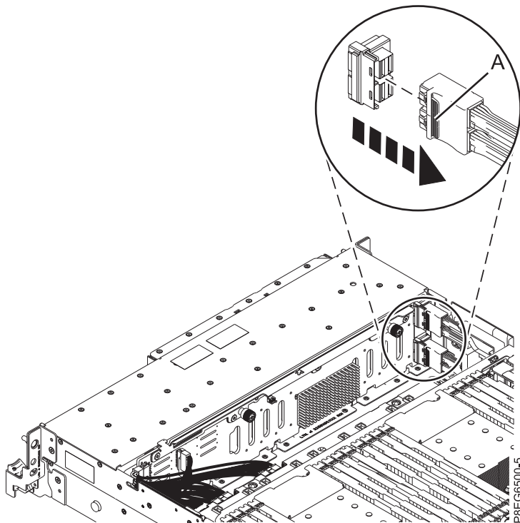
รูปที่ 2. การถอดสายเคเบิล SAS ออกจากด้านหลังดิสก์ไดรฟ์อีกครั้ง
