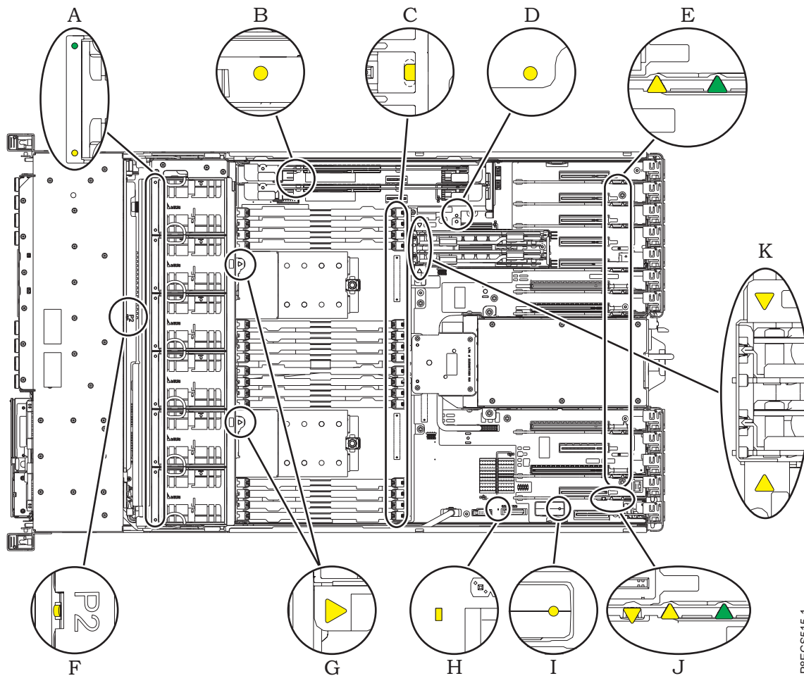
รูปที่ 1. LEDs ตัวบ่งชี้การบริการ
