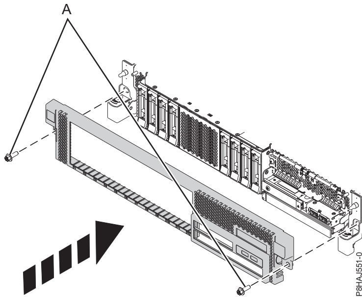
รูปที่ 20. การติดตั้งฝาครอบด้านหน้า
