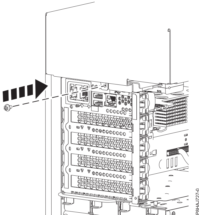
รูปที่ 27. การติดตั้งสกรูฝาครอบด้านข้าง 8286-41A
