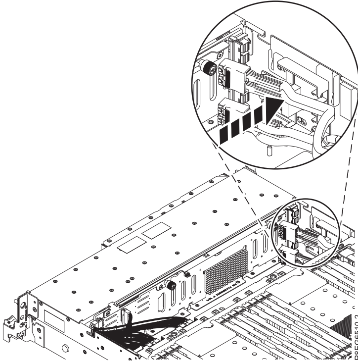
รูปที่ 7. การยัดสายเคเบิล SAS ด้านหน้าเข้ากับบล็อกนำทาง
