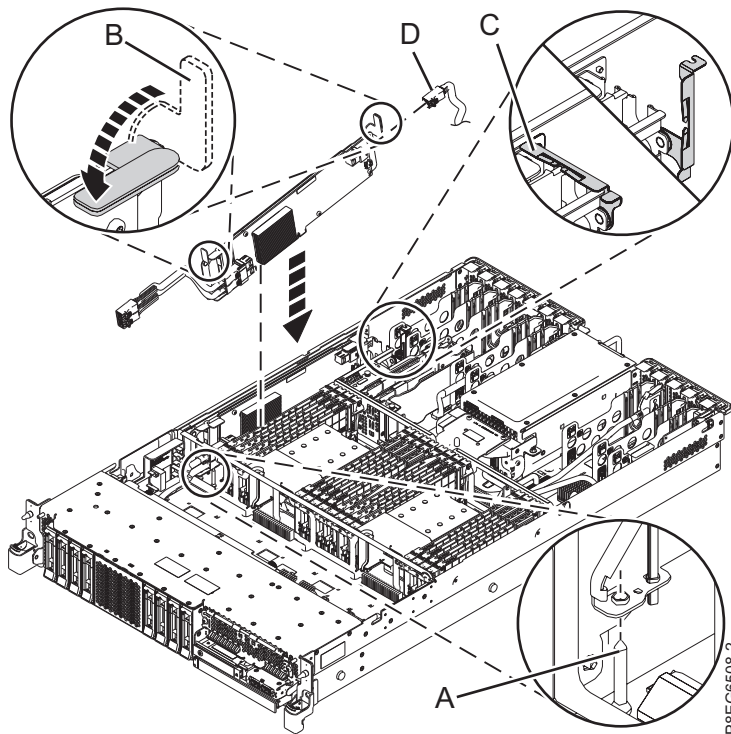
รูปที่ 6. การเปลี่ยน อะแดปเตอร์ภายใน PCIe3 x8 แคช SAS RAID ขนาด 6 Gb
