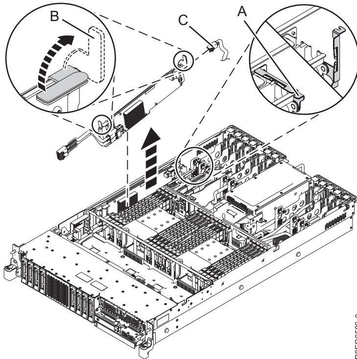
รูปที่ 4. การถอดอะแดปเตอร์ภายใน PCIe3 x8 แคช SAS RAID ขนาด 6 Gb
