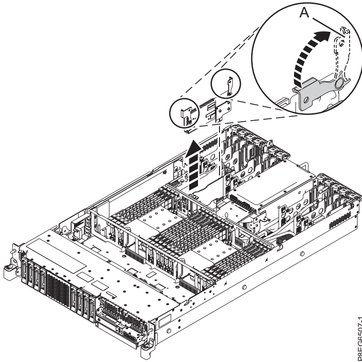
รูปที่ 5. การถอดการ์ดโมดูลไฟสำรอง
