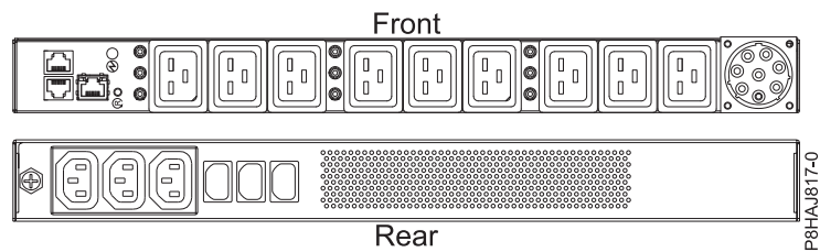
รูปที่ 41. PDU สำหรับระบบ 8408-44E
