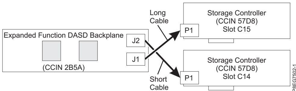
รูปที่ 8. การเชื่อมต่อสายเคเบิล SAS ในการกำหนดคอนฟิกฟังก์ชันส่วนขยายอีกครั้ง
