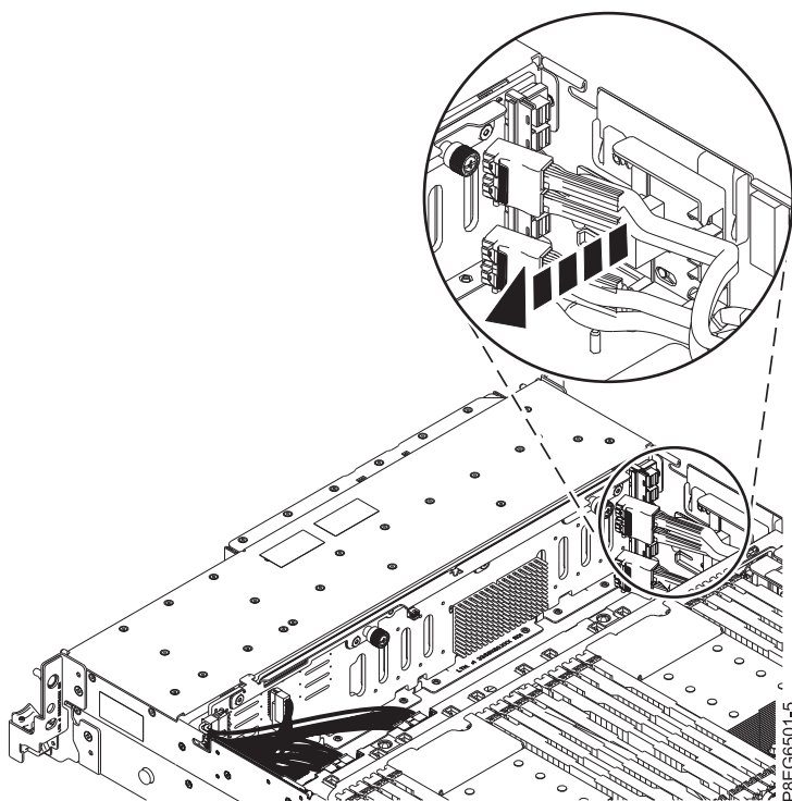
รูปที่ 3. การปลดสายเคเบิล SAS ด้านหน้าออกจากที่ยึดสายเคเบิล
