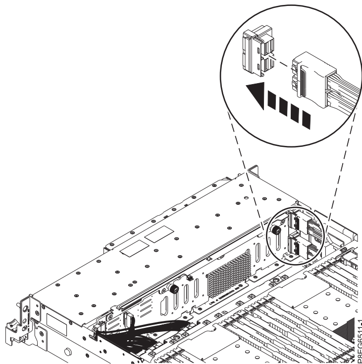
รูปที่ 9. การเชื่อมต่อสายเคเบิล SAS ด้านหน้ากับด้านหลังสล็อตไดรฟ์อีกครั้ง
