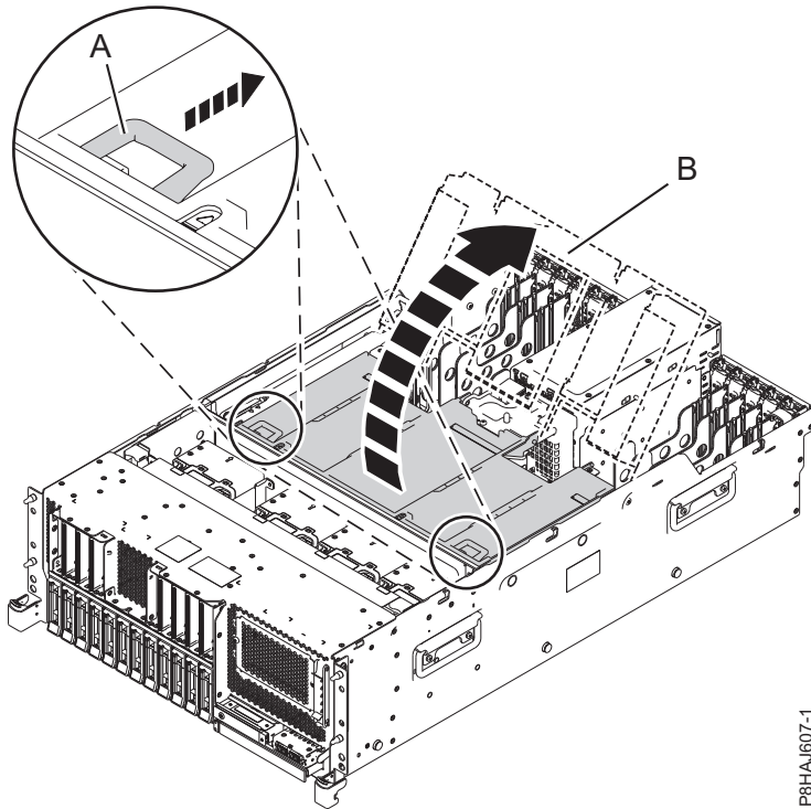
รูปที่ 32. การเปิดตัวไหลเวียนอากาศ
