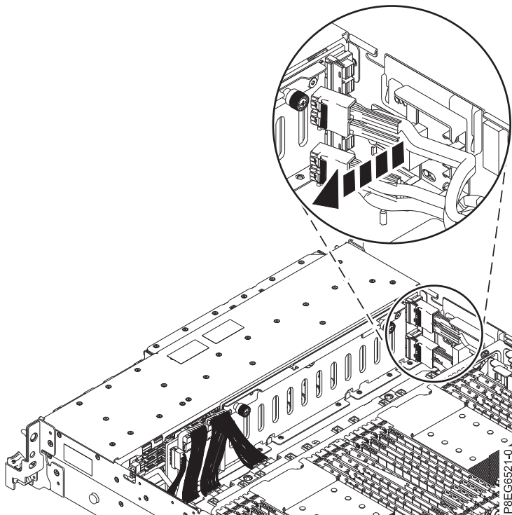
รูปที่ 3. การถอดสาย SAS
