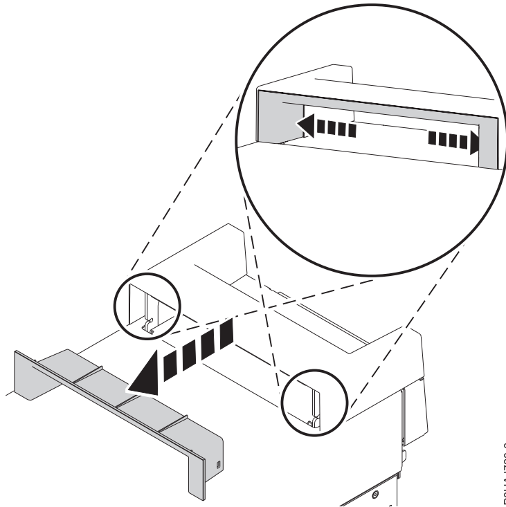
รูปที่ 29. การถอดชิ้นส่วนภายในฝาครอบด้ามจับระบบ 8286-41A สแตนด์อะโลน
