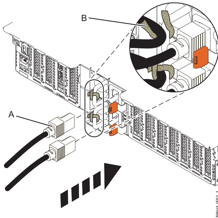
รูปที่ 62. การเชื่อมต่อสายไฟเข้ากับระบบ 5148-21L, 5148-22L, 8247-21L, 8247-22L, 8284-21A, or 8284-22A
