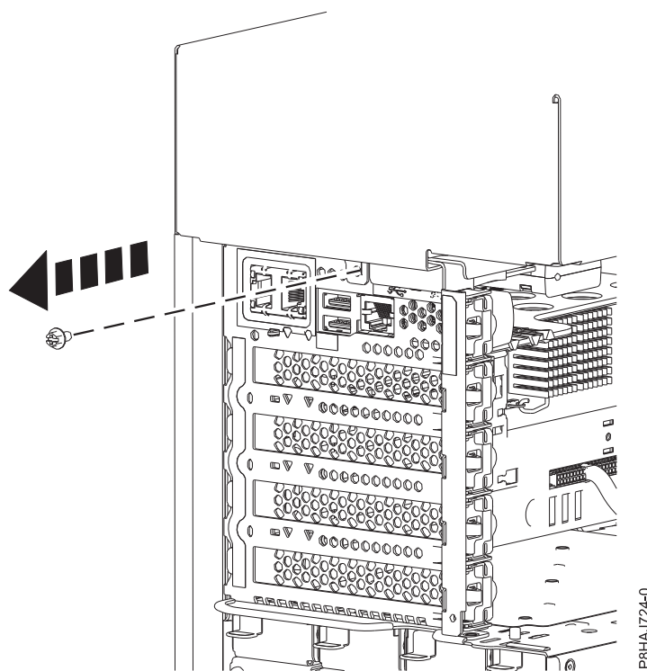
รูปที่ 31. การถอดสกรูออกจากฝาคาบด้านข้าง 8286-41A
