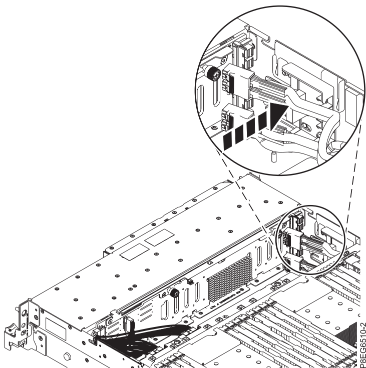
รูปที่ 20. ติดตั้งสาย SAS ด้านหน้า
