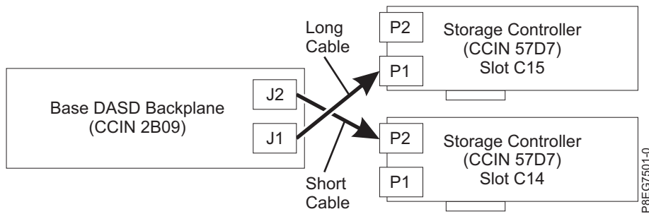
รูปที่ 11. การเชื่อมต่อสาย SAS อีกครั้งในคอนฟิกรูเรชัน ดิสก์แบบแยก
