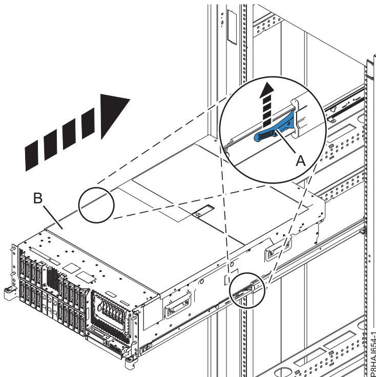
รูปที่ 51. การจัดตำแหน่งระบบในตำแหน่งการทำงาน
