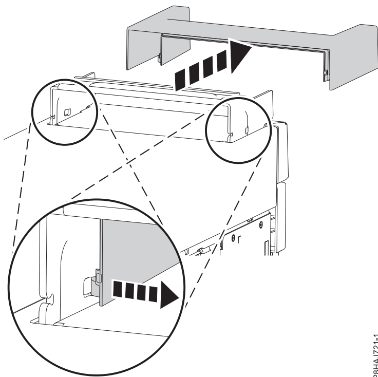
รูปที่ 30. การถอดฝาคาบด้ามจับออกจากระบบ 8286-41A สแตนด์อะโลน
