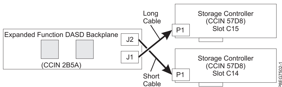
รูปที่ 22. การเชื่อมต่อสาย SAS อีกครั้ง ในคอนฟิกูเรชันฟังก์ชันแบบขยาย
