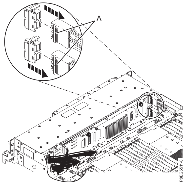
รูปที่ 14. การปลดสาย SAS ด้านหน้า
