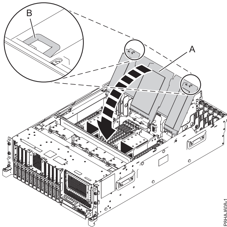
รูปที่ 46. การเปิด ตัวไล่อากาศ
