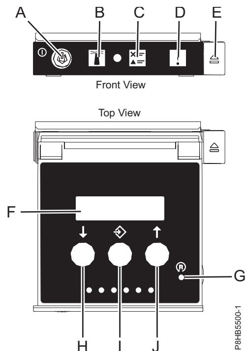
รูปที่ 25. แผงควบคุม
