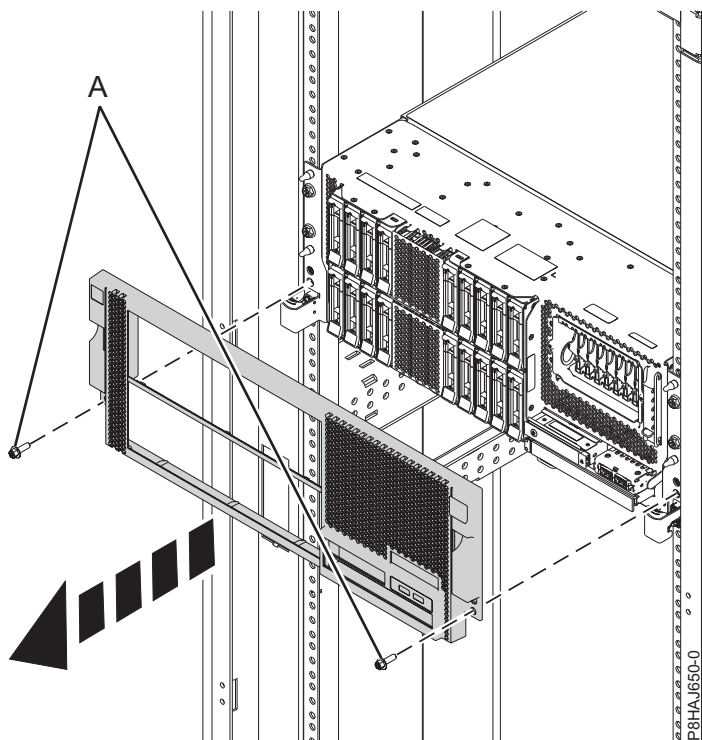
รูปที่ 27. การถอดฝาครอบด้านหน้า
