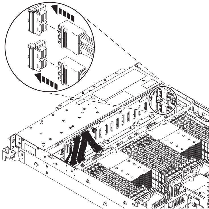
รูปที่ 9. การเชื่อมต่อสาย SAS ด้านหน้าอีกครั้ง
