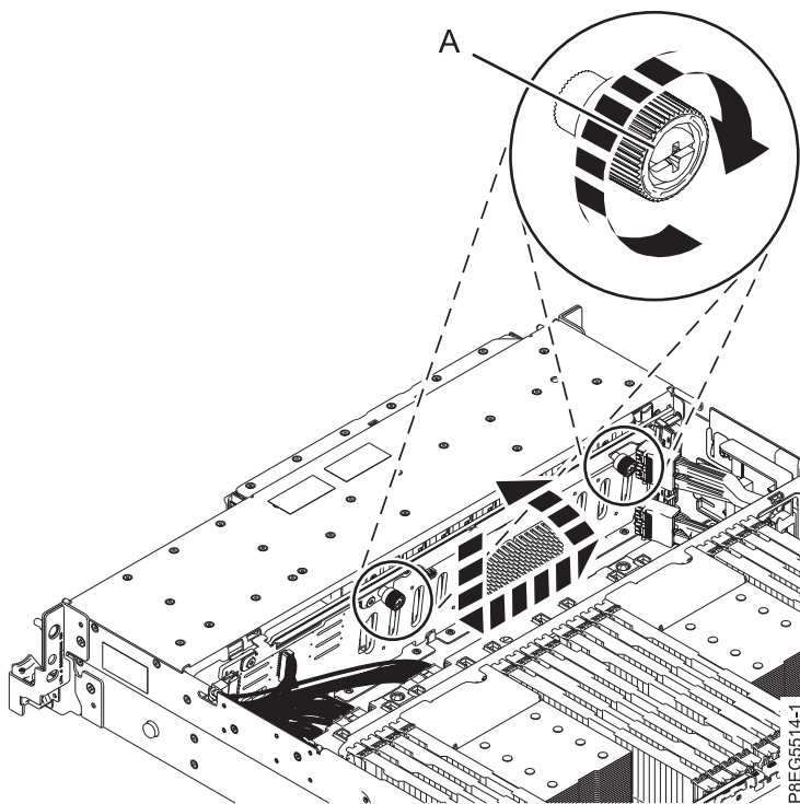
รูปที่ 19. การยึดแบ็คเพลนดิสก์ไดรฟ์ให้แน่น
