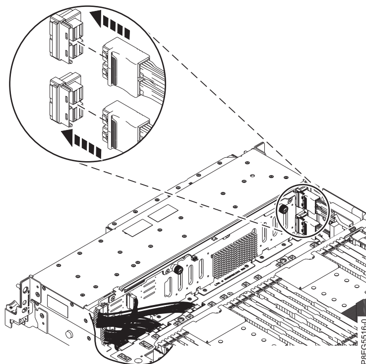
รูปที่ 21. การเชื่อมต่อสาย SAS ด้านหน้าอีกครั้ง
