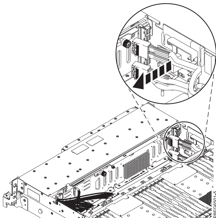
รูปที่ 15. การถอดสาย SAS
