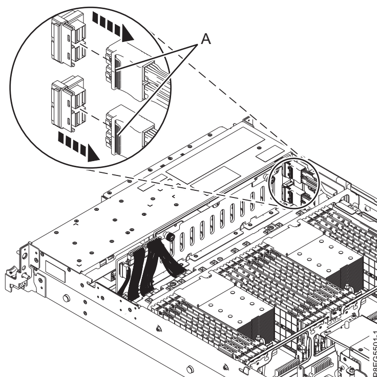
รูปที่ 2. การปลดสาย SAS ด้านหน้า
