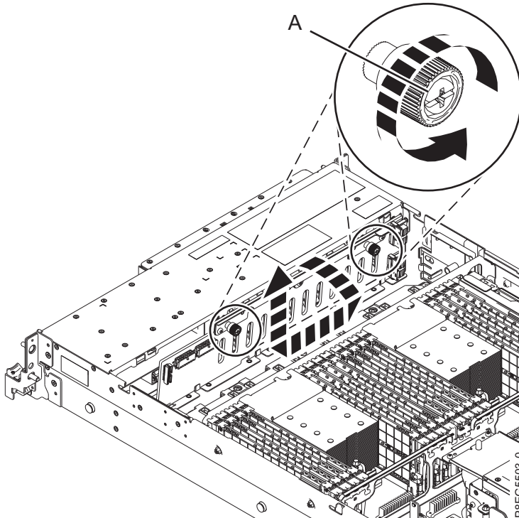
รูปที่ 5. การถอดแบ็คเพลน ดิสก์ไดรฟ์
