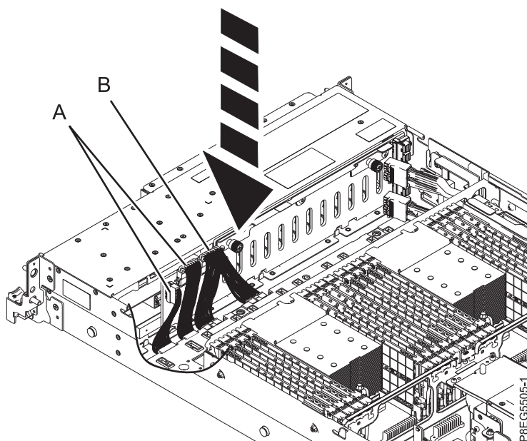
รูปที่ 7. เชื่อมต่อสายสัญญาณสายแพจควบคุม และสายไฟอีกครั้ง
