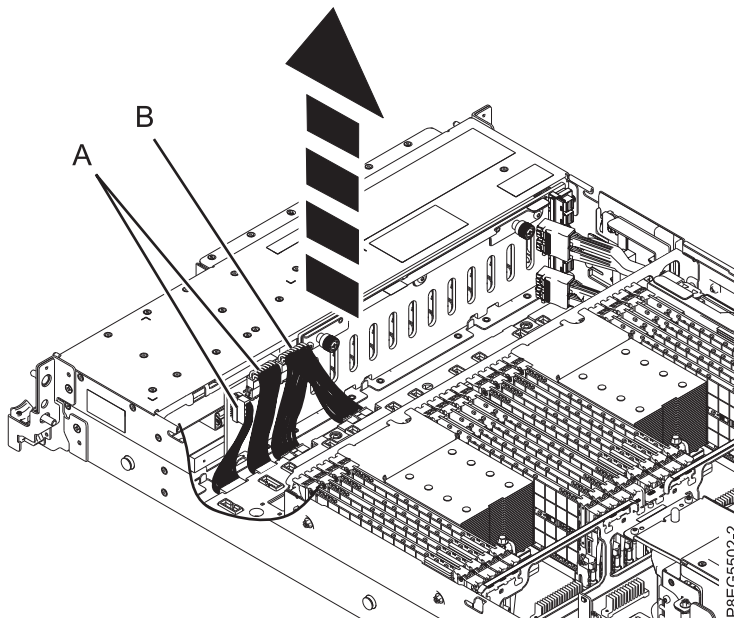
รูปที่ 4. การปลดสายสัญญาณ และสายของแผงควบคุม และสายไฟ
