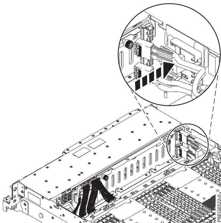
รูปที่ 8. ติดตั้งสาย SAS ด้านหน้า
