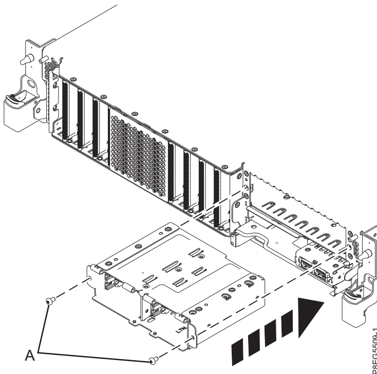
รูปที่ 23. ติดตั้งที่ใส่ SSD อีกครั้ง
