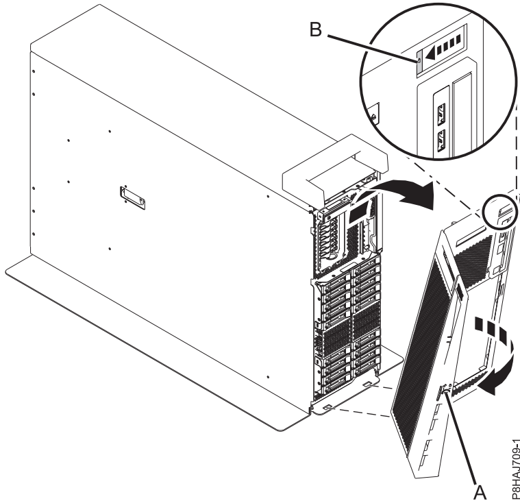
รูปที่ 28. การถอดฝาครอบด้านหน้า
