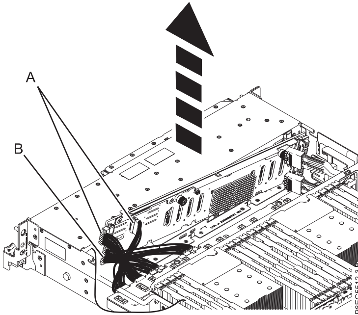
รูปที่ 17. การปลดสายไฟสายสัญญาณและสายแผงควบคุม
