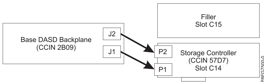
รูปที่ 10. การเชื่อมต่อสาย SAS อีกครั้งในคอนฟิกรูชัน หน่วยเก็บข้อมูลฐาน
