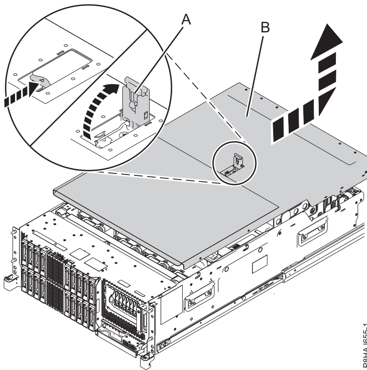
รูปที่ 41. การถอดฝาครอบการเข้าถึงเซอร์วิส
