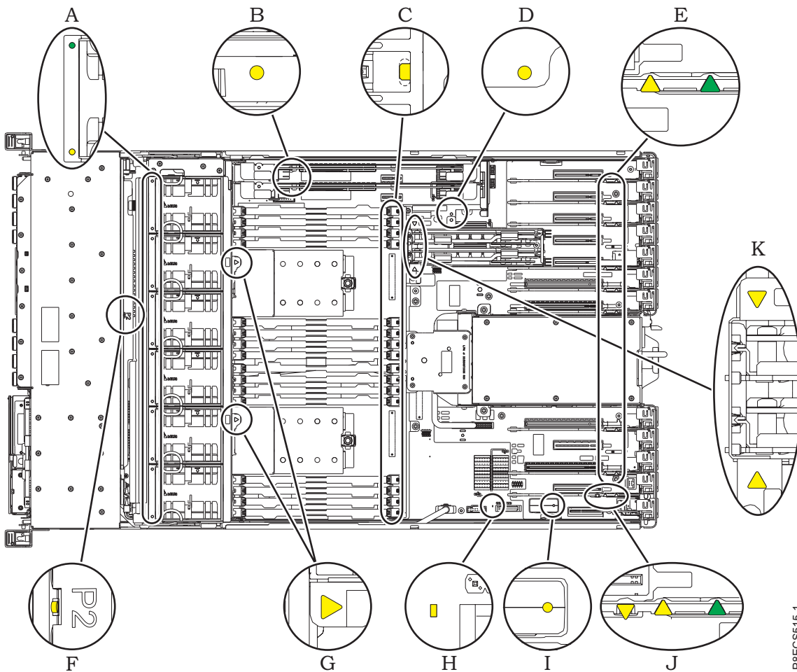
รูปที่ 12. LED แสดงสถานะเซอร์วิส
