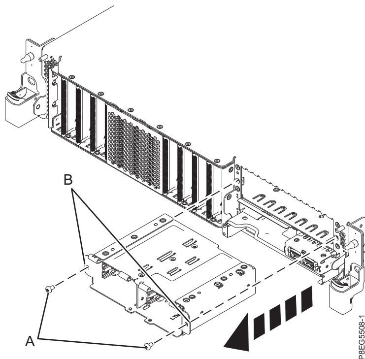
รูปที่ 13. ดึงที่เก็บ SSD ออกบางส่วน
