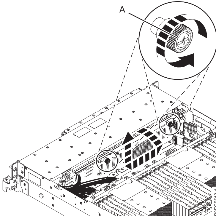
รูปที่ 16. การยี่ดแบ็คเพลนดิสก์ไดรฟ์ให้แน่น
