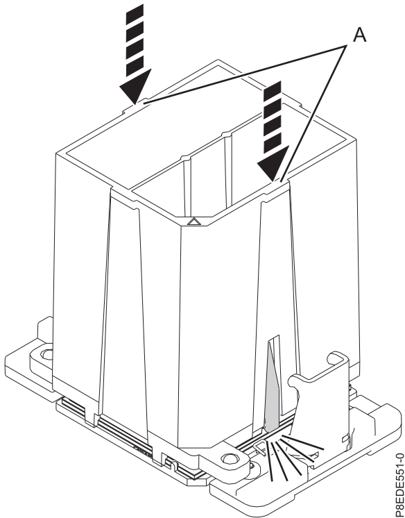
รูปที่ 30. การถอดโมดูลตัวประมวลผลระบบ เข้ากับเครื่องมือ
