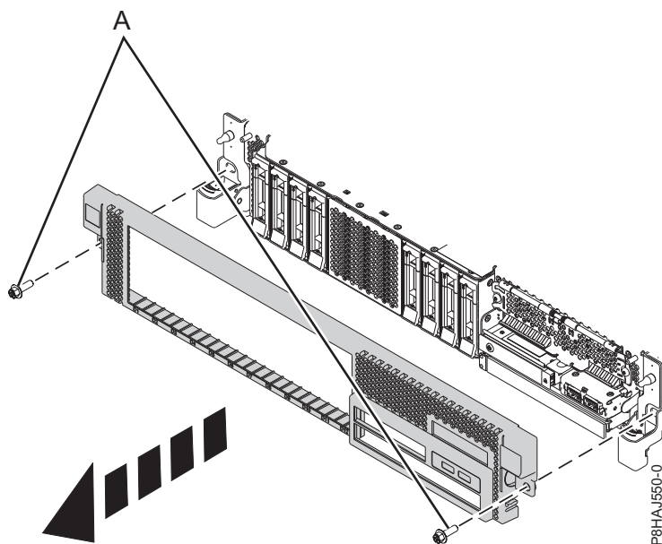
รูปที่ 48. การถอดฝาครอบด้านหน้า
