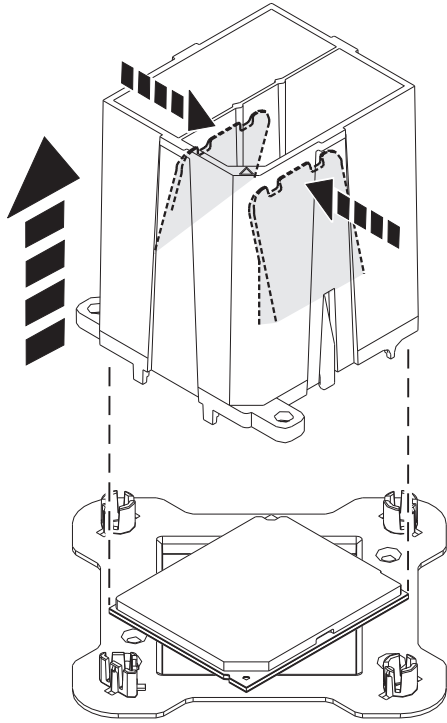
รูปที่ 32. การปลดโมดูลตัวประมวลผล ระบบออกจากเครื่องมือ
