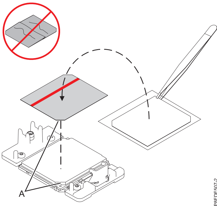
รูปที่ 17. การติดตั้ง TIM บนฝาปิดตัวประมวลผล
