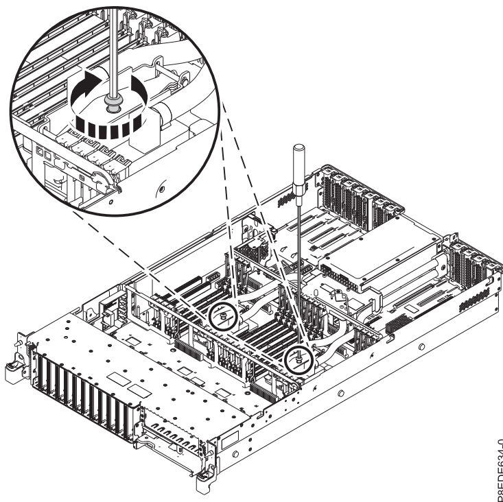
รูปที่ 42. การขันสกรูตัวยึดแผ่นระบายความร้อน
