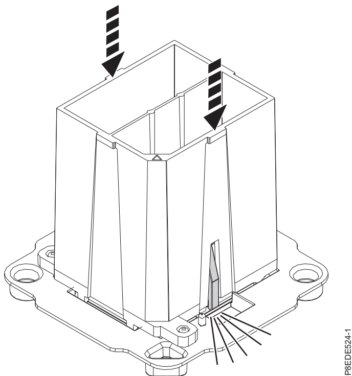
รูปที่ 11. การลีดโมดูลตัวประมวลผลระบบ เข้ากับเครื่องมือ
