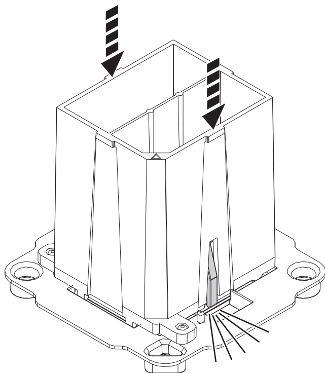
รูปที่ 34. การล๊อคโมดูลตัวประมวลผลระบบ เข้ากับเครื่องมือ
