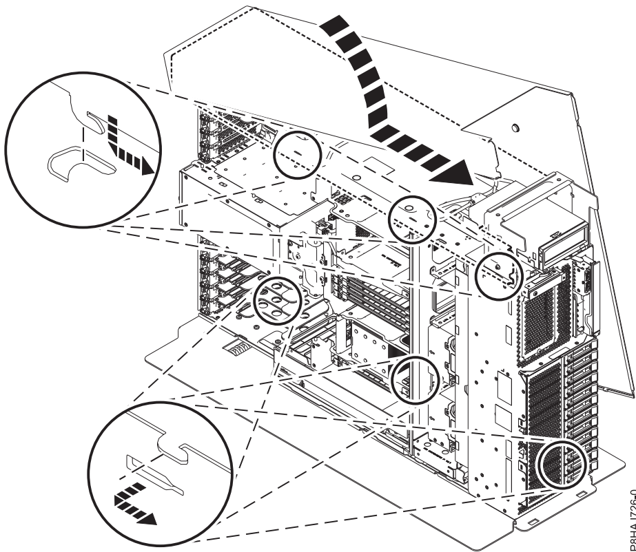
รูปที่ 61. การติดตั้งฝาครอบด้านข้าง 8286-41A
