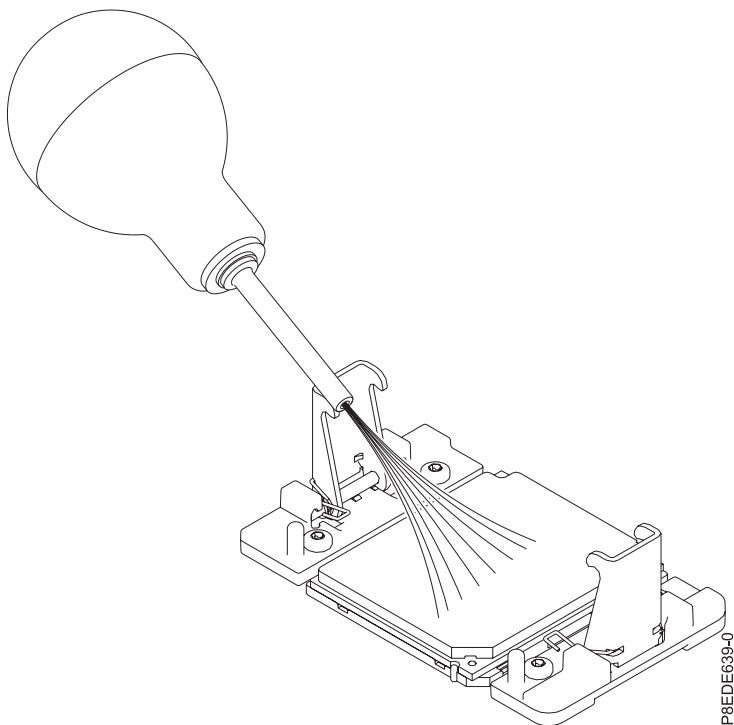
รูปที่ 28. การทำความสะอาดฝุ่นและสิ่งสกปรกในพื้นที่โมดูลตัวประมวลผลระบบ
