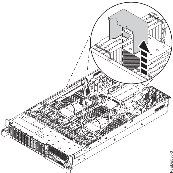
รูปที่ 3. การถอดตัวไหลเวียนอากาศ
