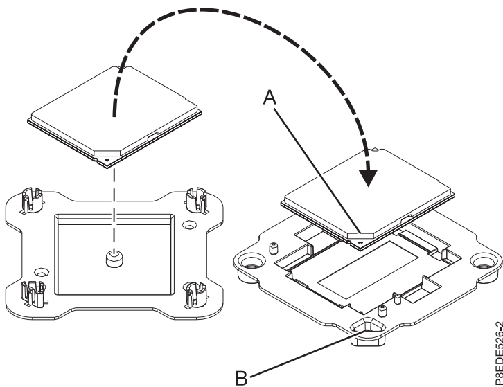
รูปที่ 45. การวาง โมดูลตัวประมวลผลระบบในแพ็คเกจ
