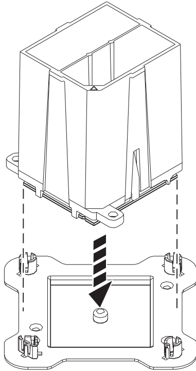
รูปที่ 31. การวางเครื่องมือ ไว้ที่มุมบนฝาปิดด้านบนของแพ็คเกจ
