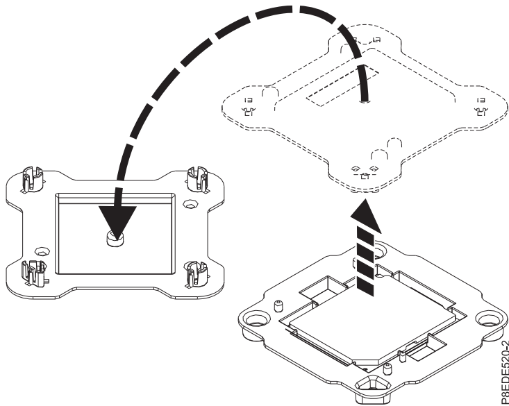
รูปที่ 23. การเปิดแพ็คเกจ โมดูลตัวประมวลผลระบบ
