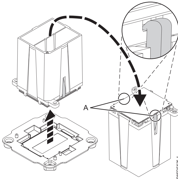
รูปที่ 12. การเตรียมสำหรับการติดตั้งโมดูลตัวประมวลผลระบบ
