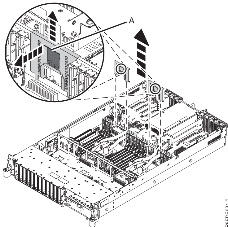
รูปที่ 24. การถอดแผ่นกัน
