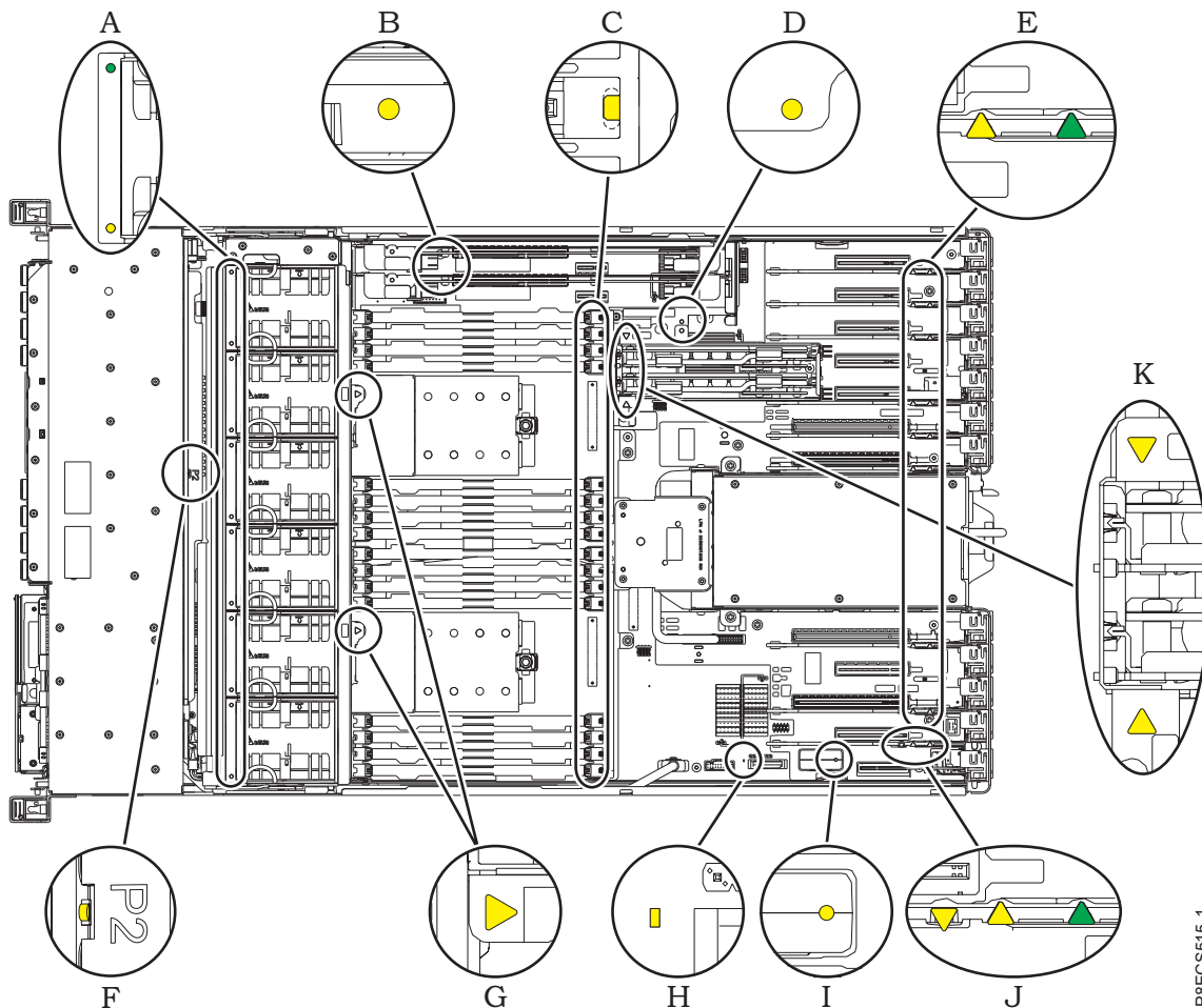
รูปที่ 1. LED แสดงสถานะเซิร์ฟเวอร์
