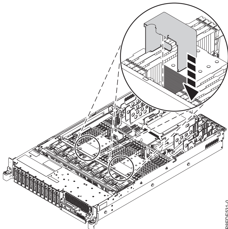
รูปที่ 20. การเปลี่ยนตัวไหลเวียนอากาศ
