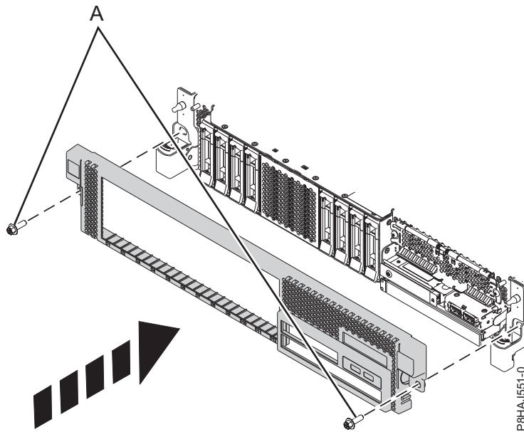
รูปที่ 55. การติดตั้งฝาครอบด้านหน้า
