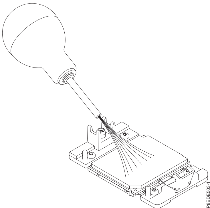
รูปที่ 5. การทำความสะอาดฝุ่นและสิ่งสกปรกในพื้นที่โมดูลตัวประมวลผลระบบ
