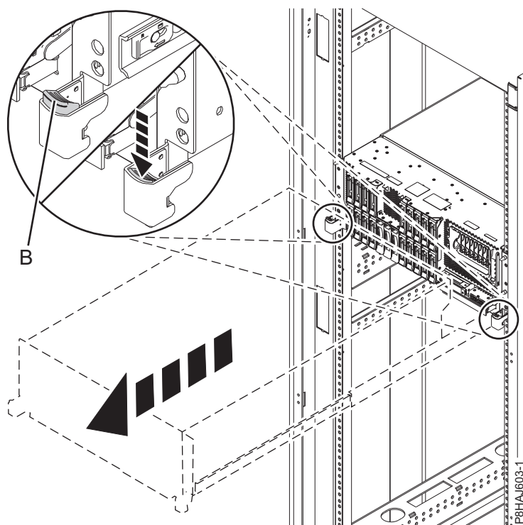
รูปที่ 72. การปลดแลตซ์ด้านข้าง
