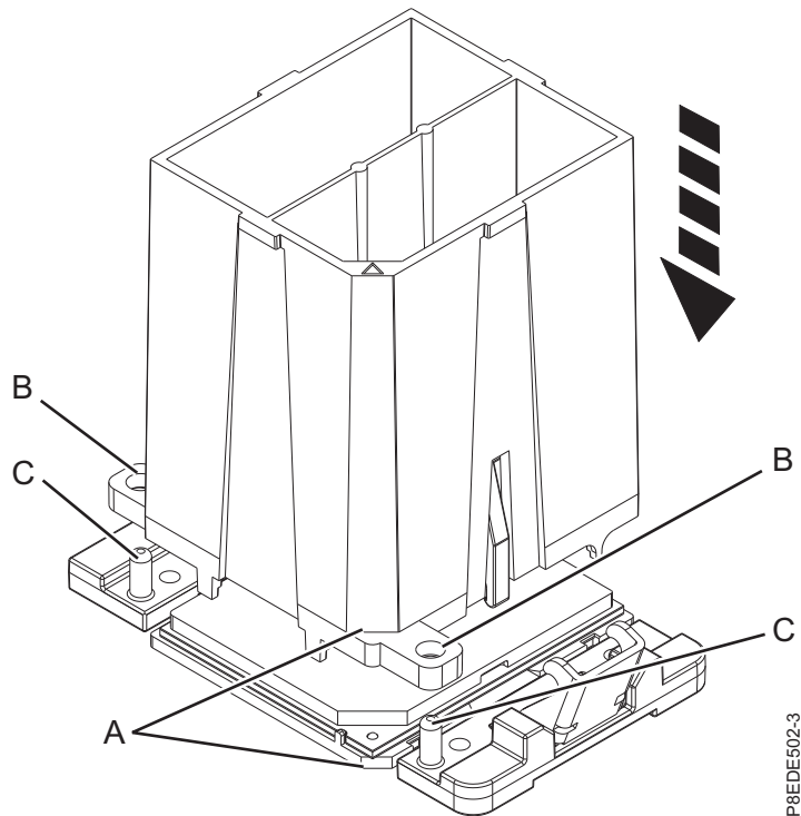
รูปที่ 6. การวางเครื่องมือสำหรับถอดลงบนโมดูลตัวประมวลผลระบบ
