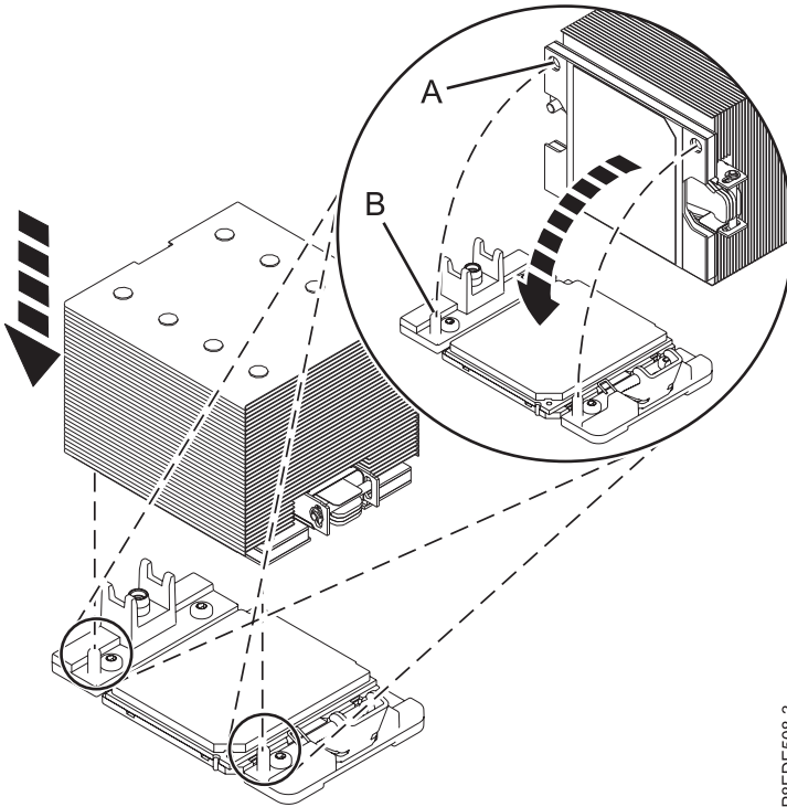
รูปที่ 18. การติดตั้งแผ่นระบายความร้อน
