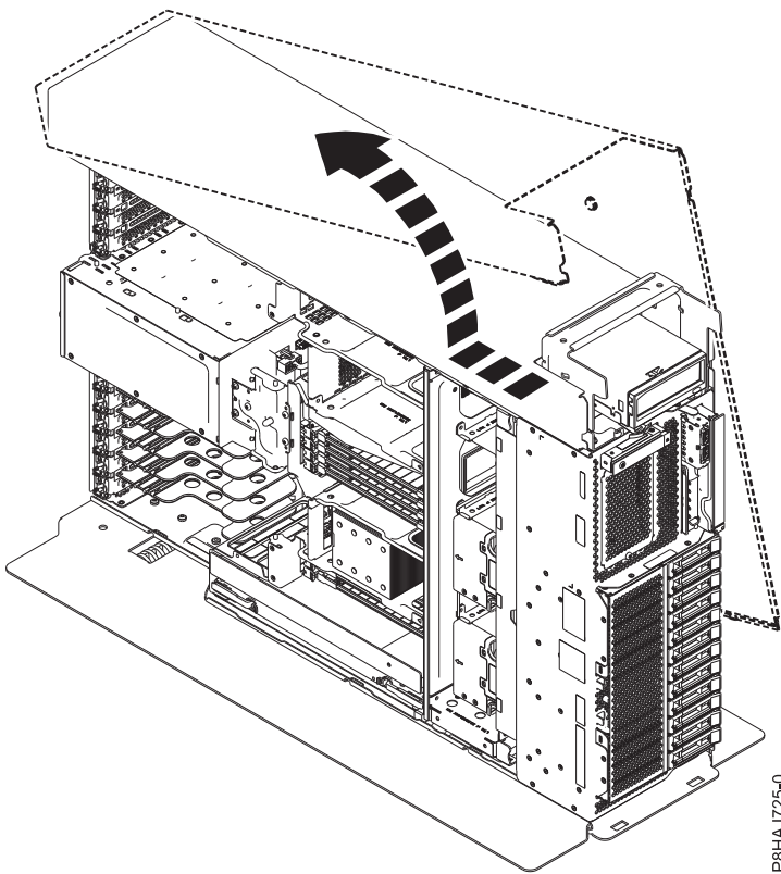
รูปที่ 54. การถอดฝาครอบด้านข้าง 8286-41A
