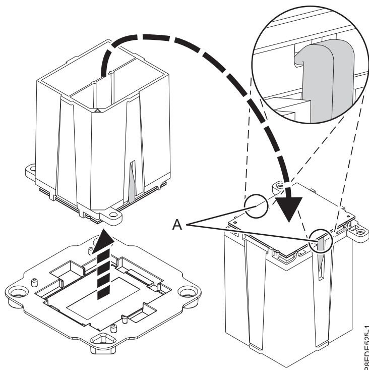
รูปที่ 35. การเตรียมสำหรับการติดตั้งโมดูลตัวประมวลผลระบบ
