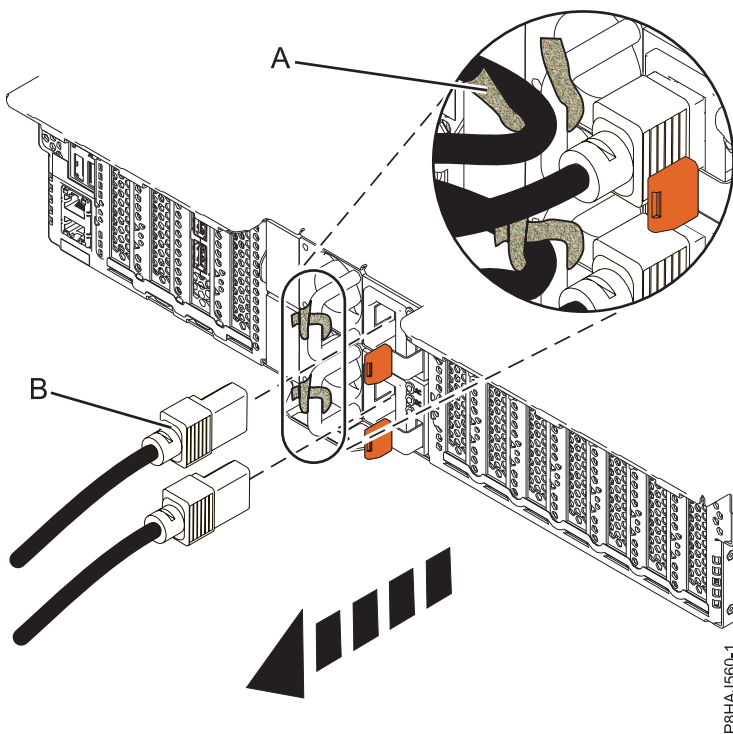
รูปที่ 78. การถอดสายไฟออกจากระบบ 5148-21L, 5148-22L, 8247-21L, 8247-22L, 8284-21A, or 8284-22A
