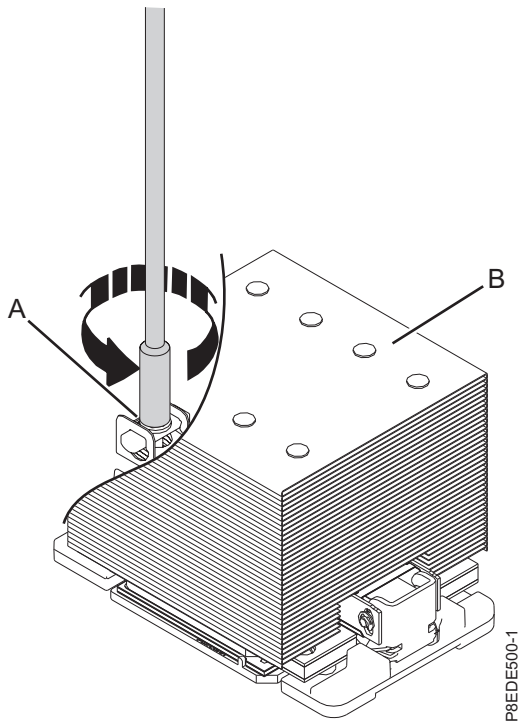
รูปที่ 4. การถอดแผ่นระบายความร้อน
