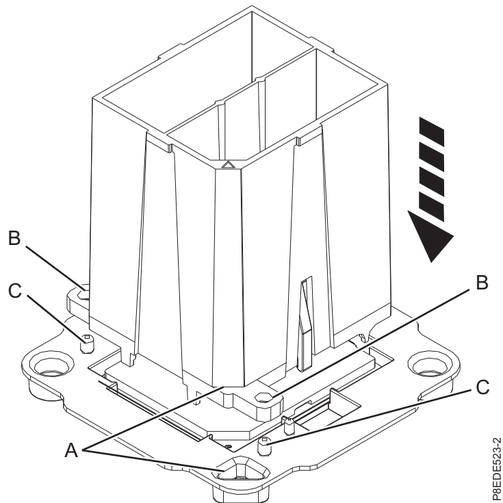
รูปที่ 33. การเตรียมสำหรับการติดตั้งโมดูลตัวประมวลผลระบบ
