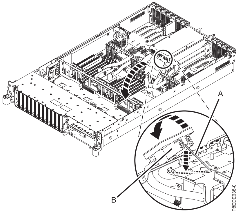
รูปที่ 41. การวางแผ่นระบายความร้อนลงบนโมดูลตัวประมวลผลระบบ
