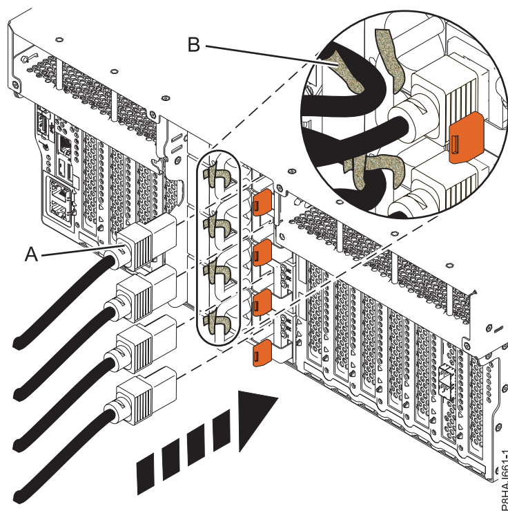
รูปที่ 83. การเชื่อมต่อสายไฟเข้ากับ ระบบ 8247-42L, 8286-41A หรือ 8286-42A
