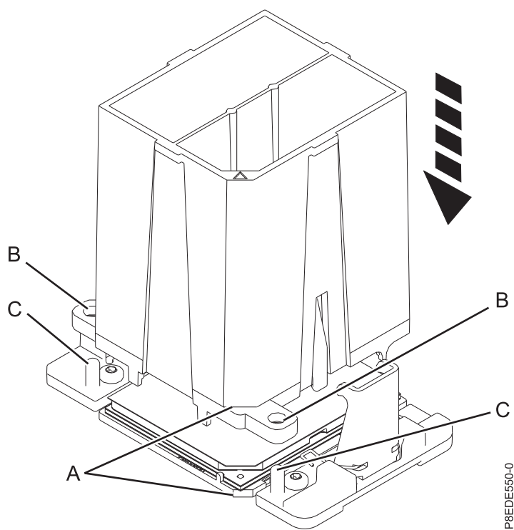
รูปที่ 29. การวางเครื่องมือสำหรับถอดบนโมดูลตัวประมวลผลระบบ
