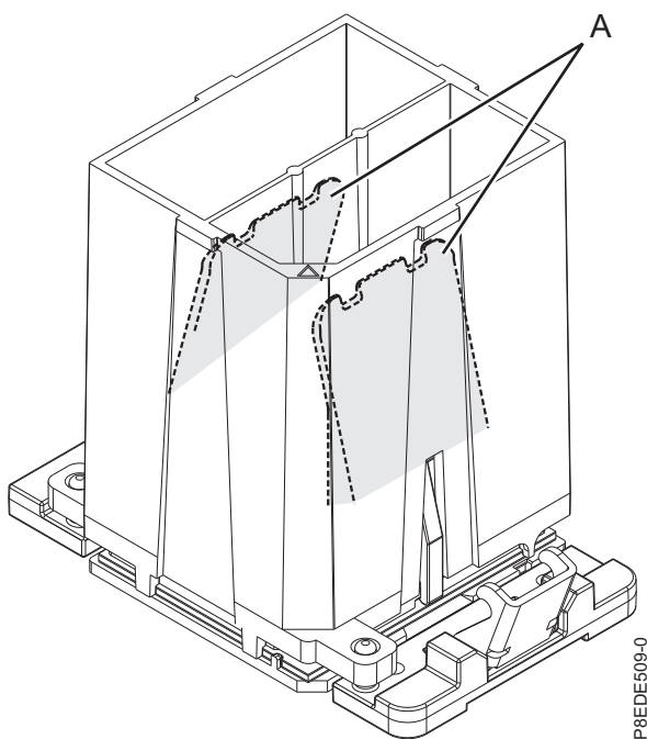
รูปที่ 15. การถอดเครื่องมือสำหรับ โมดูลตัวประมวลผลระบบ
