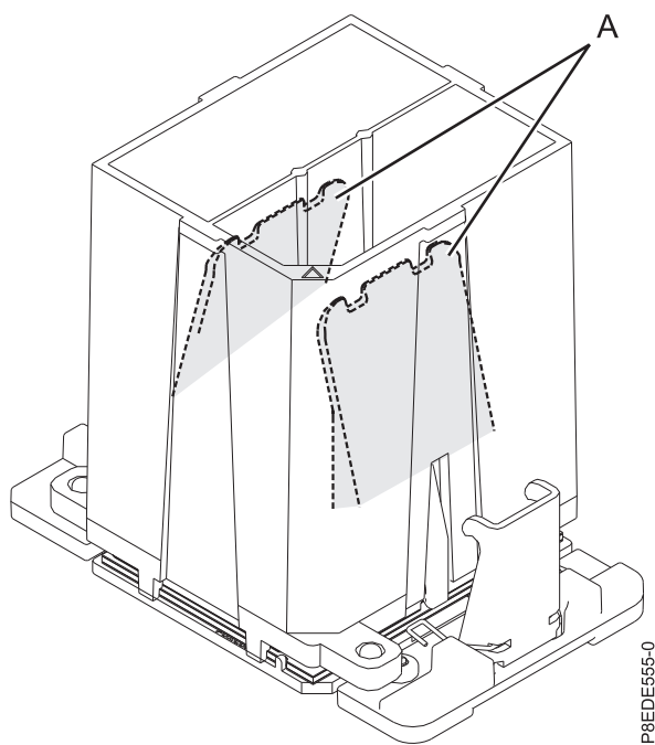
รูปที่ 38. การถอดเครื่องมือสำหรับโมดูลตัวประมวลผลระบบ
