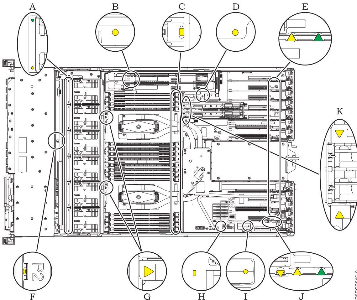
รูปที่ 22. LEDs ตัวบ่งชี้การบริการ
