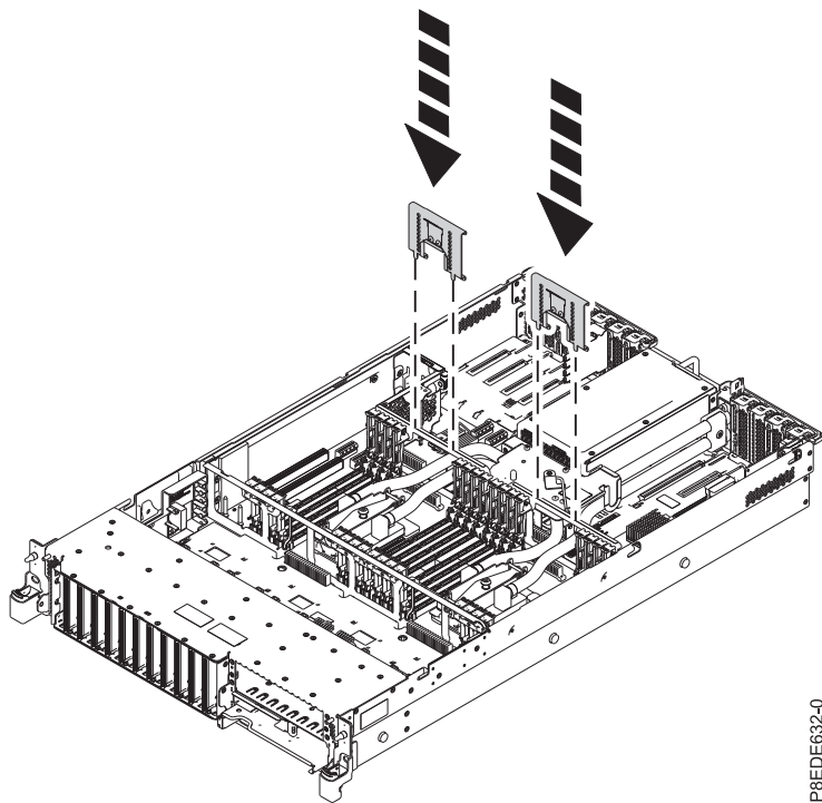
รูปที่ 44. การวางแผ่นกันลงในตำแหน่ง
