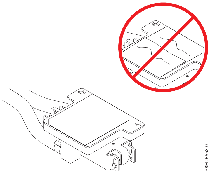
รูปที่ 39. การตรวจสอบวัสดุเชื่อมต่อการระบายความร้อน (TIM)
