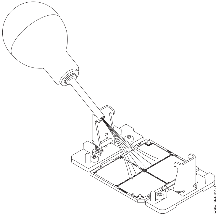
รูปที่ 36. การกำจัดฝุ่นและสิ่งสกปรกออกจากช็อกเก็ตตัวประมวลผลระบบ
