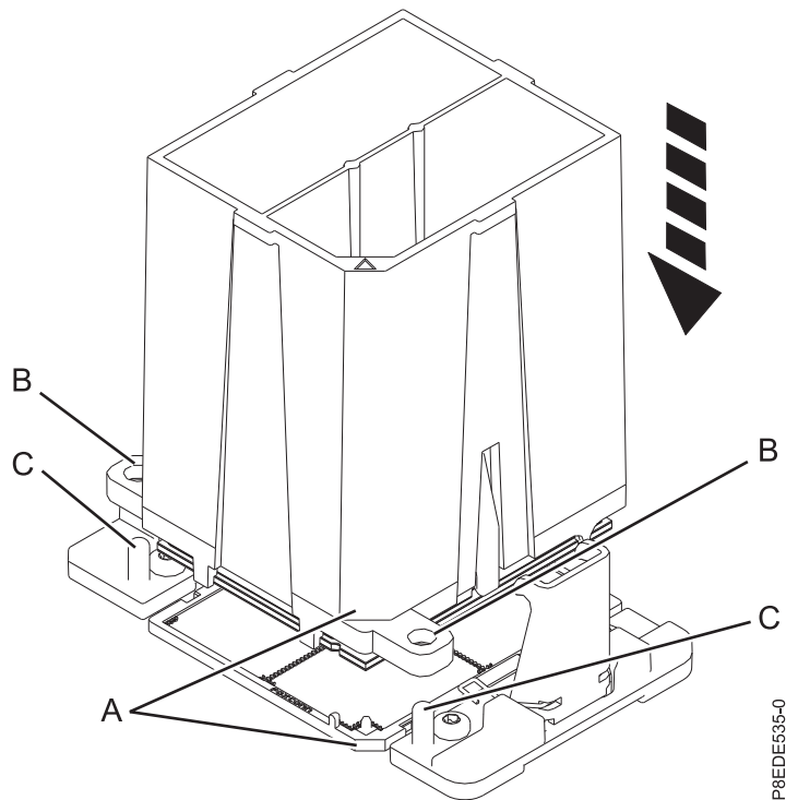
รูปที่ 37. การติดตั้งโมดูลตัวประมวลผลระบบ
