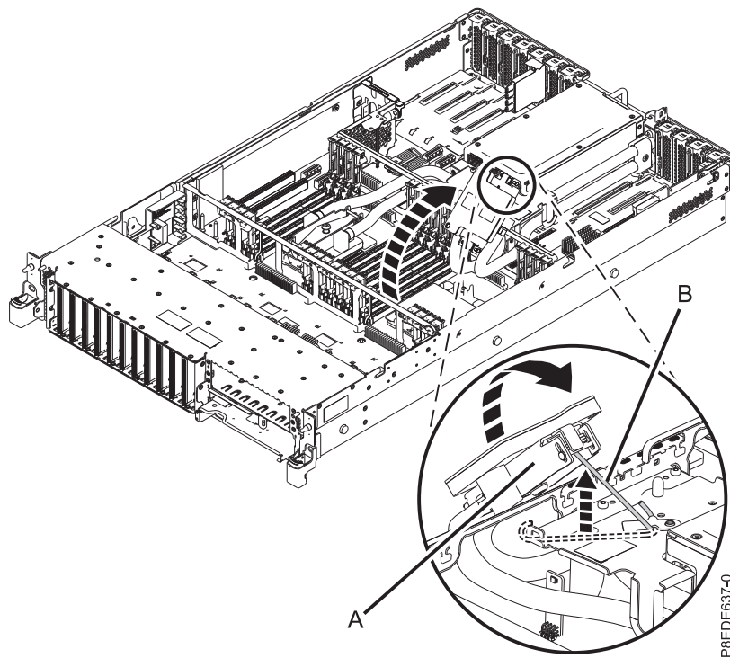
รูปที่ 27. การถอดแผ่นระบายความร้อน
