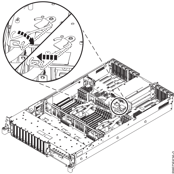
รูปที่ 43. การหมุนตะขอกลับไปยังตำแหน่งที่ใส่กลอน
