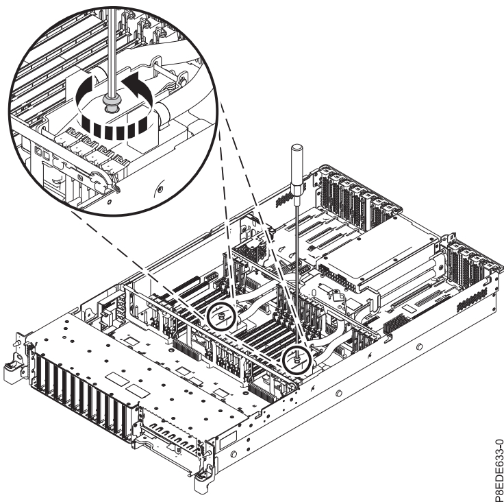
รูปที่ 26. การคลายสกรูตัวยึดแผ่นระบายความร้อน
