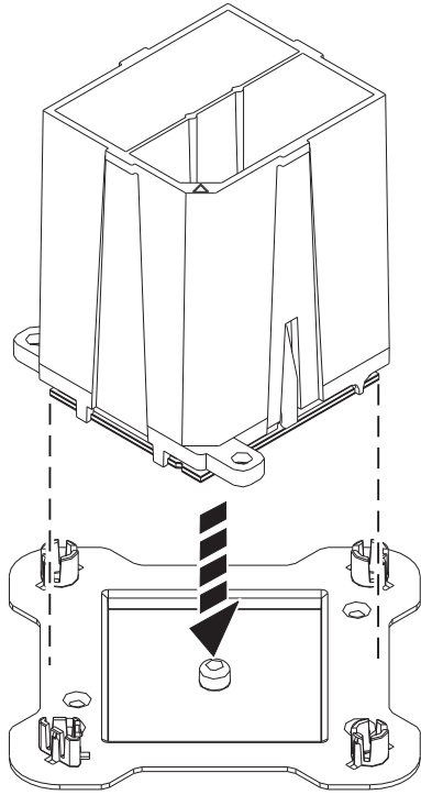
รูปที่ 8. การวางเครื่องมือ ไว้ที่มุมบนฝาปิดด้านบนของแพ็คเกจ
