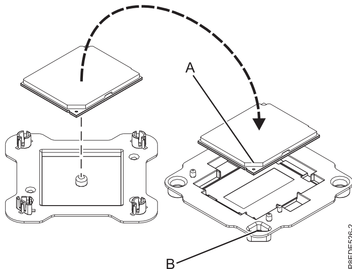
รูปที่ 21. การวาง โมดูลตัวประมวลผลระบบในแพ็คเกจ
