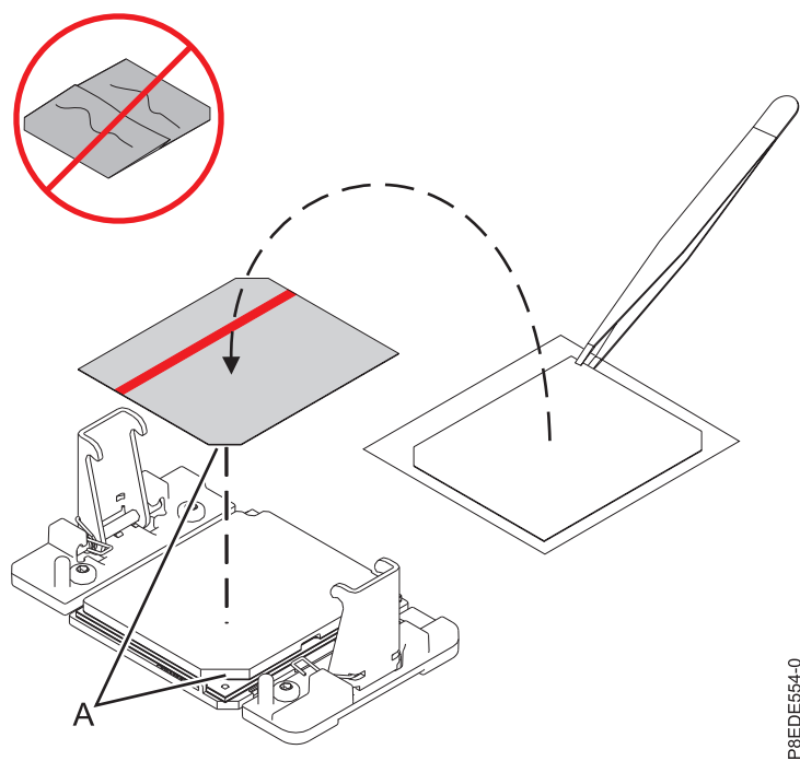
รูปที่ 40. การเปลี่ยนวัสดุเชื่อมต่อการระบายความร้อน (TIM)
