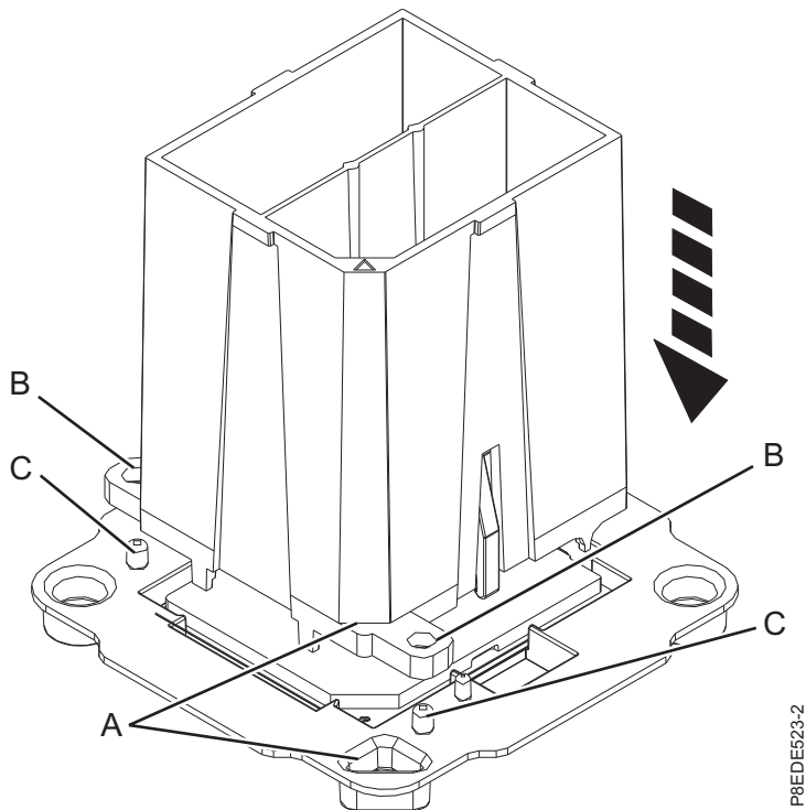
รูปที่ 10. การเตรียมสำหรับการติดตั้งโมดูลตัวประมวลผลระบบ
