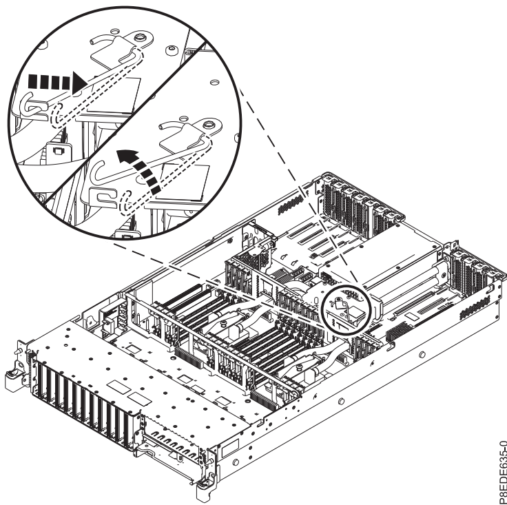
รูปที่ 25. ถอดสลักตะขอ
