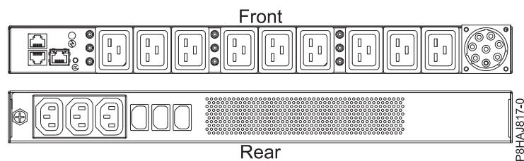
รูปที่ 76. PDU สำหรับระบบ 8408-44E
