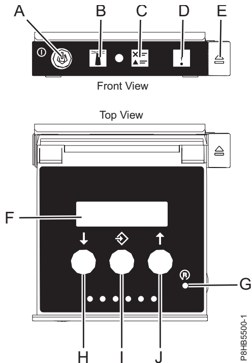
รูปที่ 47. แผงควบคุม
