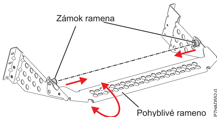
Obrázok 52. Konzola na organizáciu káblov
