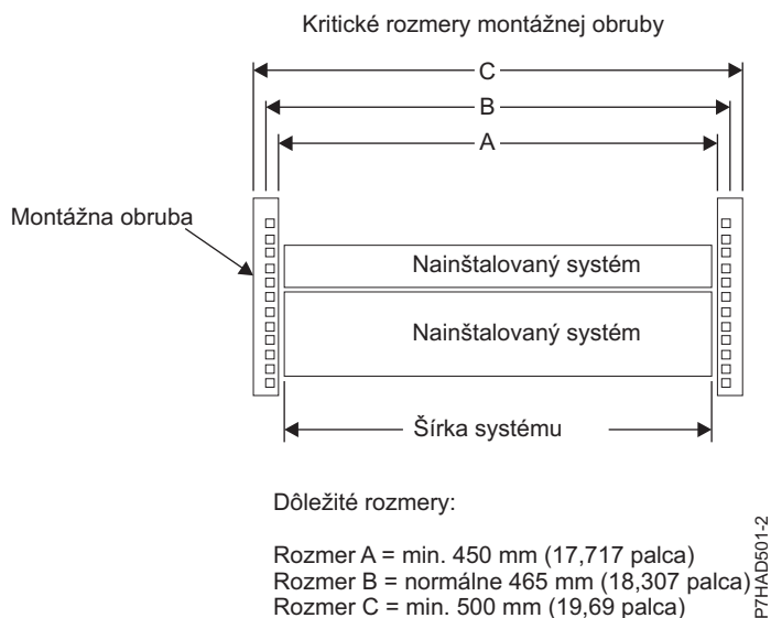
Obrázok 43. Kritické rozmery montážnej obruby
