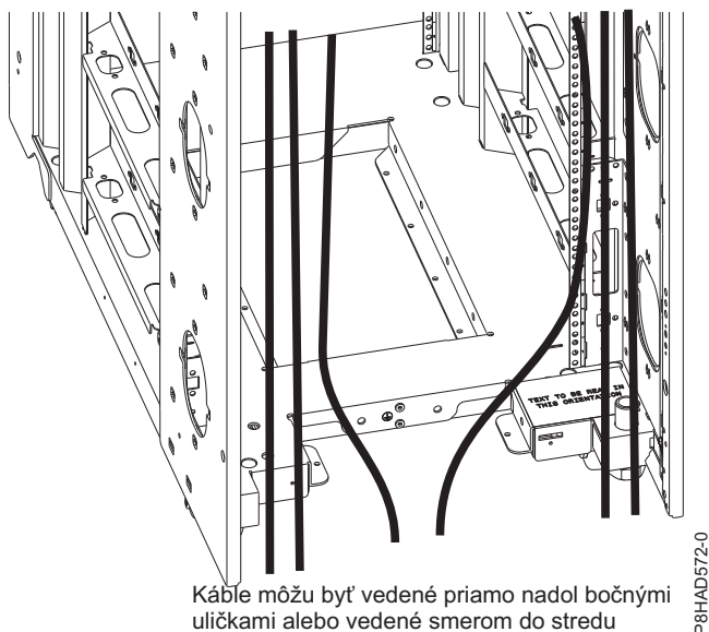
Obrázok 37. Vedenie káblov pod podlahou
