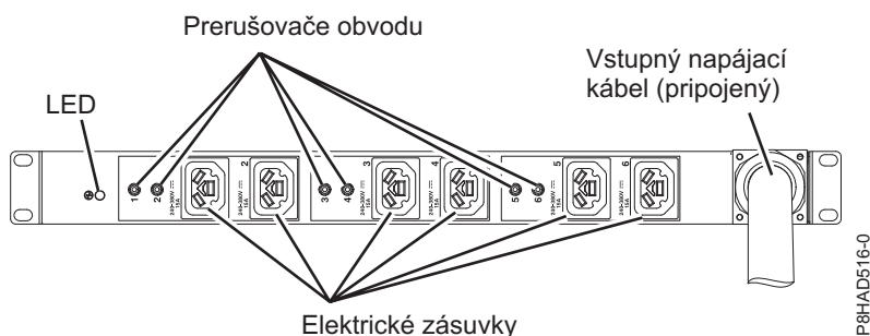
Obrázok 49. HVDC PDU
