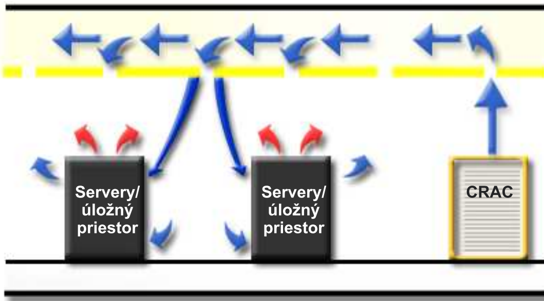
Obrázok 44. Stropný rozvod vzduchu
