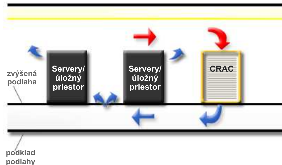
Obrázok 42. Rozvod vzduchu pod podlahou
