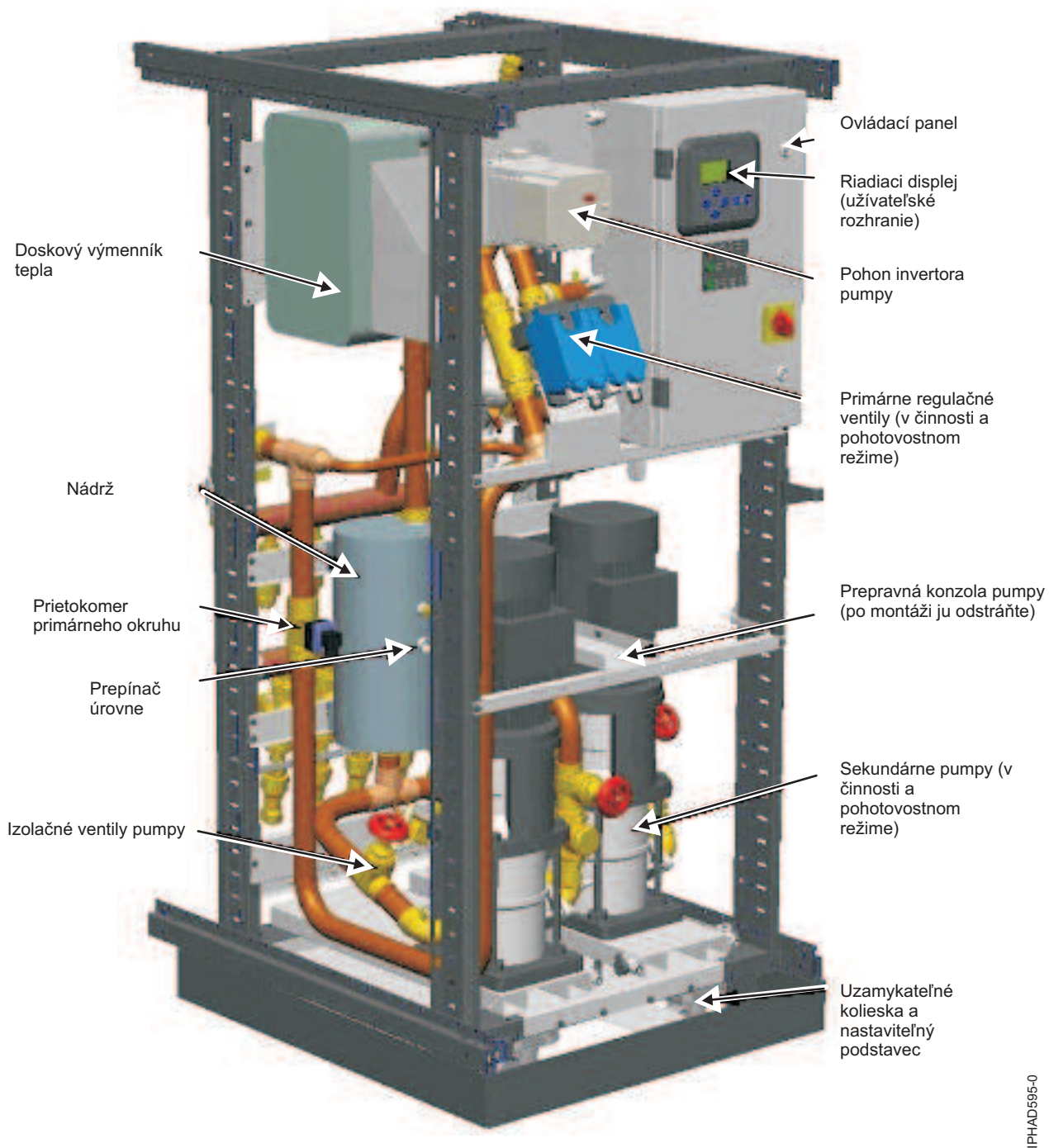
Obrázok 33. Chladiaca distribučná jednotka
