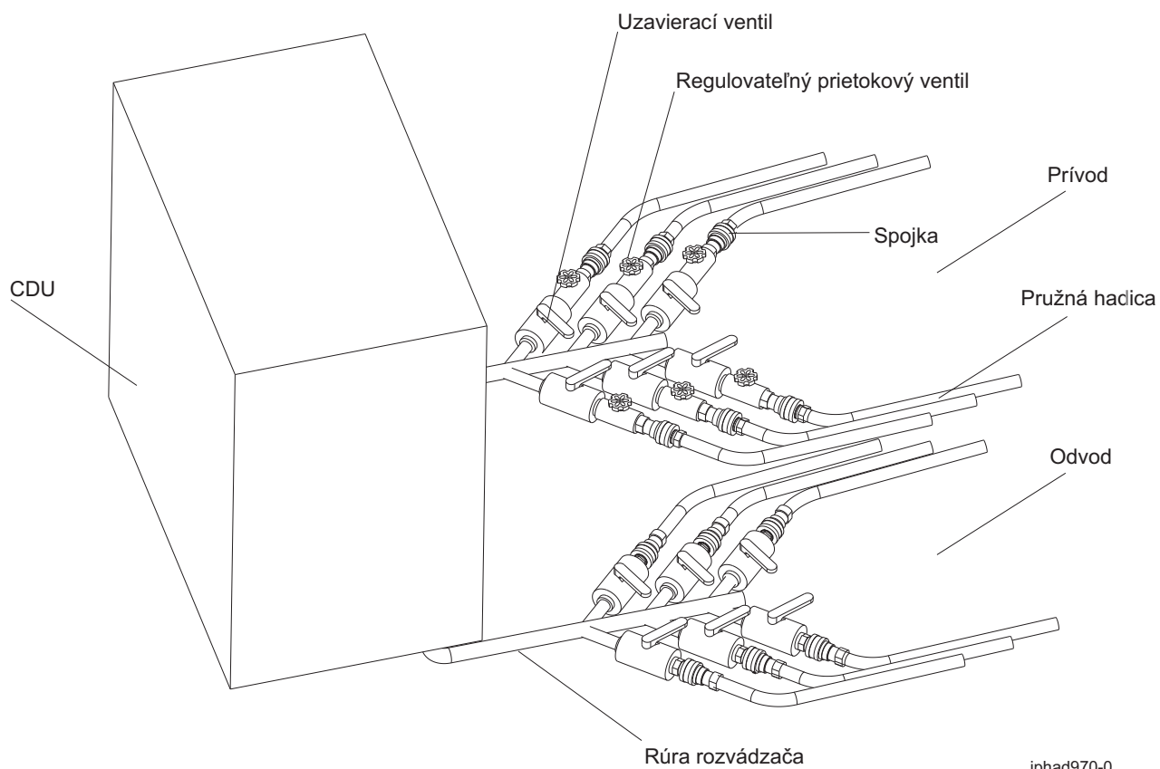
Obrázok 20. Typické umiestnenie centrálneho distribučného rozvádzača na centrálnom mieste
