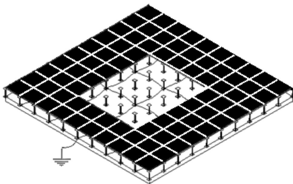
Obrázok 37. signálová referenčná zem
