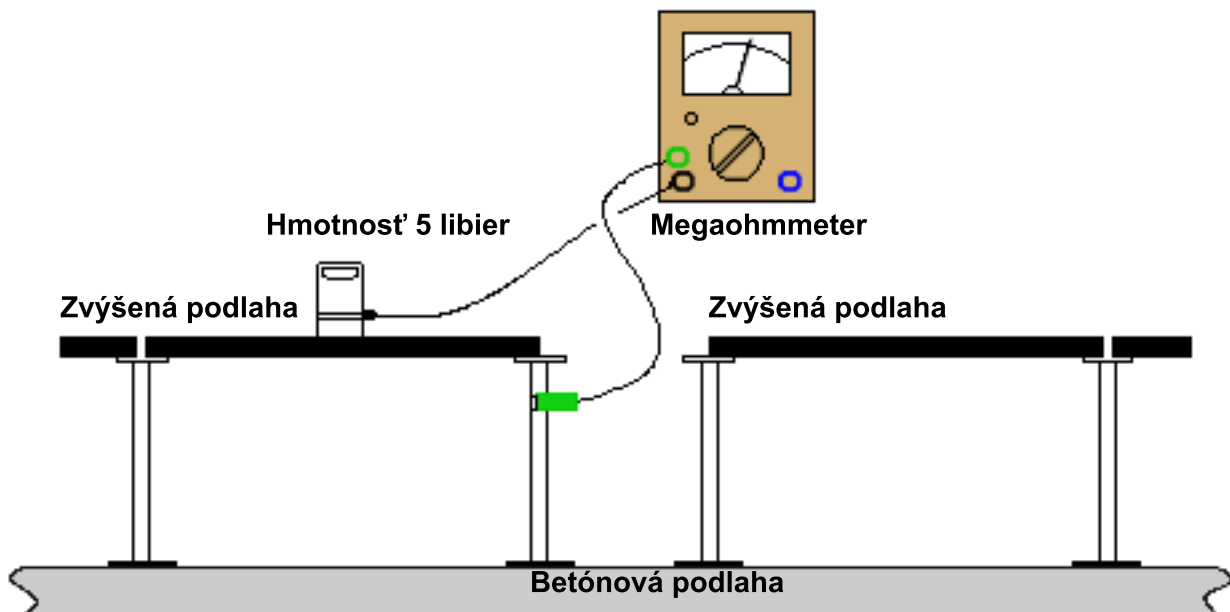
Obrázok 41. Typické testovacie zapojenie na meranie vodivosti podlahy
