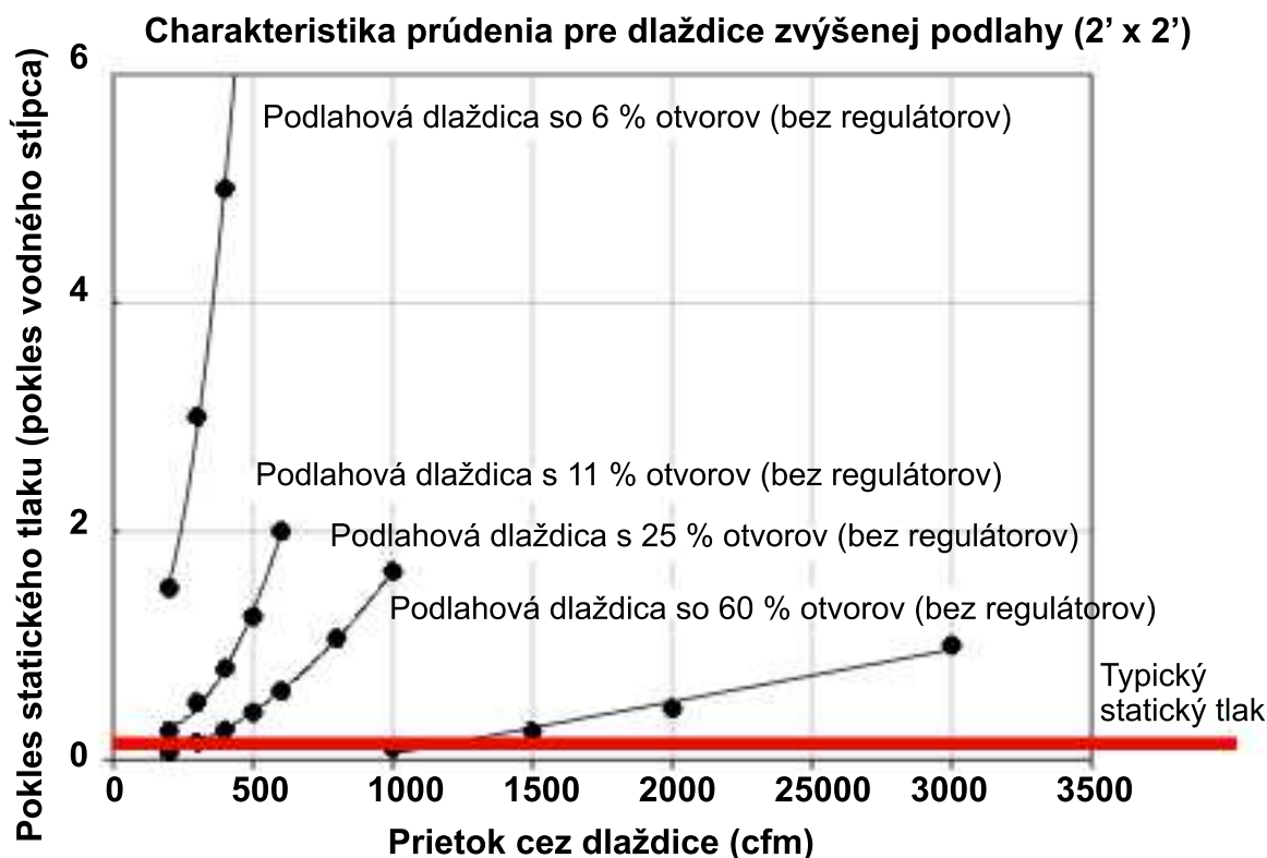
Obrázok 5. Kapacity objemového prietoku rôznych dlaždíc pre zvýšené podlahy
