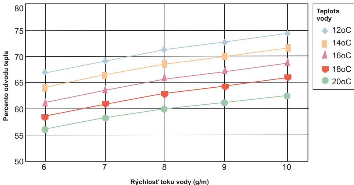
Obrázok 14. Typický výkon výmenníka tepla v zadných dvierkach pri tepelnej záťaži 32 kW. Percento odvodu tepla je funkciou teploty vody a rýchlosti toku. (Teplota vstupujúceho vzduchu do stojana 24 °C, zaťaženie stojana 32 kW, prietok vzduchu cez výmenník tepla v zadných dvierkach 1530 kubických stôp za minútu)
