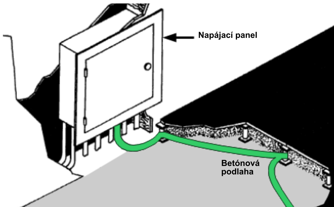
Obrázok 36. Prechodné uzemnenie, ktoré využíva podpornú štruktúru zvýšenej podlahy
