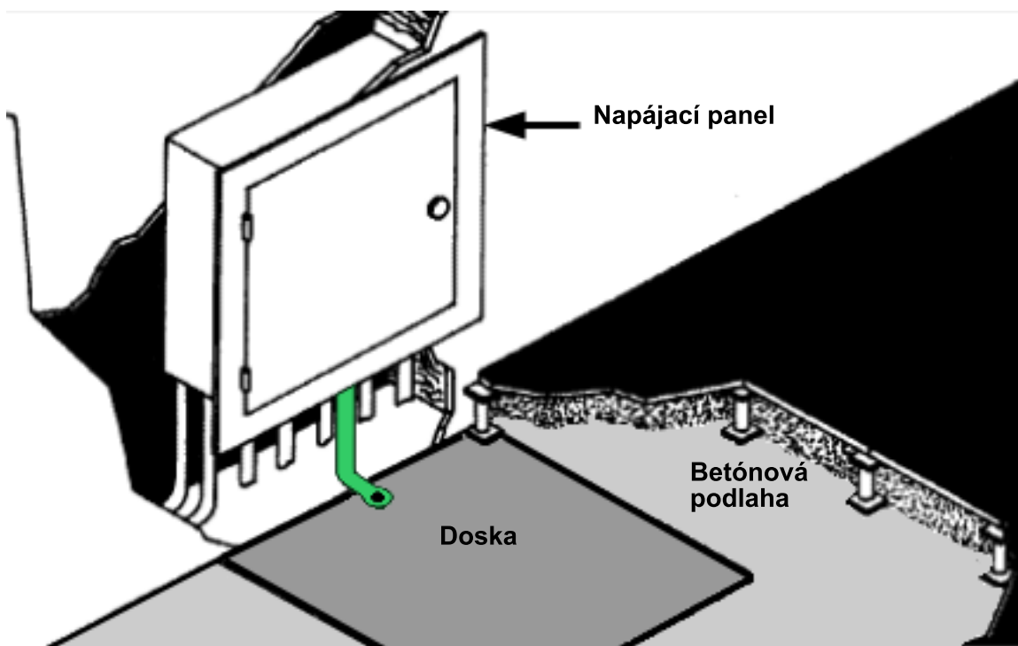
Obrázok 35. Prechodná uzemňovacia doska
