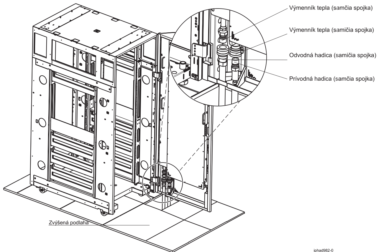
Obrázok 24. Príklad 1: Manažment hadíc pri zvýšenej podlahe; veľkosť otvoru v dlaždici a miesto pre 24-palcové stojany
