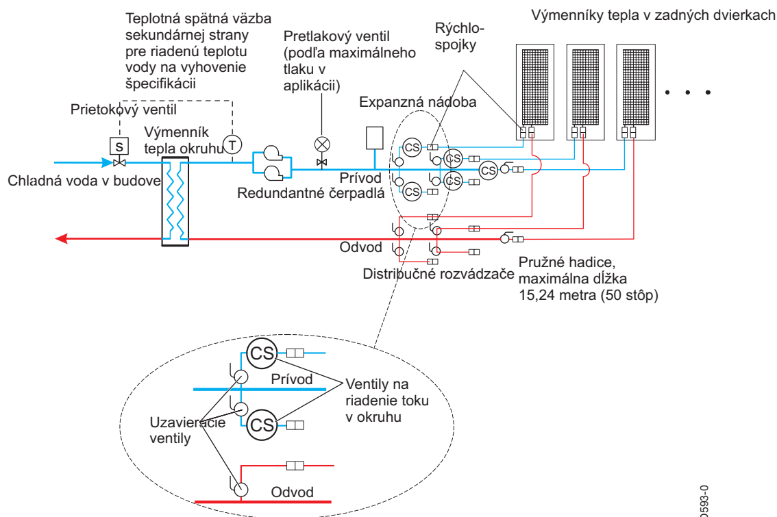
Obrázok 16. Distribúcia chladiaceho média pomocou systému na distribúciu vody v zariadení
