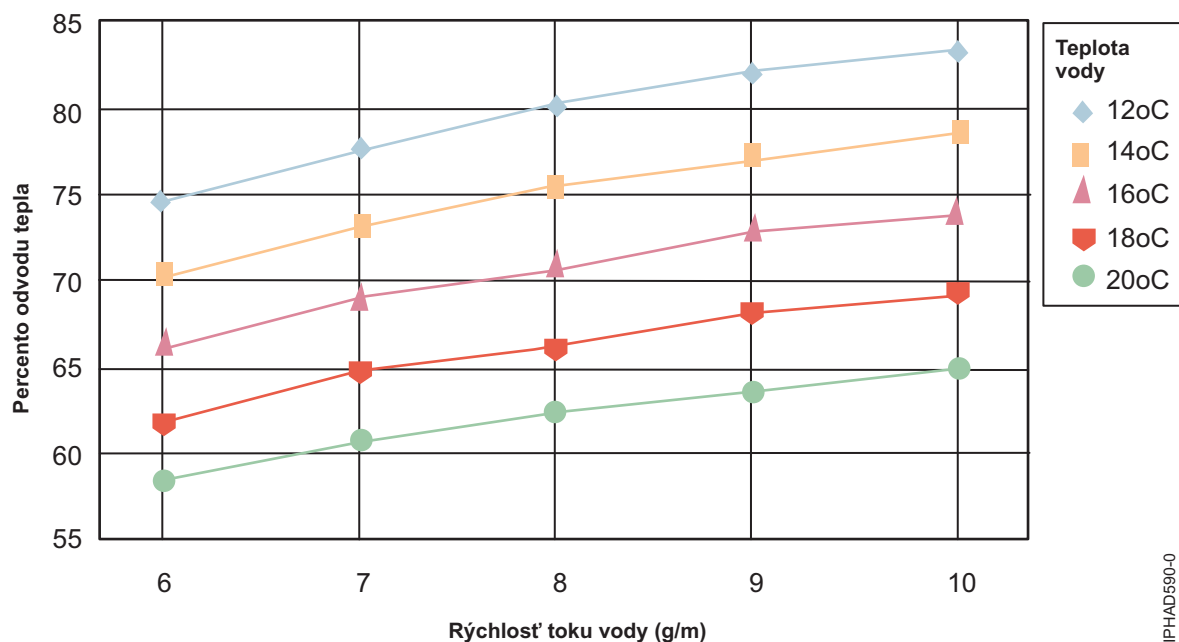
Obrázok 15. Typický výkon výmenníka tepla v zadných dvierkach pri tepelnej záťaži 20 kW. Percento odvodu tepla je funkciou teploty vody a rýchlosti toku. (Teplota vstupujúceho vzduchu do stojana 24 °C, zaťaženie stojana 20 kW, prietok vzduchu cez výmenník tepla v zadných dvierkach 1530 kubických stôp za minútu)
