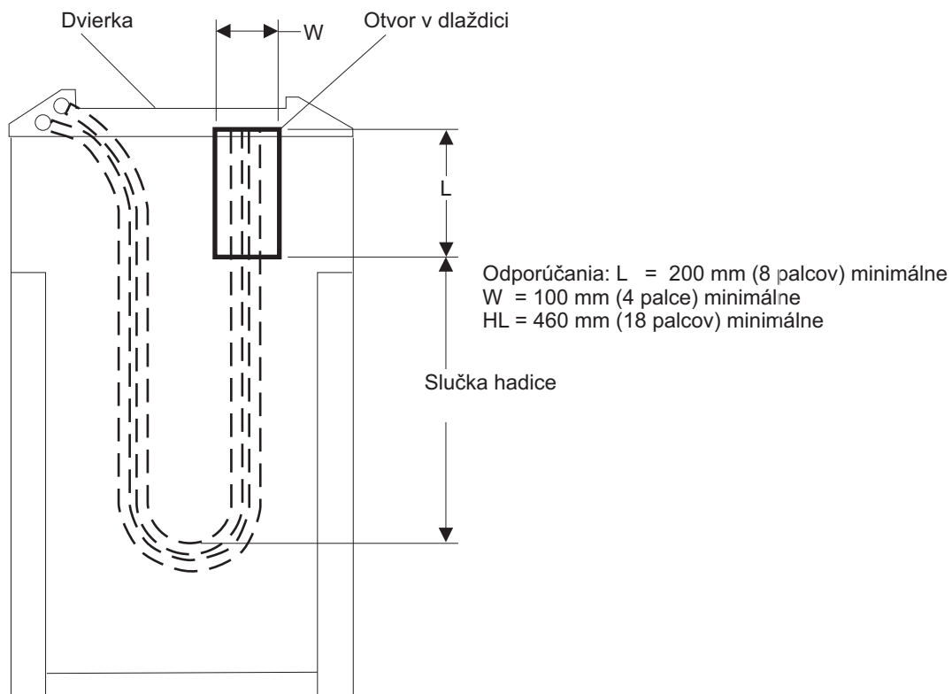
Predok 24-palcového stojana (pohľad zhora)
