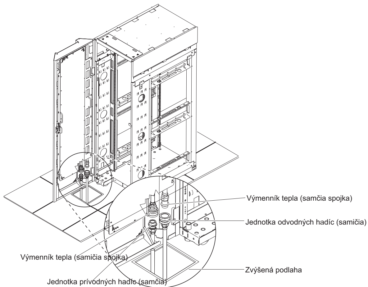
Obrázok 23. Príklad 1: Manažment hadíc pri zvýšenej podlahe; veľkosť otvoru v dlaždici a miesto pre 19-palcové stojany
