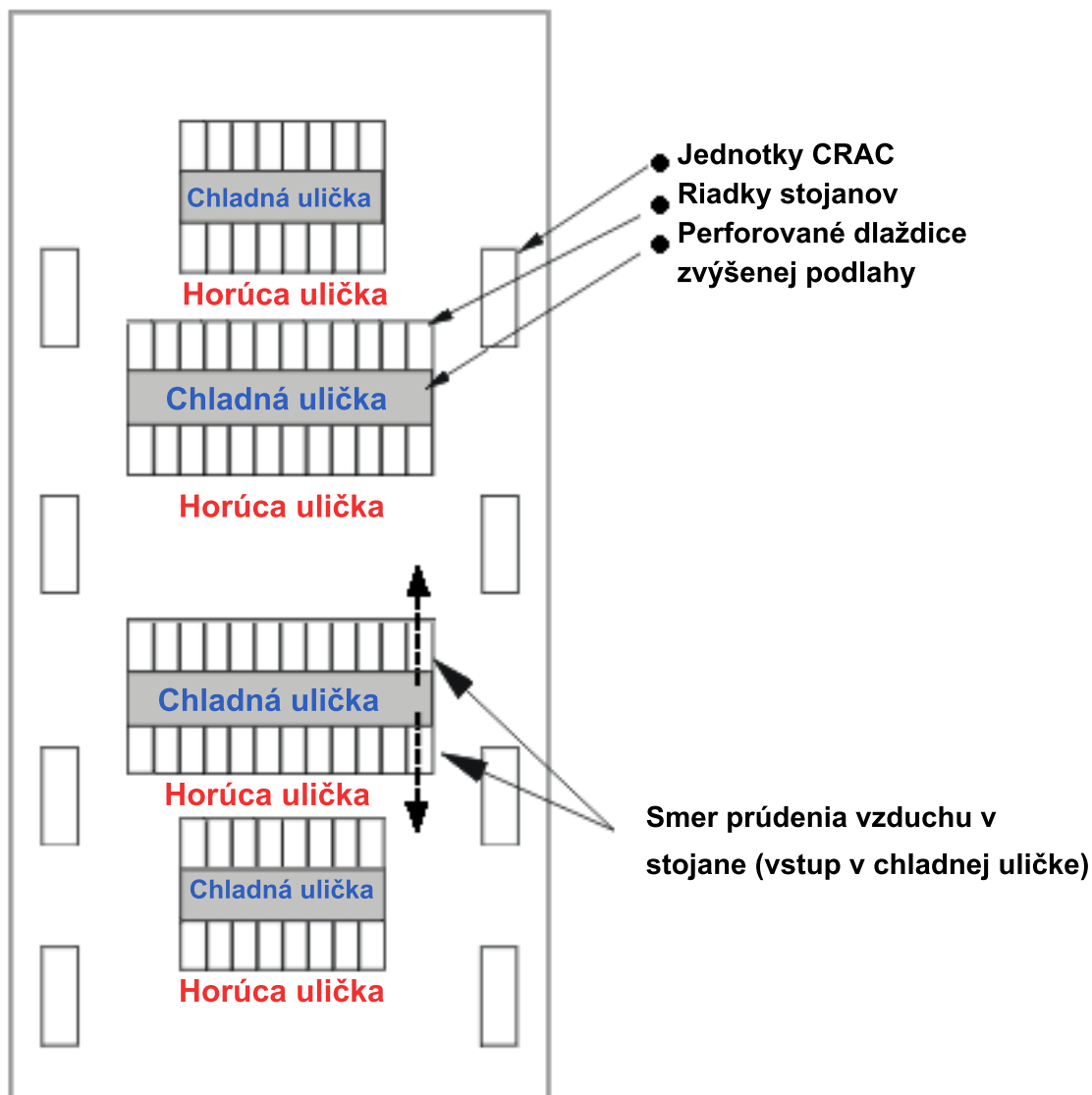
Obrázok 2. Usporiadanie teplých a studených uličiek
