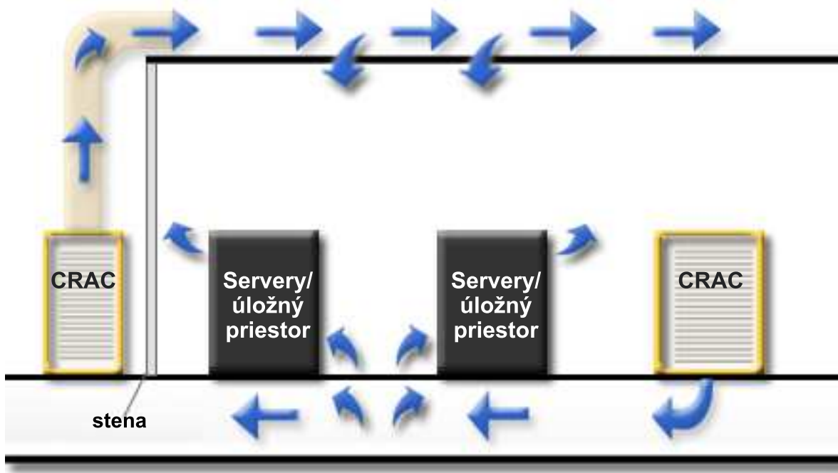
Obrázok 43. Kombinácia stropného a podpodlahového klimatizačného systému
