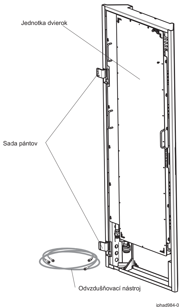
Obrázok 13. Komponenty sady výmenníka tepla pre 24-palcové stojany
