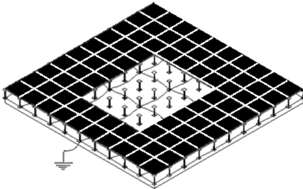
Obrázok 39. Signálová referenčná zem
