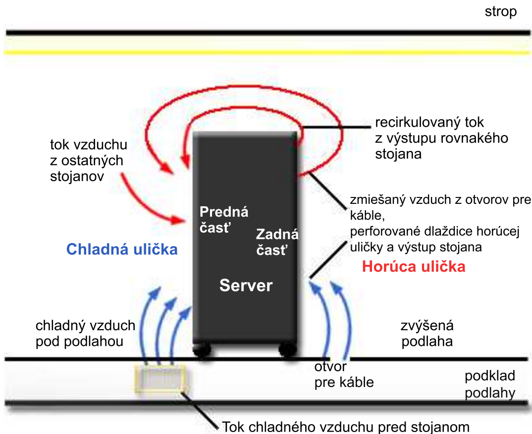
Obrázok 3. Možné vzory prúdenia vzduchu stojana
