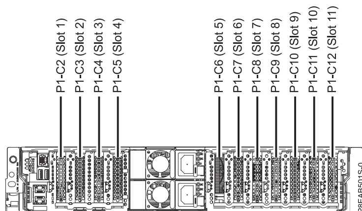
Obrázok 1. Pohľad zozadu na systém 5148-21L, 5148-22L, 8247-21L, 8247-22L, 8284-21A alebo 8284-22A s kódmi umiestnenia slotov PCIe
