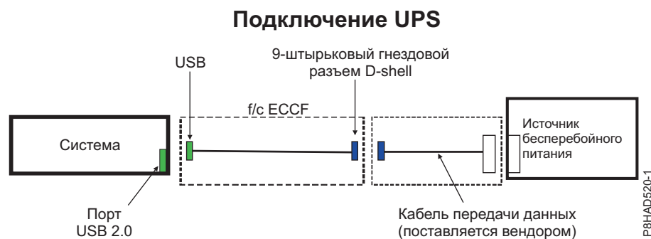
Рисунок 58. Подключение UPS для 5148-21L, 5148-22L, 8247-21L, 8247-22L, 8247-42L, 8284-22A, 8286-41A и 8286-42A
