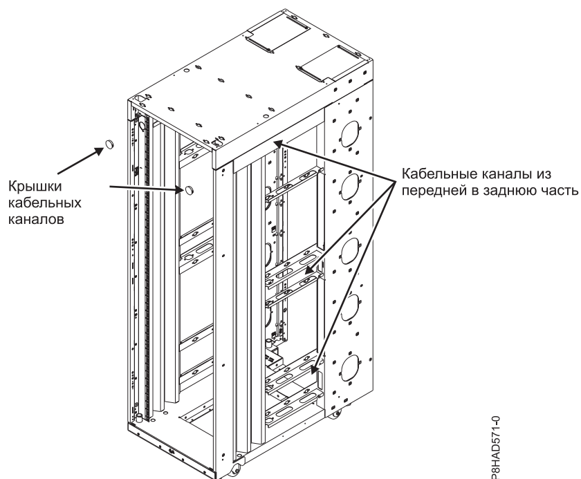
Рисунок 49. Прокладка кабелей внутри стойки
