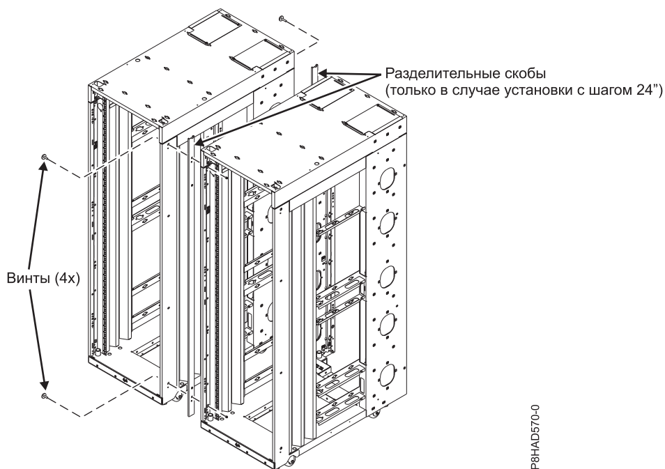
Рисунок 52. Подключение нескольких стоек
