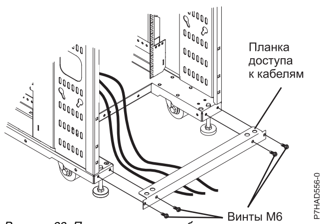
Рисунок 33. Планка доступа к кабелям
