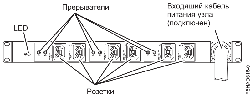
Рисунок 62. HVDC PDU
