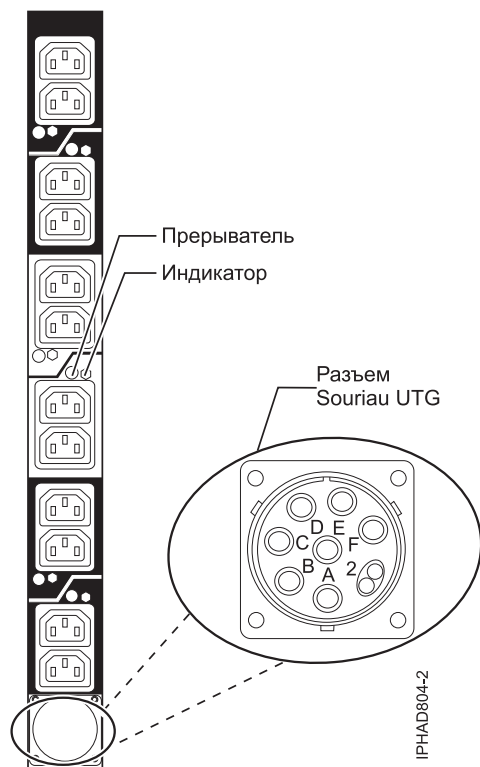
Рисунок 60. Розетка PDU
