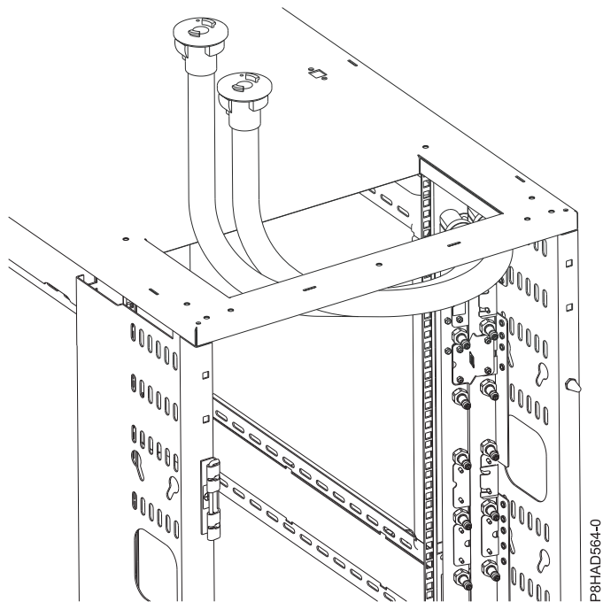
Рисунок 42. Выходные отверстия для шланга сверху
