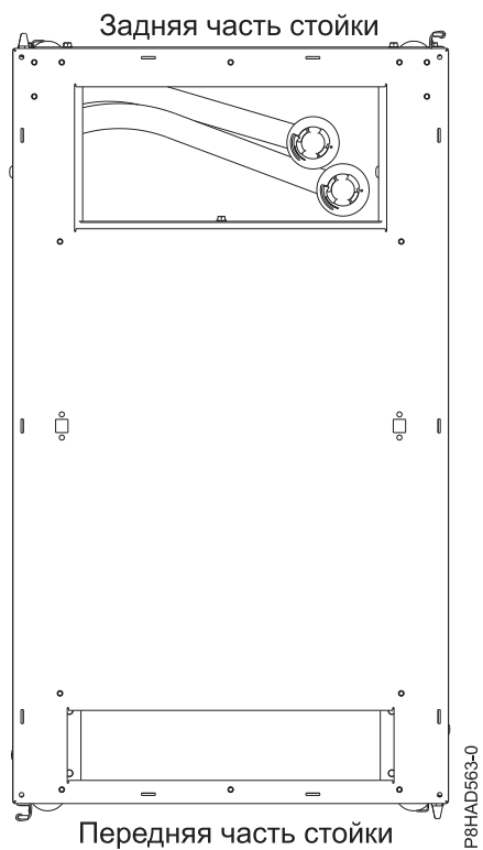
Рисунок 43. Выходные отверстия для шланга сверху (если смотреть сверху)
