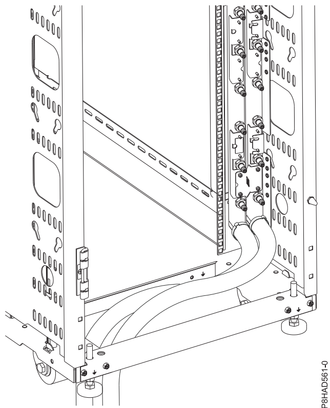
Рисунок 44. Выходные отверстия для шланга снизу
