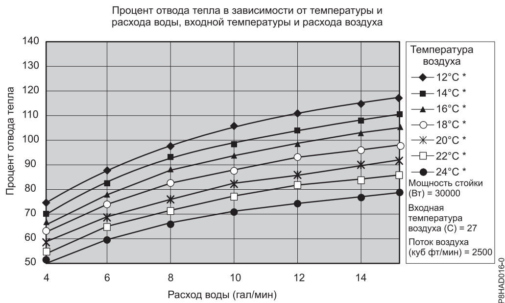
Рисунок 54. Типичная характеристика теплообменника, тепловая нагрузка 30 кВт
