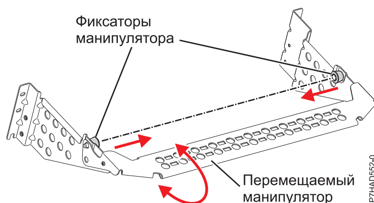
Рисунок 65. Кронштейн управления кабелями
