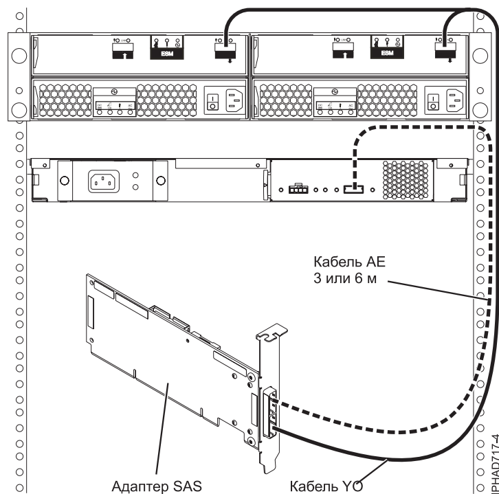
Рисунок 74. Подключение адаптера SAS одновременно и к блоку расширения для дисков, и к блоку расширения для внешних накопителей
