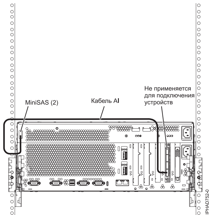
Рисунок 77. Адаптер FC5904 или FC5908, подключенный к блокам расширения диска
