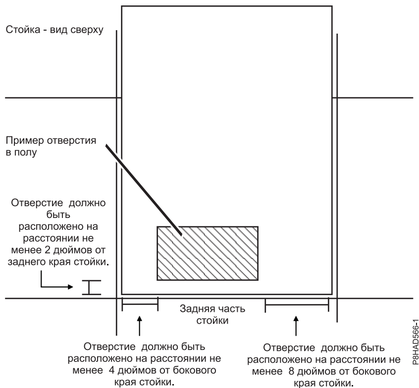
Рисунок 47. Отверстие в полу
