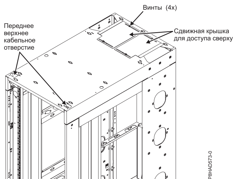
Рисунок 51. Подвесные кабели
