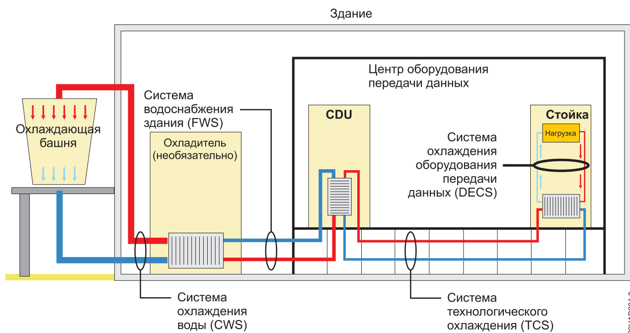
Рисунок 87. Пример контуров и жидкостных систем охлаждения в центре обработки данных
