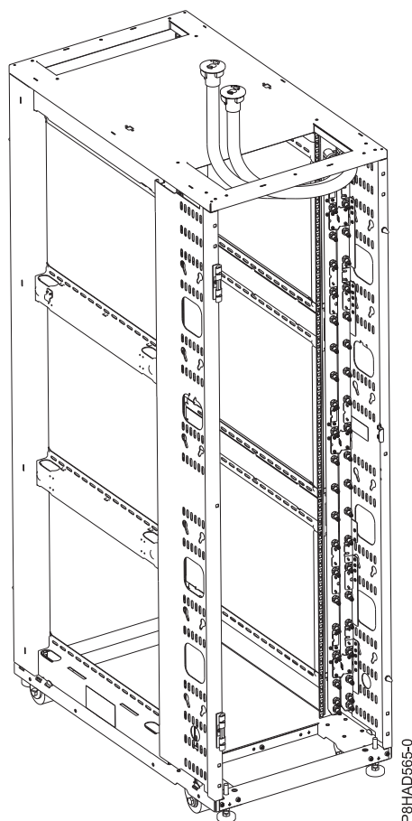
Рисунок 40. Коллектор со шлангами подачи и отвода воды, выходящими через верхнюю часть стойки
