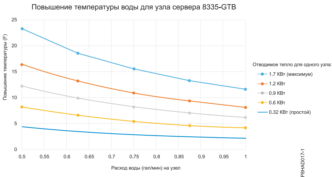
Рисунок 4. Расход воды в зависимости от температуры подаваемой воды - один сервер (стандартные единицы)
