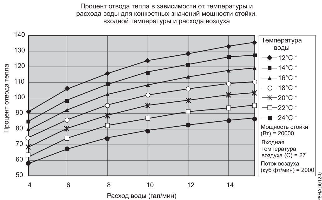
Рисунок 53. Типичная характеристика теплообменника, тепловая нагрузка 20 кВт
