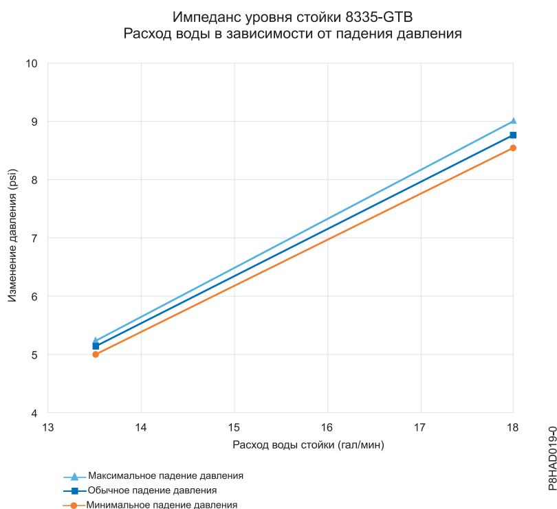
Рисунок 3. Отношение скорости потока и перепада давления (стандартные единицы) - стойка, содержащая 18 серверов
