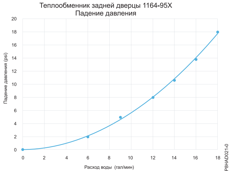
Рисунок 55. Перепад давления (стандартные единицы)
