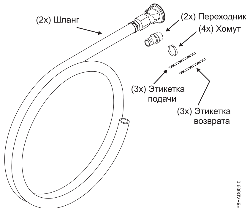
Рисунок 46. Комплект рукава
