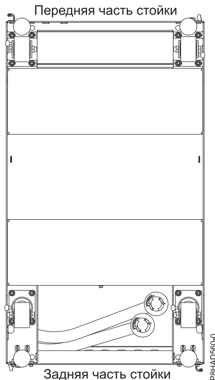
Рисунок 45. Выходные отверстия для шланга снизу (если смотреть снизу)
