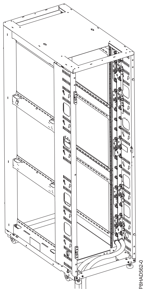
Рисунок 41. Коллектор со шлангами подачи и отвода воды, выходящими через нижнюю часть стойки
