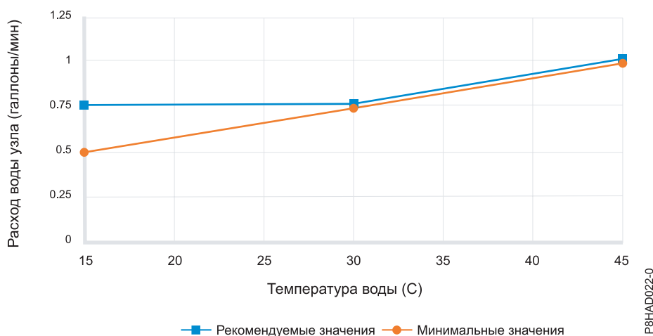
Рисунок 2. Расход воды в зависимости от требований к подаваемой воде (стандартные единицы)
