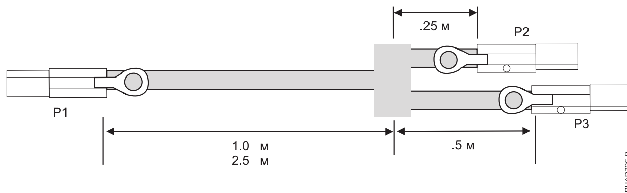
Рисунок 68. Длины внешних кабелей YI SAS
