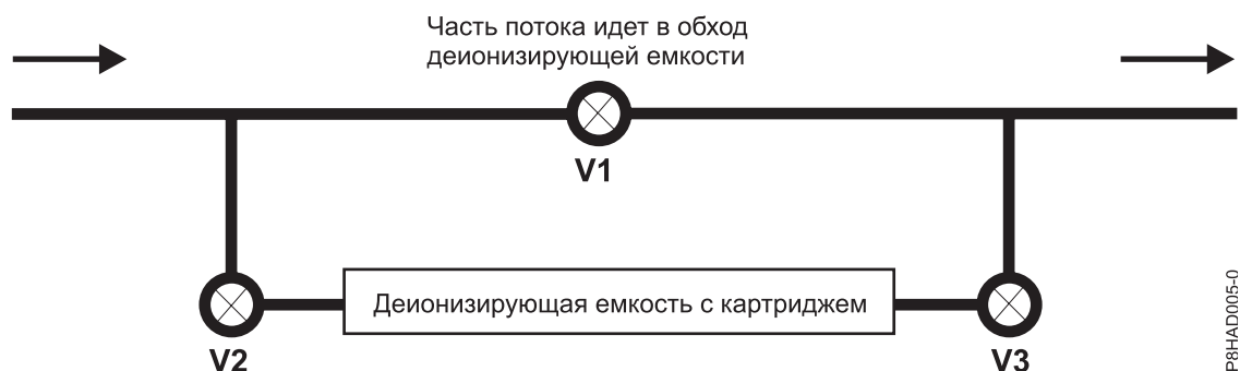
Рисунок 88. Деионизация воды с помощью деионизирующих картриджей, установленных в охлаждающем контуре
