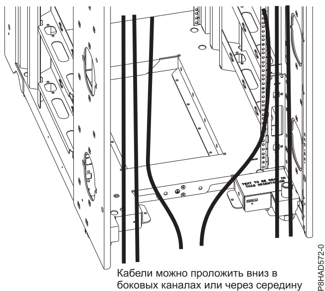
Рисунок 50. Прокладка кабелей под полом
