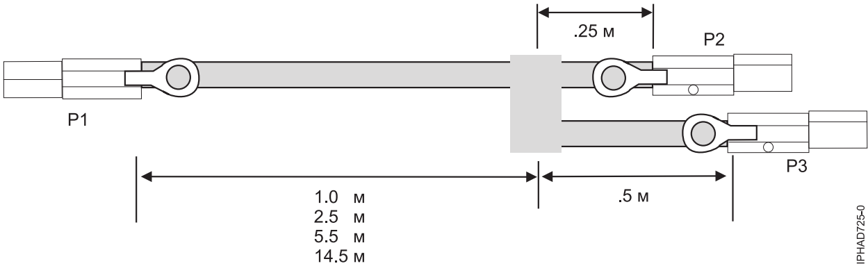
Рисунок 67. Длины внешних кабелей YO SAS
