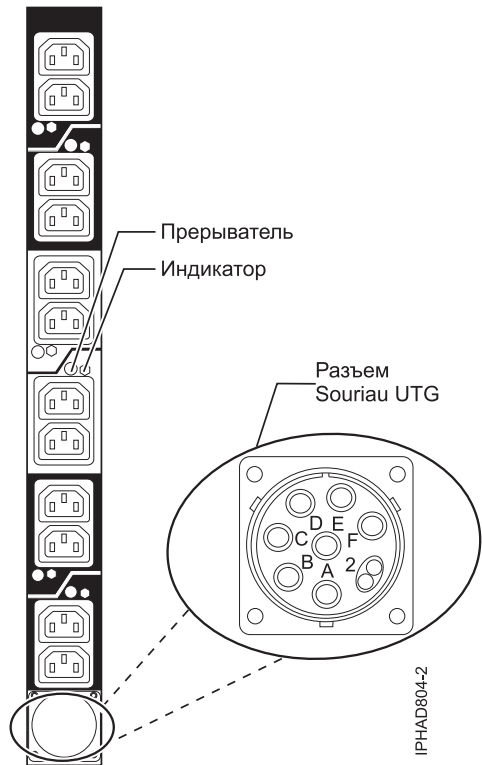
Рисунок 47. Розетка PDU
