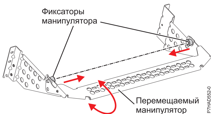
Рисунок 52. Кронштейн управления кабелями
