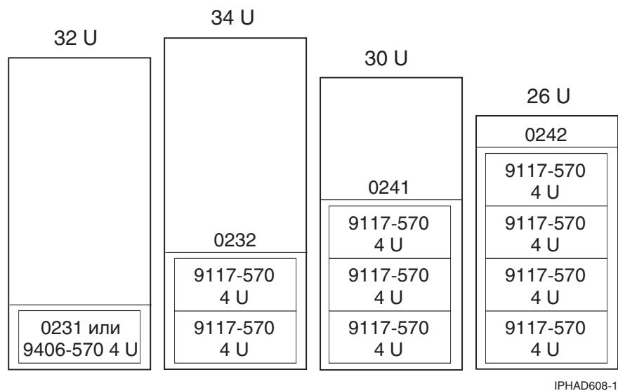
Рисунок 7. 570 в стойке
