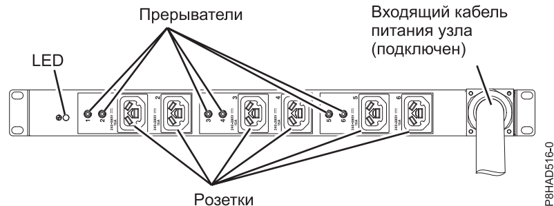
Рисунок 49. HVDC PDU
