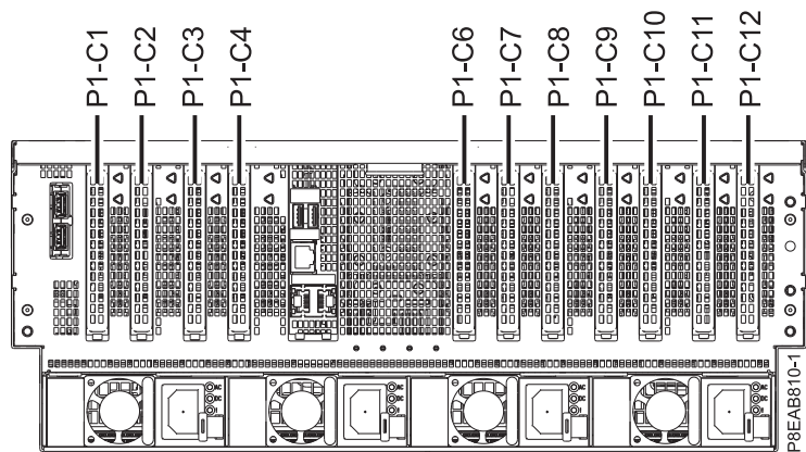
Рисунок 1. Система 8408-44E или 8408-E8E - вид сзади с кодами расположения разъемов PCIe
